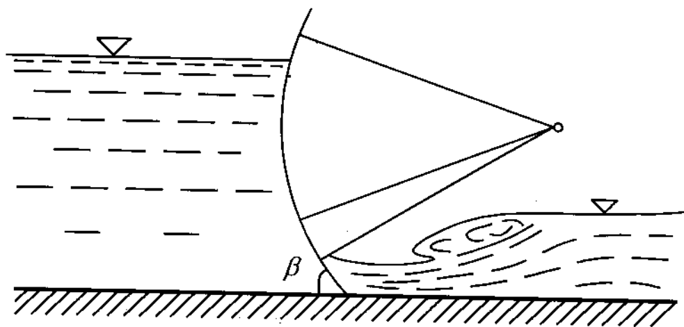
Hình 9-7. Tấm chắn hình cung
