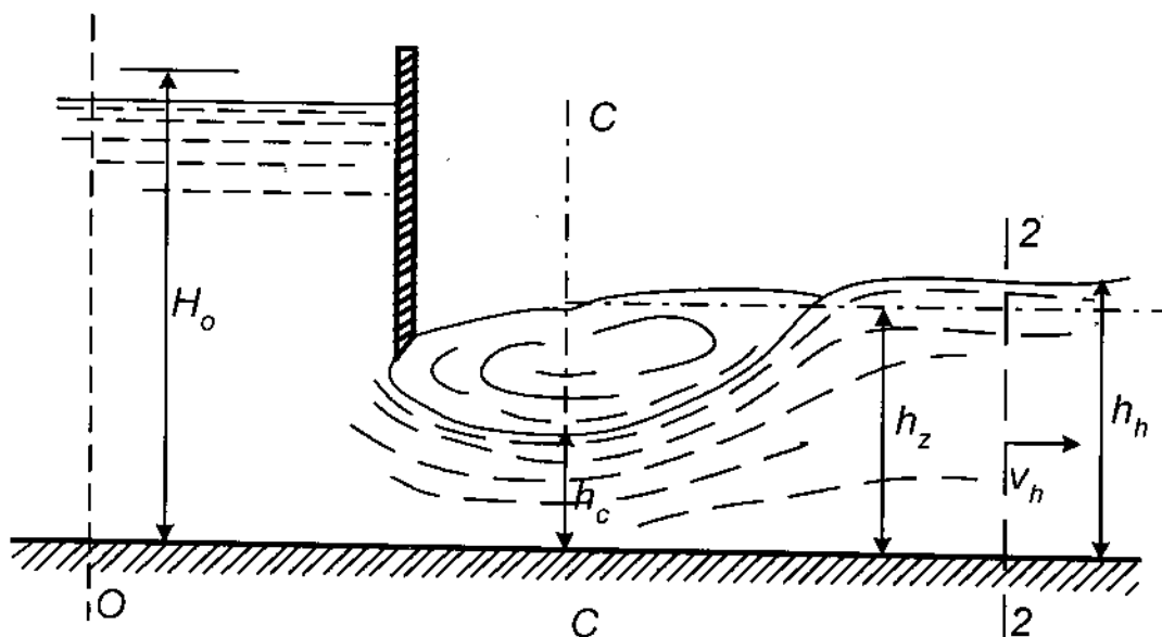
Hình 9- 6. Chảy ngập
