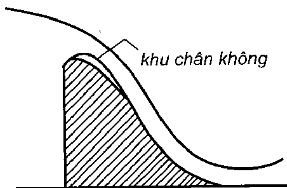
Hình 8-11. Đập tràn mặt cong
