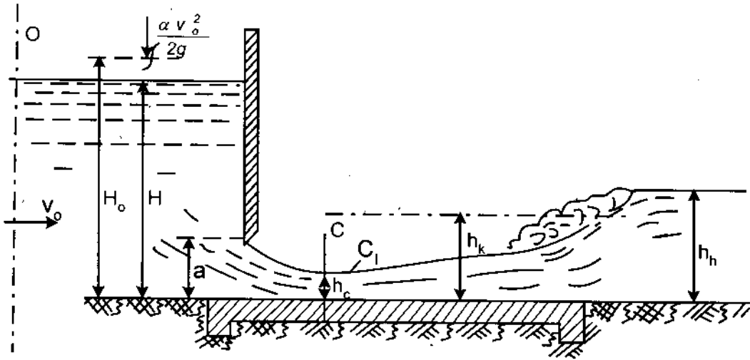
Hình 9-3. Dòng chảy dưới tấm chắn của cổng hở
