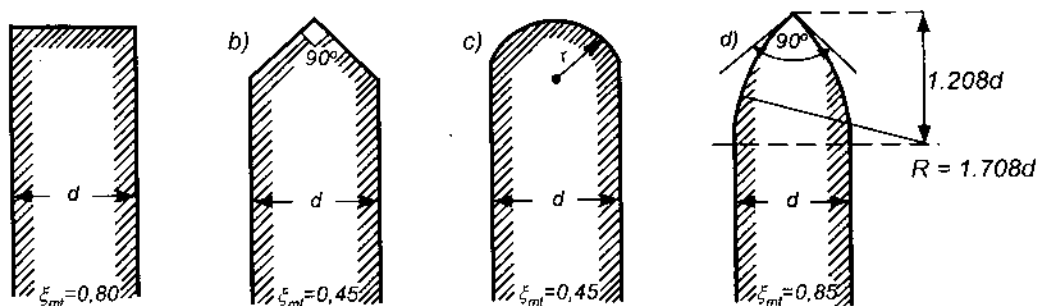
Hình 8-13. Hệ số hình dạng của mố trực
