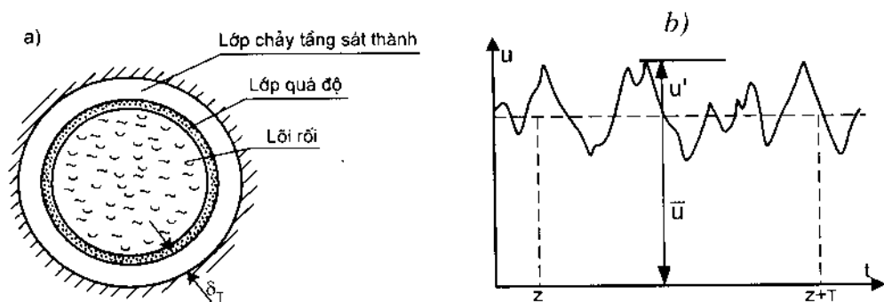
Hình 4-3. a) Mặt cắt ngang dòng chảy rối trong ống tròn
