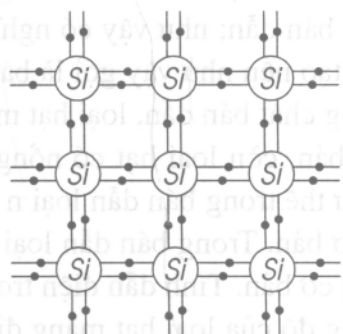
Hình 5 - 1 (b) Mạng tinh thể silic
