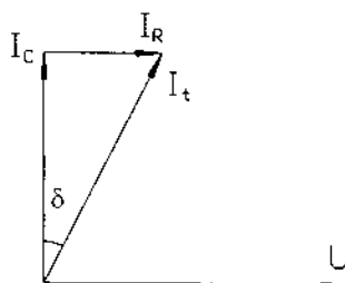
Hình 2-3. Đồ thị vectơ dòng điện và điện áp
