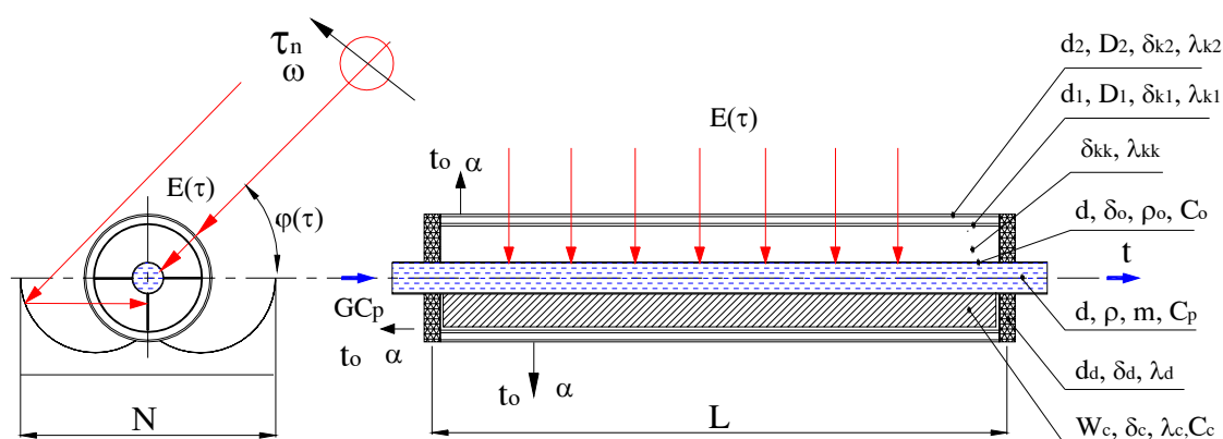
Hình 4.16. Kết cấu bộ thu dạng ống có gương phản xạ parabol trụ loại đặt nghiêng
