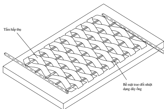
Hình 4.6. Dải tấm hấp thụ được đan xen vào bề mặt hấp thụ dạng dây ống
