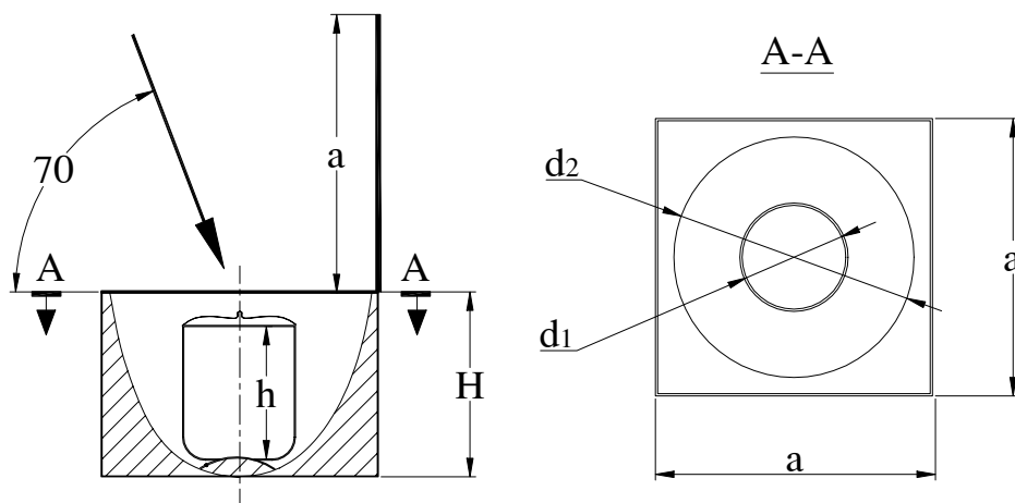
Hình 4.2. Kích thước của bếp
