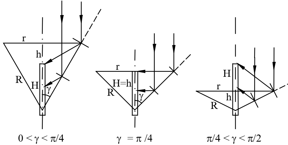
Hình 5.6. Gương nón với mặt thu hình ống trụ
