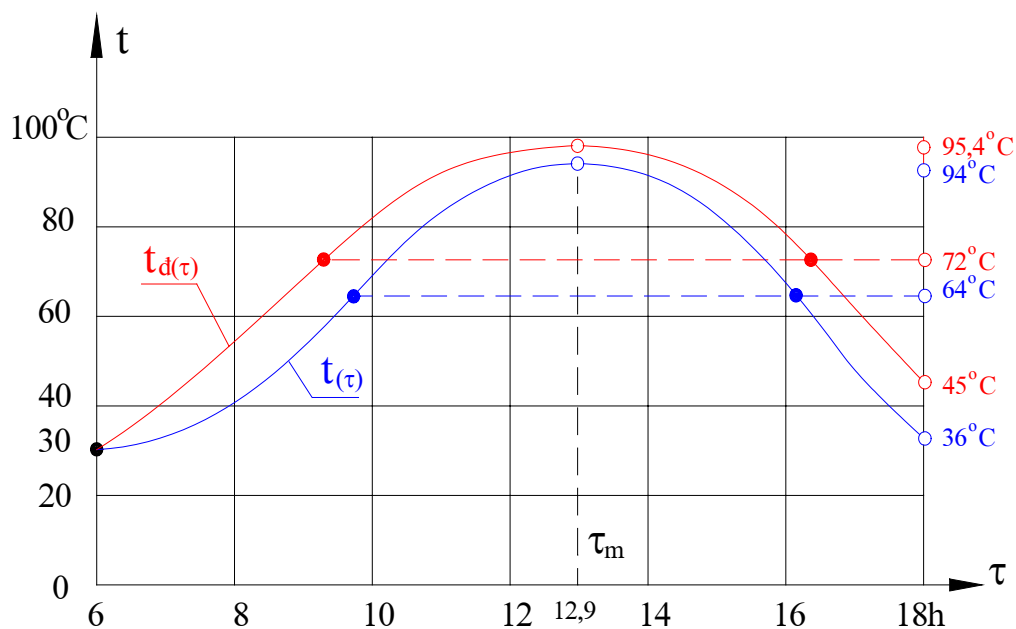
Hình 4.9. Hàm nhiệt độ khí tĩnh t(\tau) và khí động t_d(\tau) của panel 1\text{m}^2 có W > W_s
