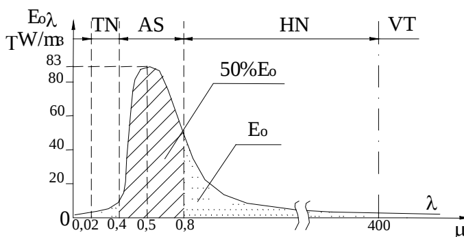
Hình 2.4. Phân bố E_{0\lambda}(\lambda) của mặt trời
