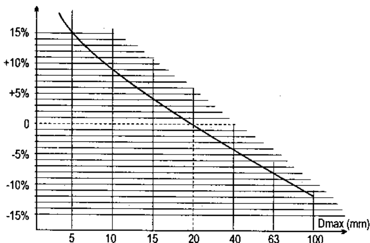
Hình 4-2. Biểu đồ xác định lượng nước điều chỉnh.
