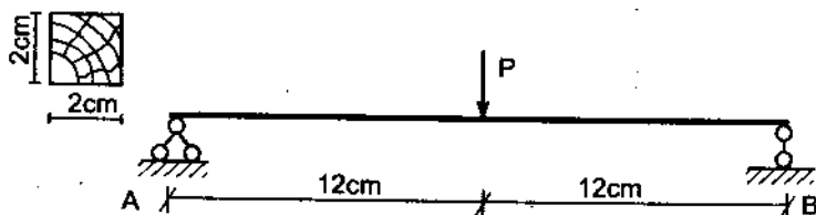
Hình 7-3. Sơ đồ thí nghiệm uốn gỗ
