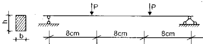
Hình 1-1. Sơ đồ làm việc của mẫu thí nghiệm
