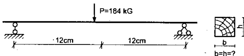
Hình 7-5. Sơ đồ thí nghiệm khả năng chịu uốn của gỗ
