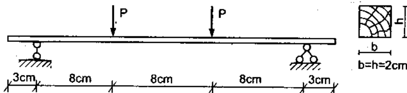
Hình 7-4. Sơ đồ thí nghiệm khả năng chịu uốn của gỗ
