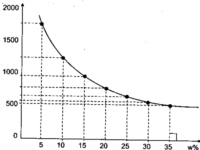
Hình 7-7. Biểu đồ quan hệ R_u và W\% .
