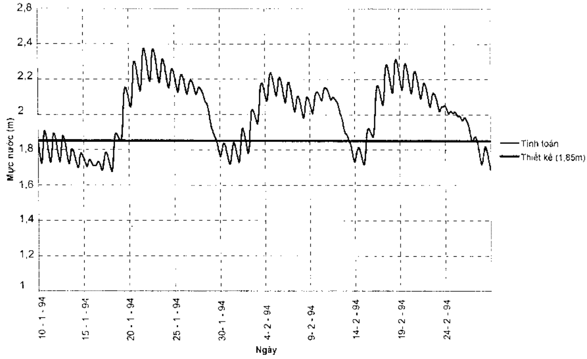
Quá trình mực nước tại Xuân Quan từ ngày 10 tháng 1 đến 28 tháng 2 năm 1994 kịch bản HB3b – Hồ Hoà Bình điều tiết theo yêu cầu cấp nước hạ du
