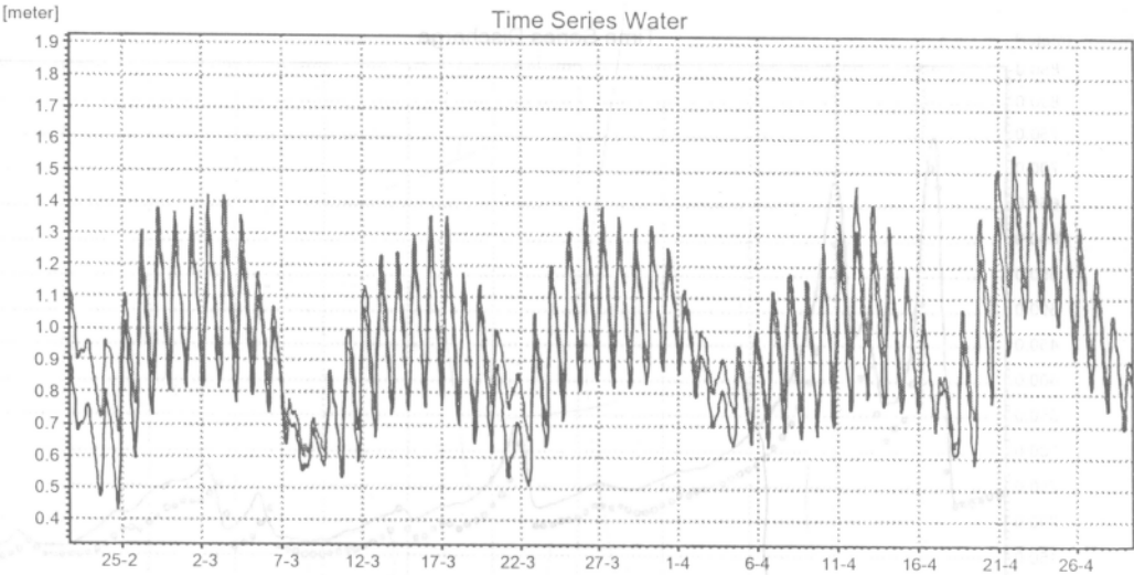
Hình 3.12.7. Tại trạm Phả Lại trên sông Thái Bình (2003)
