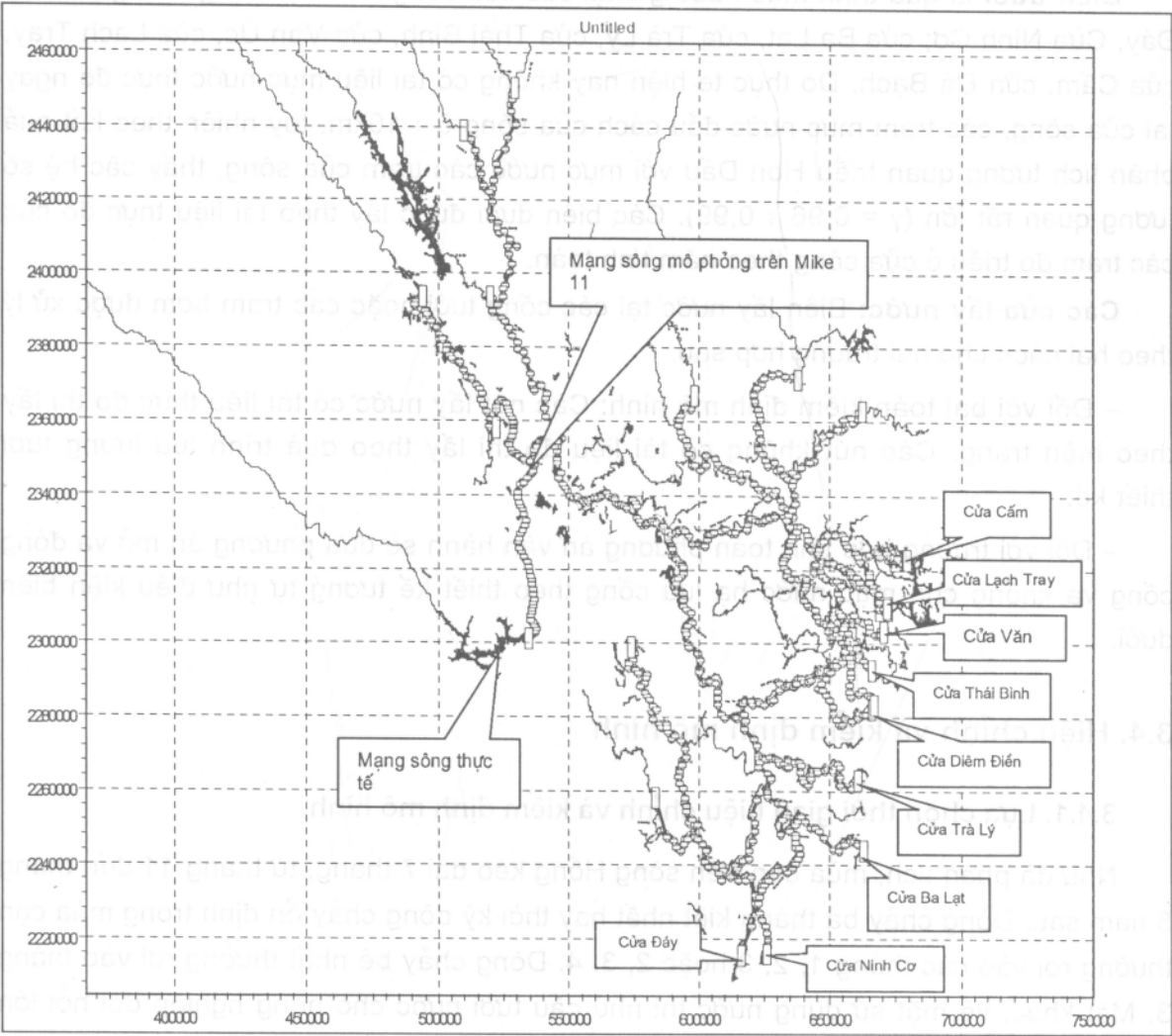
Hình 3.9. Sơ đồ mạng thủy lực sông Hồng – sông Thái Bình và hệ thống biên trên – dưới mô phỏng trên mô hình Mike11 theo hệ tọa độ VN2000
