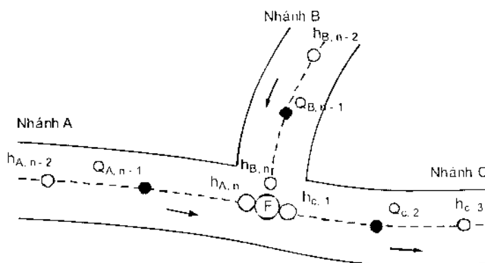
Hình 3.5. Cấu hình các điểm lưới xung quanh điểm mà tại đó ba nhánh gặp nhau
