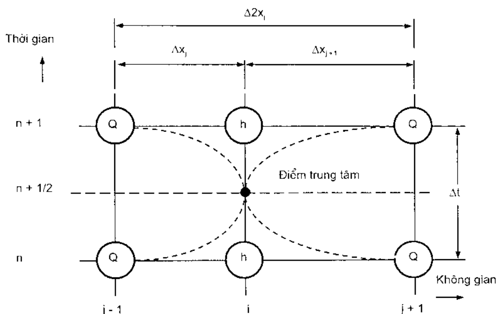
Hình 3.2. Sơ đồ sai phân 6 điểm cho phương trình liên tục
