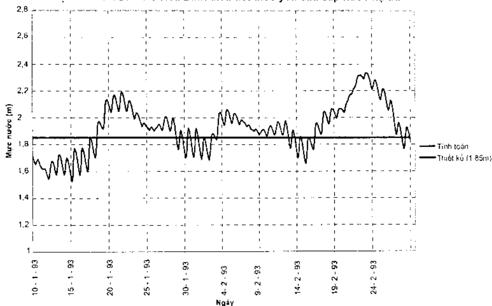
Quá trình mực nước tại Xuân Quan từ ngày 10 tháng 1 đến 28 tháng 2 năm 1993 kịch bản HB2b – Hồ Hoà Bình điều tiết theo yêu cầu cấp nước hạ du
