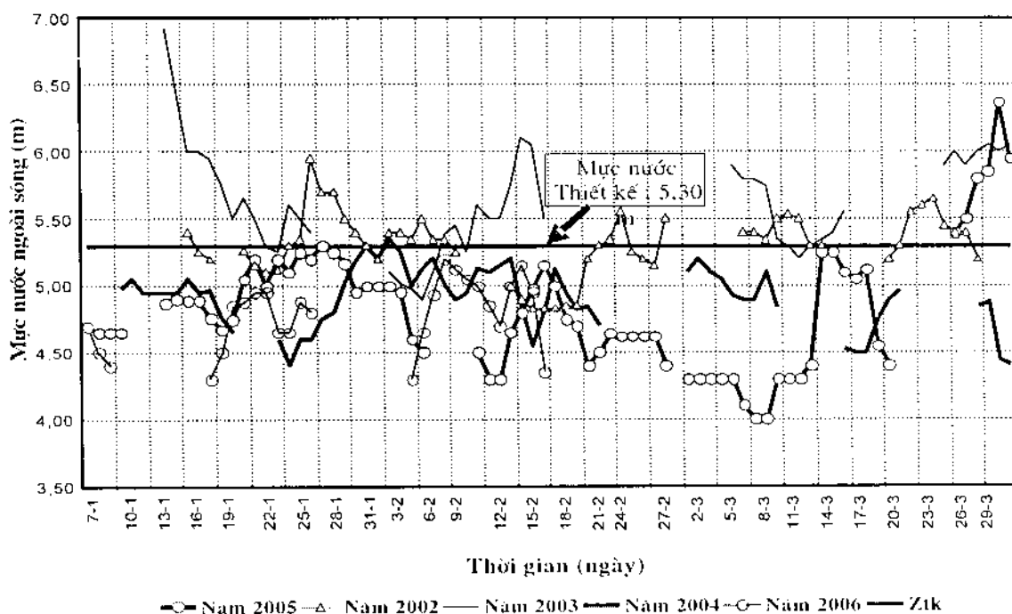
Diễn biến mực nước sông Hồng tại cửa lấy nước Phù Sa - Hà Tây (Từ 7/1 đến 31/3 các năm 2002 - 2006)
