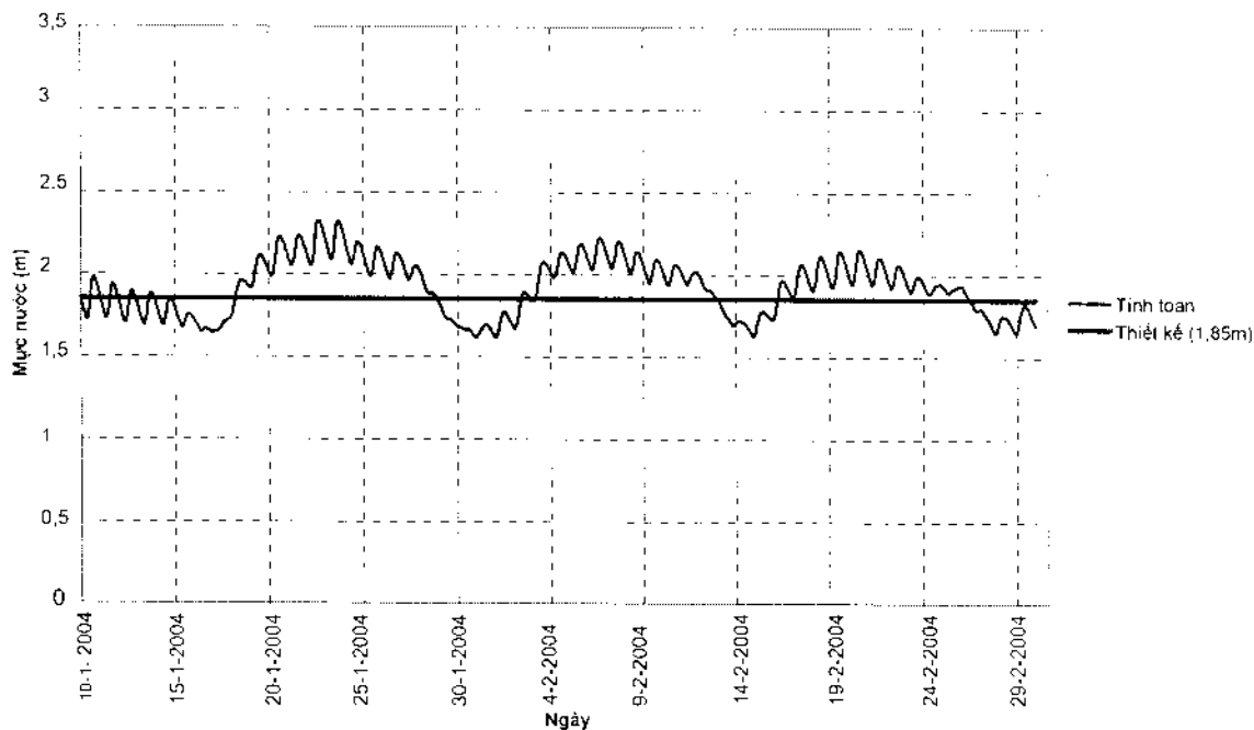
Quá trình mực nước tại Xuân Quan từ ngày 10 tháng 1 đến 28 tháng 2 năm 2004 kịch bản HB5b – Hồ Hoà Bình điều tiết theo yêu cầu cấp nước hạ du
