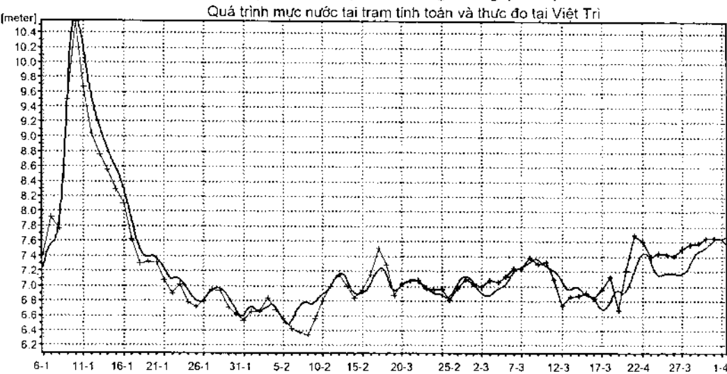
Hình 3.12.2. Tại trạm Việt Trì trên sông Hồng (2003)
