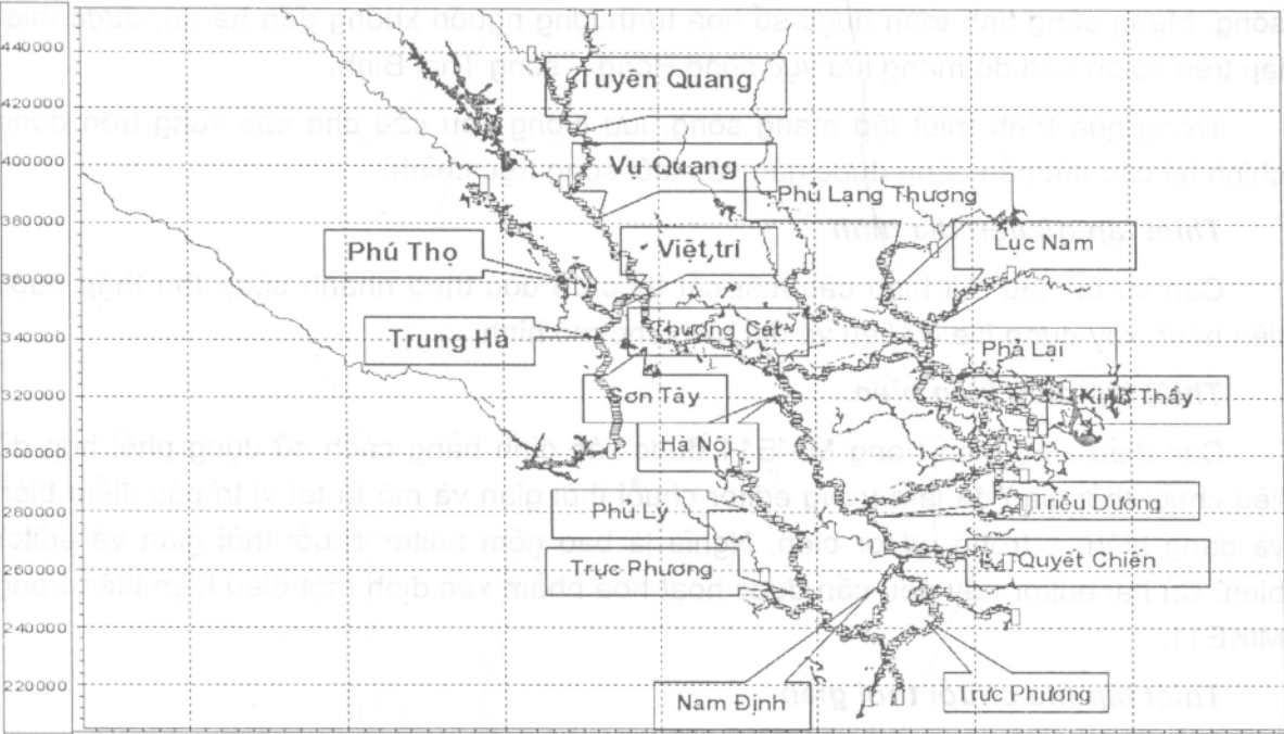
Hình 3.10. Hệ thống nút kiểm tra để kiểm định và xác định thông số mô hình
