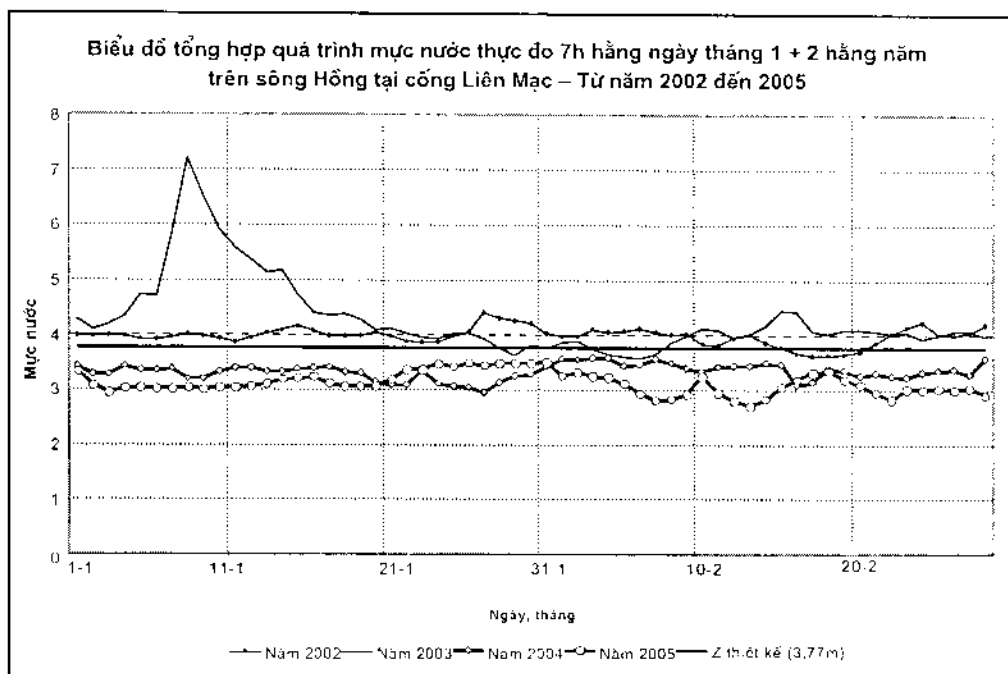
Hình 2.5. Quá trình mực nước sông Hồng tháng 1 + 2 tại cống Liên Mạc từ năm 2002 đến năm 2005 (theo tài liệu mực nước thực đo 7h hằng ngày)
