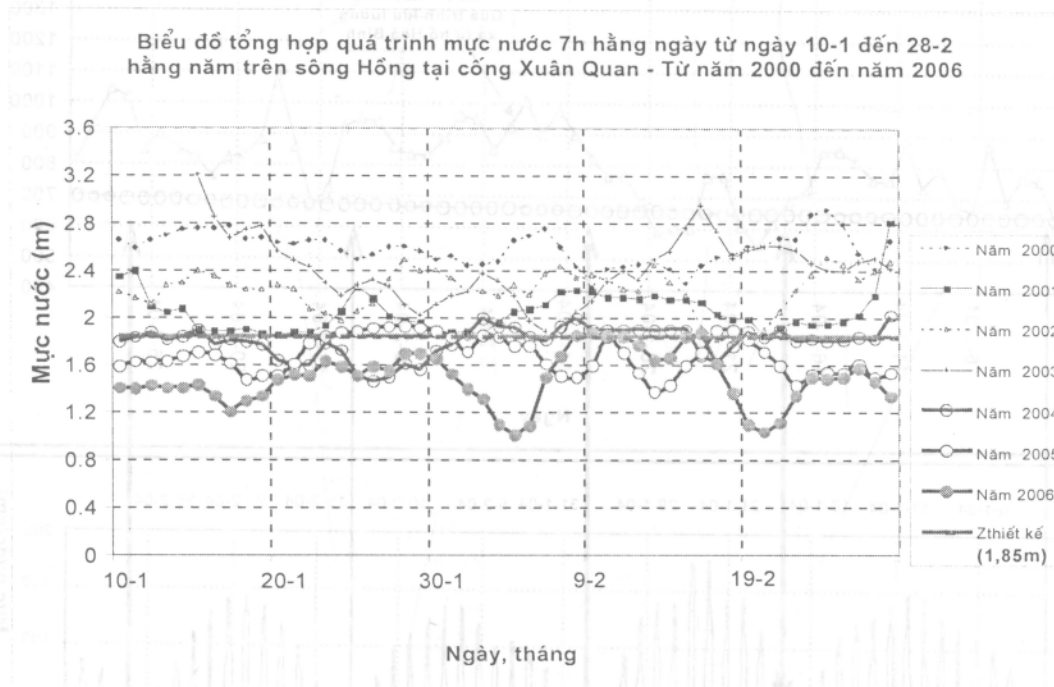
Hình 2.6. Quá trình mực nước sông Hồng tháng 1 + 2 tại cống Xuân Quan từ năm 2000 đến năm 2006 (theo tài liệu mực nước thực đo 7h hằng ngày)
