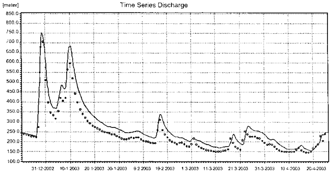
Hình 3.12.10. Tại trạm Gềnh Gà trên sông Lô
