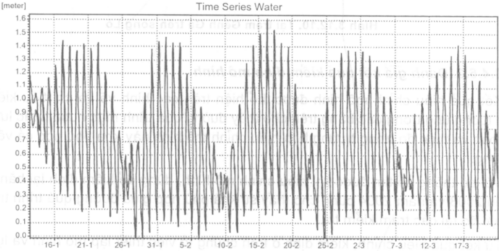
Hình 3.12.8. Tại trạm Quyết Chiến trên sông Trà Lý (2003)
