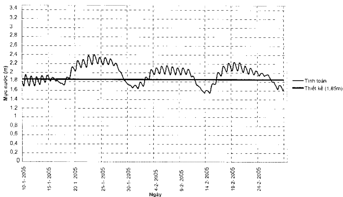
Quá trình mực nước tại Xuân Quan từ ngày 10 tháng 1 đến 28 tháng 2 năm 2005 kịch bản HB6b – Hồ Hoà Bình điều tiết theo yêu cầu cấp nước hạ du
