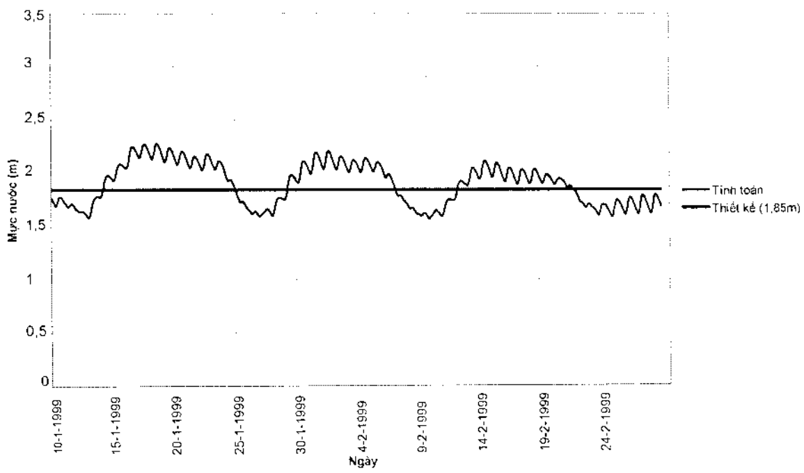
Quá trình mực nước tại Xuân Quan từ ngày 10 tháng 1 đến 28 tháng 2 năm 1994 kịch bản HB4b – Hồ Hoà Bình điều tiết theo yêu cầu cấp nước hạ du
