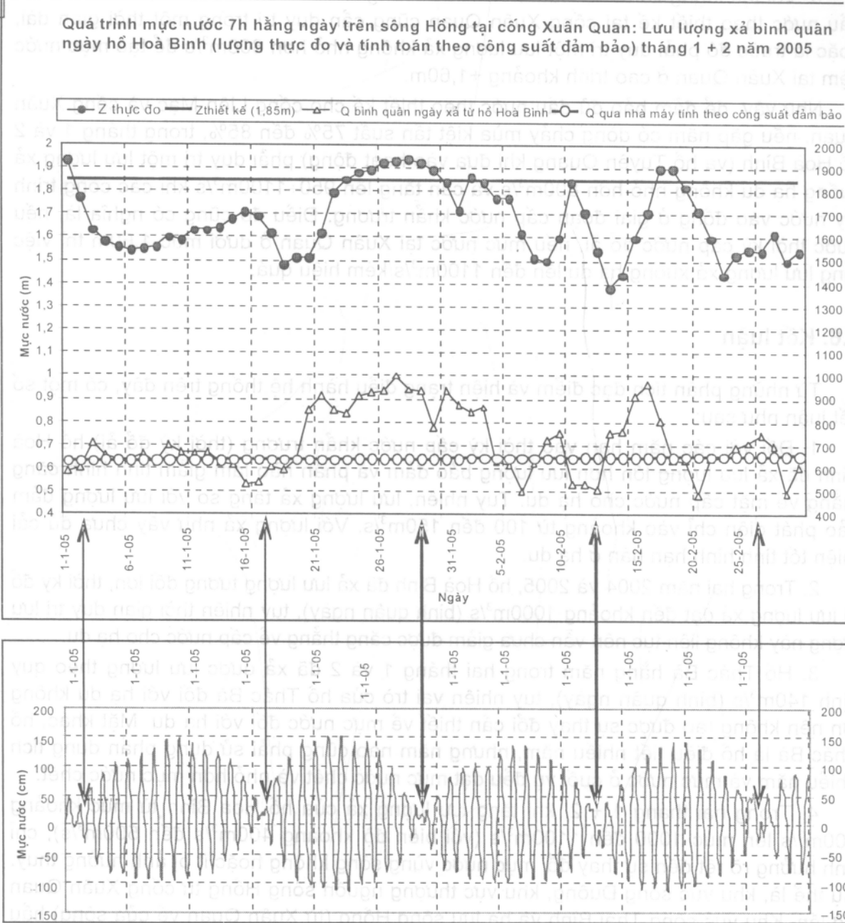
Hình 2.8. Quá trình mực nước tại cửa lấy nước cống Xuân Quan, mực nước triều tại Ba Lạt và quá trình lưu lượng thực đo bình quân ngày xả từ hồ Hoà Bình trong hai tháng 1 + 2 năm 2005
