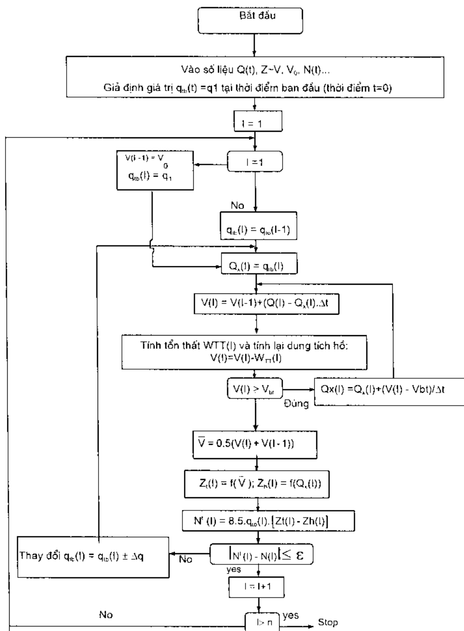
Hình 4.1. Thuật toán tính điều tiết dòng chảy đối với hệ thống hồ độc lập phát điện theo biểu đồ công suất cho trước sử dụng trong chương trình thực nghiệm
