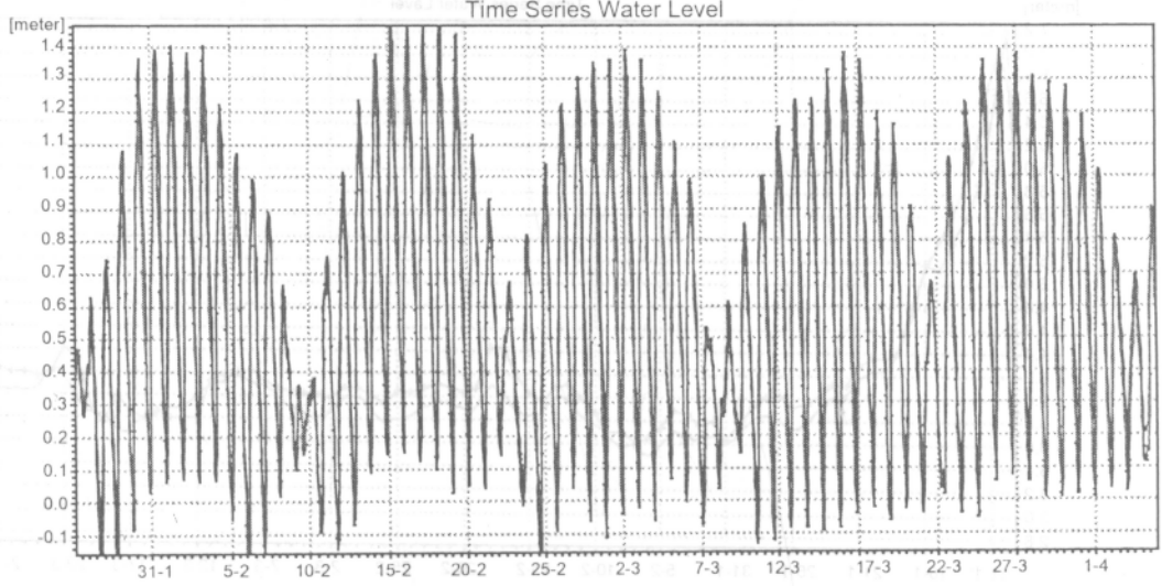
Hình 3.12.6. Tại trạm Chanh Chữ trên sông Luộc (2003)
