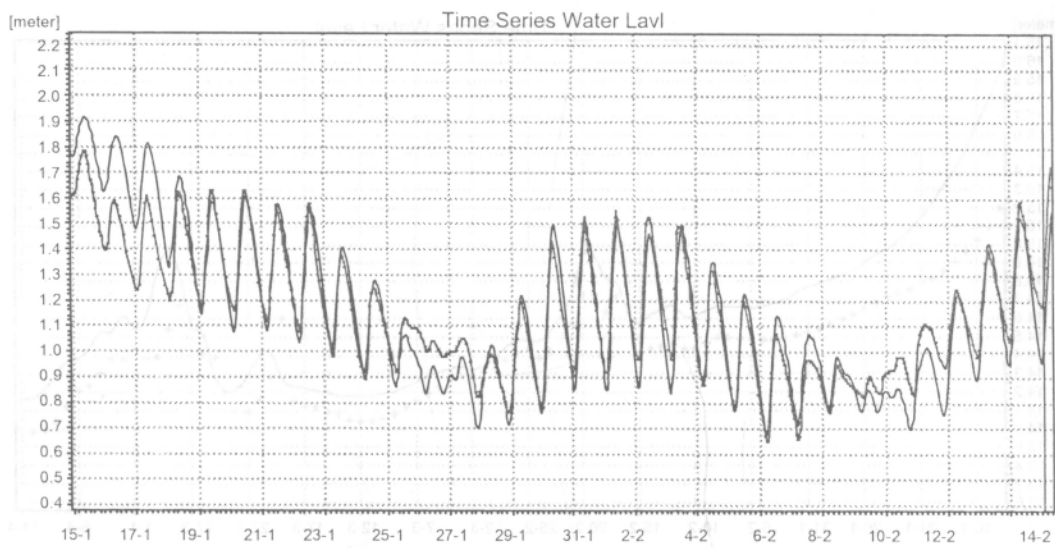
Hình 3.12.4. Tại trạm Hưng Yên trên sông Hồng (2003)
