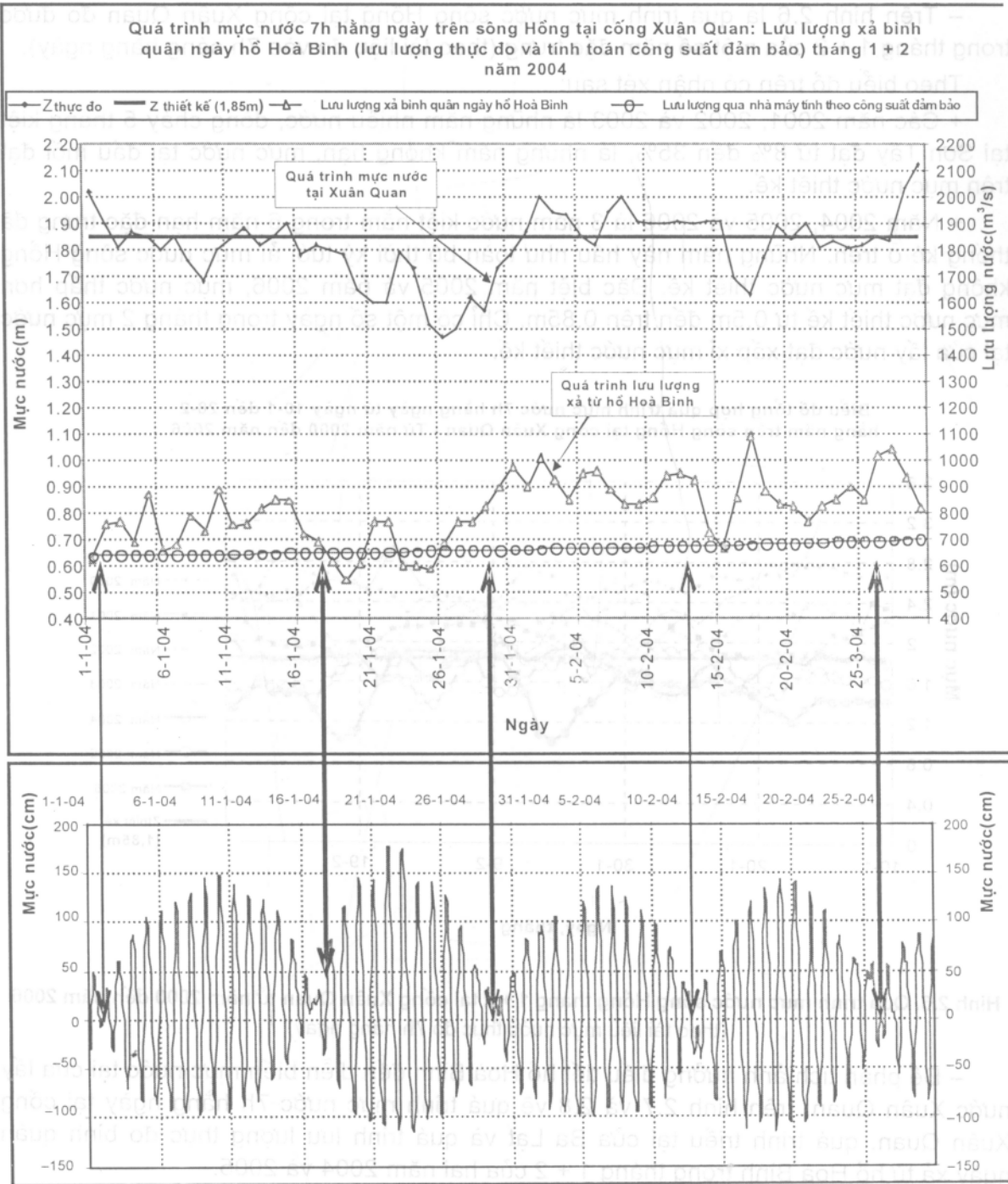
Hình 2.7. Quá trình mực nước tại cửa lấy nước cống Xuân Quan, mực nước triều tại Ba Lạt và quá trình lưu lượng thực đo bình quân ngày xả từ hồ Hoà Bình trong hai tháng 1 + 2 năm 2004
