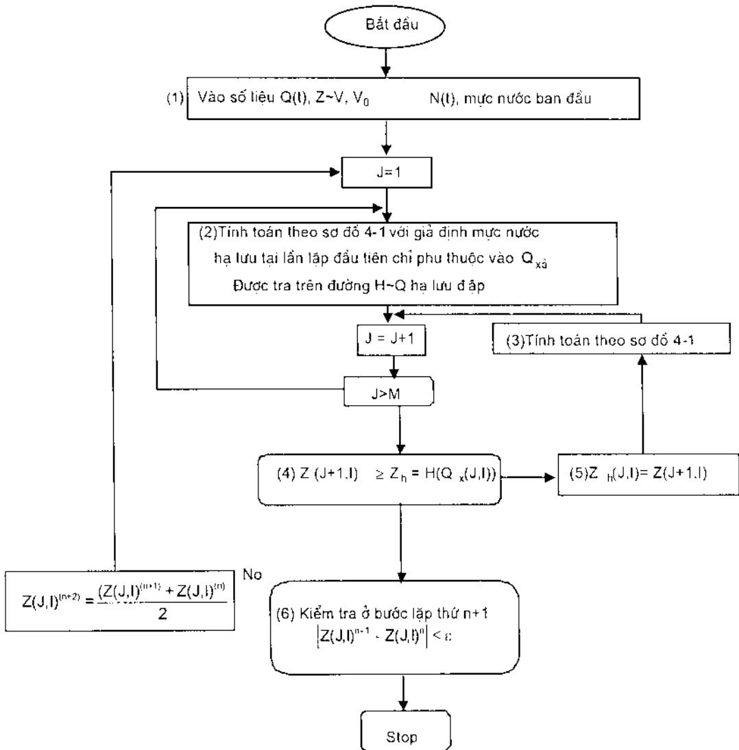
Hình 4.2. Sơ đồ thuật toán tính điều tiết dòng chảy đối với hệ thống hồ bậc thang phát điện theo biểu đồ công suất cho trước sử dụng trong chương trình thực nghiệm
