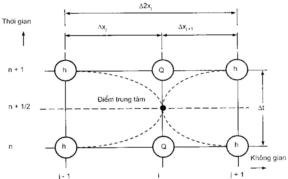
Hình 3.3. Sơ đồ sai phân 6 điểm cho phương trình động lượng
