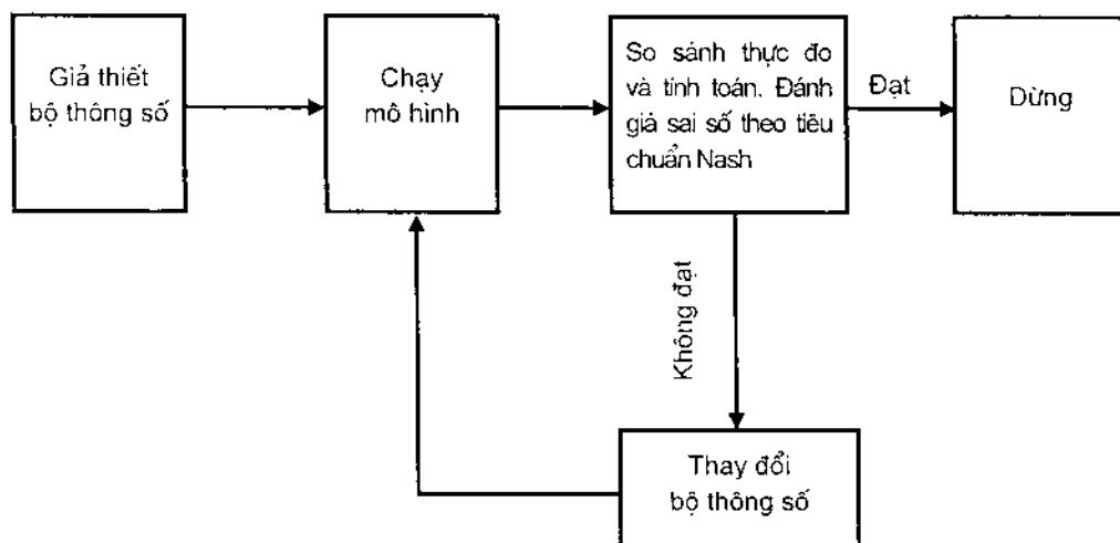
Hình 3.11. Sơ đồ quá trình hiệu chỉnh bộ thông số mô hình
