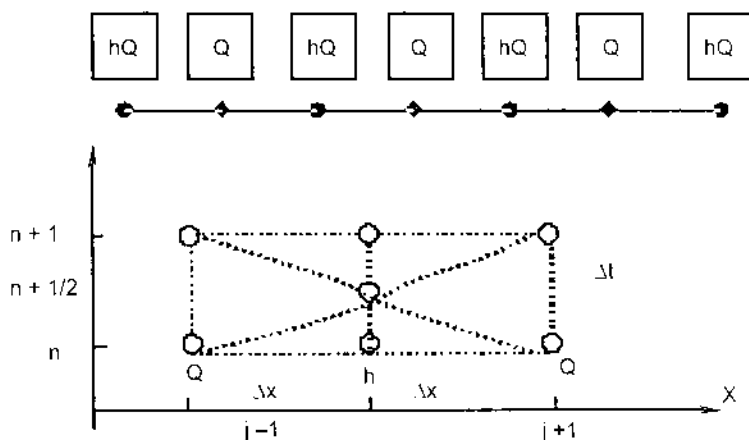
Hình 3.1. Sơ đồ giải
