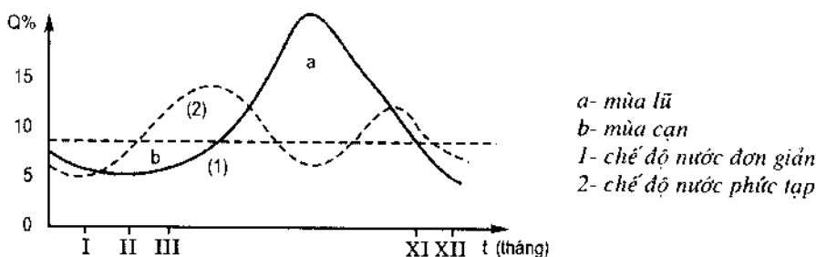
Hình 62 : Các đường Q - t (Biến trình năm của lưu lượng).
