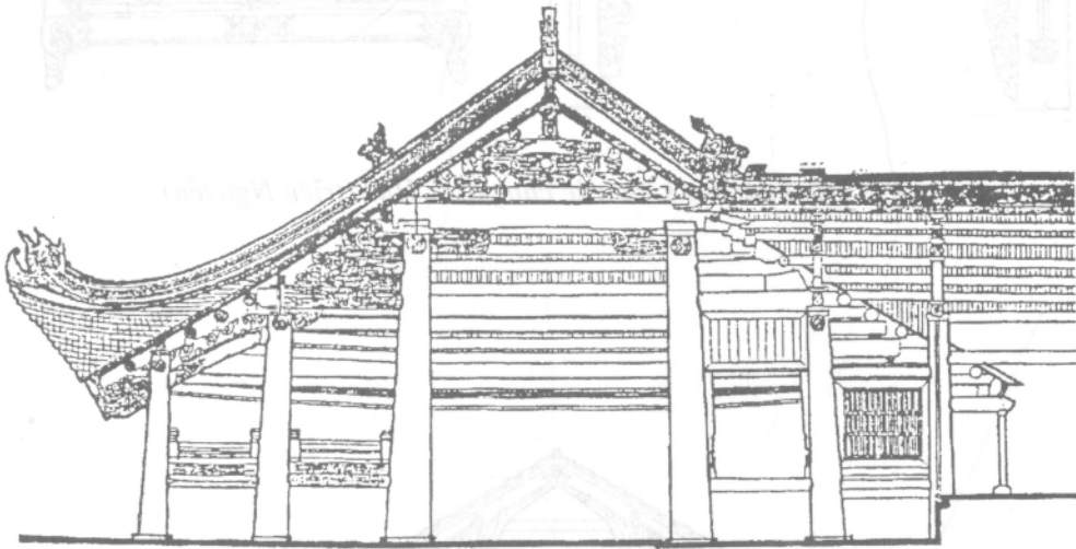
Vì thượng rường - hạ kẻ ở đình Thổ Hà
