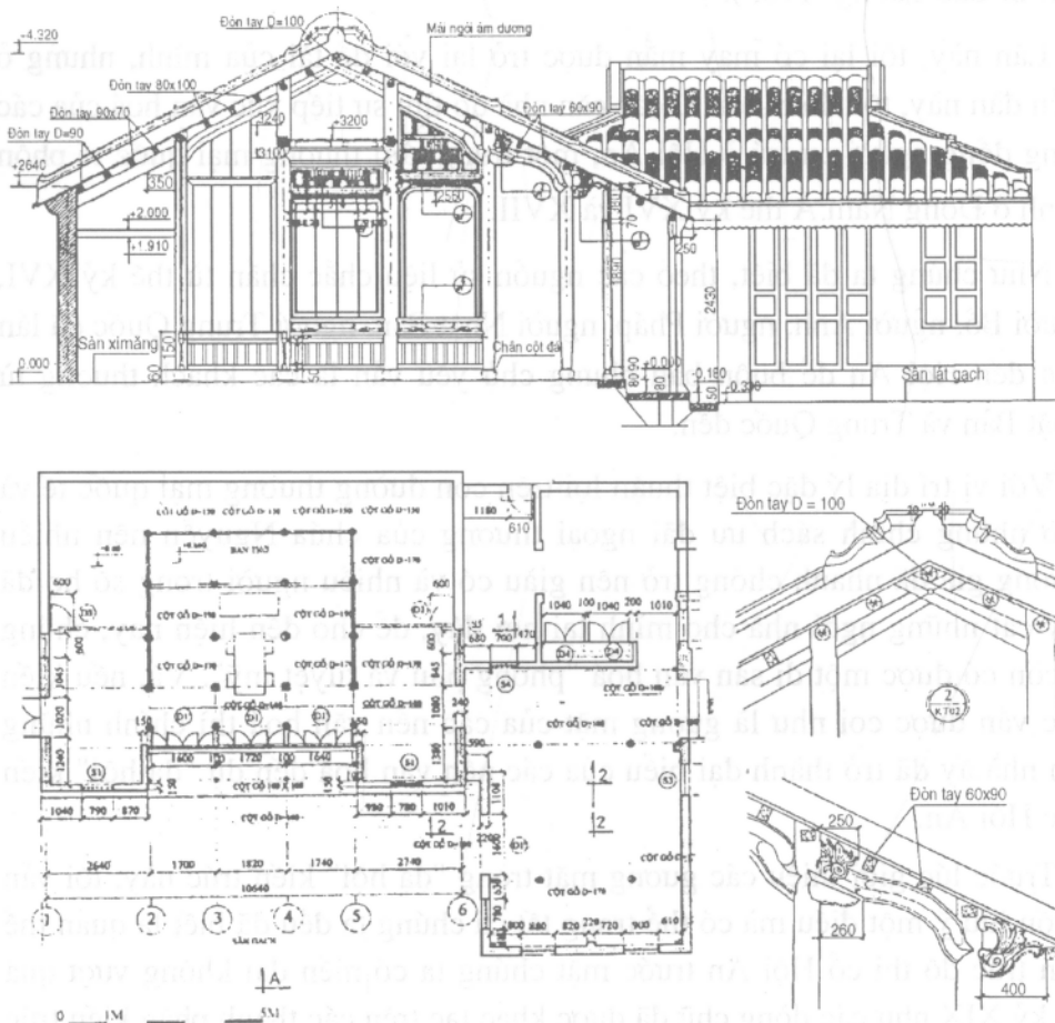
Một bản vẽ nghiên cứu về nhà cổ ở Hội An
