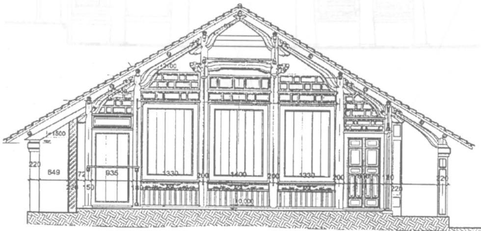
Kèo chống - nhà rường. Nhà ở dân gian ở Quảng Ngãi
