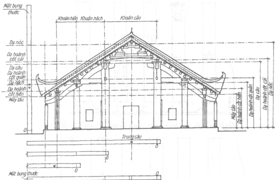
Hình 3. Cách thể hiện các số đo trên mặt lưng và bụng thước
