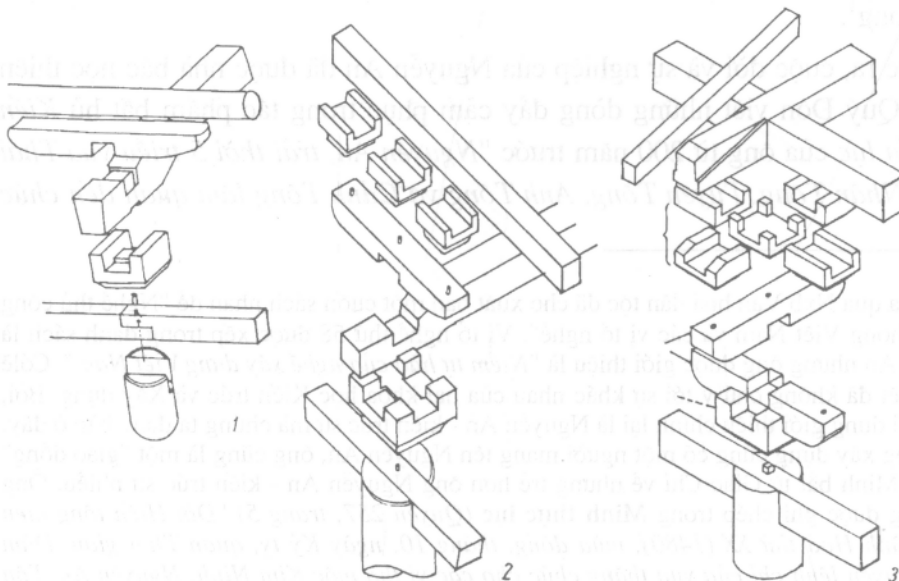
Hình 2. Giải phẫu kết cấu Củng:
