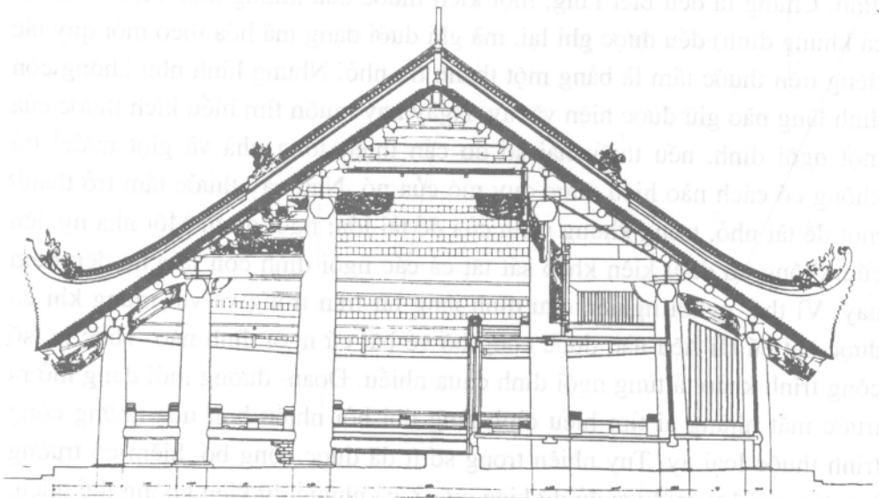
Mặt cắt đình làng Chu Quyến (Hà Tây) Bản vẽ ghi của Lê Đại (HKTSVN)
