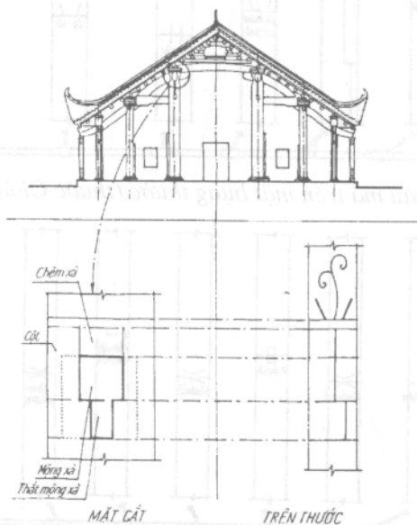
Hình 8. Thể hiện lỗ mộng trên thước
