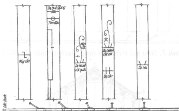
Hình 4. Dấu mã trên mặt bụng thước (thước Chàng Sơn)
