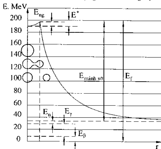
Hình 1.4. Sơ đồ giải phóng năng lượng khi phân hạch hạt nhân
