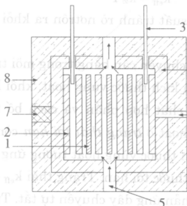
Hình 1.11. Sơ đồ lò phản ứng nơtron nhiệt
