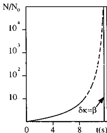
Hình 4.5. Sự thay đổi mật độ nơtrôn theo thời gian khi thay đổi tuyến tính độ phản ứng
