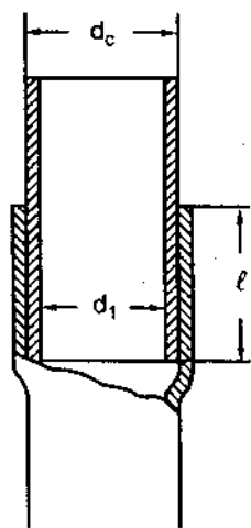
Hình 13.13. Kích thước măng sông phụ thuộc đường kính ống và cỡ mối hàn
