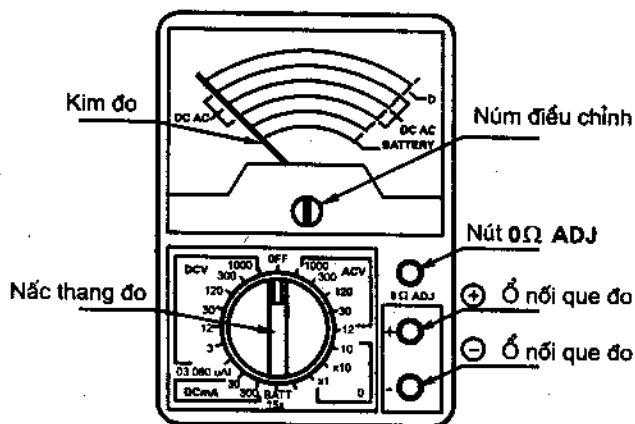
Hình 14.23. Vạn năng kế Hioki Hi tester Model 3000
