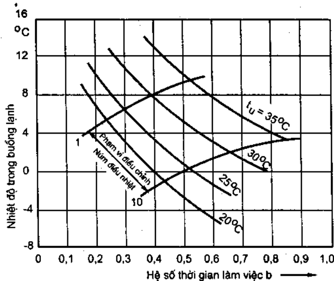
Hình 6.3. Sự phụ thuộc của b vào nhiệt độ buồng lạnh, nhiệt độ ngoài trời và vị trí núm rôle nhiệt độ
