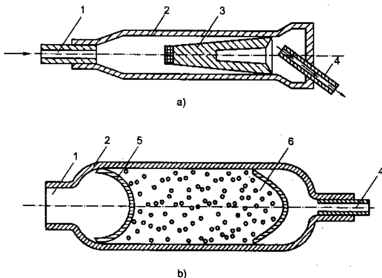
Hình 9.18. Cấu tạo phin lọc máy điều hòa
