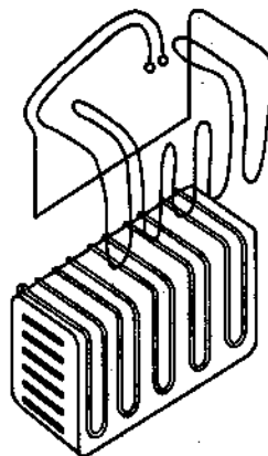
Hình 5.18. Dây điện trở xà đá được uốn lượn theo rãnh dàn bay hơi
