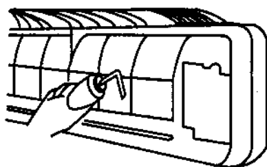
Hình 12.15. Thử thông dòng ống thoát nước ngưng
