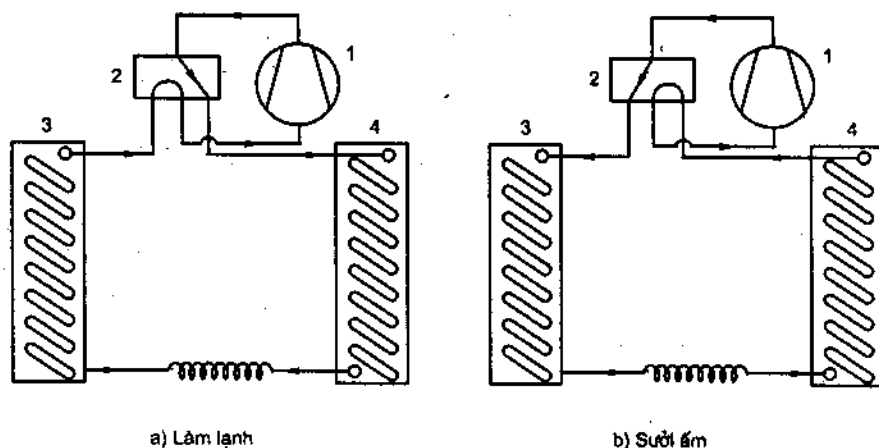
Hình 9.11. Nguyên tắc cấu tạo và làm việc của máy điều hòa 2 chiều
