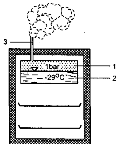
Hình 1.4. Tủ lạnh bằng R12 sôi tự nhiên trong khí quyển 1. Bình bốc hơi; 2. R12 lỏng; 3. Ống thông hơi.
