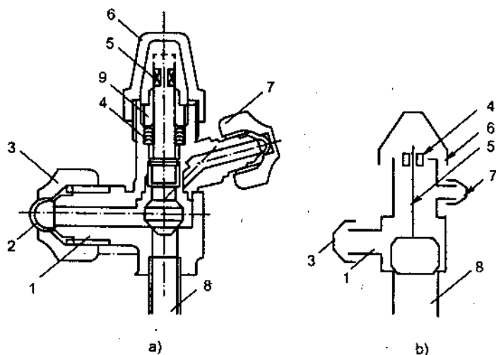
Hình 14.7. Van dịch vụ dàn nóng
