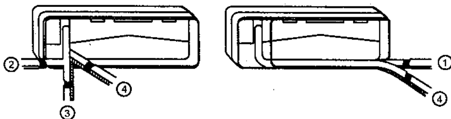
Hình 12.10. Các hướng nối ống của dàn lạnh (trong nhà)
