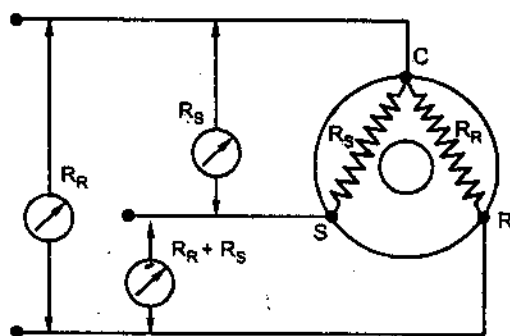
Hình 5.19. Phương pháp đo điện trở
