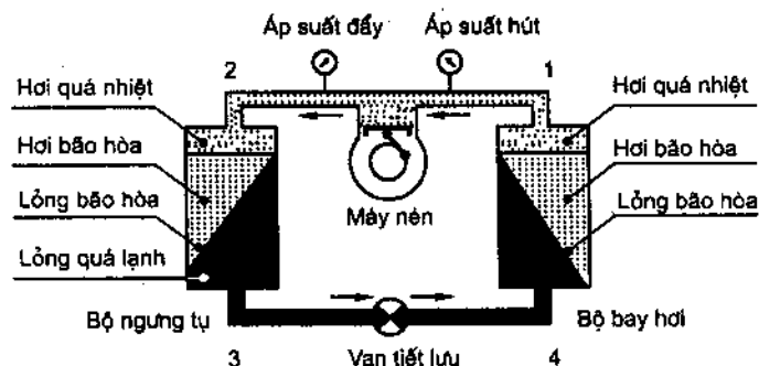
Hình 3.13. Chu trình thiết bị máy lạnh và trạng thái môi chất ở từng vị trí
