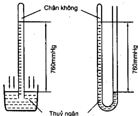
Hình 2.6. Nguyên tắc cấu tạo và hoạt động của barômet đo áp suất khí quyển 760mmHg = 1atm là áp suất khí quyển trên mặt nước biển ở 0°C
