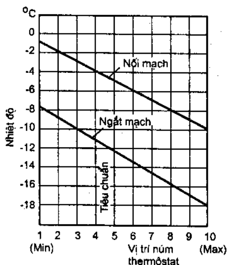
Hình 5.12. Đường đặc tính nhiệt độ của role APT-2
