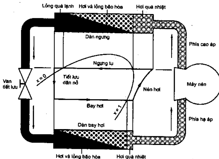
Hình 3.15. Quan hệ giữa các thiết bị và các quá trình biểu diễn trên đồ thị Mollier của một chu trình lạnh
