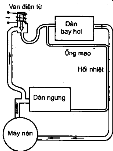
Hình 5.15. Hệ thống xả băng bằng hơi nóng (có van điện tử)
