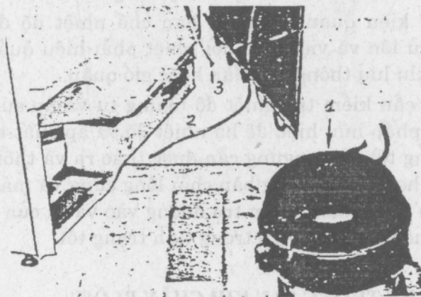
Hình 15.15. Block cũ được tách ra khỏi hệ thống lạnh. Các đường ống được bảo vệ bằng kẹp ống hoặc bằng nút bịt. Cần bảo vệ để dầu khỏi chảy tràn ra ngoài cũng như để phòng ôxi hóa, han gỉ bên trong
