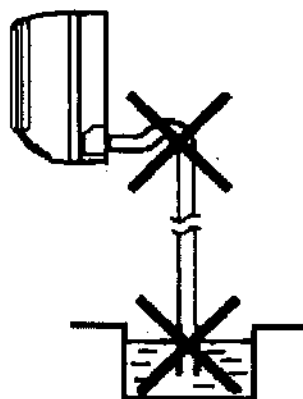
Hình 12.14. Không dùng bể nước ngưng trên đường thoát nước ngưng và không nhúng đầu thoát nước ngưng vào chậu nước hoặc rãnh thoát nước
