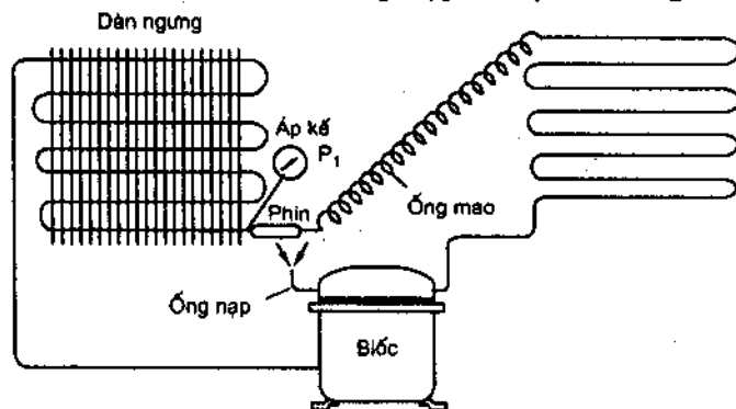
Hình 4.18. Phương pháp cân cáp thứ hai
