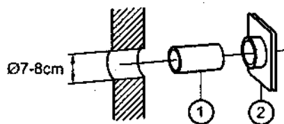
Hình 12.8. Lỗ khoét trên tường đi ống ga, nước, điện
