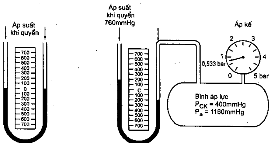
Hình 2.7. Áp chân không kế hình chữ U, thang đo là mmHg ở hai đầu
