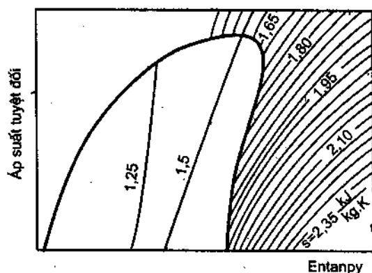
Hình 3.12. Các đường đẳng entropy s = \text{const}
