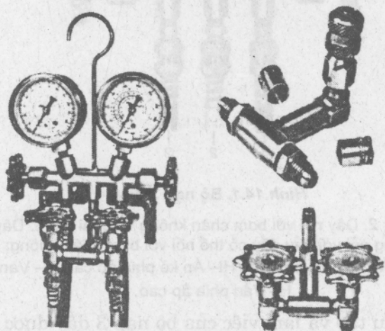
Hình 14.3. Đồ gá để chuyển bộ nạp 3 dây thành bộ nạp 4 dây
