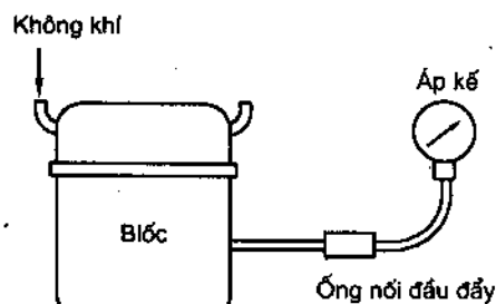
Hình 4.7. Sơ đồ thí nghiệm phần cơ block
