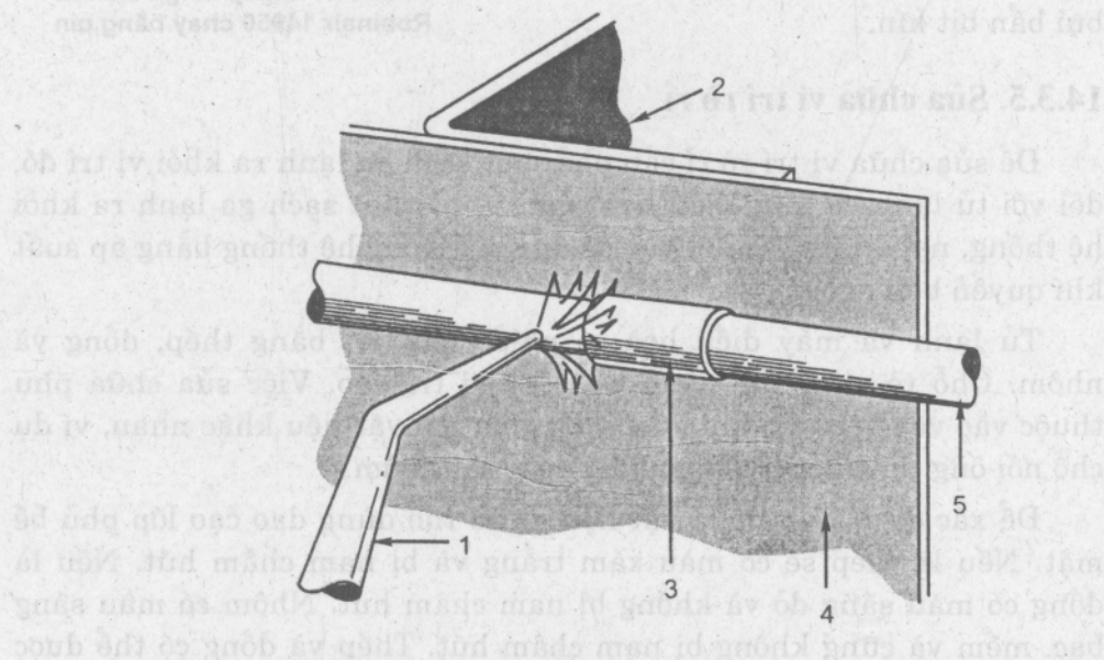
Hình 14.12. Dùng tấm kim loại che ngọn lửa hàn tránh ảnh hưởng đến các chi tiết khác
