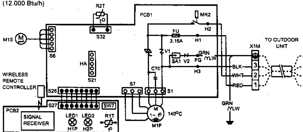
Dàn lạnh FT35BVM (12.000 Btu/h)
