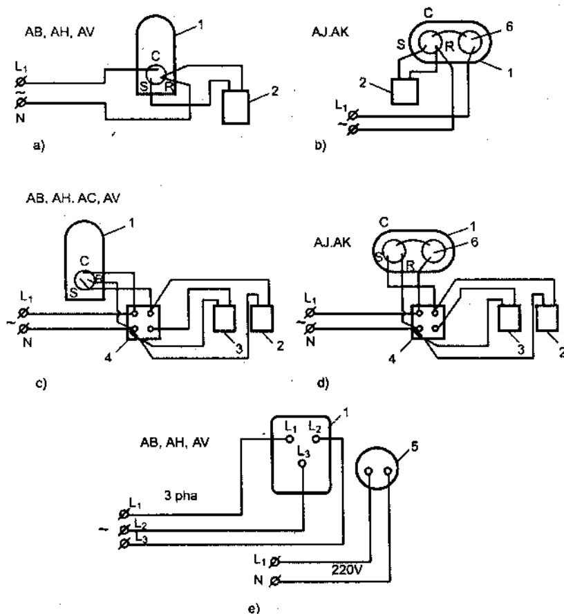
Hình 10.2. Cách đấu dây blốc TECUMSEH
