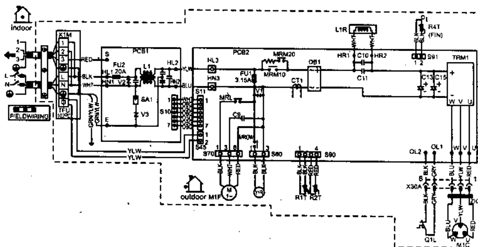
Hình 10.14. Sơ đồ điện máy điều hòa 2 chiều bơm nhiệt DAIKIN 9.000 và 12.000 Btu/h
