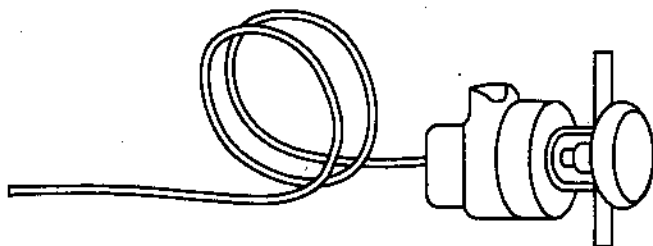
Hình 5.10. Hình dáng rơle nhiệt độ APT - 2
