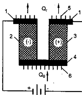
Hình 1.10. Cặp nhiệt điện
