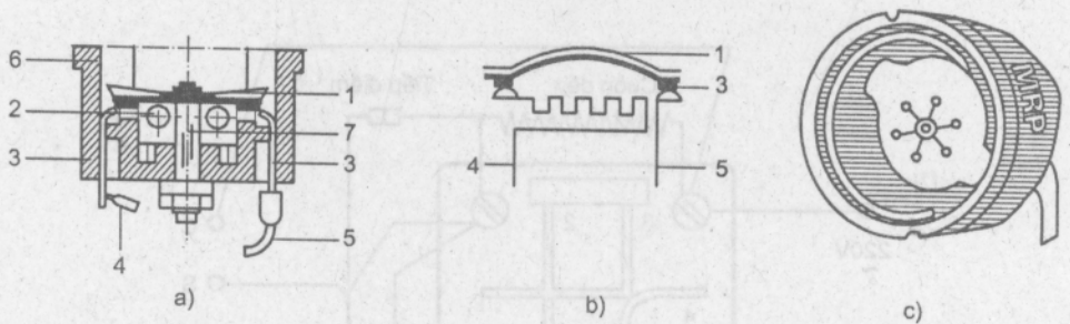
Hình 10.7. Nguyên tắc cấu tạo role bảo vệ kiểu tròn
