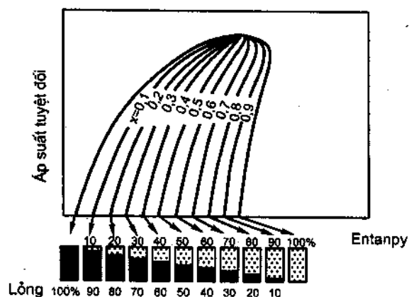
Hình 3.9. Các đường thành phần hơi không đổi x = \text{const}
