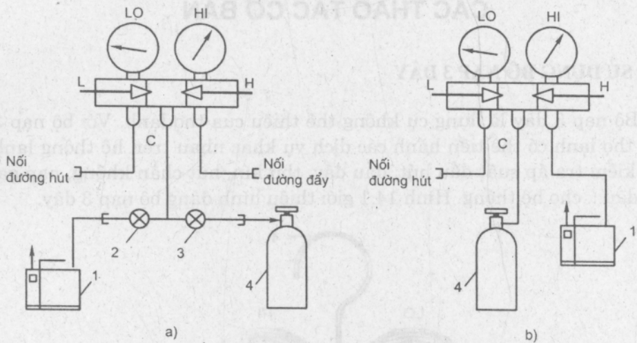
Hình 14.2. Nguyên tắc cấu tạo và làm việc
