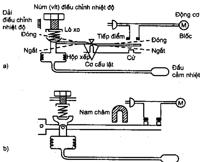
Hình 5.9. Nguyên tắc cấu tạo và hoạt động của role nhiệt độ
