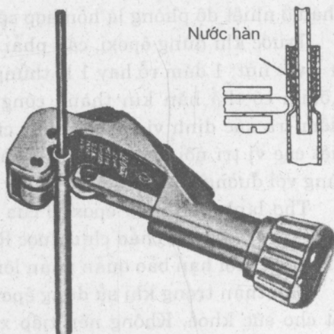
Hình 13.15. Dụng cụ thắt ống
