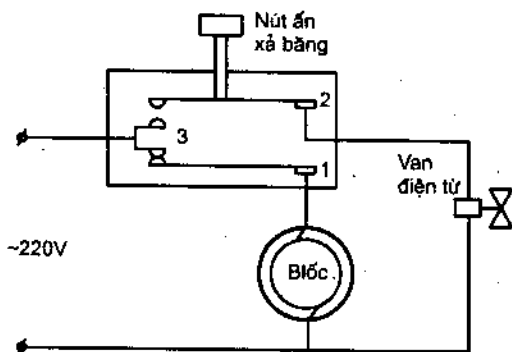
Hình 5.13. Nút ấn xả băng bán tự động dùng hơi nóng, khi xả băng block vẫn làm việc
