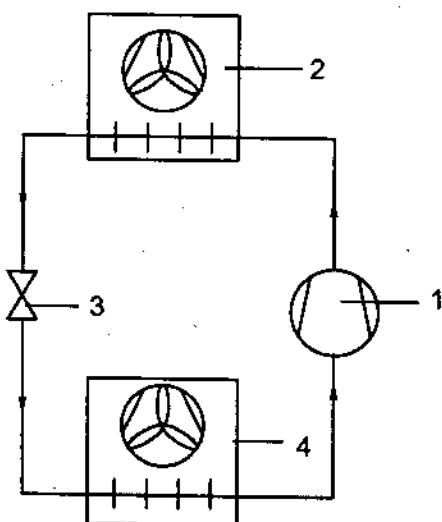
Hình 1.7. Bốn thiết bị chính của hệ thống lạnh nén hơi theo ký hiệu ISO
