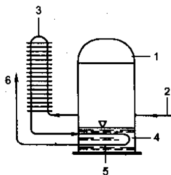
Hình 9.21. Vòng ống xoắn làm mát dầu
