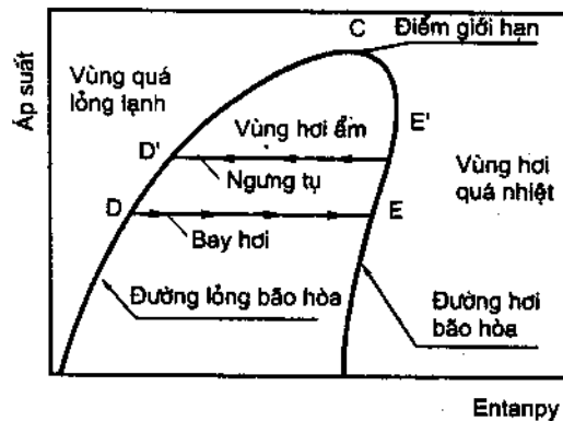
Hình 3.8. Đường lỏng và hơi bão hoà
