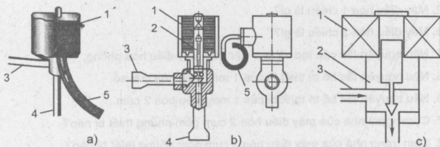
Hình 9.23. Van điện từ kiểu góc
