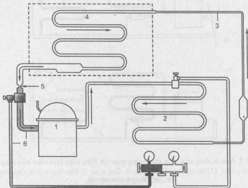
Hình 15.2. Kẹp ống đường hút để thử nghiệm
