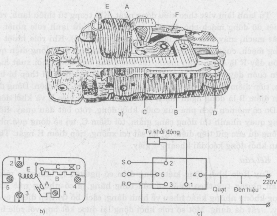
Hình 5.5. Role khởi động bảo vệ (lắp chung trong 1 vỏ) hãng Copeland
