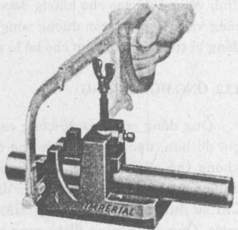
Hình 13.2. Cắt ống bằng cửa có đồ gá
