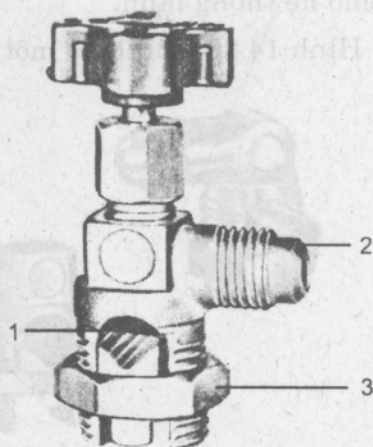
Hình 14.18. Một kiểu van trích thường dùng
