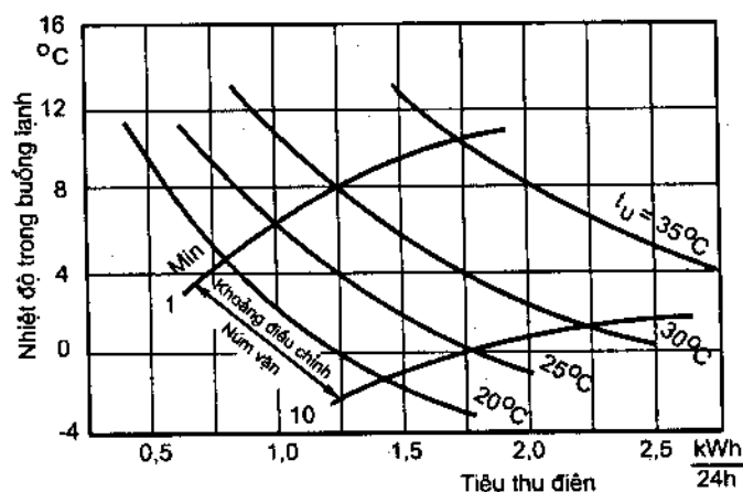
Hình 6.4. Điện năng tiêu thụ phụ thuộc vào nhiệt độ trong và ngoài buồng lạnh cũng như vị trí điều chỉnh núm vặn thermostat tủ ZIL-KX240l
