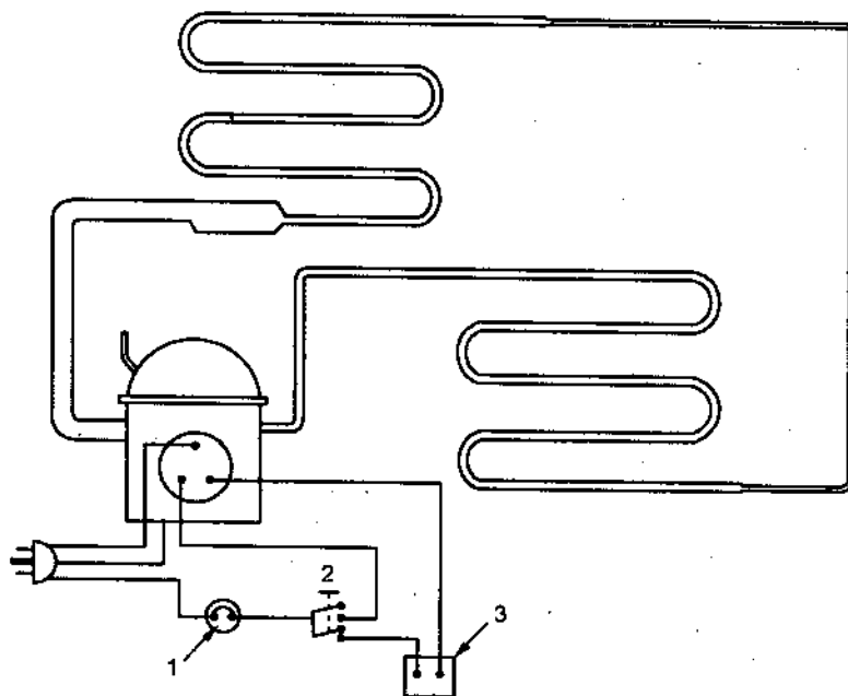
Hình 15.1. Thử nghiệm khởi động động cơ máy nén sau khi tháo nắp bảo vệ rơle khởi động, bảo vệ và lắp mạch khởi động khác
