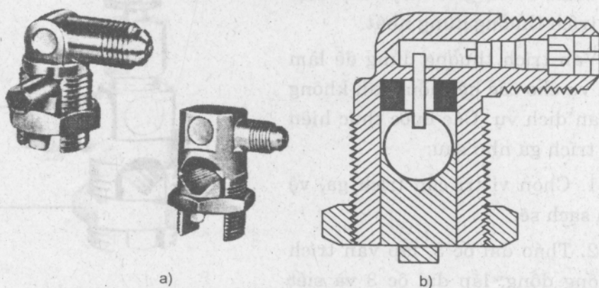
Hình 14.20. Van trích có lõi
