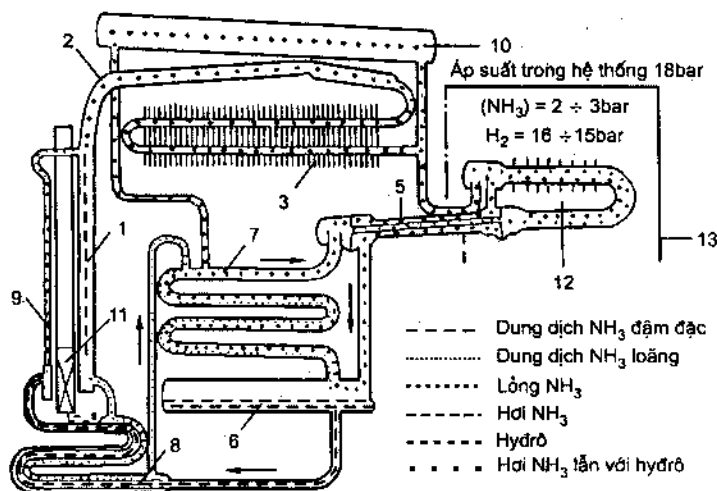
Hình 1.9. Cấu tạo của tủ lạnh hấp thụ khuếch tán
