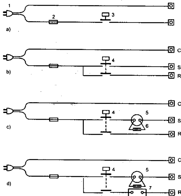
Hình 8.2. Một số kiểu dây thử khởi động block tủ lạnh
