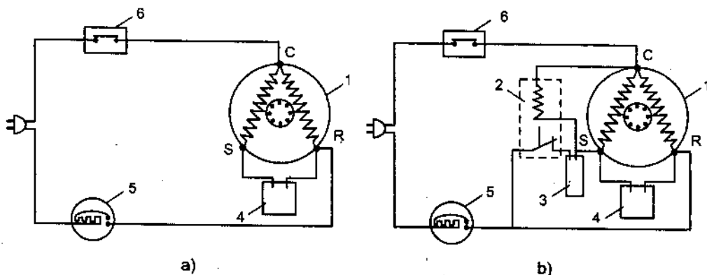
Hình 10.1. Sơ đồ đấu điện thông dụng của block ĐHKK
