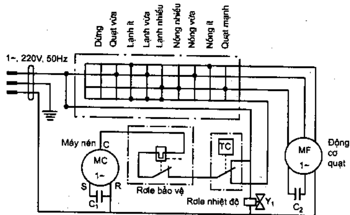
Hình 10.11. Sơ đồ điện đơn giản của một máy điều hòa cửa sổ 2 chiều bơm nhiệt. Y 1 – Van điện từ điều khiển van đổi dòng 4 ngã.
