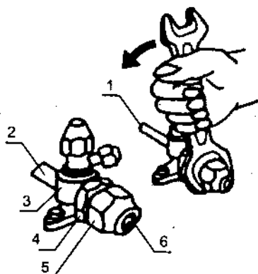
Hình 13.17. Tháo mũ ren cụm nhà ngoài
