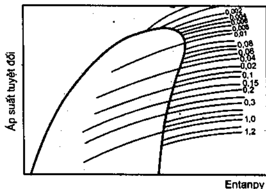
Hình 3.11. Các đường v = \text{const}
