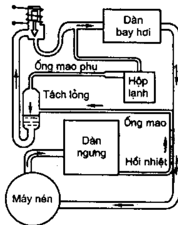
Hình 5.16. Tủ lạnh hai nhiệt độ dùng van điện tử khống chế nhiệt độ ở hộp lạnh
