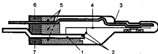
Hình 10.8. Hình dáng một role bảo vệ kiểu lưỡng kim để gắn trực tiếp lên cuộn dây động cơ
