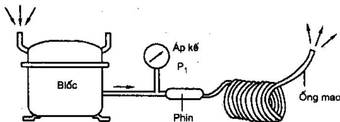
Hình 4.17. Phương pháp cân cáp thứ nhất
