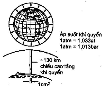
Hình 2.5. 1\text{atm} = 1,033\text{at} = 1,033\text{kG/cm}^2 = 760\text{mmHg} là trọng lực của cột khí quyển lên tiết diện 1\text{cm}^2 của nó trên mặt nước biển. Trọng lực đó bằng 1,033\text{kG}
