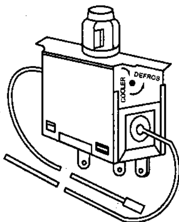
Hình 5.11. Rơle nhiệt độ hai chức năng RANKO (Mỹ) (điều chỉnh nhiệt độ buồng lạnh và xả băng dàn lạnh)
