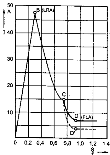
Hình 10.3. Đặc tính dòng khởi động của role khởi động kiểu điện áp (9000Btu/h, động cơ 0,75kW)
