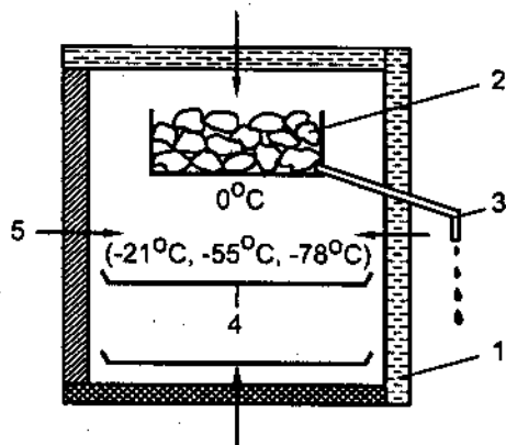
Hình 1.1. Tủ lạnh dùng nước đá
