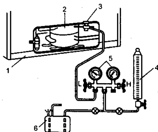
Hình 14.16. Nối xi lanh nạp ga vào hệ thống lạnh
