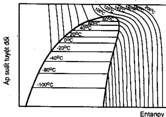
Hình 3.10. Các đường đẳng nhiệt t = \text{const}
