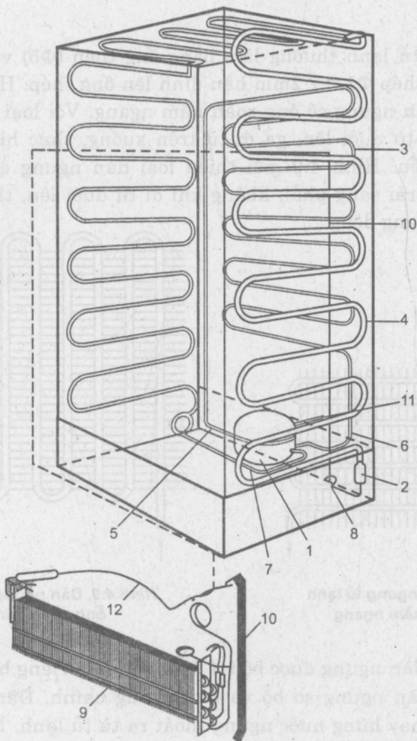
Hình 4.10. Tủ lạnh có dàn ngưng bố trí trên vỏ tủ, dàn bay hơi phía sau, trên tủ (vẽ riêng biệt xuống dưới để dễ quan sát dàn ngưng)
