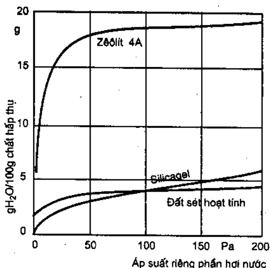
Hình 4.19. Khả năng hấp thụ ẩm của Zeolit 4A, Silicagel và đất sét hoạt tính
