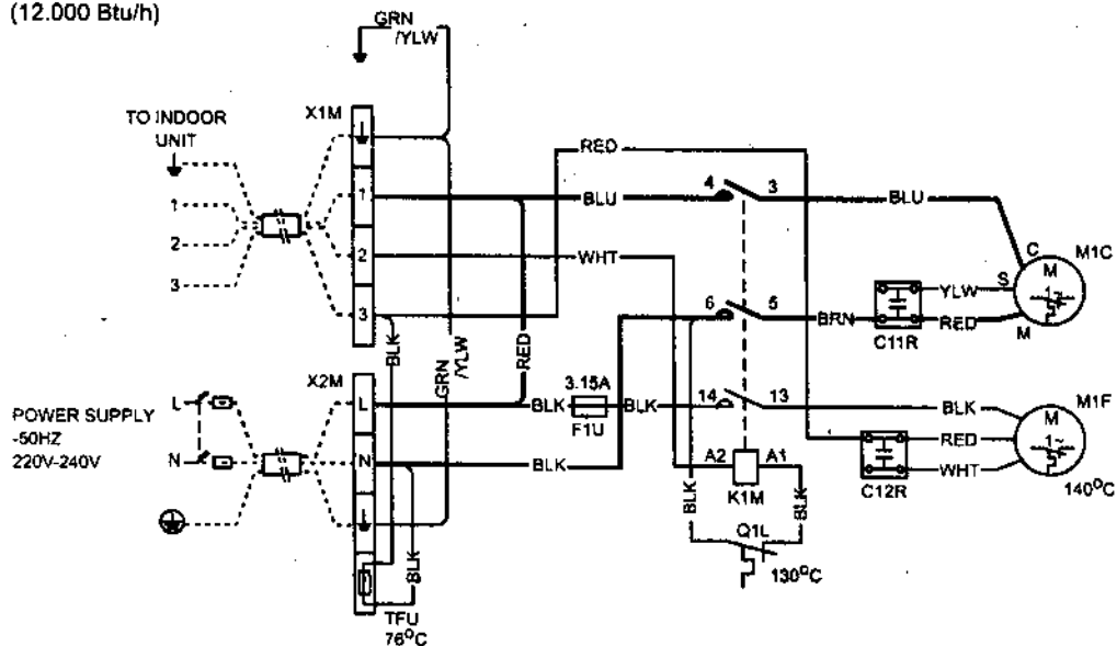
Dàn nóng R35JV16 (12.000 Btu/h)
