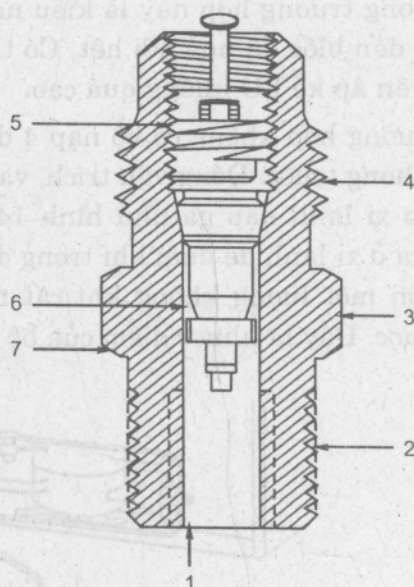
Hình 14.19. Đầu gá mũ loe có lõi
