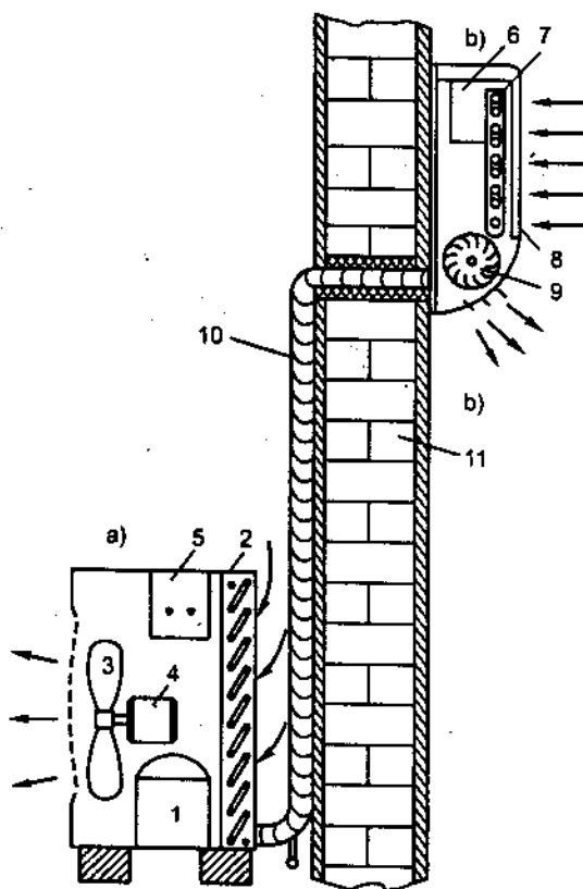
Hình 9.6. Cấu tạo máy điều hòa hai cụm
