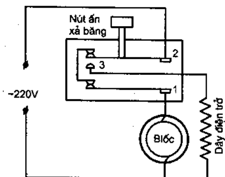
Hình 5.14. Nút ấn xả băng bán tự động dùng dây điện trở, khi xả băng block ngừng làm việc
