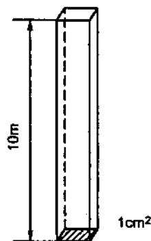
Hình 2.4. 1\text{at} = 1\text{kG/cm}^2 là trọng lực của cột nước cao 10\text{m} tác dụng lên tiết diện 1\text{cm}^2 của nó. Trọng lực đó bằng 1\text{kG}
