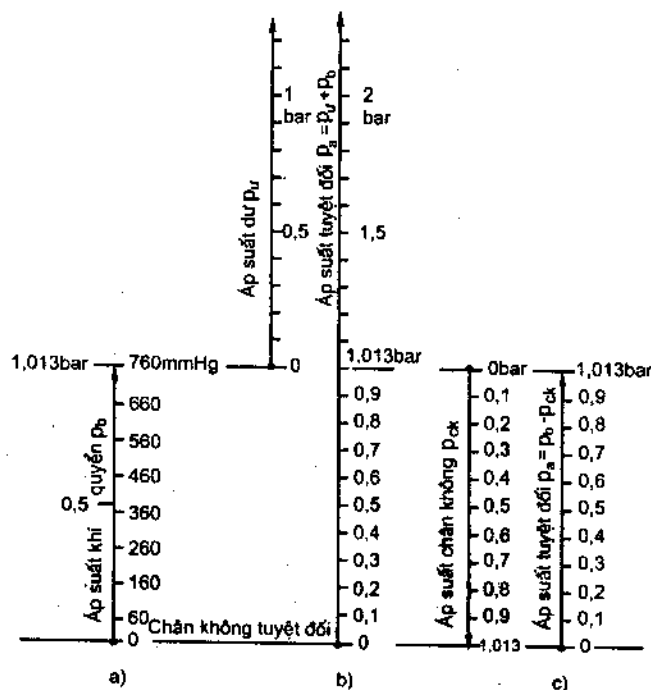
Hình 2.10. Các loại áp suất
