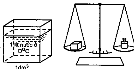
Hình 2.1. Khối lượng của 1 lít nước ở 0°C bằng 1kg và đo khối lượng bằng cân có quả cân
