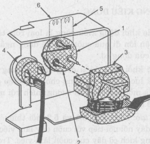
Hình 5.1b. Rôle khởi động kiểu dòng và rôle bảo vệ hăng Kelvinator ở tư thế lắp vào 3 cọc tiếp điện của khối
