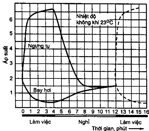
Hình 6.2. Biến thiên áp suất trong dàn ngưng và dàn bay hơi tủ lạnh R12, nhiệt độ trong phòng 23°C, nhiệt độ ngưng tụ 31°C, nhiệt độ bay hơi -22°C, chu kỳ làm việc 4 phút, nghỉ 12 phút
