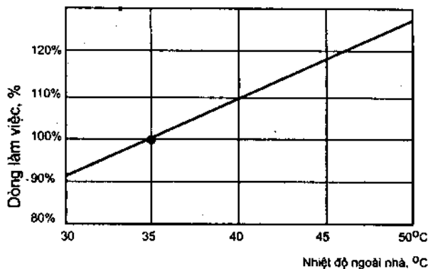
Hình 11.3. Cường độ dòng điện làm việc (FLA) phụ thuộc nhiệt độ ngoài trời
