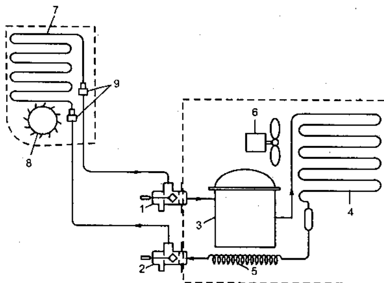
Hình 14.6. Máy điều hoà 2 cụm
