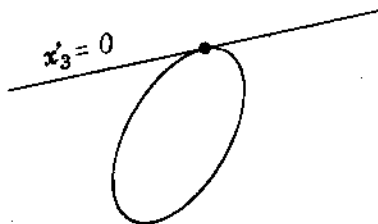
hình 46: đường parabol
