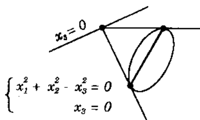
hình 44: đường elip
