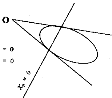
Hình 45: đường hypebol
