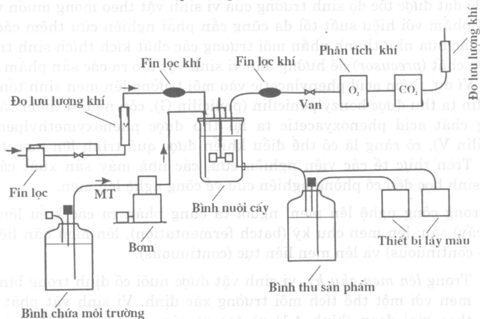
Hình 4.2. Sơ đồ đơn giản mô tả nguyên tắc lên men liên tục
