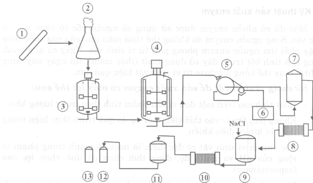
Hình 5.1. Sơ đồ minh họa các giai đoạn sản xuất enzyme dạng dung dịch.
