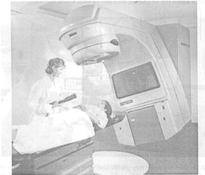
Hình 2-10: Một máy gia tốc tuyến tính năng lượng cao trong xạ trị
