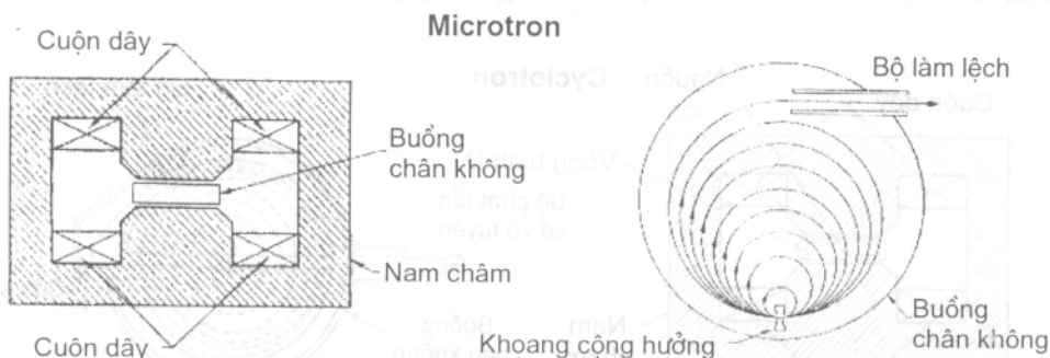
Hình 2-4: Sơ đồ khối của máy gia tốc Microtron
