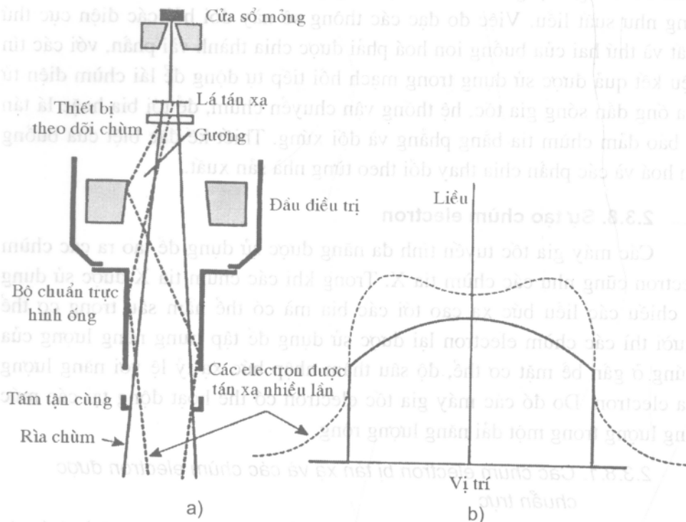
Hình 2-32: (a) Chùm electron với một lá tán xạ và bộ chuẩn trực hình ống.
