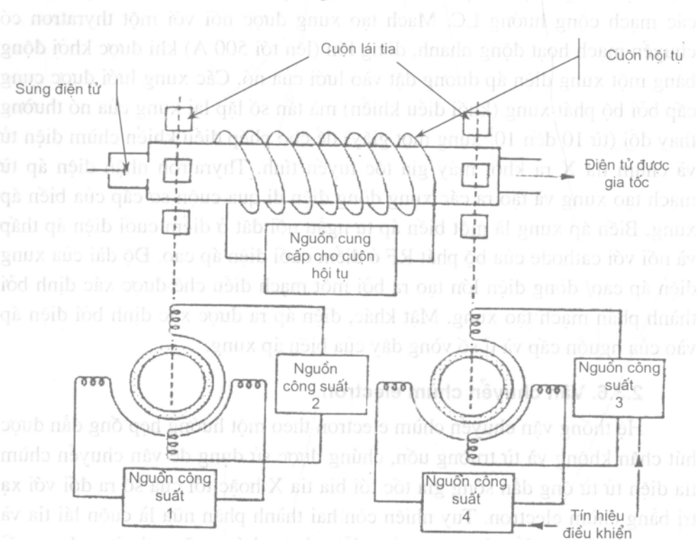
Hình 2-20: Bộ phận phát chùm tia
