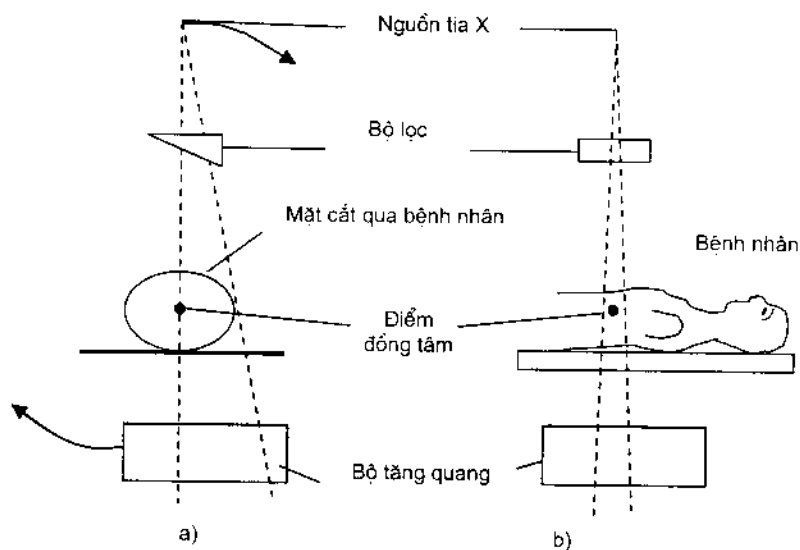
Hình 2-42: Sử dụng một máy mô phỏng để tạo ảnh
