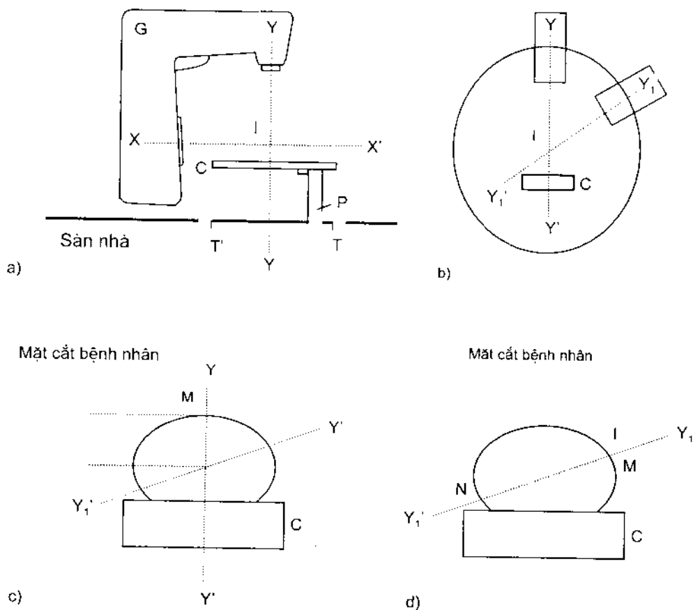
Hình 2-34: (a) Sơ đồ khối điều trị và các mặt cắt theo các hướng X-X', Y-Y': trục hoành X-X' là trục quay của đàn quay, trục tung Y-Y' là trục quay của bộ chuẩn trục; (b) Phác thảo trong mặt phẳng qua Y-Y', vuông góc với X-X', Y 1 -Y 1 ' là hướng của một chùm tia thứ hai; (c) Minh họa một lần điều trị đồng tâm. Hai chùm tia giao nhau tại một độ sâu d bên trong bệnh nhân; (d) Minh họa một chùm tia của một lần điều trị bó SSD cố định. Tâm đặt tại bề mặt da bệnh nhân.
