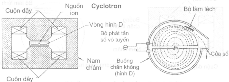
Hình 2-3: Sơ đồ khối máy gia tốc cyclotron
