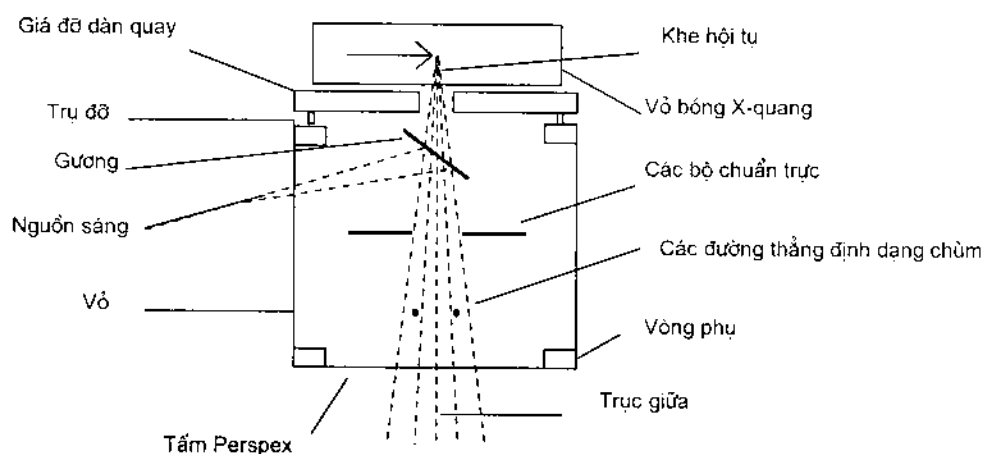
Hình 2-43: Đầu phát tia X trong thiết bị mô phỏng
