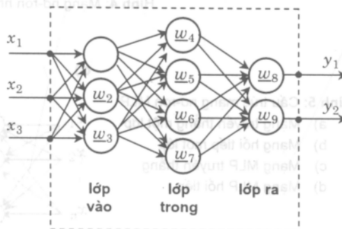
Hình 3: Mạng nơ-ron ba lớp truyền thẳng
