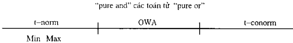
Hình 1: Mối liên hệ giữa toán tử OWA, t -chuẩn và t -đối chuẩn
