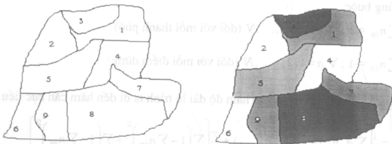
Hình 3 : Bản đồ 9 nước và 4 màu
