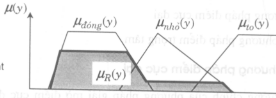
Hình 9: Xác định giá trị mờ của luật hợp thành.
