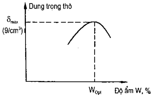
Hình 1. Đường cong Proctor
