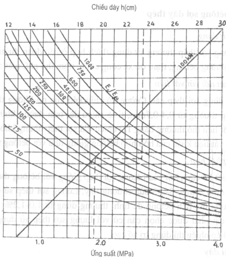
Hình 8-17. Toán đồ tính ứng suất khi tải trọng trực đơn tác dụng ở giữa cạnh dọc của tấm
