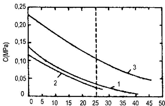
Hình 7-1 Quan hệ của C và khi ngăn ngừa hỗn hợp đá nhựa chảy dẻo và phá hoại
