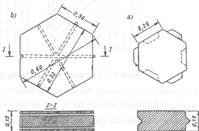
Hình 9-9. Các tấm bê tông sáu cạnh của Kiriencó
