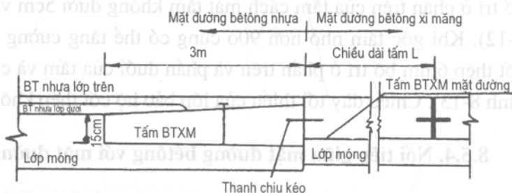
Hình 8-14. Xử lý chỗ nối tiếp giữa mặt đường bê tông với mặt đường nhựa
