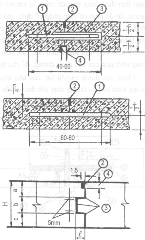
Hình 8-5. Các kiểu khe co thường dùng
