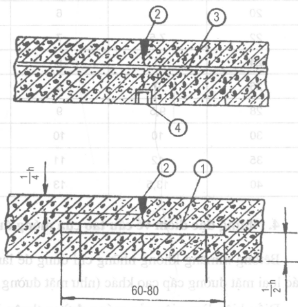
Hình 8-7. Các kiểu khe uốn vòng
