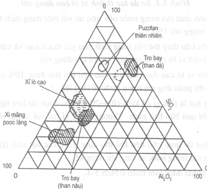
Hình 5.2. Biểu thị thành phần các chất liên kết vô cơ trên toạ độ tam giác đều.
