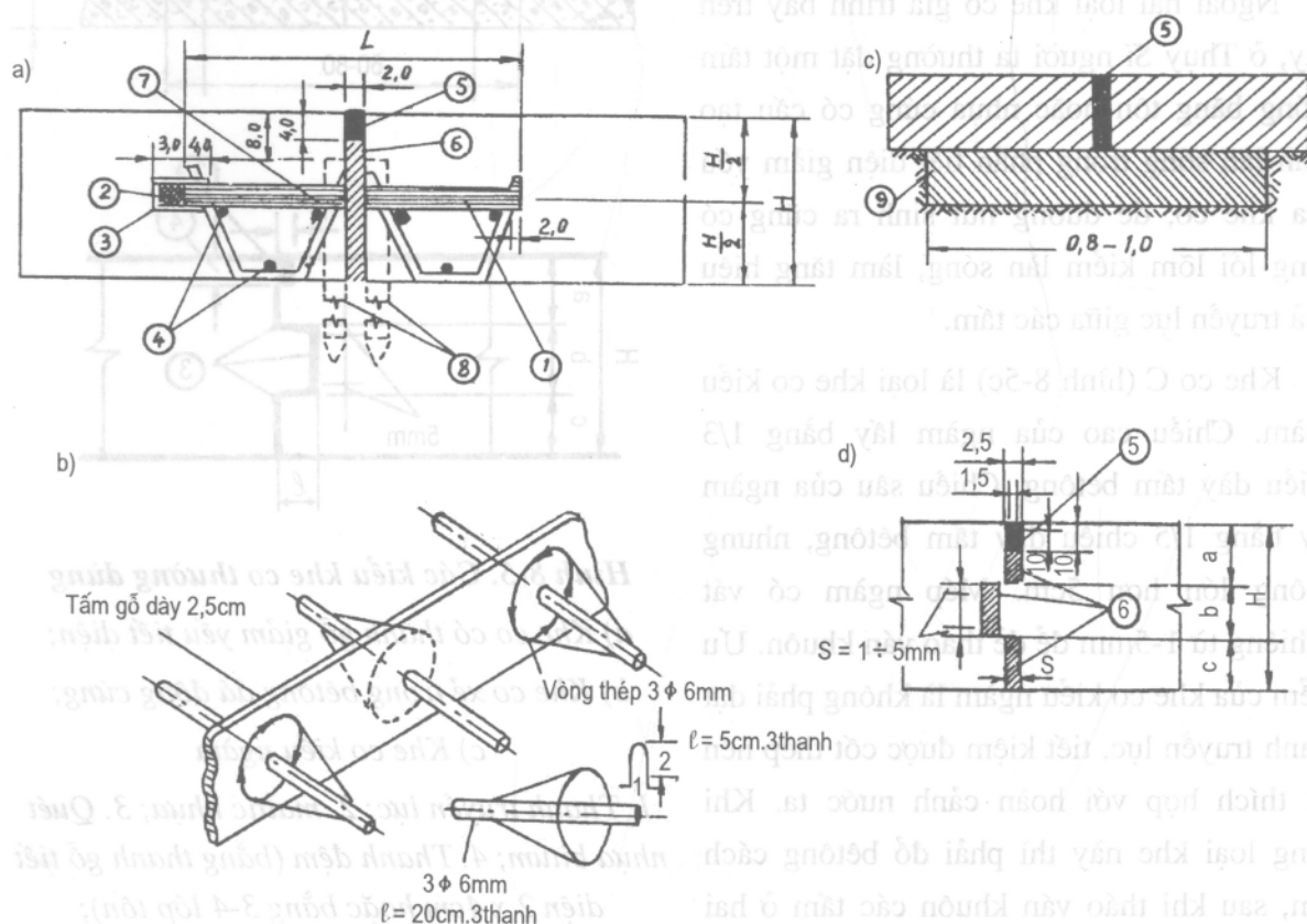
Hình 8-6. Các kiểu khe dẫn thường dùng
