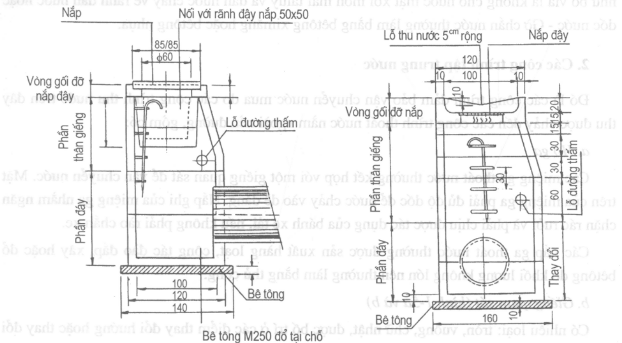
Hình 1-5. a. Giếng quan sát; b. Ga thu nước kết hợp với giếng quan sát
