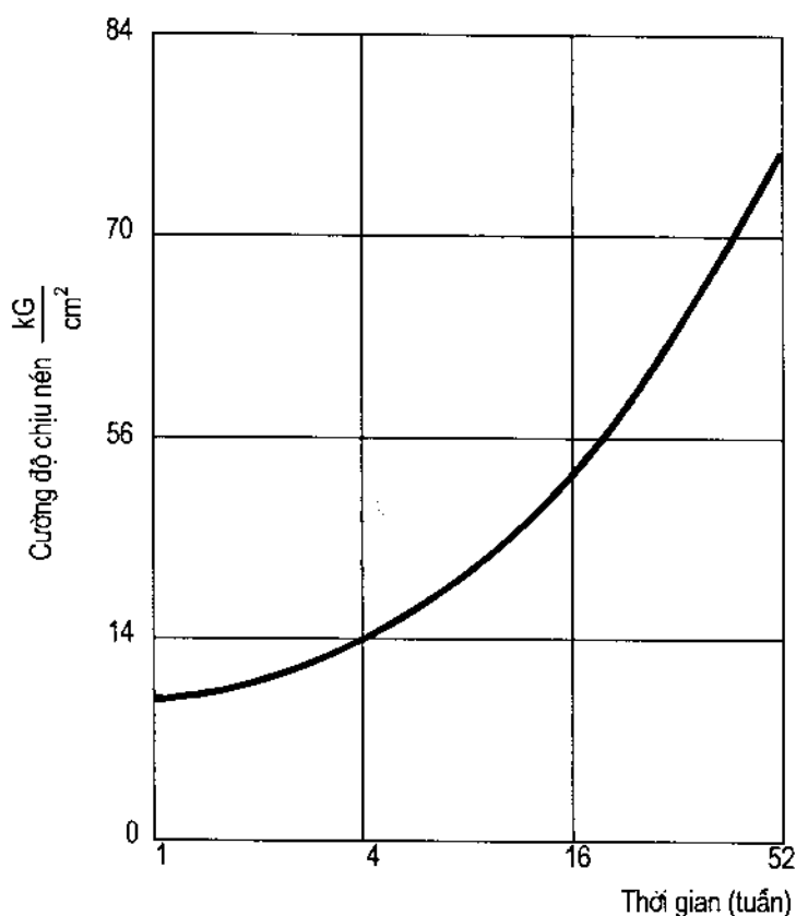
Hình 2.2. Sự tăng của cường độ đất gia cố vôi theo thời gian (đất sét gia cố 10% vôi)
