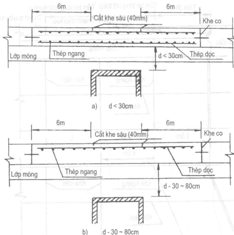
Hình 8-16-1. Xử lý tại vị trí đường ô tô đi qua công trình dạng hình hộp
