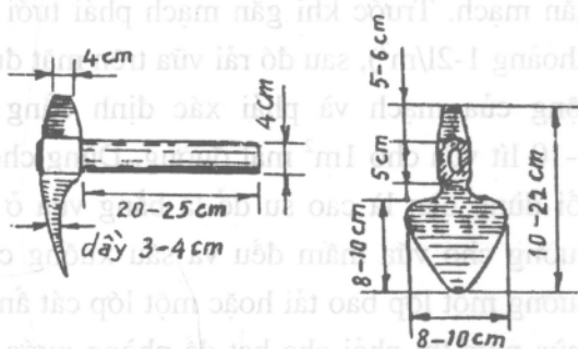
Hình 9-5. Búa chèn để lát mặt đường
