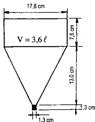
Hình 4-1. Phễu dùng để xác định độ sệt của vữa xi măng cát
