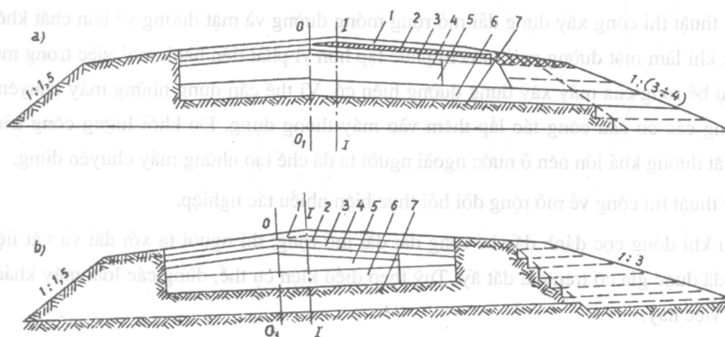
Hình 10.1. Sơ đồ mở rộng mặt đường và nền đường về một bên
