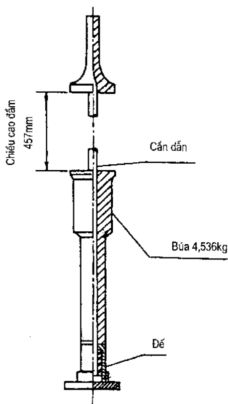
Hình 1. Đầm Marshall
