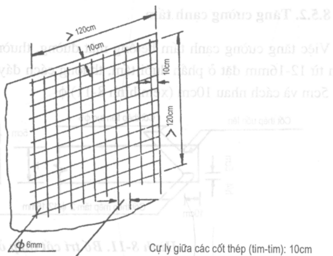
Hình 8-13. Bố trí tăng cường lưới thép
