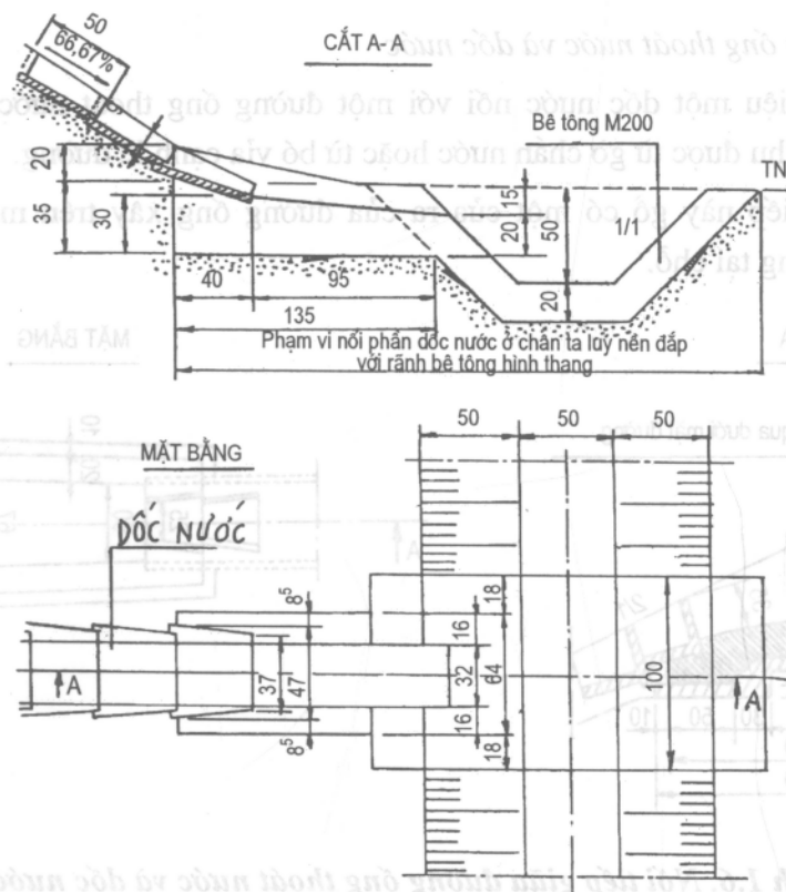
Hình 1-7. Nối tiếp giữa dốc nước và rãnh hình thang ở chân taluy nền đắp
