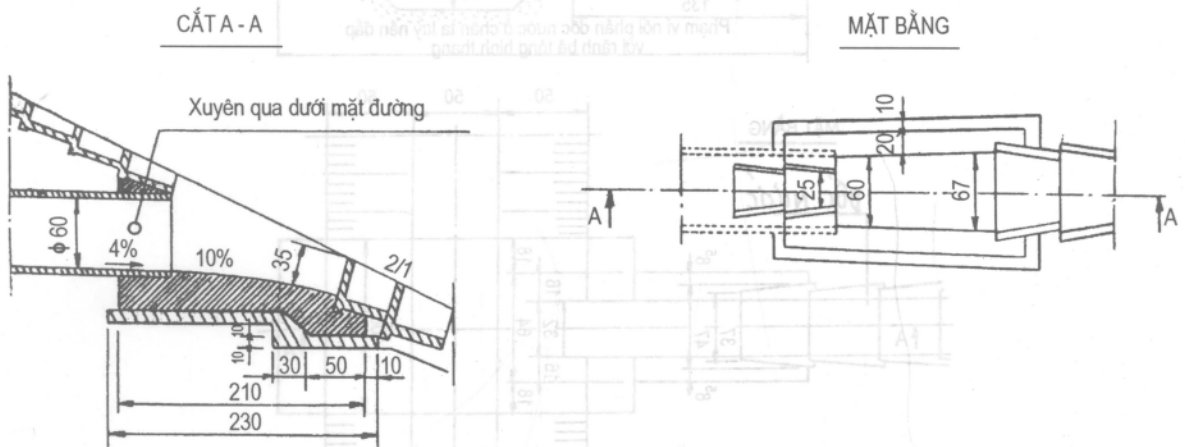
Hình 1.6. Nối tiếp giữa đường ống thoát nước và dốc nước
