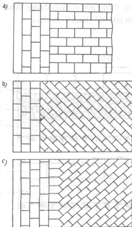
Hình 9-3. Các hình thức lát mặt đường đá tảng
