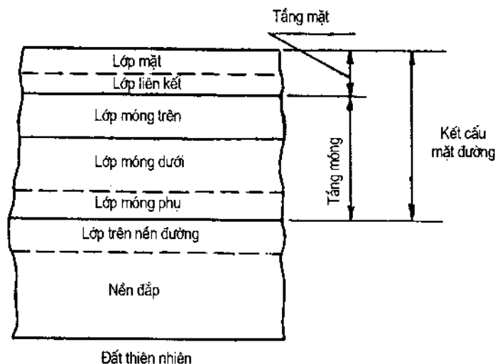
Hình 1.1. Kết cấu mặt đường
