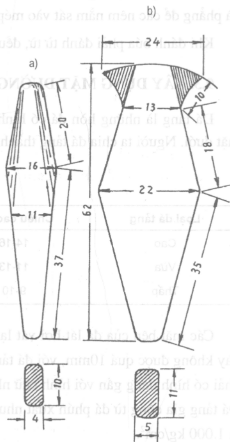
Hình 9-1. Các loại nê-m
