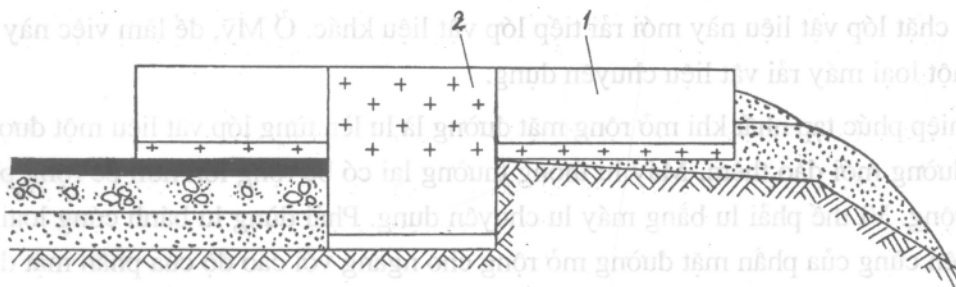
Hình 10.3. Sơ đồ cấu tạo lưới san của máy san tự hành khi lắp bộ phận phụ để đào lòng đường
