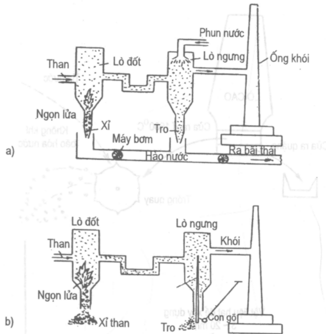
Hình 5-5. Sơ đồ thu tro bay ở các nhà máy nhiệt điện
