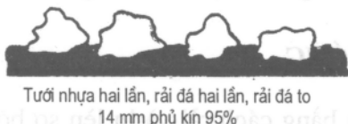
Hình 6.1. Các phương pháp láng nhựa dùng nhựa nóng của công ty Shell (Anh).
