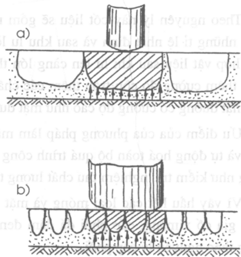
Hình 1-2. Mặt đường làm theo nguyên lý lát
