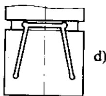
Hình 2-9. Các biện pháp chống bó kẹt piston
