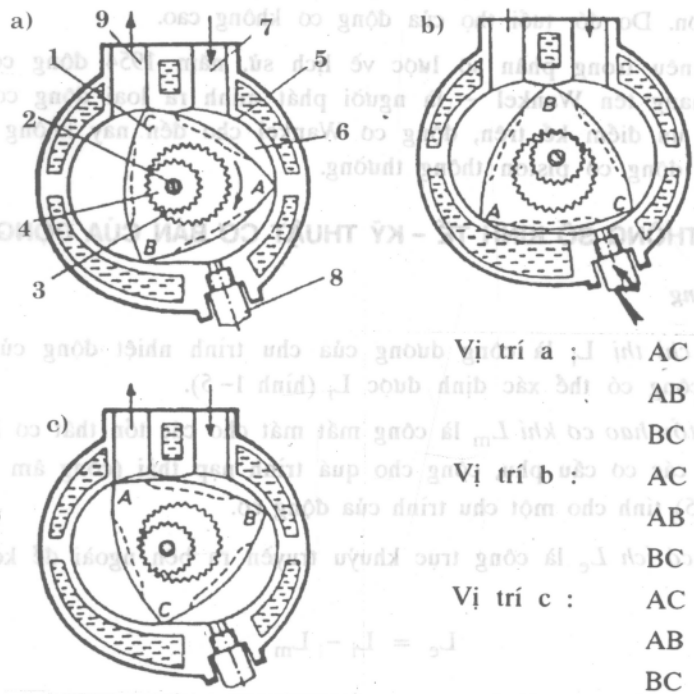
Hình 1.13. Nguyên lý làm việc của động cơ piston quay 1. rôto (piston quay), 2. trục cơ, 3. vành răng của rôto, 4. bánh răng trục cơ, 5. xy lanh, 6. buồng nạp, 7. cửa nạp, 8. bugi, 9. cửa thải
