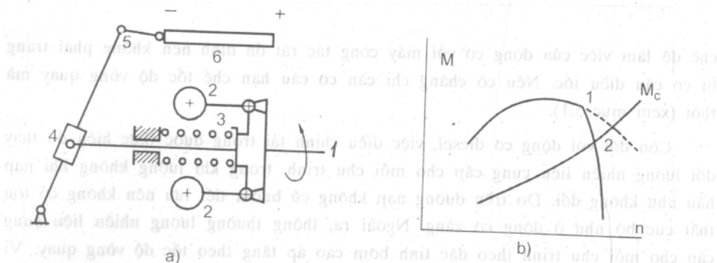
Hình 5-37. Cơ cấu điều tốc kiểu Wan
