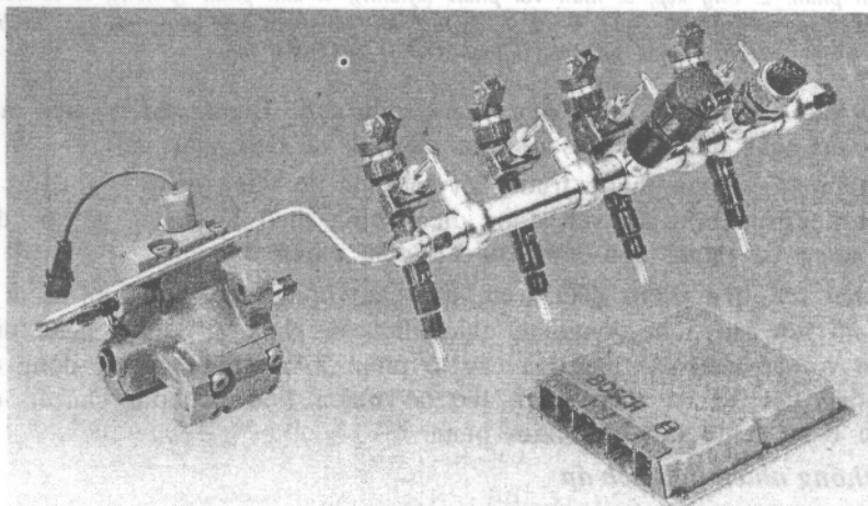
Hình 5-27. Các bộ phận chính của hệ thống nhiên liệu tích áp
