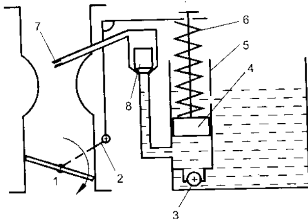
Hình 5-13. Hệ thống tăng tốc 1. bướm ga, 2. đòn dẫn động, 3. van bi, 4. piston, 5. xy-lanh, 6. lò xo, 7. vòi phun, 8. van rơi
