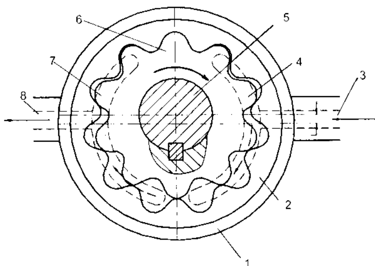
Hình 6-4. Bơm bánh răng ăn khớp trong
