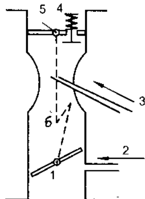
Hình 5-12. Hệ thống khởi động 1. bướm ga, 2. đường hỗn hợp không tải, 3. hệ thống chính, 4. van an toàn, 5. bướm gió, 6. liên kết bướm gió - bướm ga
