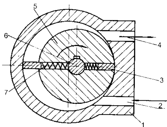
Hình 6-5. Bơm cánh gạt
