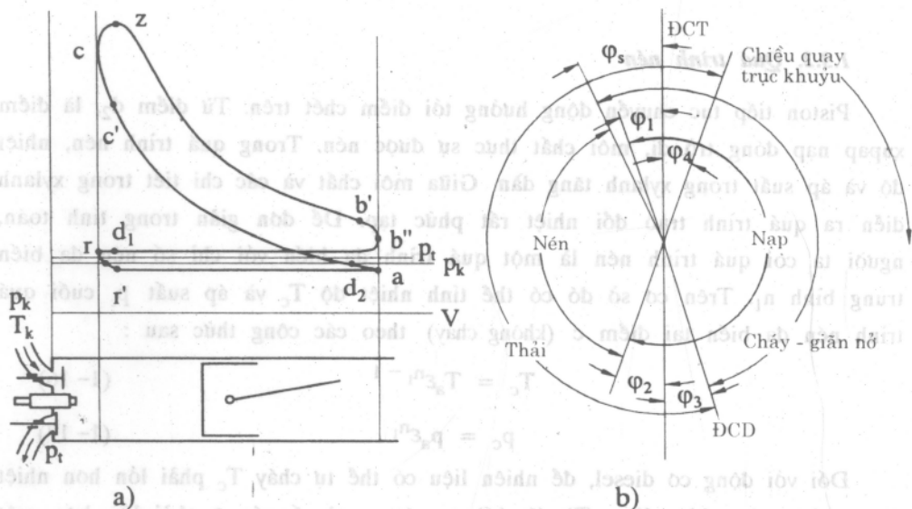
Hình 1-5. Đồ thị nguyên lý làm việc của động cơ 4 kỳ không tăng áp a. Đồ thị công ; b. Đồ thị pha
