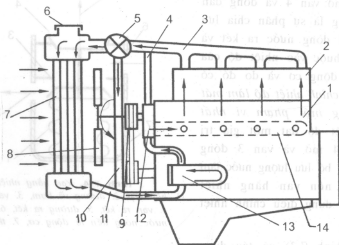
Hình 7-3. Hệ thống làm mát cưỡng bức tuần hoàn kín một vòng
