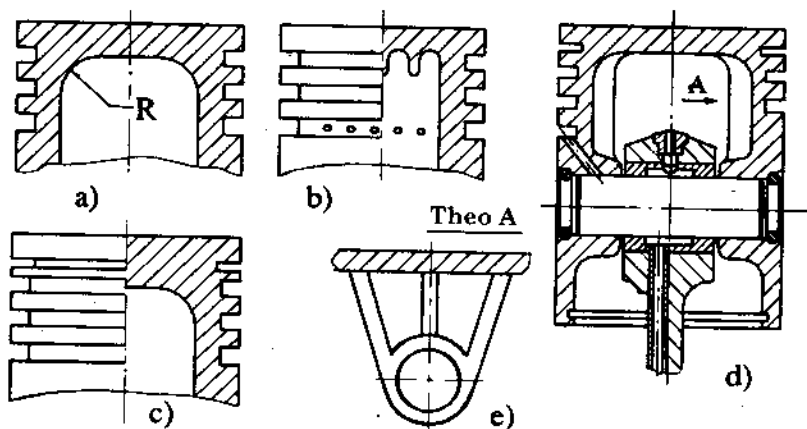
Hình 2-5. Kết cấu đầu piston
