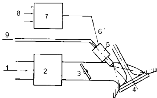
Hình 5-17. Sơ đồ hệ thống phun xăng
