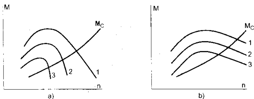
Hình 5-36. Vẽ tính cần thiết đặt điều tốc trên động cơ diesel a) động cơ xăng, b) động cơ diesel, 1. tải lớn, 2. tải trung bình, 3. tải nhỏ
