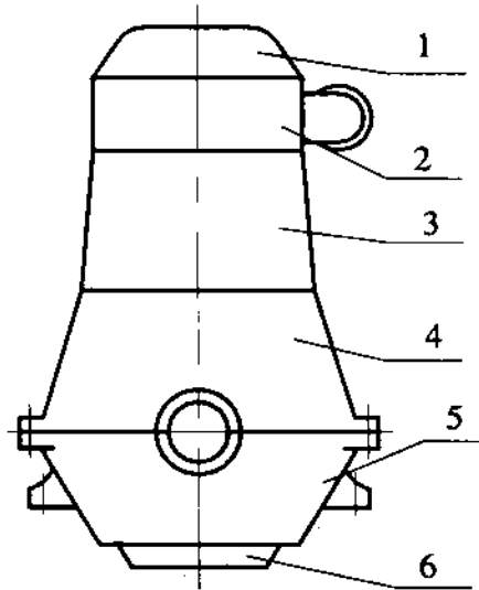
Hình 3-1. Sơ đồ phân chia động cơ 1. nắp che, 2. nắp xylanh, 3. thân xylanh, 4. hộp trục khuỷu, 5. đế máy, 6. cacte dầu (máng dầu)
