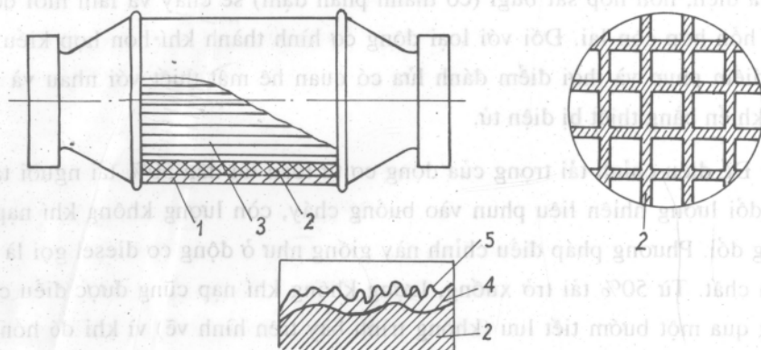
Hình 10-3. Bộ xử lý ba thành phần
