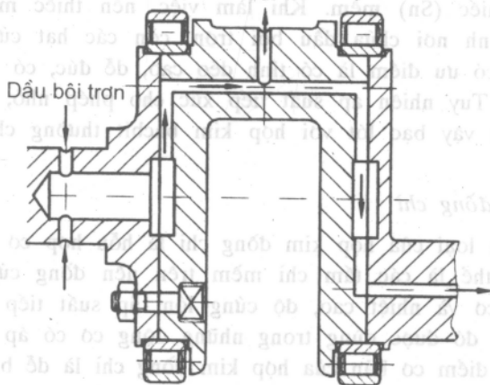
Hình 2.35. Trục khuỷu dùng ổ bi
