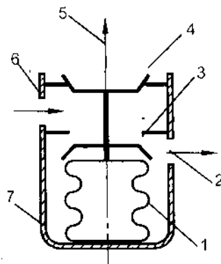
Hình 7-4. Van hằng nhiệt
