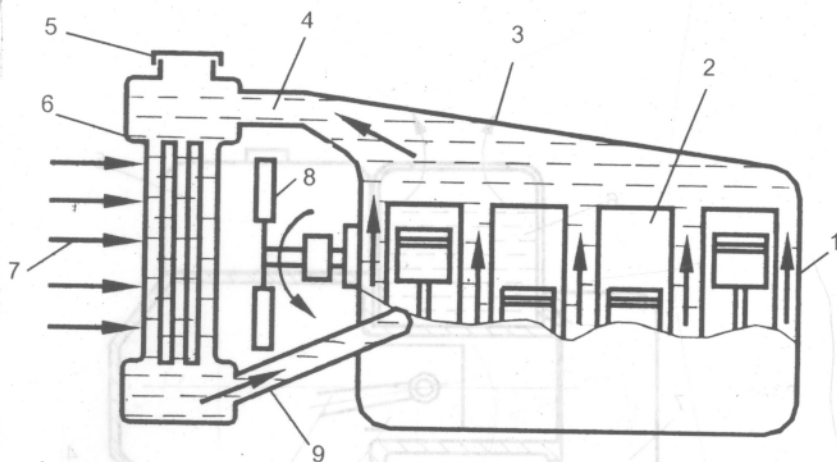
Hình 7-2. Hệ thống làm mát đối lưu tự nhiên
