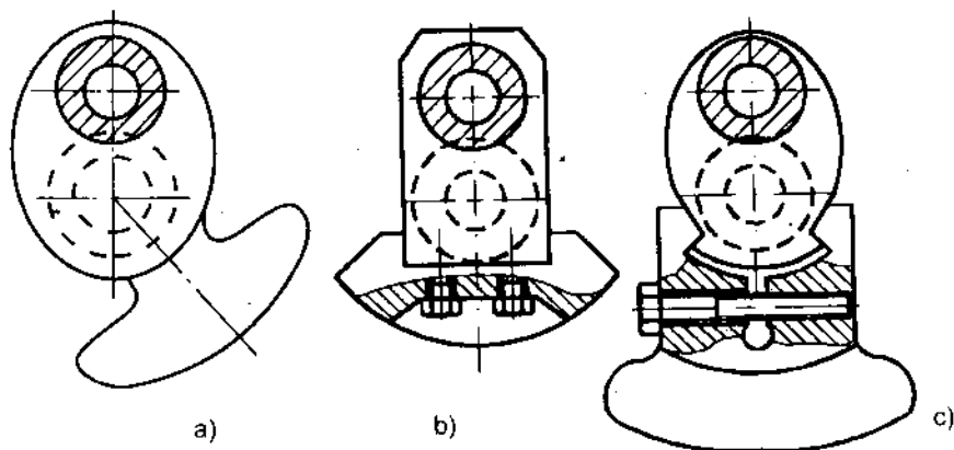
Hình 2-31. Kết cấu đối trọng
