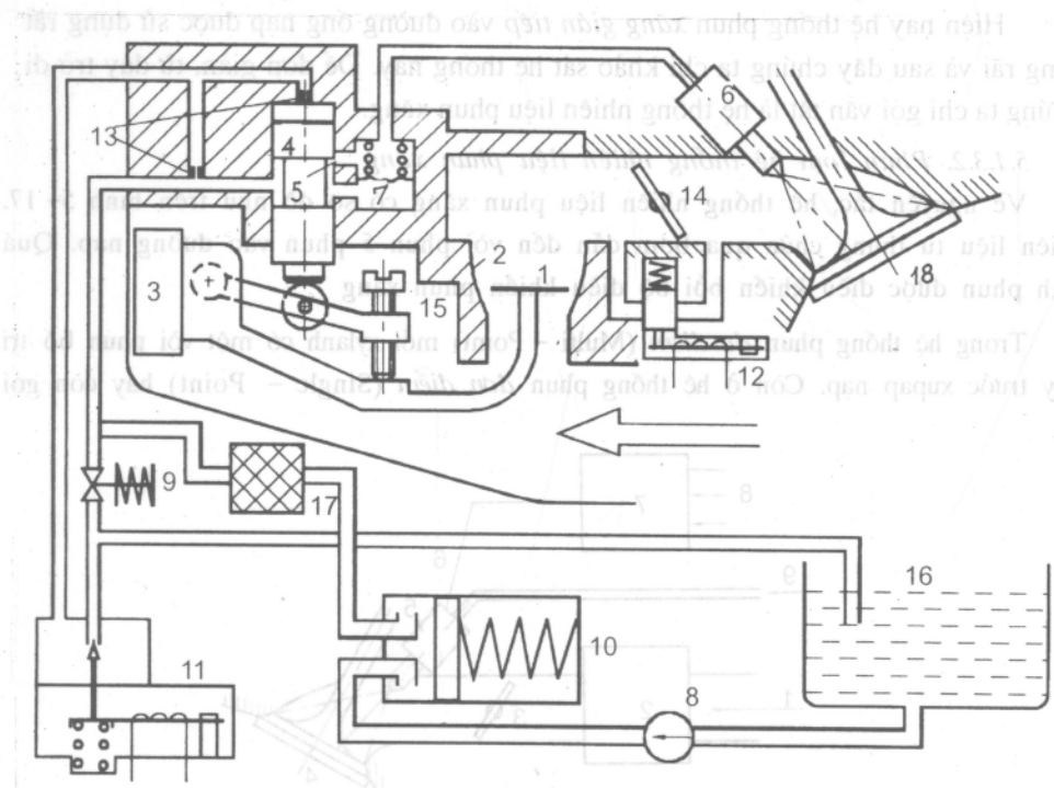
Hình 5-18. Hệ thống phun xăng K - Jetronic
