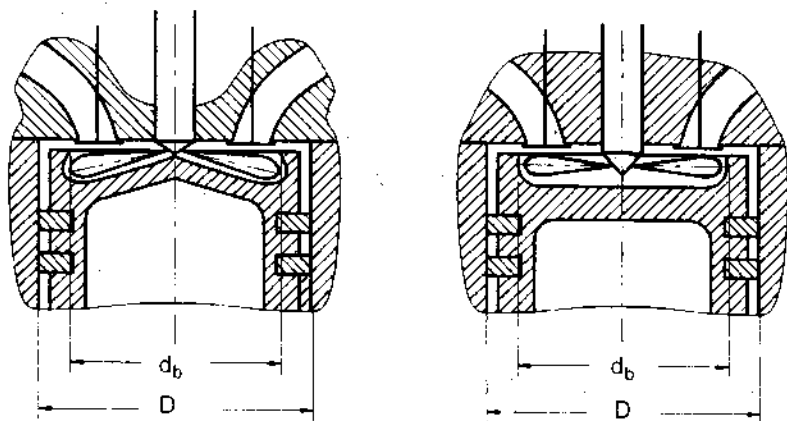
Hình 5-31. Buồng cháy thống nhất với phương pháp hỗn hợp thể tích
