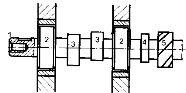
Hình 4-17. Trục cam
