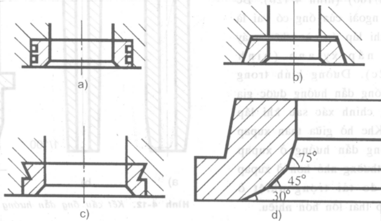
Hình 4-11. Kết cấu đế xupap
