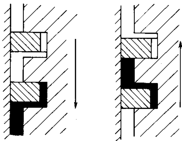
Hình 2.15. Hiện tượng bơm dầu của xecmăng khí
