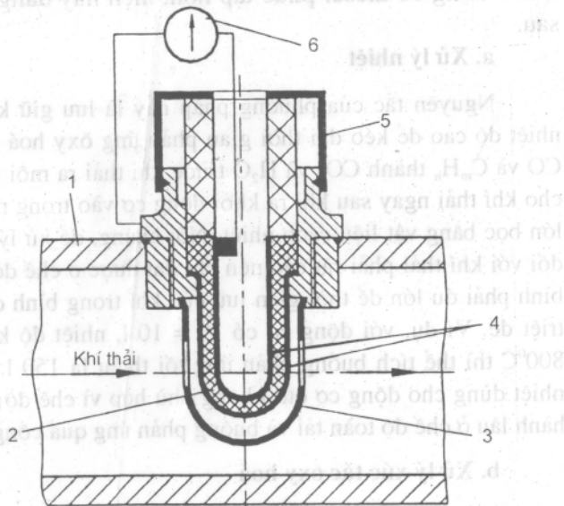
Hình 10.5. Cảm biến thành phần hệ số dư lượng không khí \lambda
