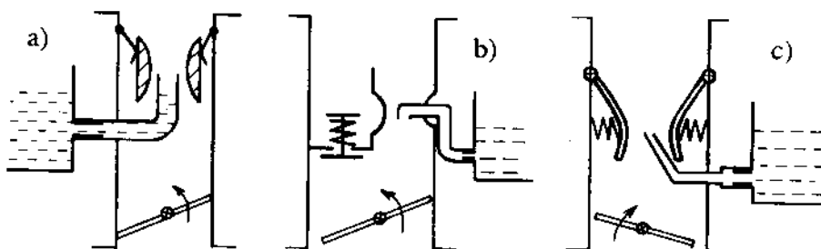
Hình 5-6. Hệ thống chính điều chỉnh độ chân không ở họng
