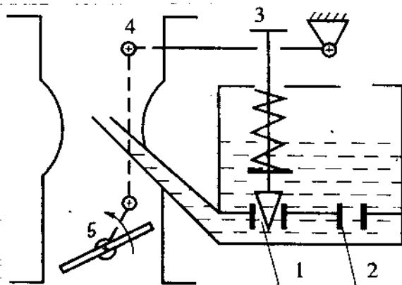
Hình 5-9. Hệ thống làm đậm cơ khí 1. giclô làm đậm, 2. giclô của hệ thống chính, 3. kim điều chỉnh, 4. đòn dẫn động, 5. bướm ga
