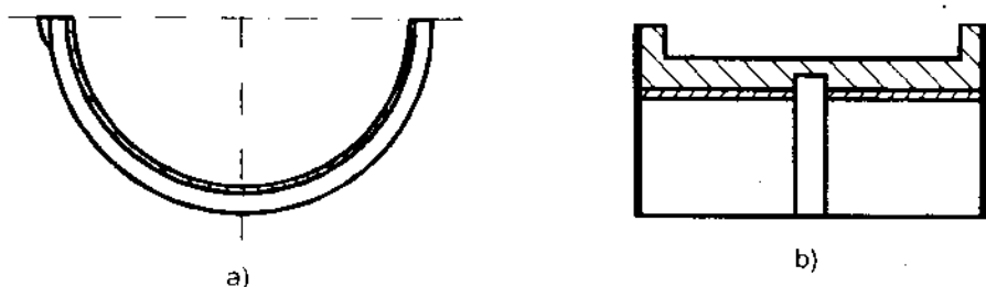
Hình 2-34. Bạc lót mỏng a) và bạc lót dày b)
