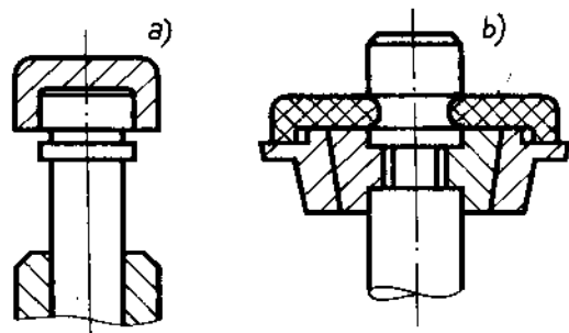
Hình 4-13. Kết cấu ngăn dầu ở đuôi xupap
