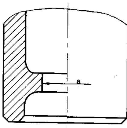
Hình 2-10. Kết cấu chân piston
