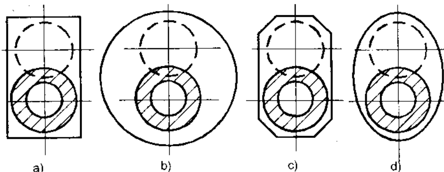
Hình 2-28. Các dạng má khuỷu
