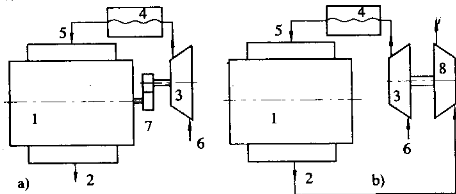
Hình 1-10. Tăng áp a) cơ khí, b) tuabin-máy nén
