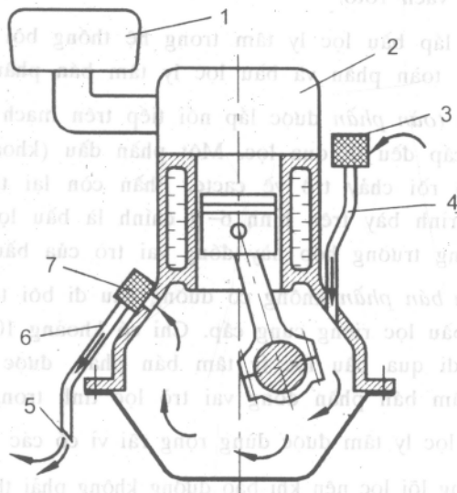
H 6-10. Thông gió hở (hộp trục khuỷu)
