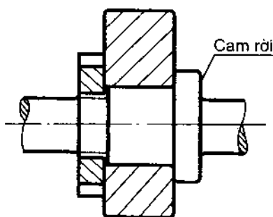
Hình 4-18. Cam rơ-lê lắp trên trục
