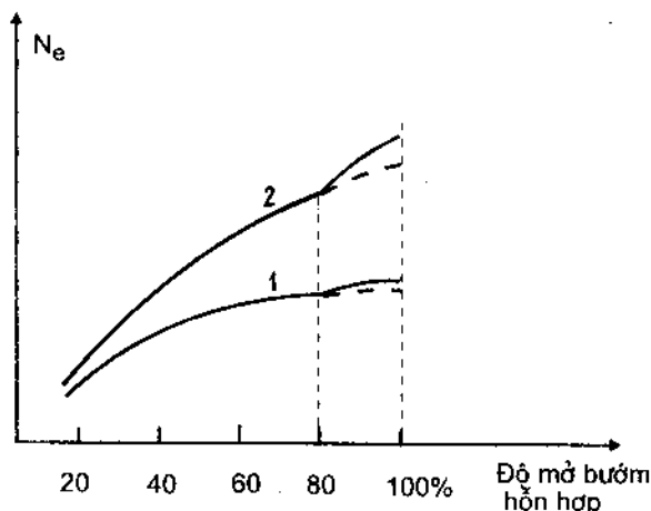
Hình 5-10. Đặc tính tải của động cơ khi làm đậm cơ khí
