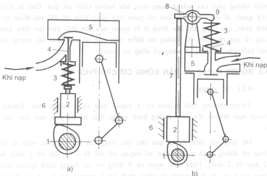
Hình 4-1. Cơ cấu phối khí dùng xupap
