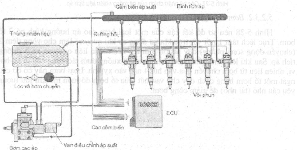
Hình 5-26. Sơ đồ hệ thống nhiên liệu tích áp
