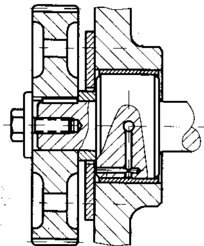
Hình 4-21. Chấn dọc trục cam
