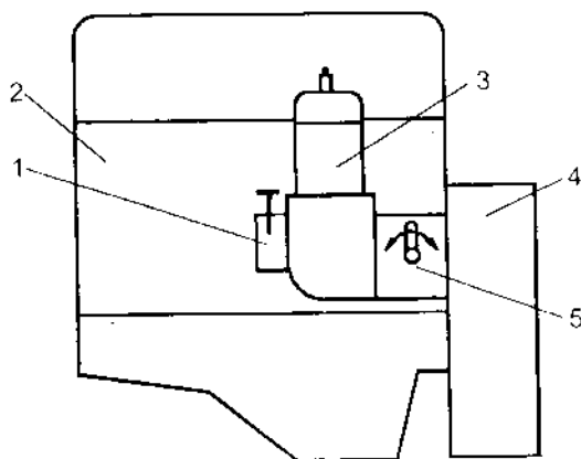
Hình 9-3. Hệ thống khởi động bằng động cơ xăng phụ 1. cơ cấu khởi động cơ phụ, 2. động cơ chính, 3. động cơ xăng phụ, 4. hộp bánh đà, 5. ly hợp
