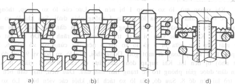
Hình 4-8. Kết cấu đuôi xupap
