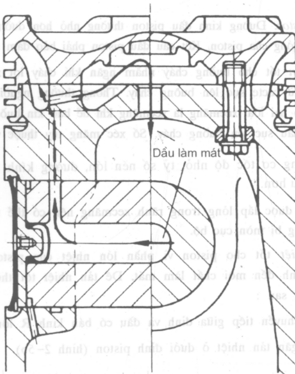
Hình 2-6. Dầu piston rỗng, làm mát bằng dầu lưu thông
