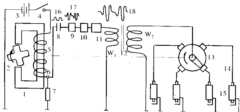
1. khung từ, 2. rô-lô, 3. acqui, 4. khóa điện, 5. cuộn dây, 6. điểm nối, 7. điện trở mạch sơ cấp, 8. tụ điện, 9. bộ rung bán dẫn, 10. bộ chuyển pha, 11. bộ khuếch đại, 12. biến áp đánh lửa, 13. bộ chia điện, 14. dây cao áp, 15. bugi, 16. xung điều khiển, 17. xung đã được môđun hóa, 18. xung sau khuếch đại.
