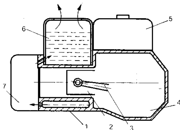
Hình 7-1. Hệ thống làm mát bốc hơi
