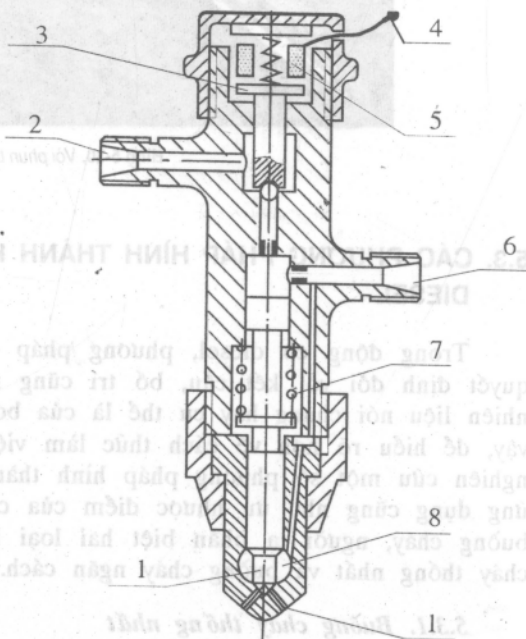
Hình 5-29. Vòi phun điện từ dùng trong hệ thống nhiên liệu tích áp
