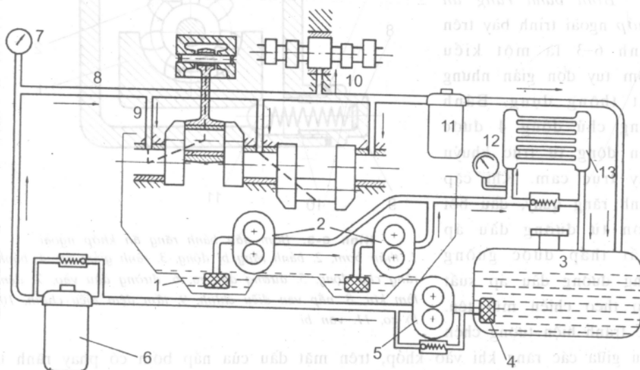
Hình 6-2. Hệ thống bôi trơn cacte khô
