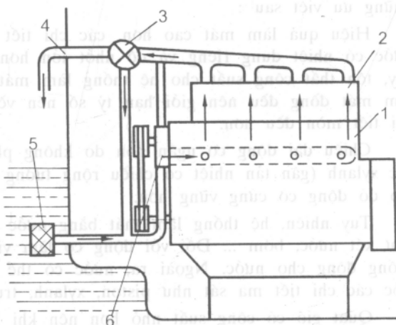
Hình 7-7. Hệ thống làm mát một vòng hở
