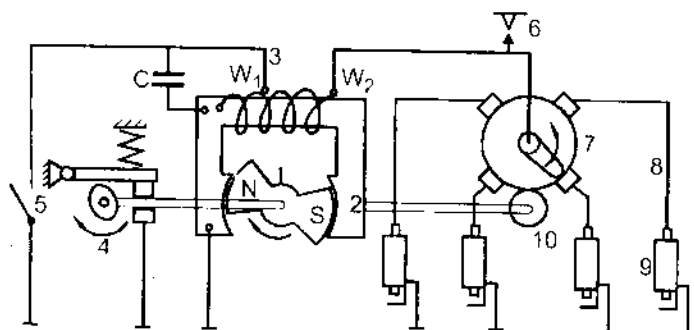
Hình 8-2. Hệ thống đánh lửa bằng nam châm
