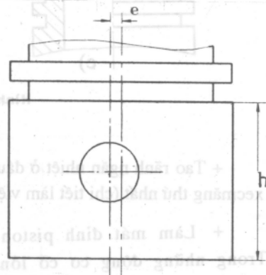
Hình 2-7. Thân piston
