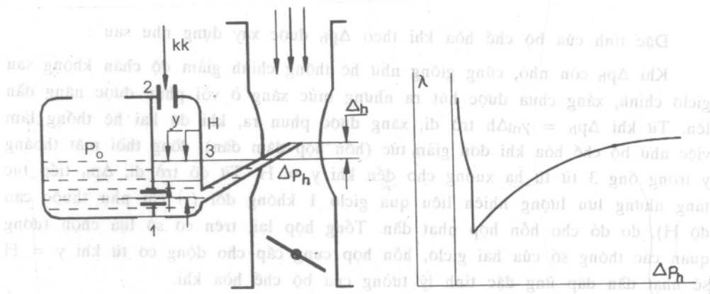
Hình 5-4. Hệ thống chính giảm độ chân không sau giclo chính
