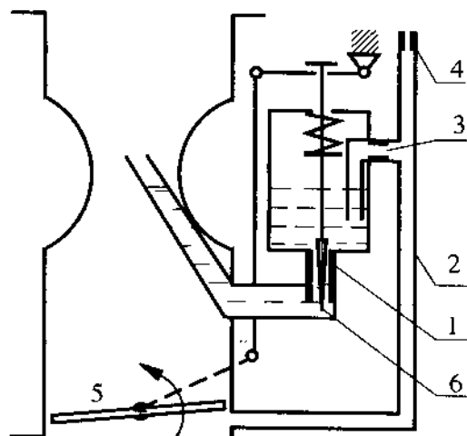
Hình 5-7. Hệ thống chính thay đổi tiết diện giclô kết hợp với hệ thống không tải
