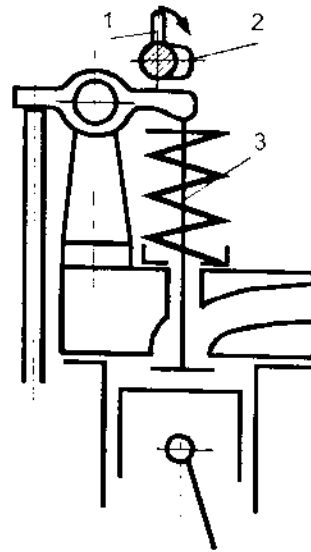
Hình 9-4. Cơ cấu giảm áp trên nắp xy lanh 1. Cam, 2. tay gạt, 3. xupap thải
