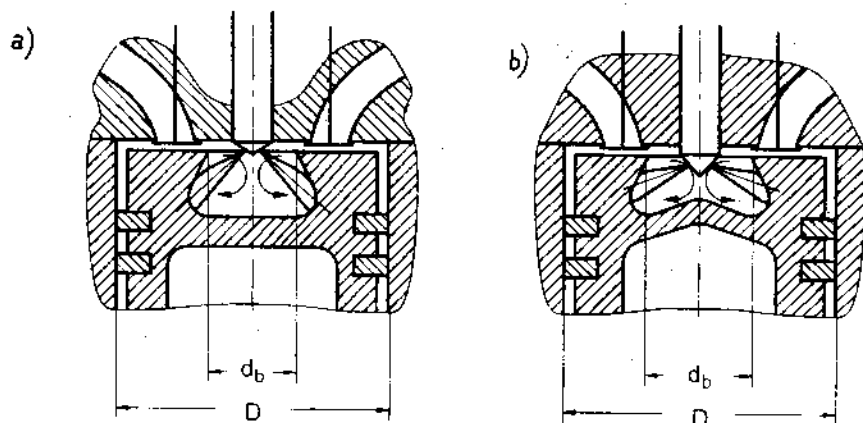
Hình 5-32. Buồng cháy với hỗn hợp thể tích-màng
