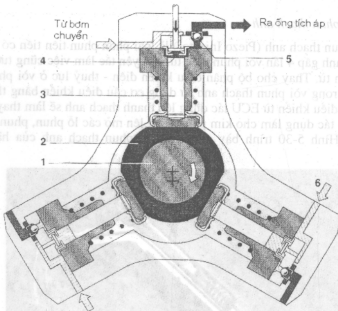
Hình 5-28. Bơm cao áp hướng kính dùng trong hệ thống nhiên liệu tích áp
