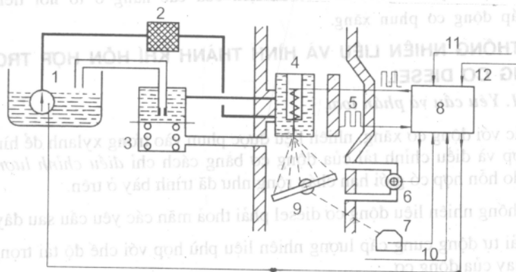
Hình 5-20. Hệ thống phun xăng Mono - Jetronic
