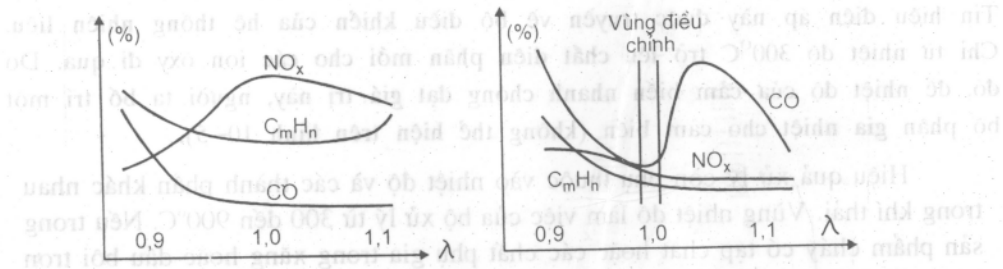
Hình 10.4. Thành phần độc hại của khí thải trước xử lý a) và sau xử lý b)
