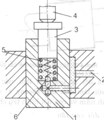
Hình 4-25. Nguyên lý làm việc con đội thủy lực
