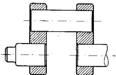
Hình 2-23. Trục khuỷu ghép
