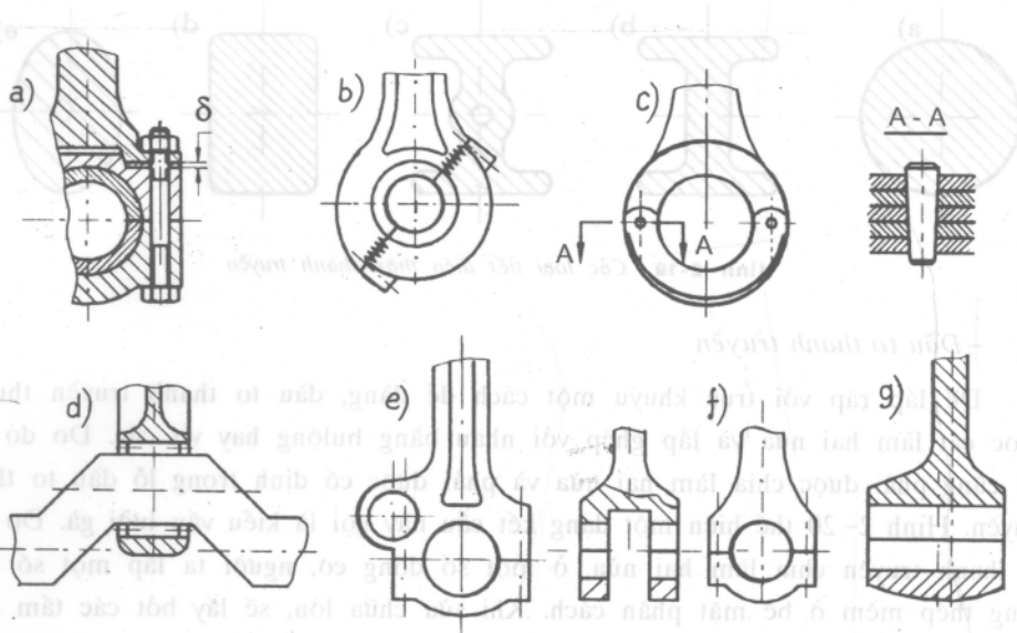
Hình 2.21. Các dạng kết cấu đầu to thanh truyền
