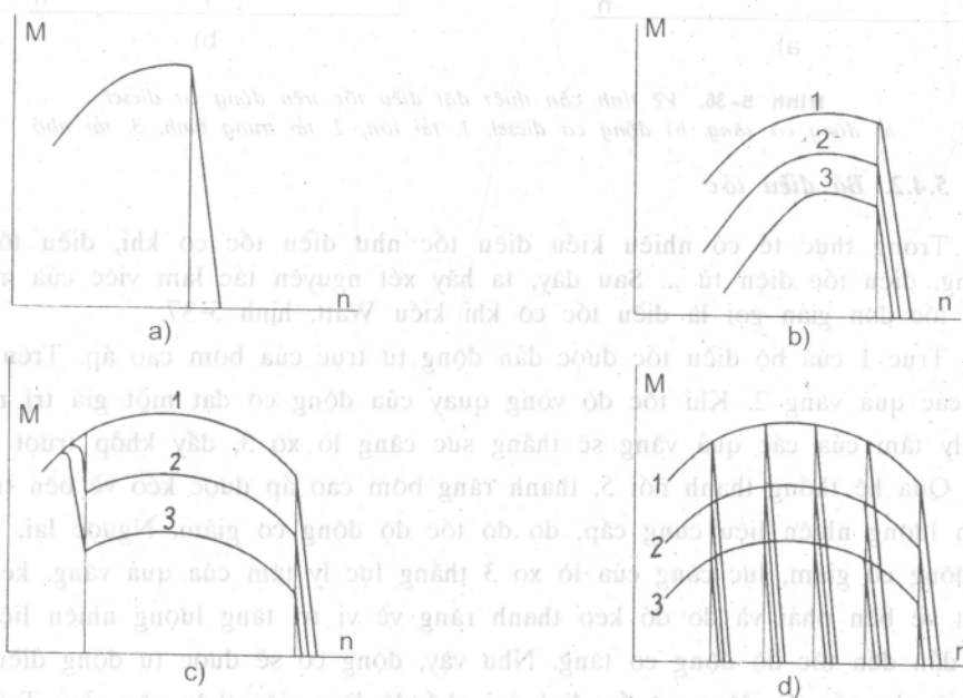
Hình 5-38. Đặc tính động cơ với các loại điều tốc
