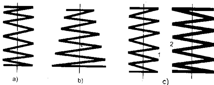
Hình 4-15. Các biện pháp kết cấu lò xo xupap tránh cộng hưởng
