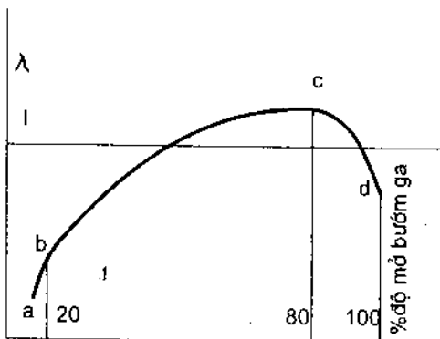
Hình 5-2. Đặc tính lý tưởng của bộ chế hòa khí
