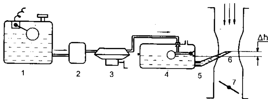
Hình 5-1. Sơ đồ hệ thống nhiên liệu dùng bộ chế hòa khí
