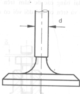
Hình 4-7. Thân xupap
