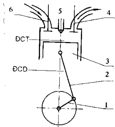
Hình 1-4. Sơ đồ động cơ 1. trục khuỷu, 2. thanh truyền, 3. piston, 4. xupap, 5. vòi phun (động cơ diesel) hoặc bugi (động cơ xăng), 6. xupap nạp, DCT. điểm chết trên, ĐCD. điểm chết dưới
