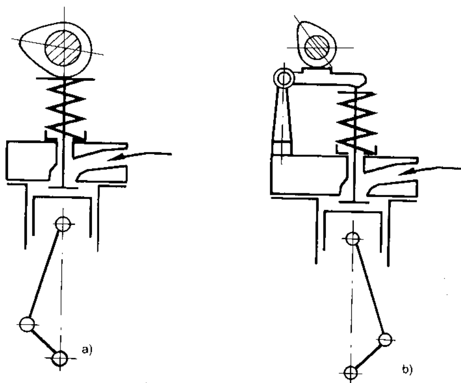
Hình 4-3. Dẫn động trực tiếp xupap
