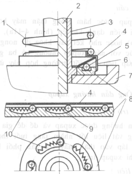
Hình 4-10. Kết cấu xupap tự xoay
