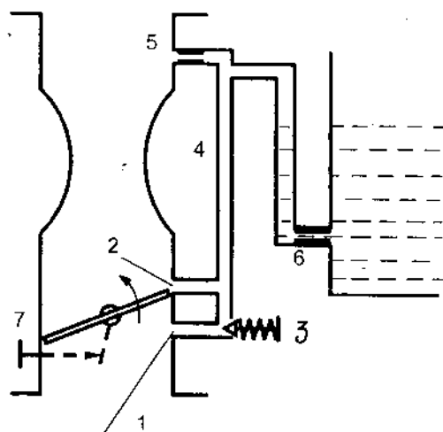
Hình 5-8. Hệ thống không tải
