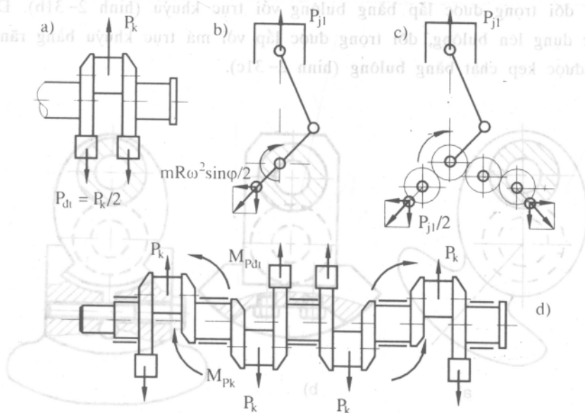
Hình 2-30. Vai trò của đối trọng
