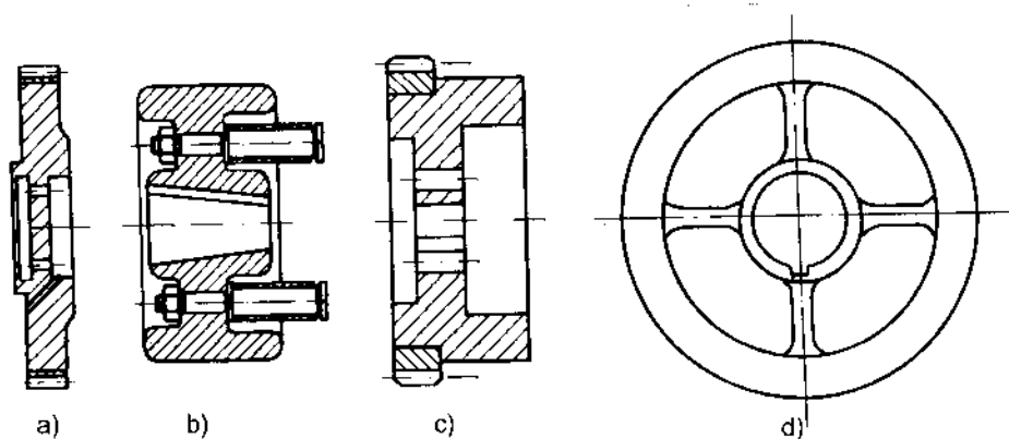
Hình 2-33. Kết cấu bánh đà
