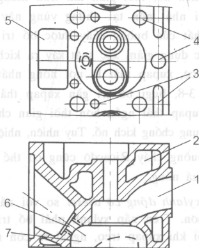
Hình 3-7. Buồng cháy bán cầu trong động cơ xăng
