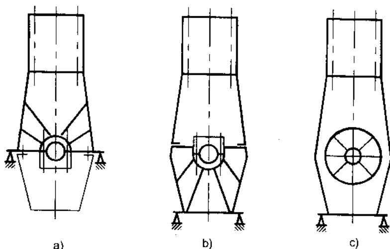
Hình 3-5. Các kiểu lắp đặt trục khuỷu
