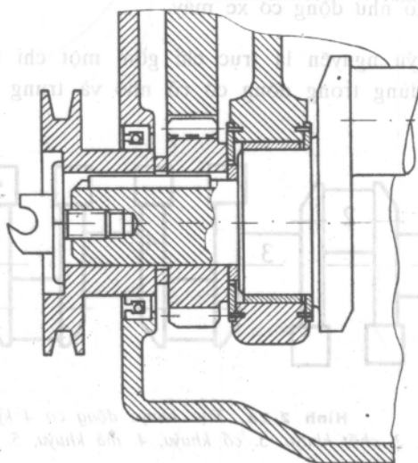
Hình 2-26. Một loại kết cấu đầu trục khuỷu động cơ ô tô
