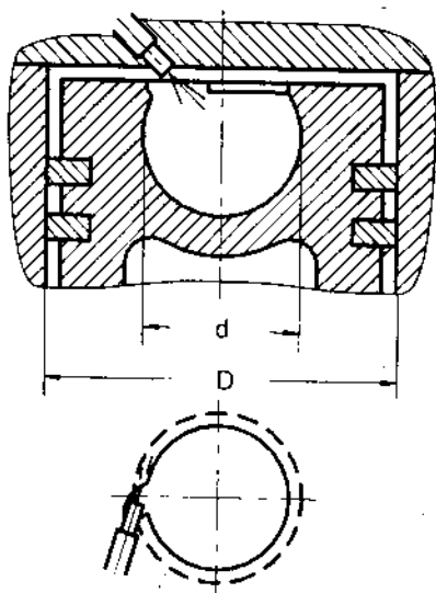
Hình 5-33. Buồng cháy hỗn hợp màng
