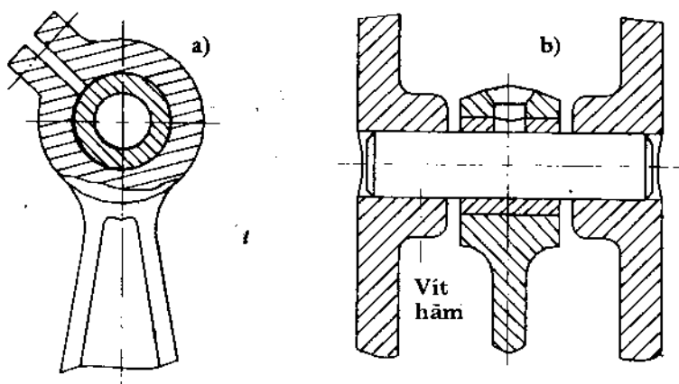
Hình 2-11. Lắp cố định chốt piston trên đầu nhỏ thanh truyền a) và trên bệ chốt b)
