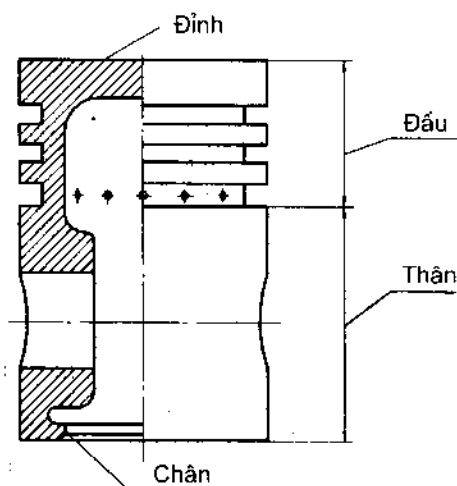
Hình 2-3. Kết cấu piston
