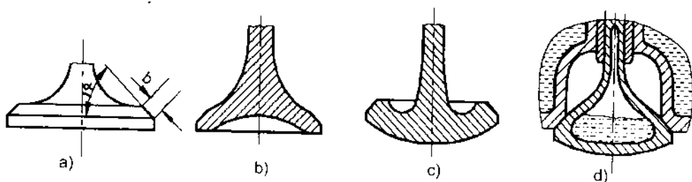
Hình 4-6. Kết cấu nấm xupap
