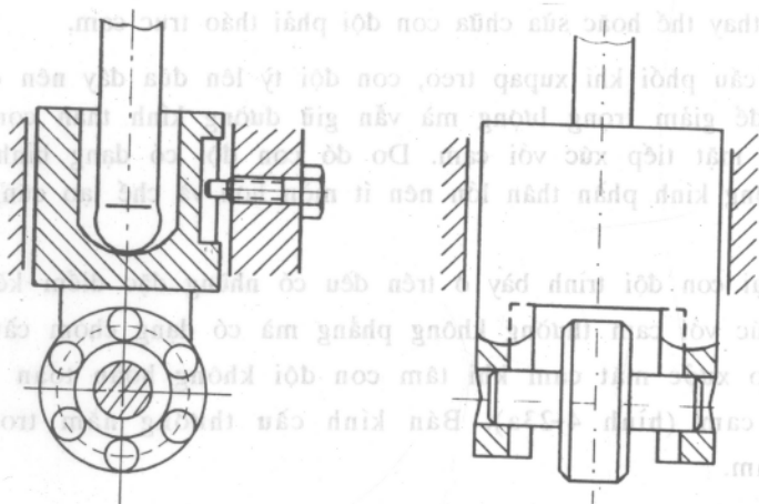
Hình 4-24. Con đội con lăn
