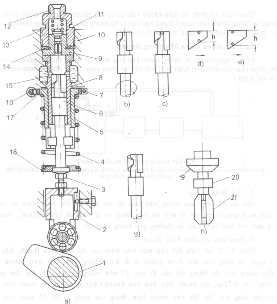
Hình 5-22. Bơm cao áp đơn kiểu Bosh
