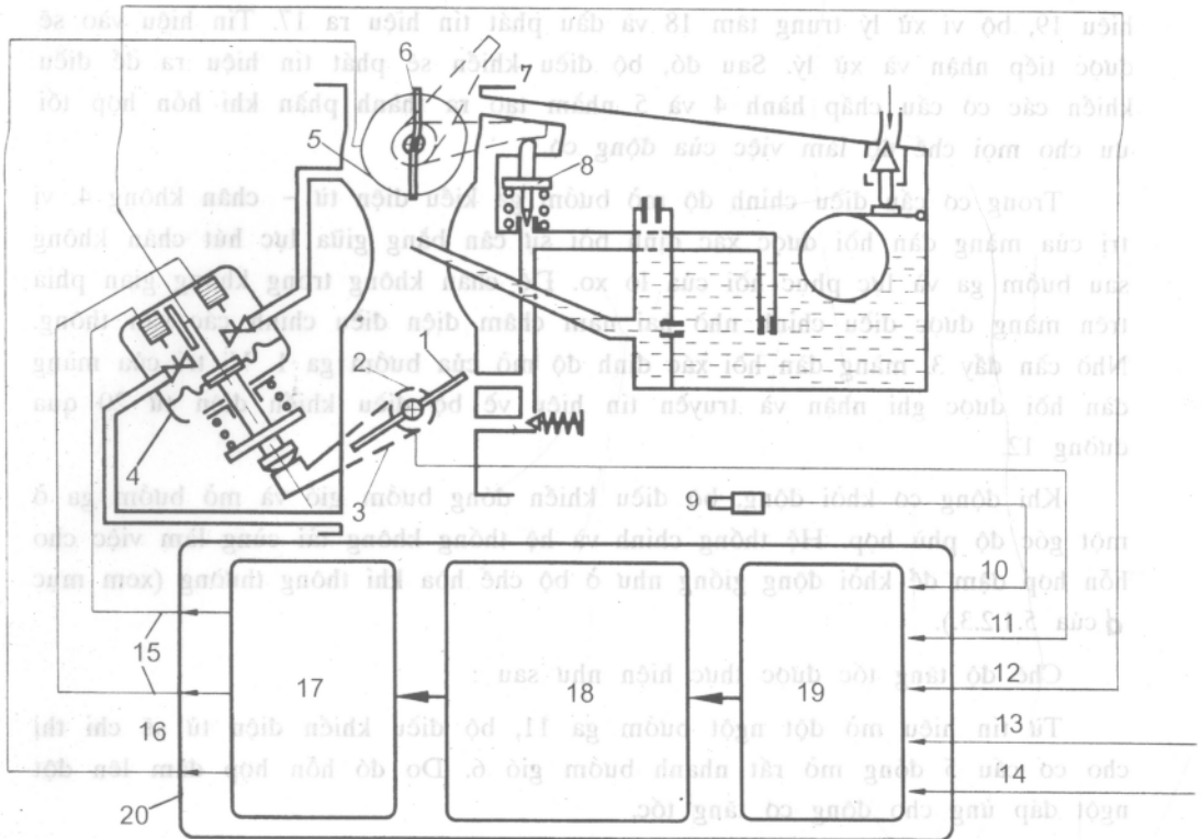
Hình 5-16. Bộ chế hòa khí điều khiển bằng điện tử
