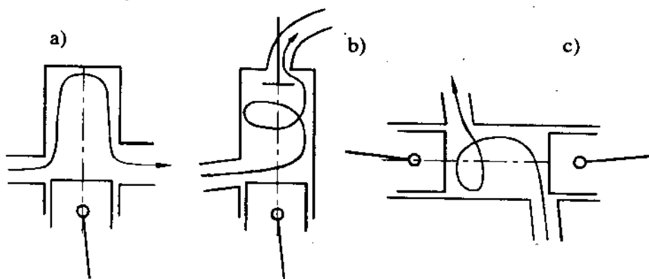
Hình 1-8. Các kiểu quét khí của động cơ 2 kỳ a) quét vòng, b) và c) quét thẳng
