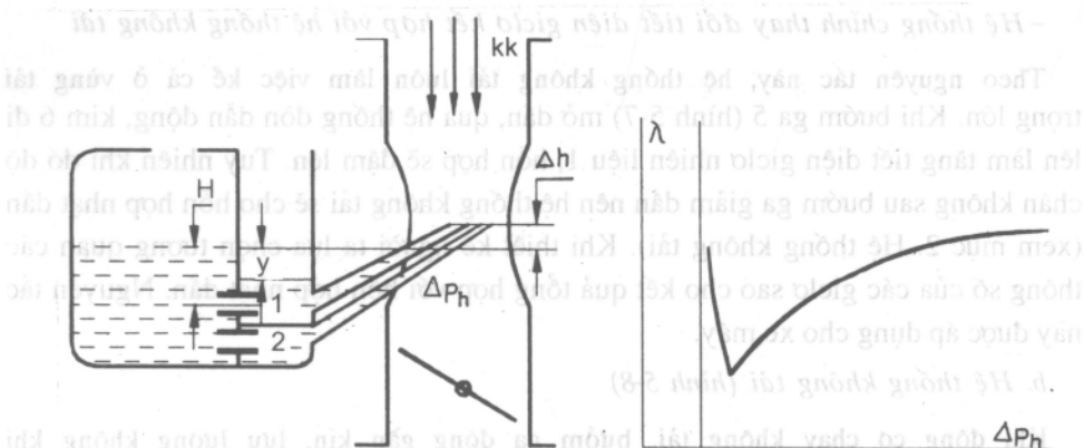
Hình 5-5. Hệ thống chính là giclo bổ sung
