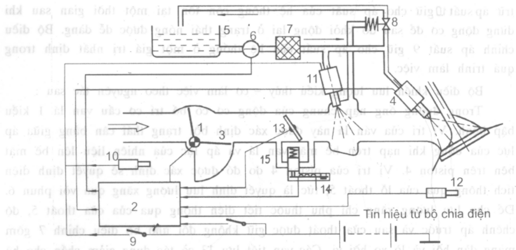
Hình 5-19. L-Jectronic
