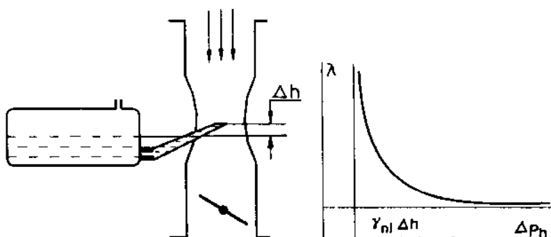
Hình 5-3. Đặc tính bộ chế hòa khí đơn giản
