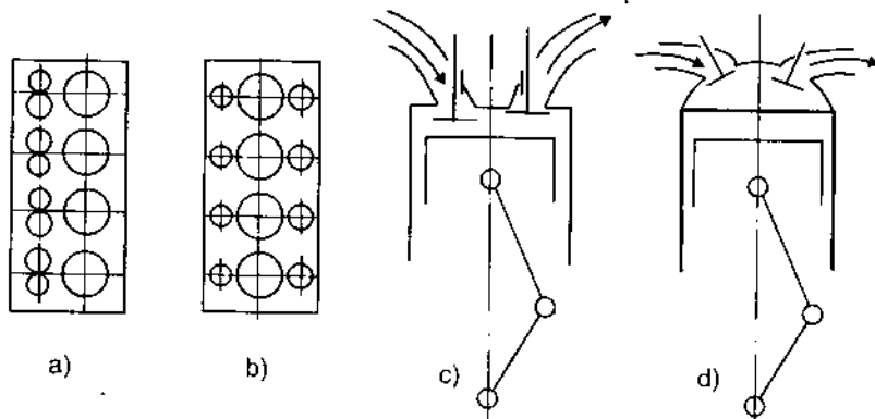
Hình 4-2. Bố trí xupap
