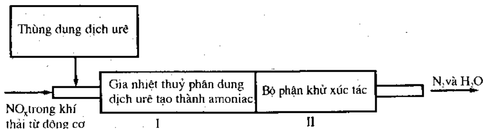
Hình 10-6. Xử lý xúc tác khử \text{NO}_x
