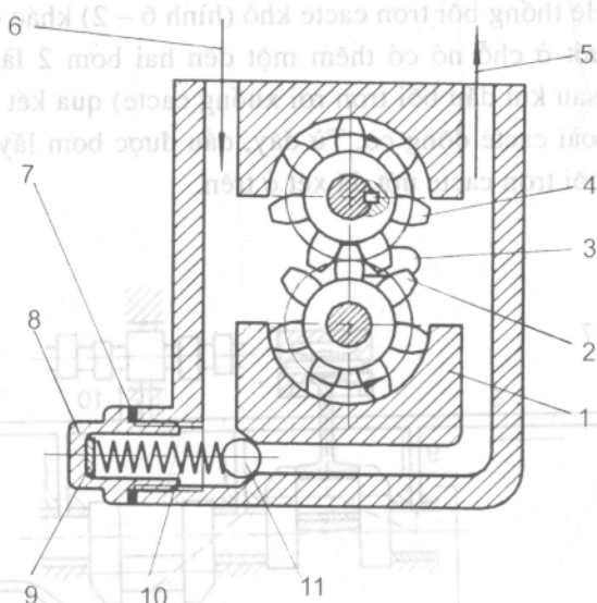
Hình 6-3. Bơm dầu bánh răng ăn khớp ngoài 1. thân bơm, 2. bánh răng bị động, 3. rãnh giảm áp, 4. bánh răng chủ động, 5. đường dầu ra, 6. đường dầu vào, 7. đệm làm kín, 8. nắp van điều chỉnh, 9. tấm đệm điều chỉnh, 10. lò xo, 11. van bi
