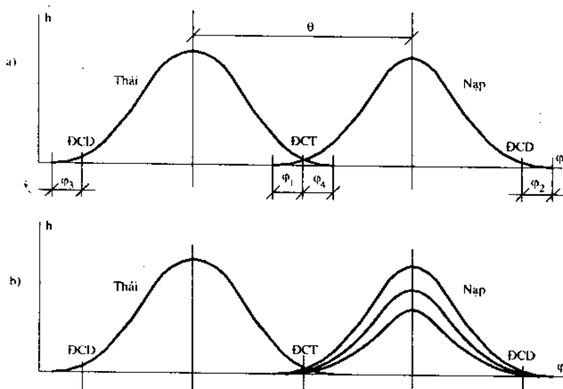
Hình 4-20. Hành trình xupap nạp và thải của một xy lanh
