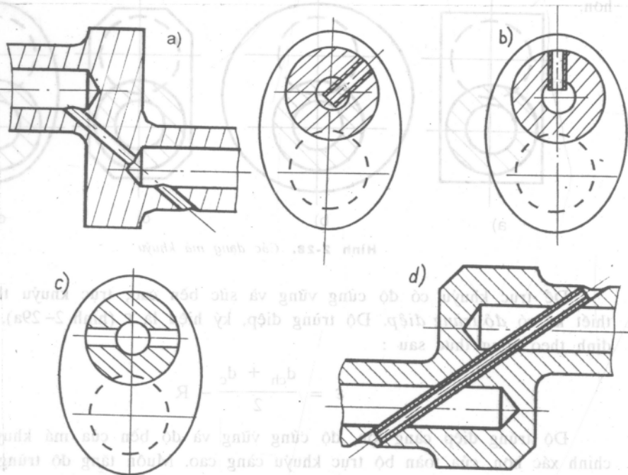
Hình 2-27. Kết cấu dẫn dầu bôi trơn chốt khuỷu
