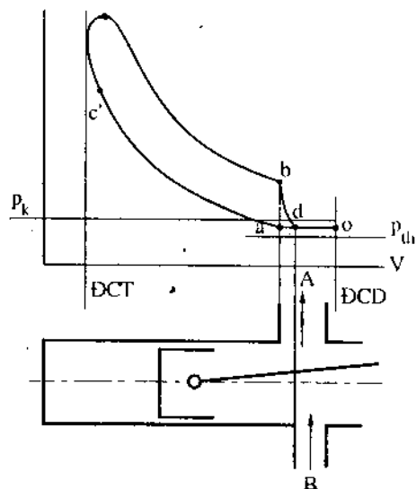
Hình 1-7. Nguyên lý làm việc của động cơ 2 kỳ
