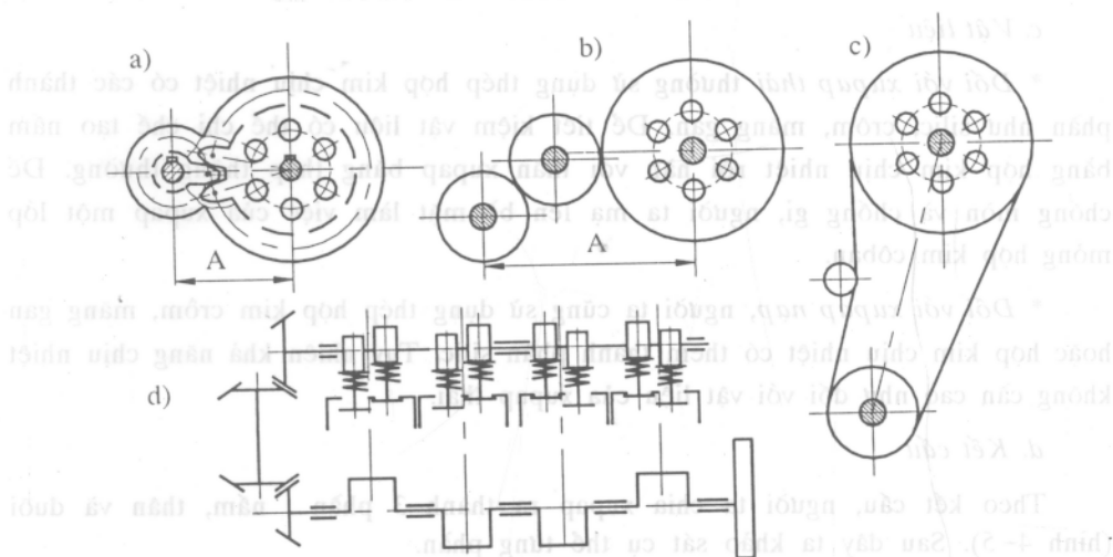
Hình 4-4. Dẫn động trực cam
