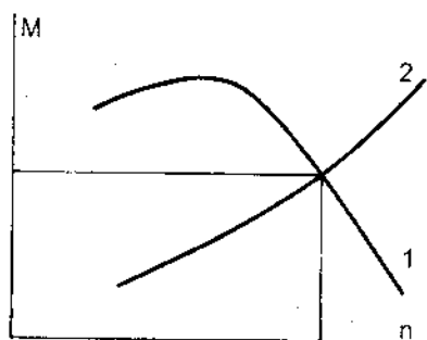
Hình 5-35. Đặc tính của động cơ và máy công tác 1. mômen động cơ, 2. mômen cản của máy công tác
