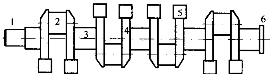
Hình 2-24. Trục khuỷu động cơ 4 kỳ, 4 xylanh
