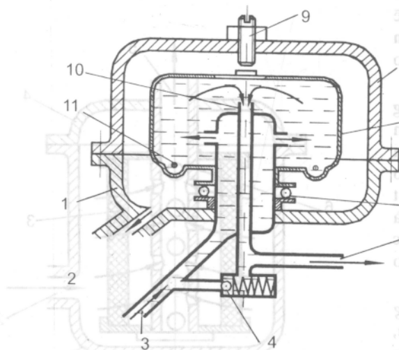
Hình 6-9. Bầu lọc ly tâm
