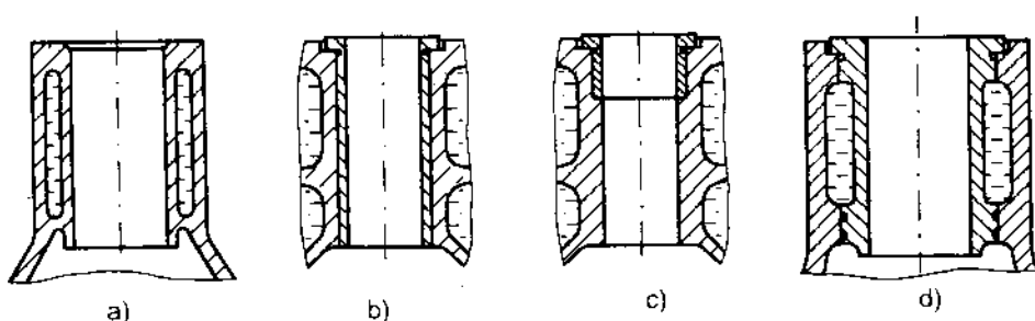
Hình 3-5. Các loại xylan a) thân xylan, b) và c) lót xylan khô, d) lót xylan ướt
