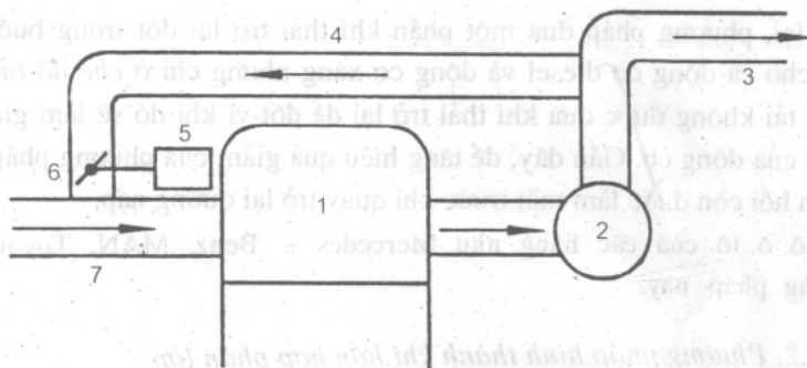
Hình 10-1. Sơ đồ động cơ sử dụng luân hồi khí thải
