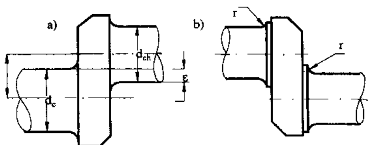
Hình 2-29. Các biện pháp kết cấu tăng bền má khuỷu
