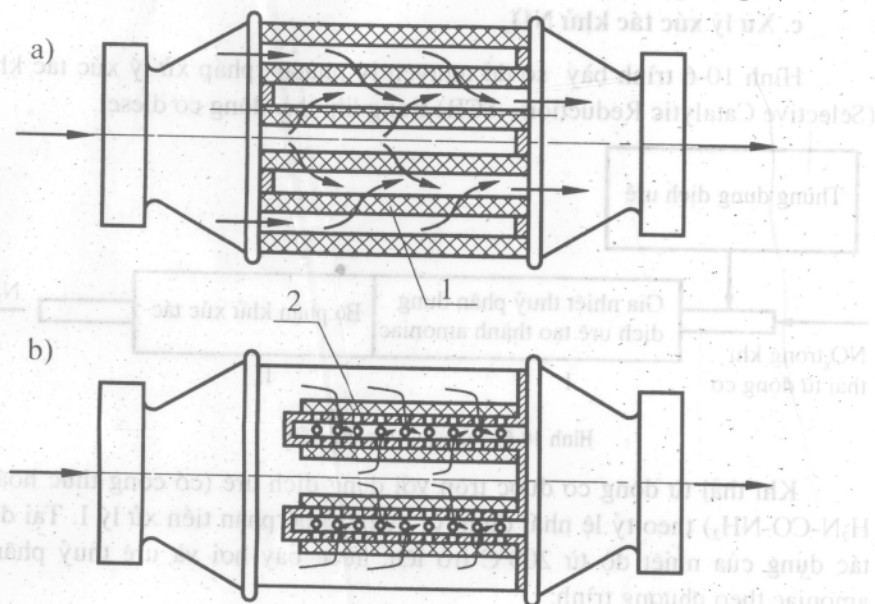
Hình 10-7. Lọc muối than trong khí thải động cơ diesel.
