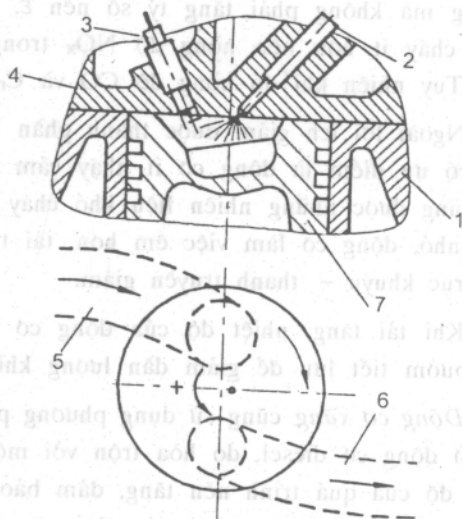
Hình 10-2. Phương pháp hình thành khí hỗn hợp phân lớp Ford Proco 1. xylanh, 2. vòi phun, 3. bugi, 4. nắp xylanh, 5. đường nạp, 6. đường thải, 7. piston
