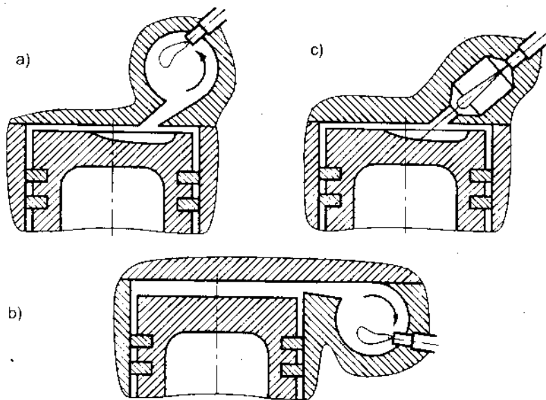
Hình 5-34. Buồng cháy ngăn cách a) và b) buồng cháy xoáy lốc, c) buồng cháy dự bị
