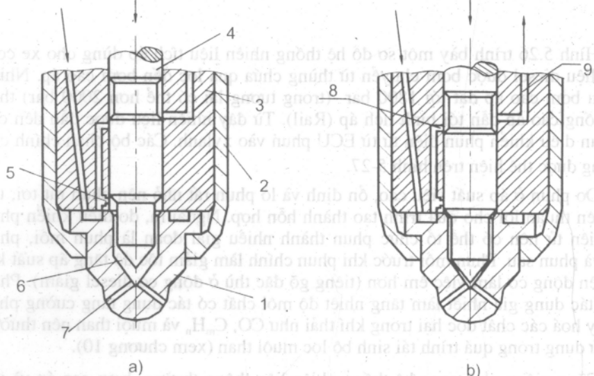
Hình 5-25. Bơm cao áp - vòi phun
