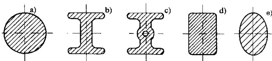
Hình 2-19. Các loại tiết diện thân thanh truyền
