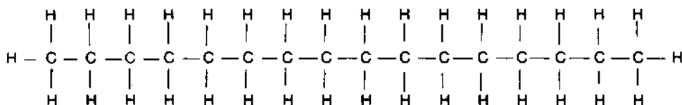
Hình 1-1. Xêtan C_{16}H_{34} , một loại cacbua-hydrô no mạch thẳng
