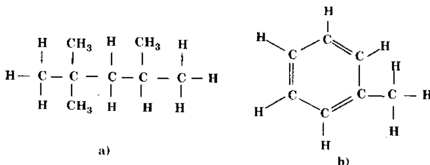
Hình 1-3. Sơ đồ cấu tạo phân tử : a) isooctan C_8H_{18} và b) metylbenzen C_6H_5CH_3
