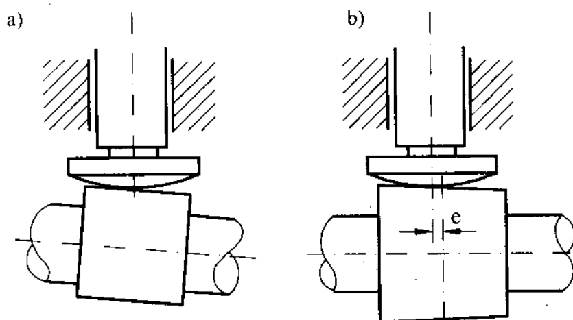
Hình 4-23. Một số đặc điểm kết cấu của con đội hình nấm và con đội hình trụ
