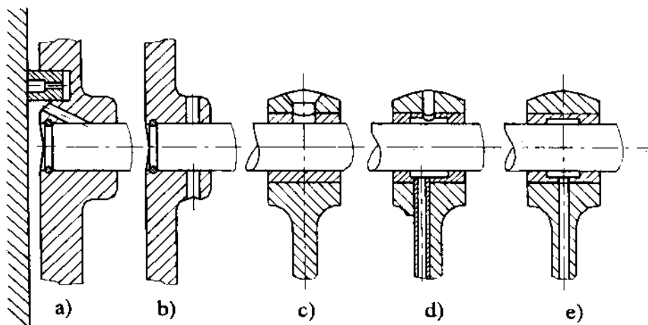
Hình 2-13. Bôi trơn các mối ghép chốt piston
