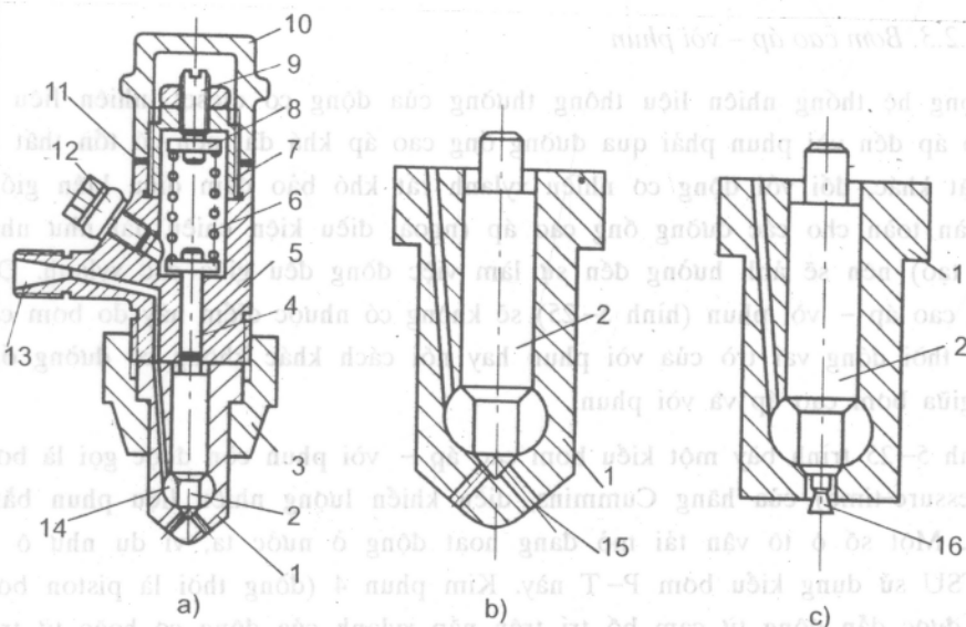
Hình 5-24. Vòi phun.
