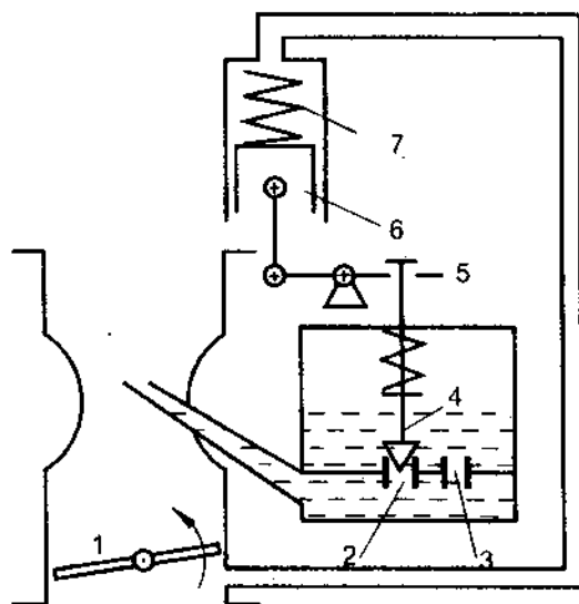
Hình 5-11. Hệ thống làm đậm chân không 1. bướm ga, 2. giclơ làm đậm, 3. giclơ hệ thống chính, 4. kim điều chỉnh làm đậm, 5. đòn dẫn động, 6. piston, 7. lò xo
