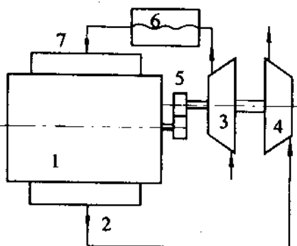
Hình 1-11. Tăng áp hỗn hợp 1. động cơ, 2. đường thải, 3. máy nén, 4. tuabin, 5. bộ truyền cơ khí, 6. bình làm mát trung gian, 7. đường nạp
