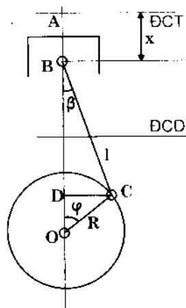
Hình 2-1. Sơ đồ của cơ cấu trục khuỷu - thanh truyền
