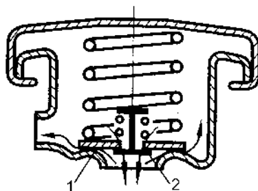
Hình 7-5. Nắp kết nước 1. van xả, 2. van hút
