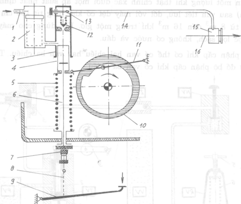
Hình 61. Bộ phận cấp nước cho đầu phun máy dẹt nước:
