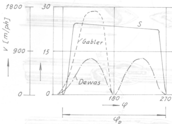
Hình 32. Tốc độ đưa sợi ngang phụ thuộc vào góc quay trục chính máy dệt: v - tốc độ đưa sợi ngang [m/phút]; \varphi - góc quay trục chính máy dệt; \varphi_p - góc quay trục chính máy dệt ứng với thời gian đưa sợi ngang.
