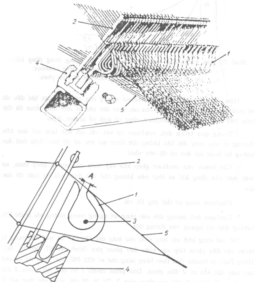
Hình 54. Vị trí của confusor khi đưa sợi ngang vào miệng vải: 1 - confusor, 2 - khổ, 3 - sợi ngang, 4 - batăng, 5 - sợi dọc.
