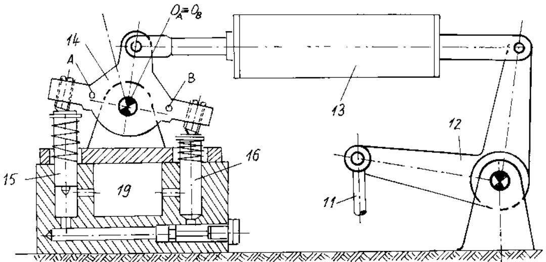
Hình 69. Sơ đồ truyền động từ đầu tay kéo đến bộ phận đổi sợi ngang.
