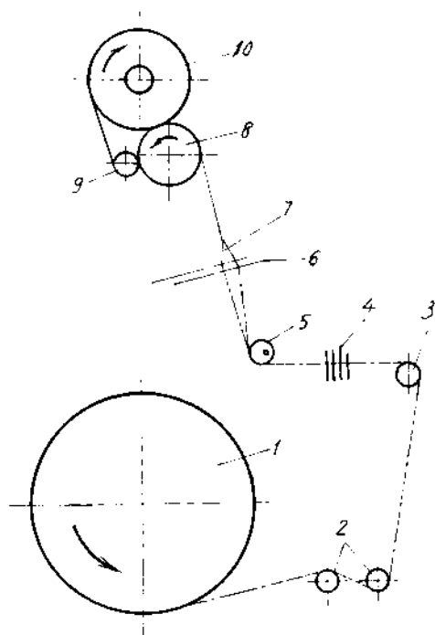
Hình 119. Sơ đồ công nghệ máy dệt nhiều miệng vải
