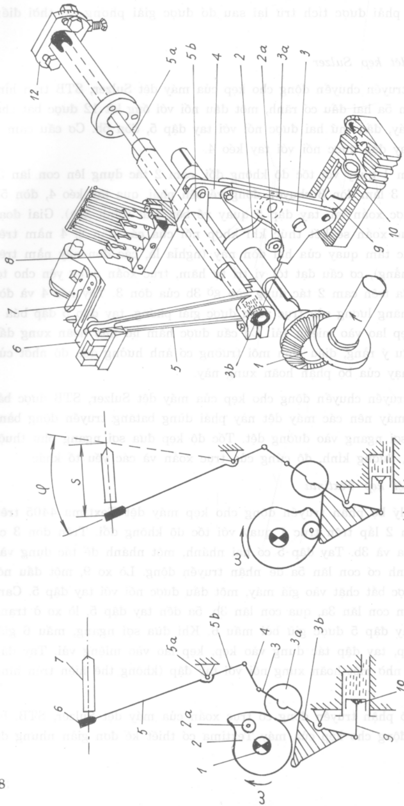
Hình 22. Cơ cấu truyền chuyển động cho kẹp máy dệt Sulzer (STB).
