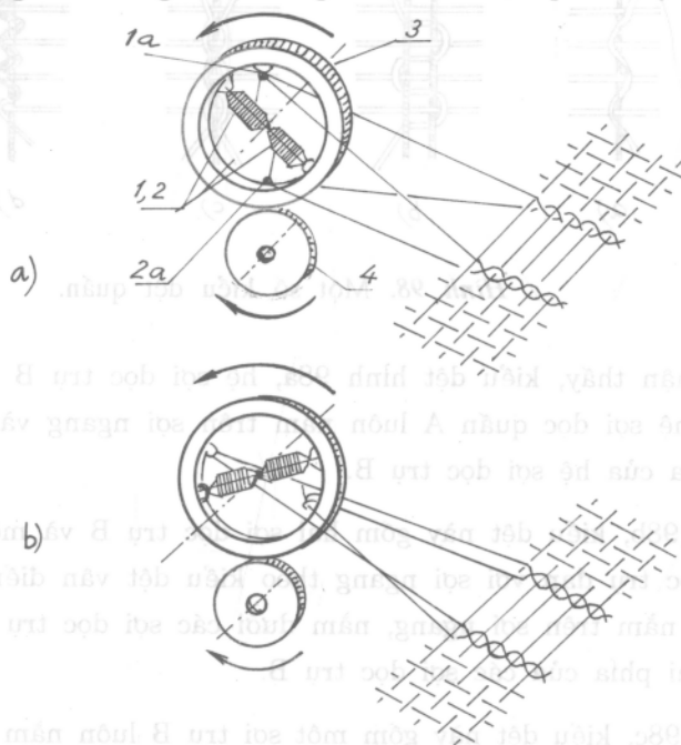
Hình 99. Cơ cấu dệt biên quần : a) Miệng vải mở ; b) Miệng vải đóng.
