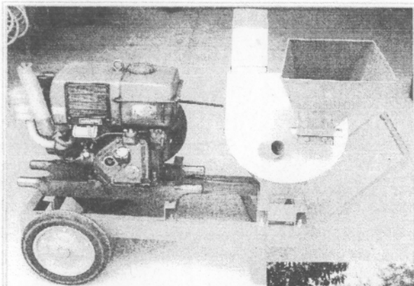
Máy thái cỏ với động cơ Diesel
