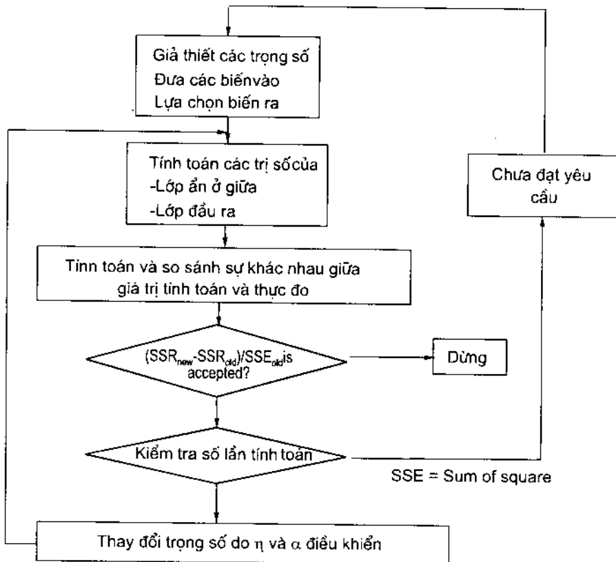
Hình 3.4: Sơ đồ khối của thuật toán lan truyền ngược
