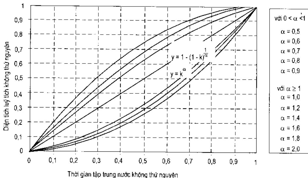
Hình 2.4: Các đường cong thời gian tập trung nước và lũy tích diện tích theo thời gian của thời gian tập trung nước trong mô hình MOUSE
