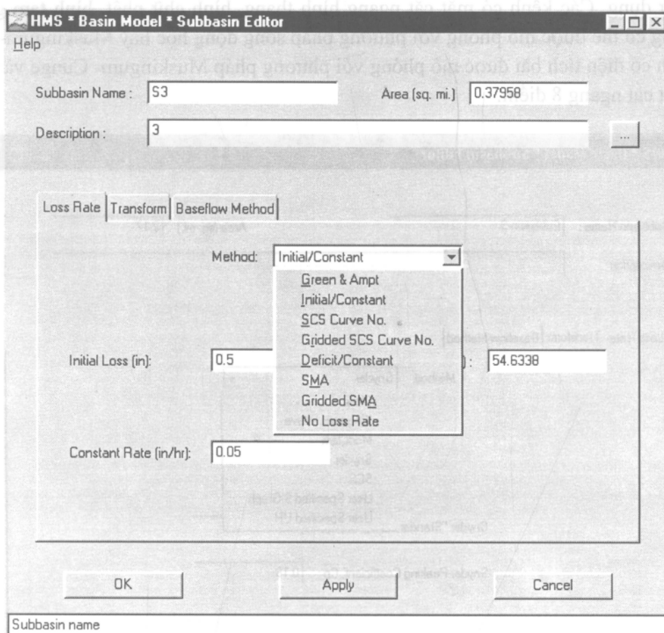
Hình 2.7: Cửa sổ lựa chọn phương pháp tính tồn thất
