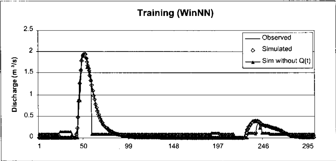
Hình 3.11: So sánh đường quá trình tính toán và thực đo (training - hiệu chỉnh)
