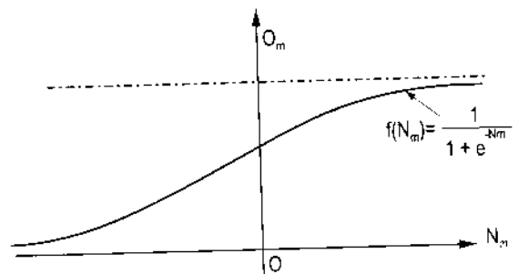
Hình 3.3: Hàm kích hoạt Logistic
