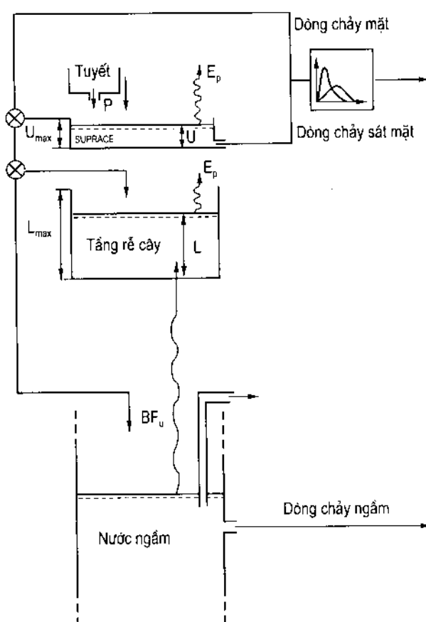
Hình 2.11: Sơ đồ mô phỏng của mô hình NAM
