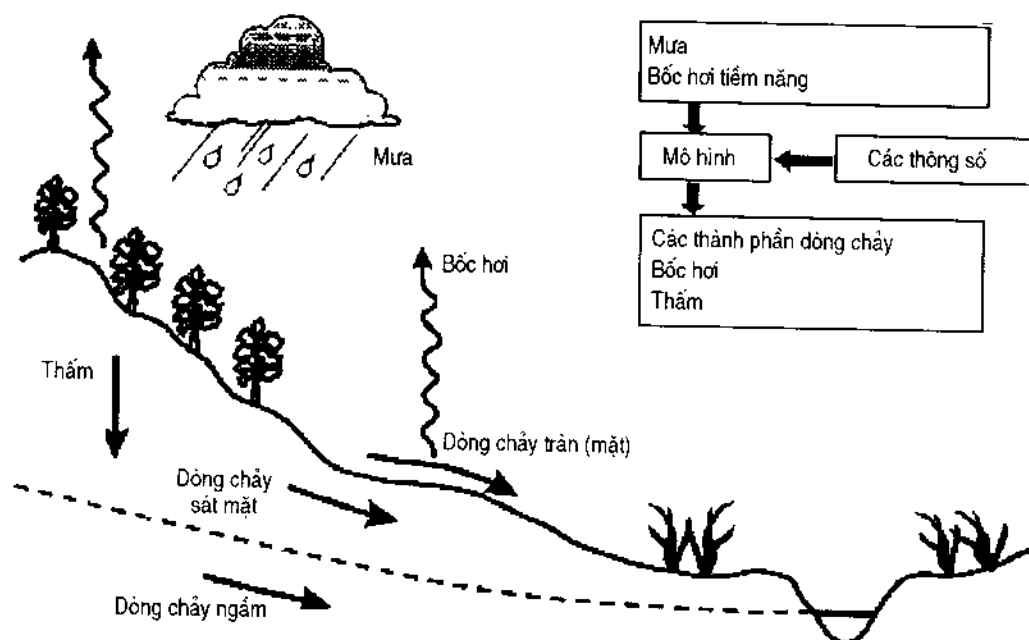
Hình 2.1: Quá trình hình thành dòng chảy
