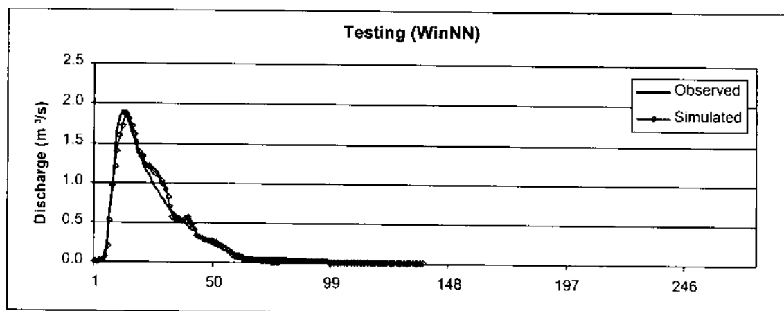
Hình 3.14: Đường quá trình lưu lượng thực đo và tính toán trong giai đoạn kiểm định mô hình (testing)
