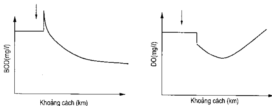
Hình 5.2: Sự biến đổi của BOD và DO dọc theo dòng chảy
