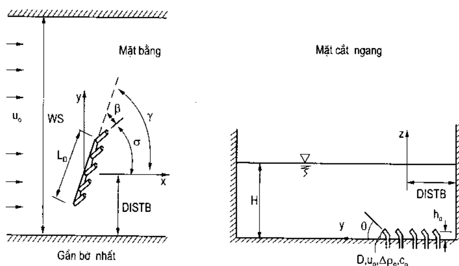
Hình 5.5: Sơ đồ đặc trưng lòng dẫn nước thải trong CORMIX 2
