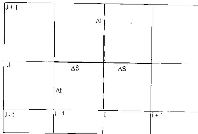
Hình 4.3: Sơ đồ sai phân bốn điểm hình thoi
