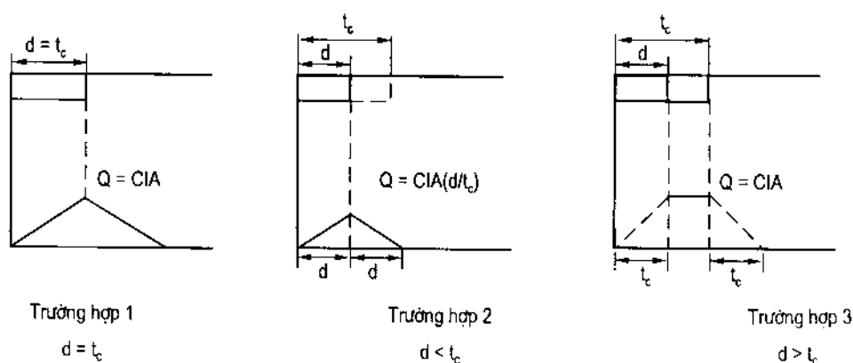
Hình 2.3: Đường quá trình lũ cho các thời khoảng mưa khác nhau
