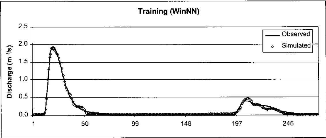
Hình 3.13: Đường quá trình lưu lượng thực đo và tính toán trong giai đoạn hiệu chỉnh mô hình (training)
