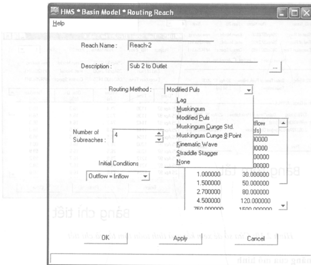
Hình 2.9: Cửa sổ lựa chọn phương pháp diễn toán dòng chảy trên sông hay kênh hở
