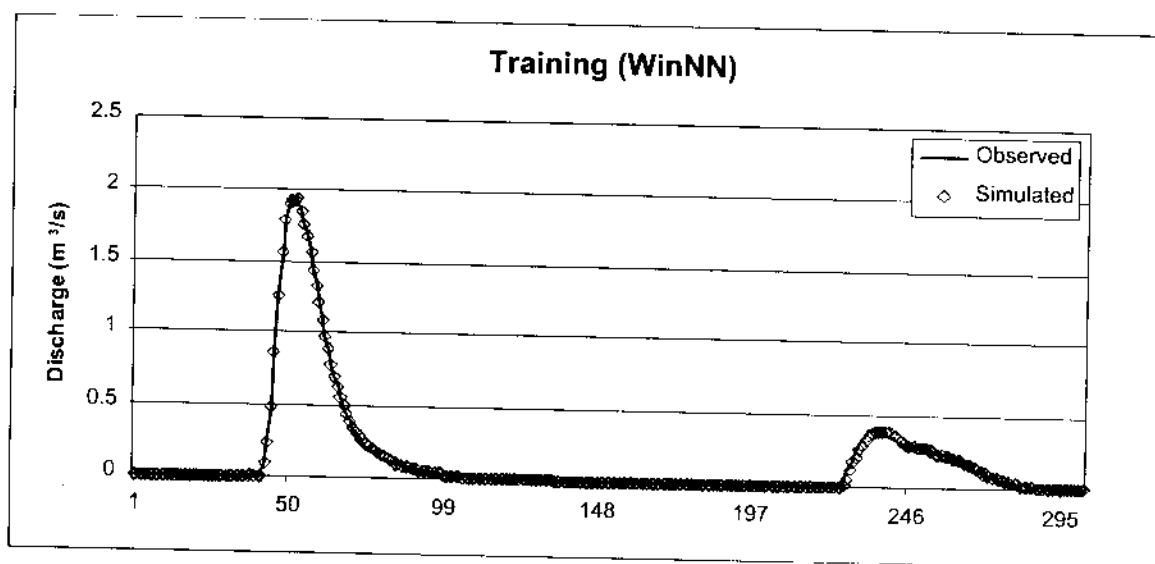
Hình 3.9: So sánh quá trình thực đo và tính toán (Training - hiệu chỉnh)
