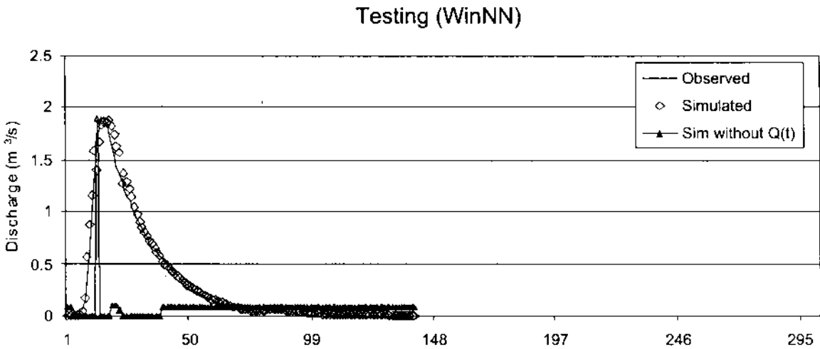
Hình 3.12: So sánh đường quá trình tính toán và thực đo (testing - kiểm định)
