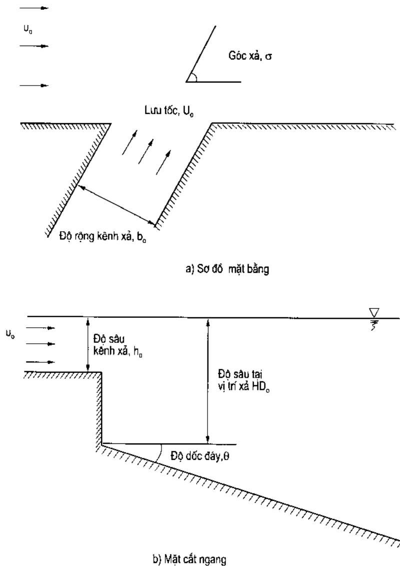
Hình 5.6: Đặc trưng hình học kênh xả của CORMIX3
