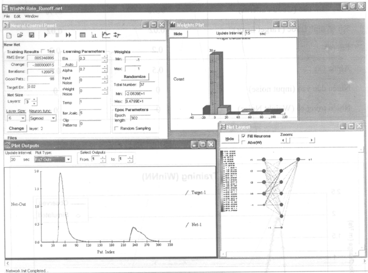
Hình 3.8: Chạy mô hình WinNN32
