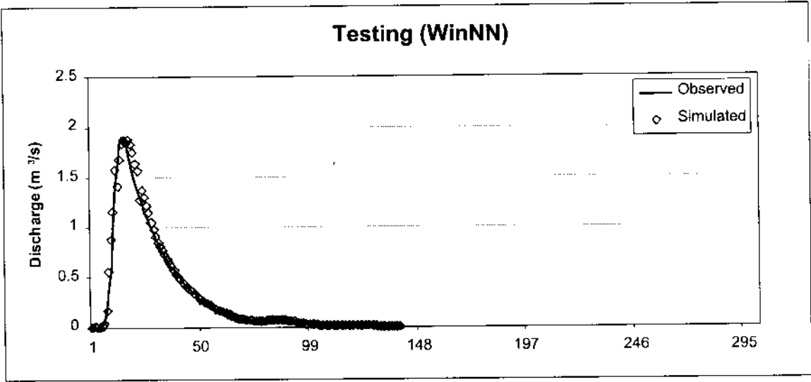
Hình 3.10: So sánh quá trình thực đo và tính toán (Testing - Kiểm định)
