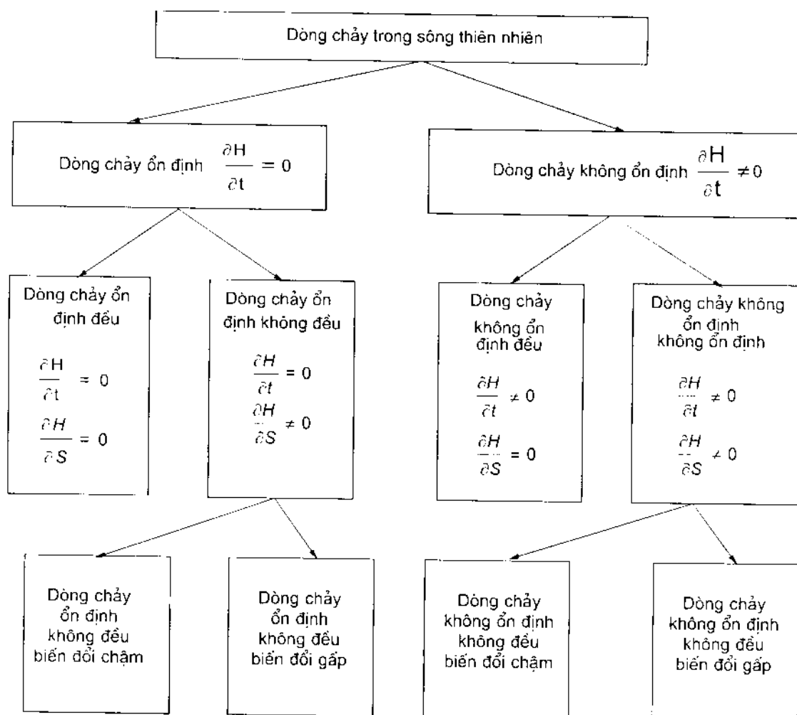
Hình 4.1: Sơ đồ phân chia dòng chảy trong sông thiên nhiên
