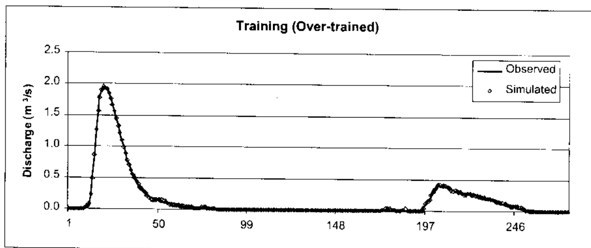
Hình 3.15: Đường quá trình lưu lượng thực đo và tính toán trong giai đoạn hiệu chỉnh mô hình (mô hình bị đào tạo quá mức – over trained)
