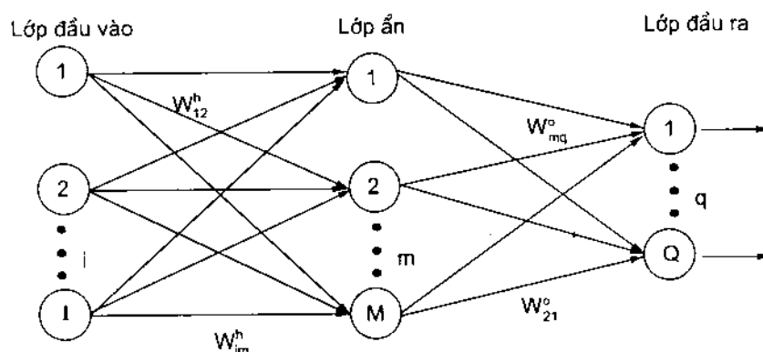
Hình 3.1: Mạng nơron thần kinh 3 lớp
