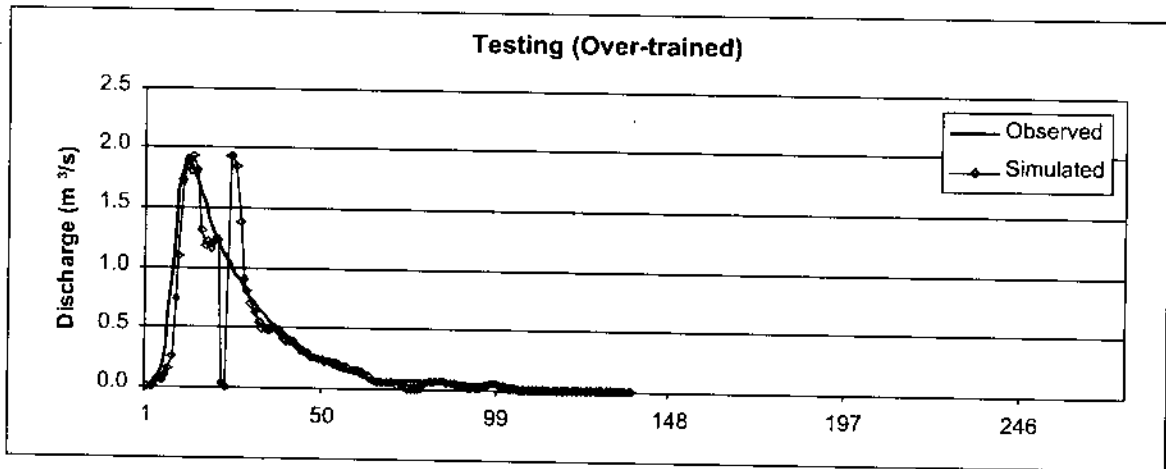
Hình 3.16: Đường quá trình lưu lượng thực đo và tính toán trong giai đoạn kiểm định mô hình (mô hình bị đào tạo quá mức – over trained)
