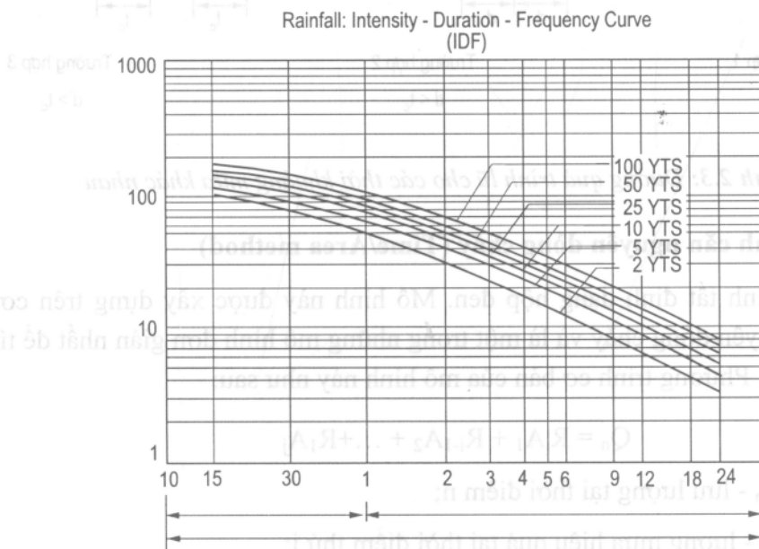
Hình 2.2: Ví dụ về đường cong IDF cho khu vực Bangkok, Thailand
