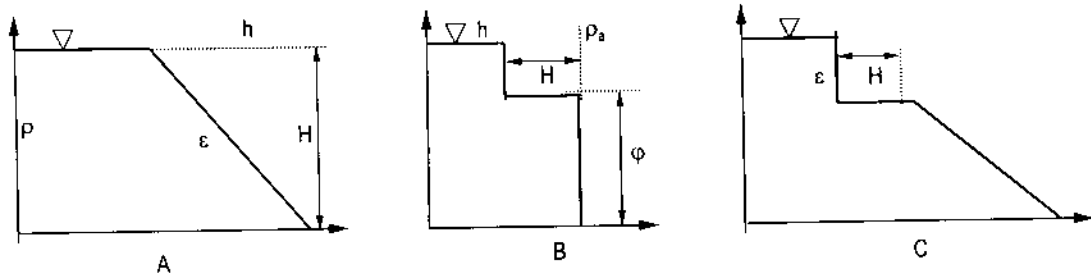
Hình 5.3: Các kiểu phân bố mật độ theo phương thẳng đứng
