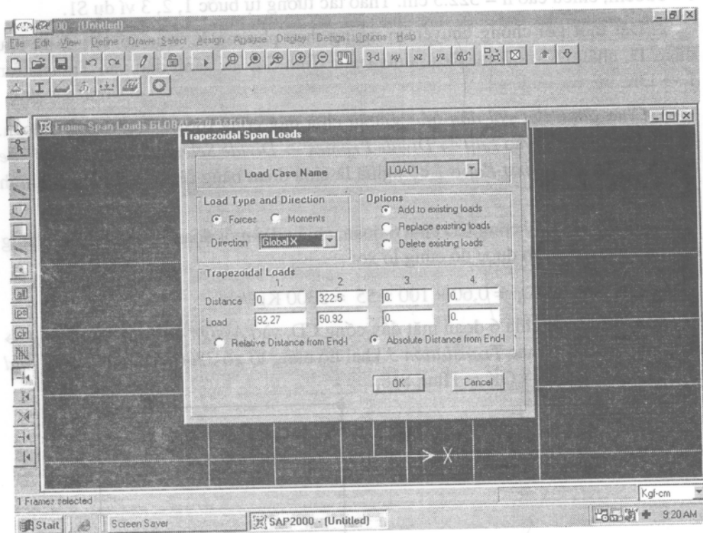
Hình S19: Nhập số liệu lực ngang hình thang
