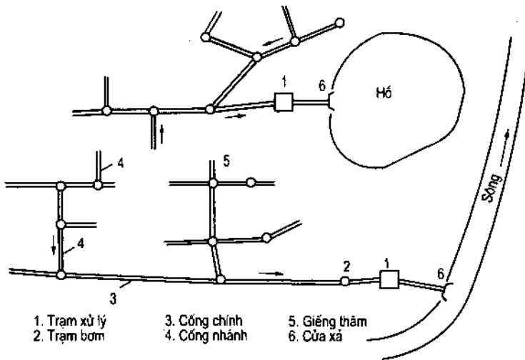
Hình 4-1: Hệ thống thoát nước chung
