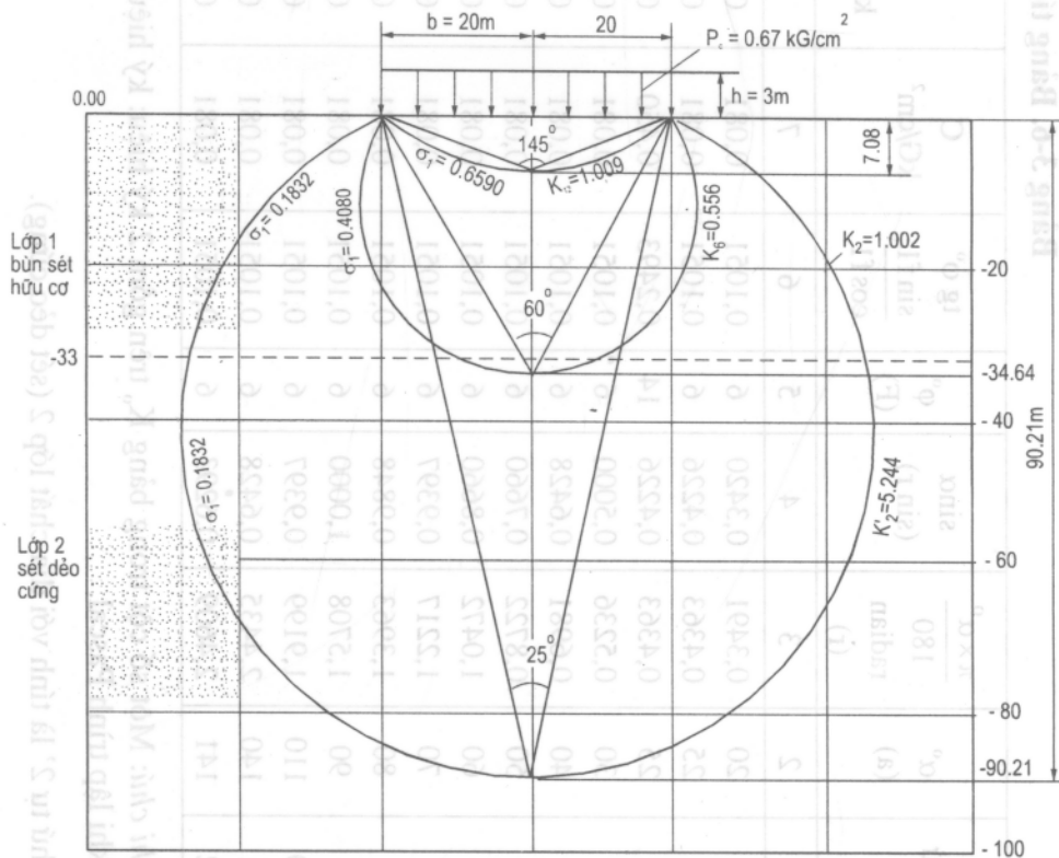
Hình 3-5: Đồ thị đường đẳng trị \sigma_1, \sigma_3, \tau_{\max}, K_0 theo ví dụ 3-1
