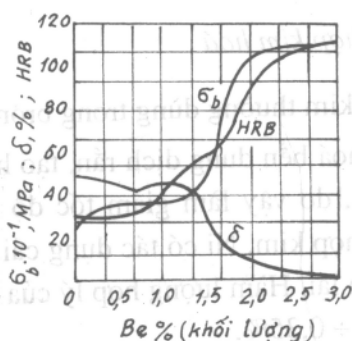
Hình 4.23. Cơ tính phụ thuộc vào hàm lượng Be. Mẫu: brông berili cán nguội, tôi từ 780^{\circ}\text{C} , hoá già ở 300^{\circ}\text{C} trong 3 giờ.
