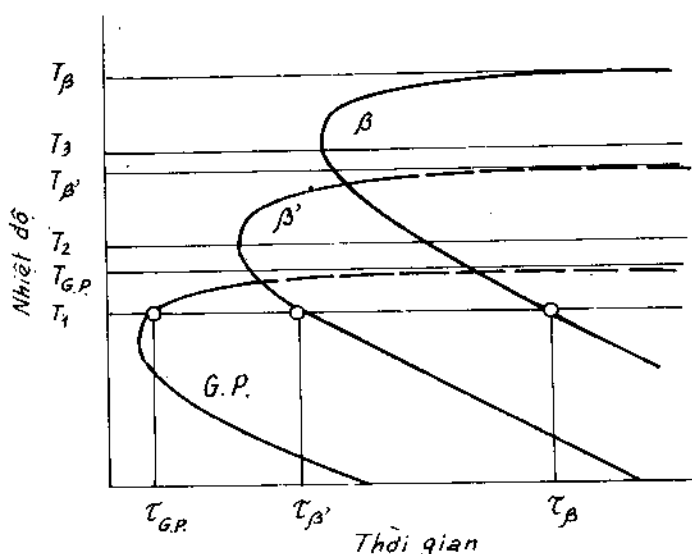
Hình 1.25. Đường cong chữ "C" hình thành VGP, pha \beta' và \beta khi phân hoá dung dịch rắn quá bão hoà. T_{GP} , T_{\beta'} , T_{\beta} là nhiệt độ hoà tan của các sản phẩm tiết ra VGP, \beta' và \beta .
