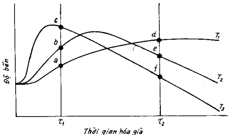
Hình 1.27. Ảnh hưởng của thời gian hóa già ở các nhiệt độ khác nhau ( T_1 < T_2 < T_3 ) tới độ bền của hợp kim.
