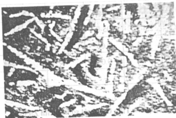
Ảnh 6.4. Tổ chức tế vi của hợp kim kẽm với 4%Al và 3%Cu. Các nhánh cây dài sáng là pha ε. Nền cơ bản là cùng tinh hai pha ( \epsilon + \eta ) và cùng tinh ba pha ( \eta + \beta + \epsilon ). x 150
