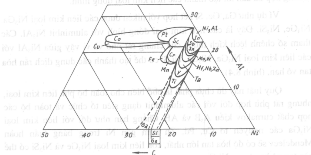
Hình 8.4. Vùng dung dịch rắn đồng nhất trên cơ sở \text{Ni}_3\text{Al} ở 1000^\circ\text{C}
