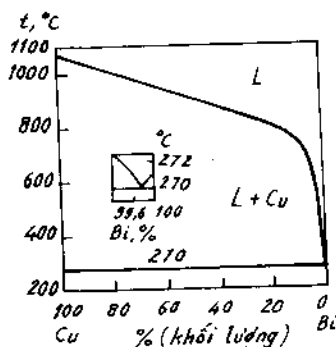
Hình 4.5. Giản đồ pha Cu - Bi.
