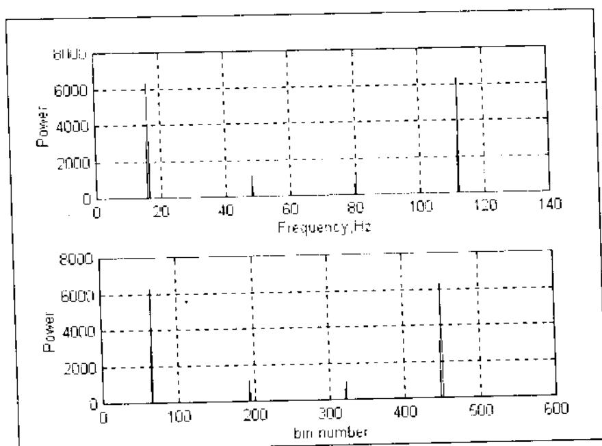
Hình 6.14 Phổ năng lượng của tín hiệu x=x_1+x_2
