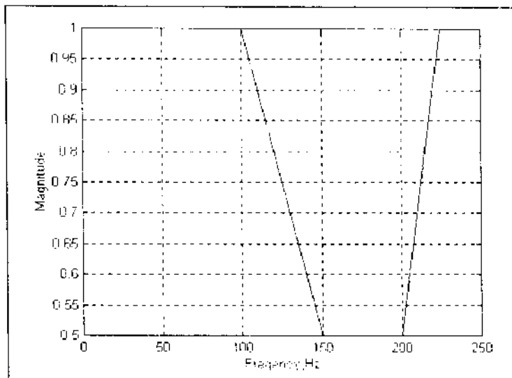
Hình 6.6 Đặc tính tần của bộ lọc
