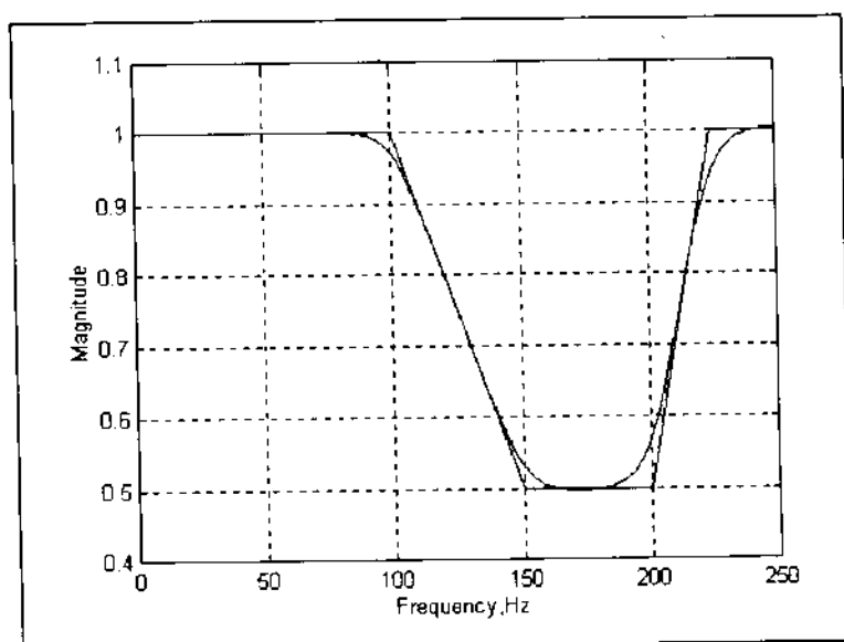
Hình 6.7 Bộ lọc IIR định nghĩa và bộ lọc thực
