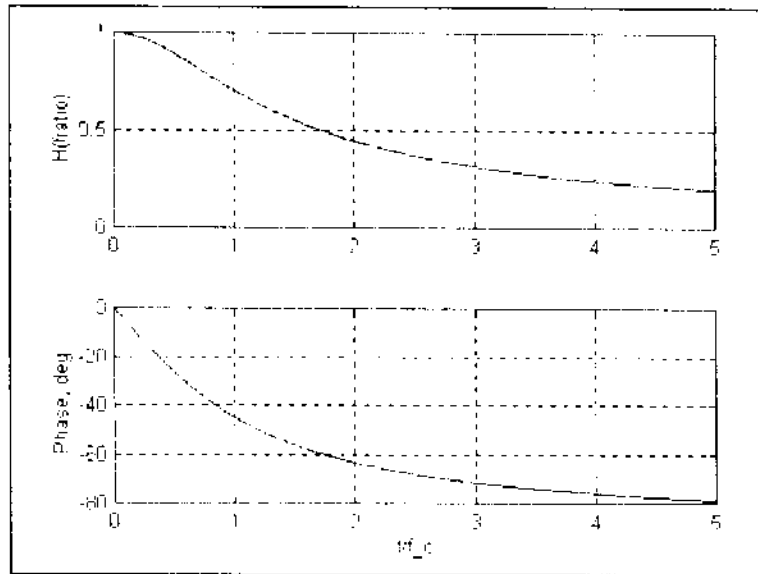
Hình 6.3 Đồ thị biên và tần của mạch thông thấp RC
