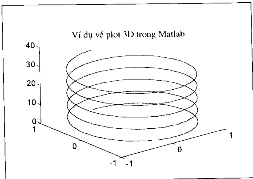
Hình 1.4 Đường Helix trong không gian 3D.
