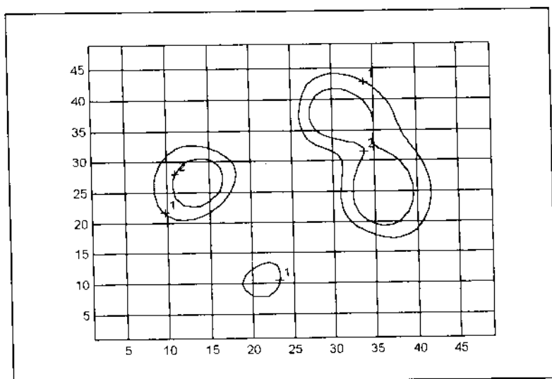
Hình 5.2 Đồ thị contour 2 mức độ cho bởi ví dụ b
