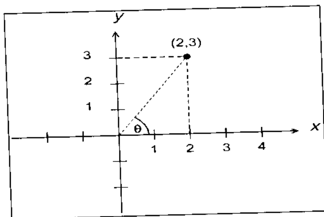
Hình 1.3 Biểu diễn số phức
