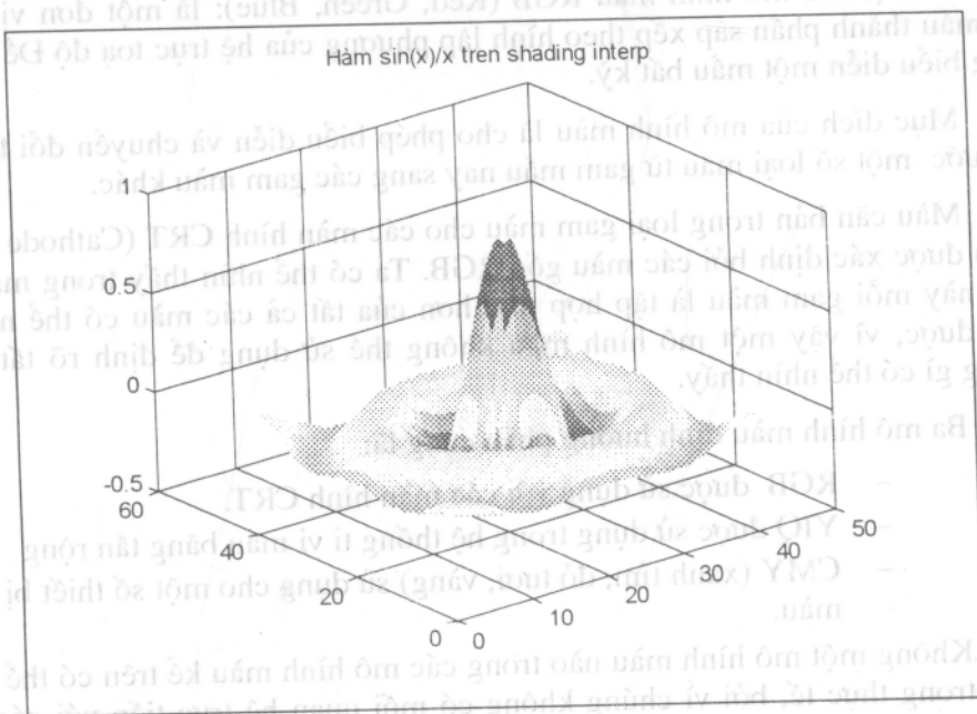
Hình 5.18 Phân bố màu trên bề mặt lưới với hiệu ứng bóng
