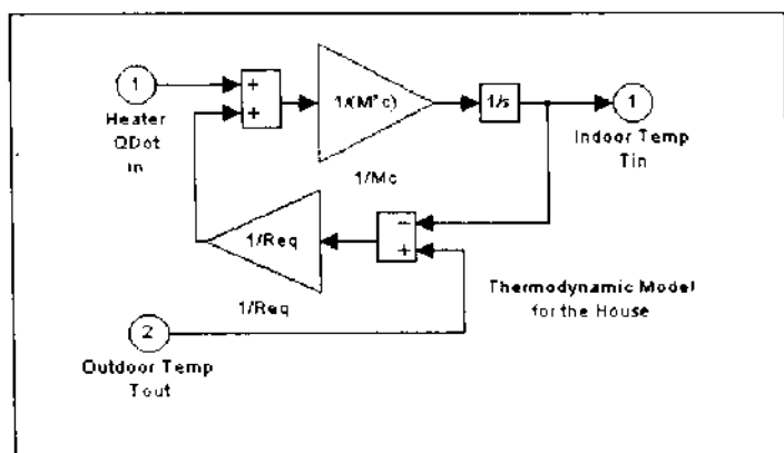
Hình 7.2 Mô hình nhiệt động của ngôi nhà
