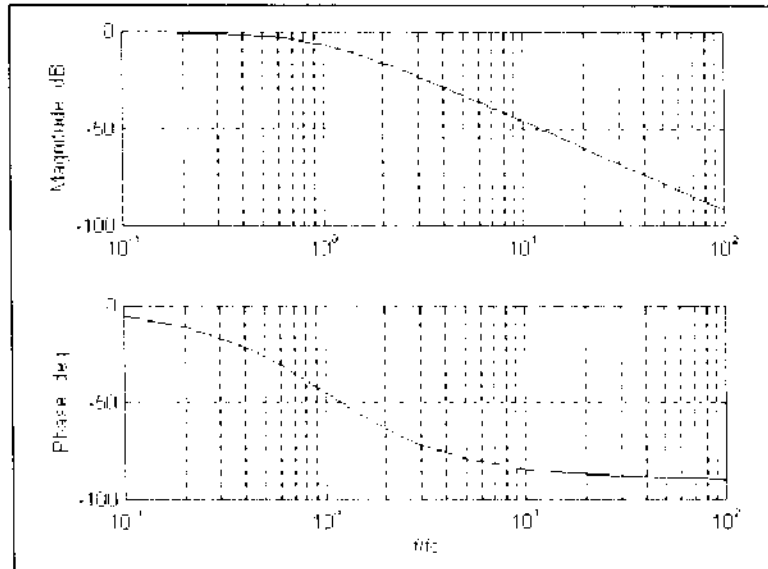
Hình 6.4 Mạch thông thấp dự tính trước
