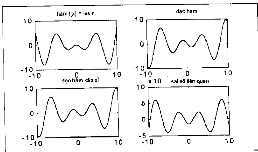
Hình 4.20 Hàm -x\sin(x) và các hàm liên quan
