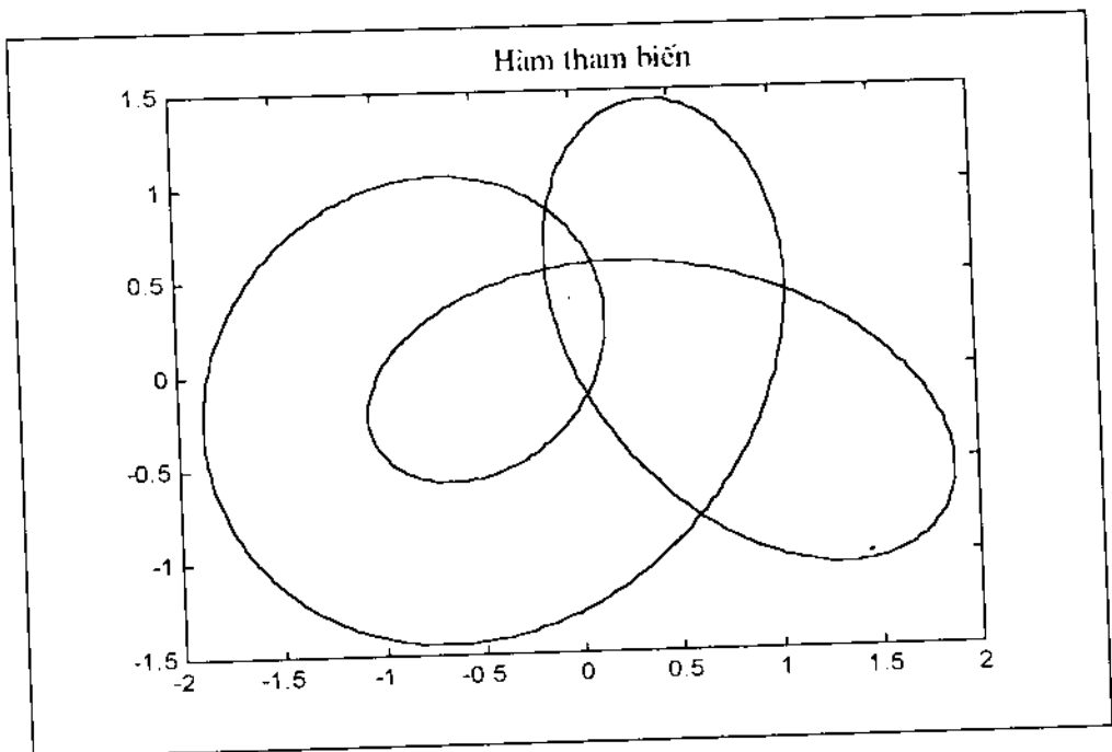
Hình 1.6 Hàm tham biến 2D
