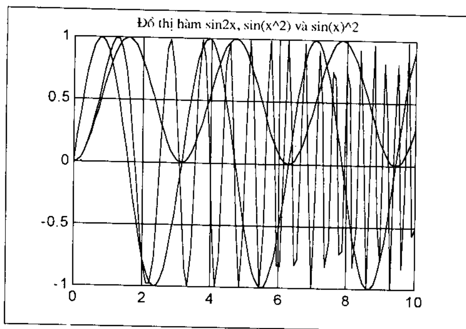
Hình 1.5 Hàm \sin 2x , \sin(x)^2 và \sin(x^2)
