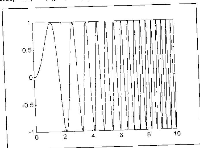
Hình 4.16 Phương trình \sin x^2 qua hàm fplot()
