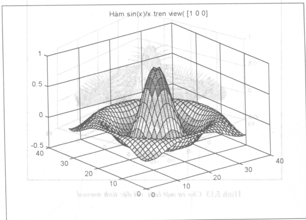
Hình 5.12 Mô tả mặt lưới \sin(r)/r . Với dải mẫu C phụ thuộc vào Z
