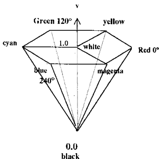
Hình 5.21 Mô hình màu HS
