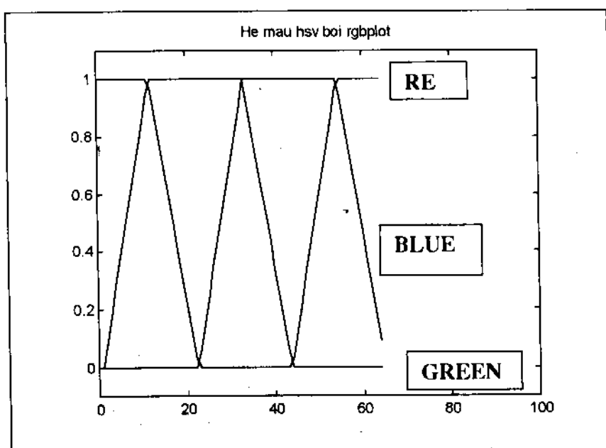
Hình 5.26 Hệ mẫu hsv trên cơ sở lệnh rgbplot.
