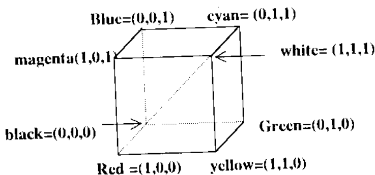
Hình 5.19 Mô hình không gian màu RGB
