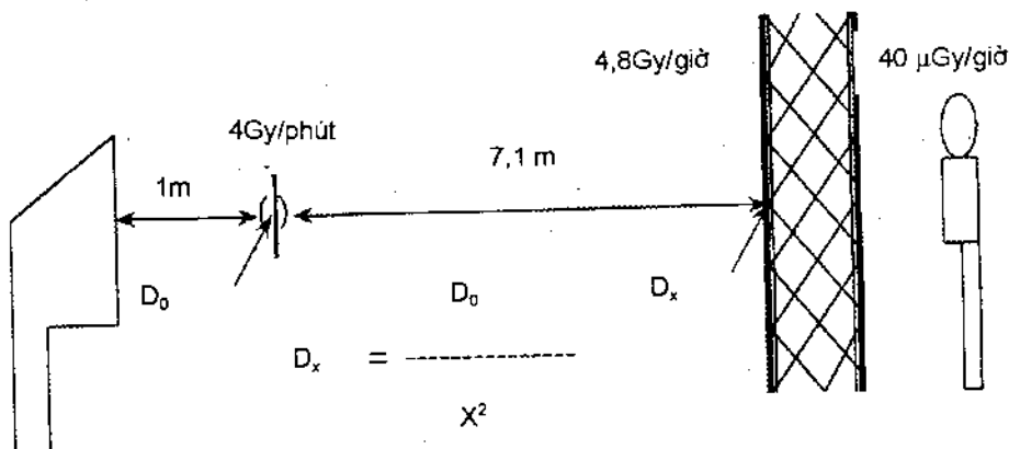
Hình 12.17. Mô phỏng ví dụ tính toán độ dày tường chắn sơ cấp và tường chắn thứ cấp
