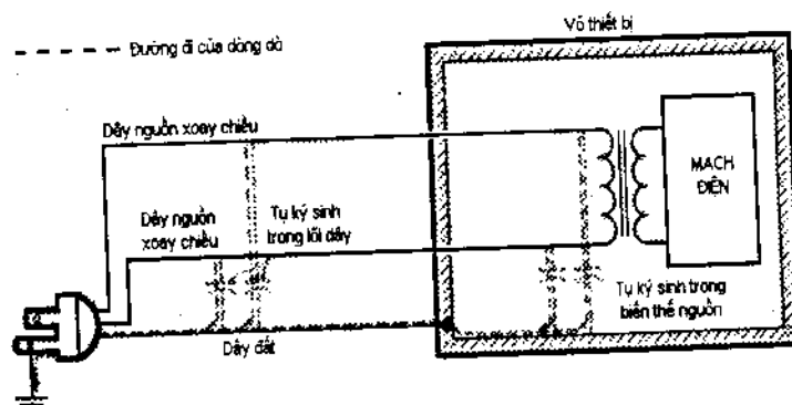
Hình 13.7. Nguồn gốc của dòng dò (tụ ký sinh).
