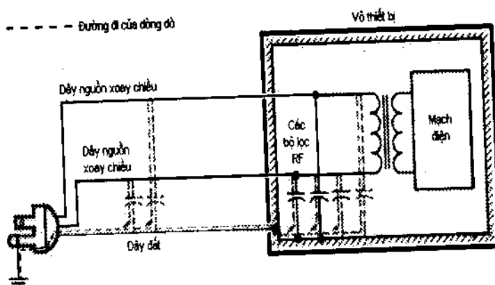
Hình 13.8. Các bộ lọc RF làm tăng dòng dò
