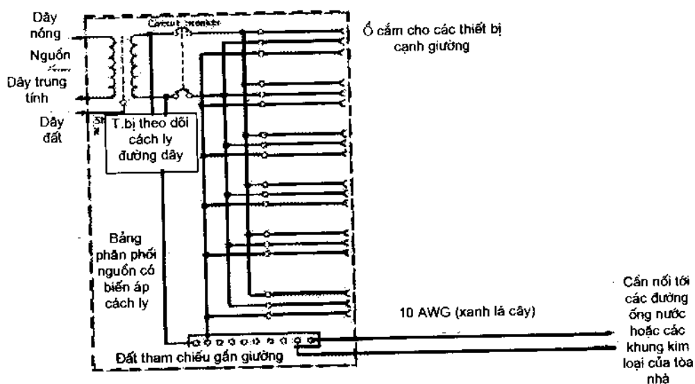
Hình 13.28. Hệ thống đường dây cách ly gần giường bệnh
