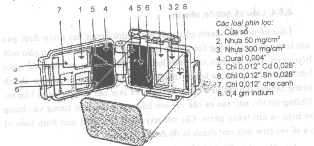
Hình 8.5. Hộp phim dùng để đo liều tích lũy
