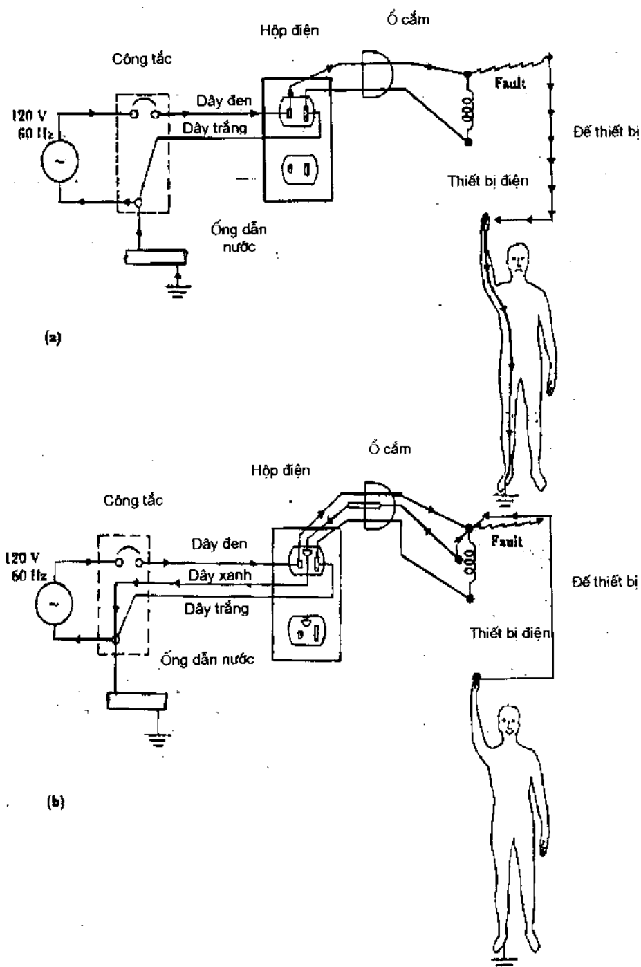
Hình 13.6. Nguy cơ giết vĩ mô do tiếp đất
