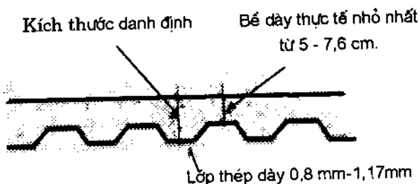
Cấu trúc sàn phòng điển hình bằng bê tông
