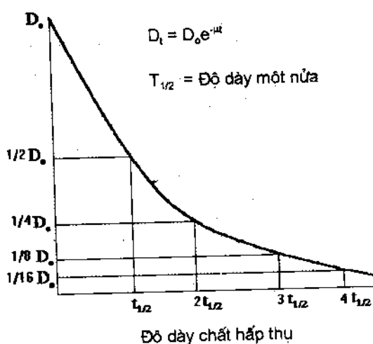
Hình 8.1. Sự thay đổi của suất liều gamma theo độ dày của chất hấp thụ.
