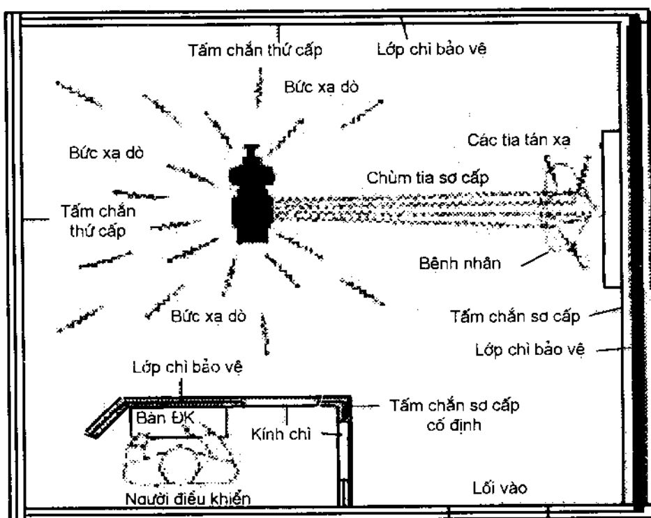
Hình 12. 6. Sự phân bố chùm tia bức xạ sơ cấp và bức xạ thứ cấp (bức xạ dò và tán xạ) trong một phòng chụp X quang
