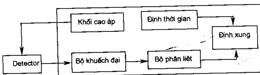
Hình 7.10. Sơ đồ khối của một máy đếm
