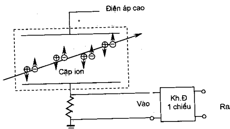
Hình 7.2 Sơ đồ buồng ion hóa
