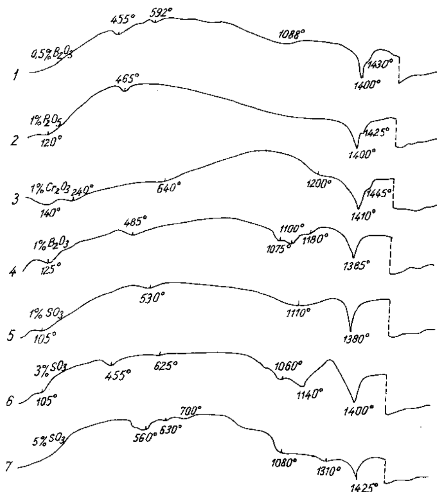
Hình 18. Các đường cong gián đồ DTA nhiệt độ cao - 1500°C.
