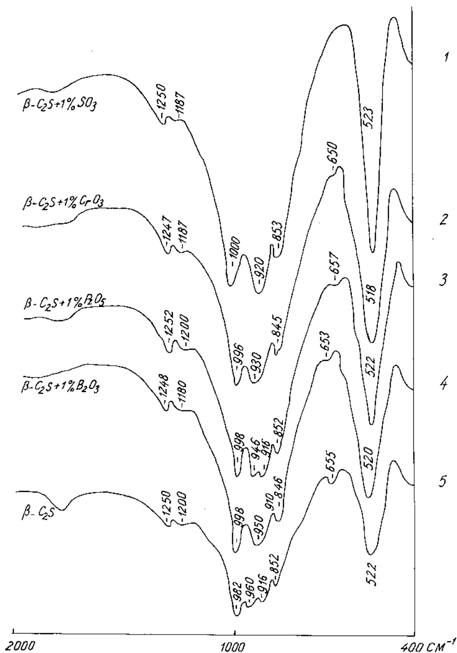
Hình 20a. Giảm đồ quang phổ hồng ngoại \beta\text{-C}_2\text{S} với các phụ gia.
