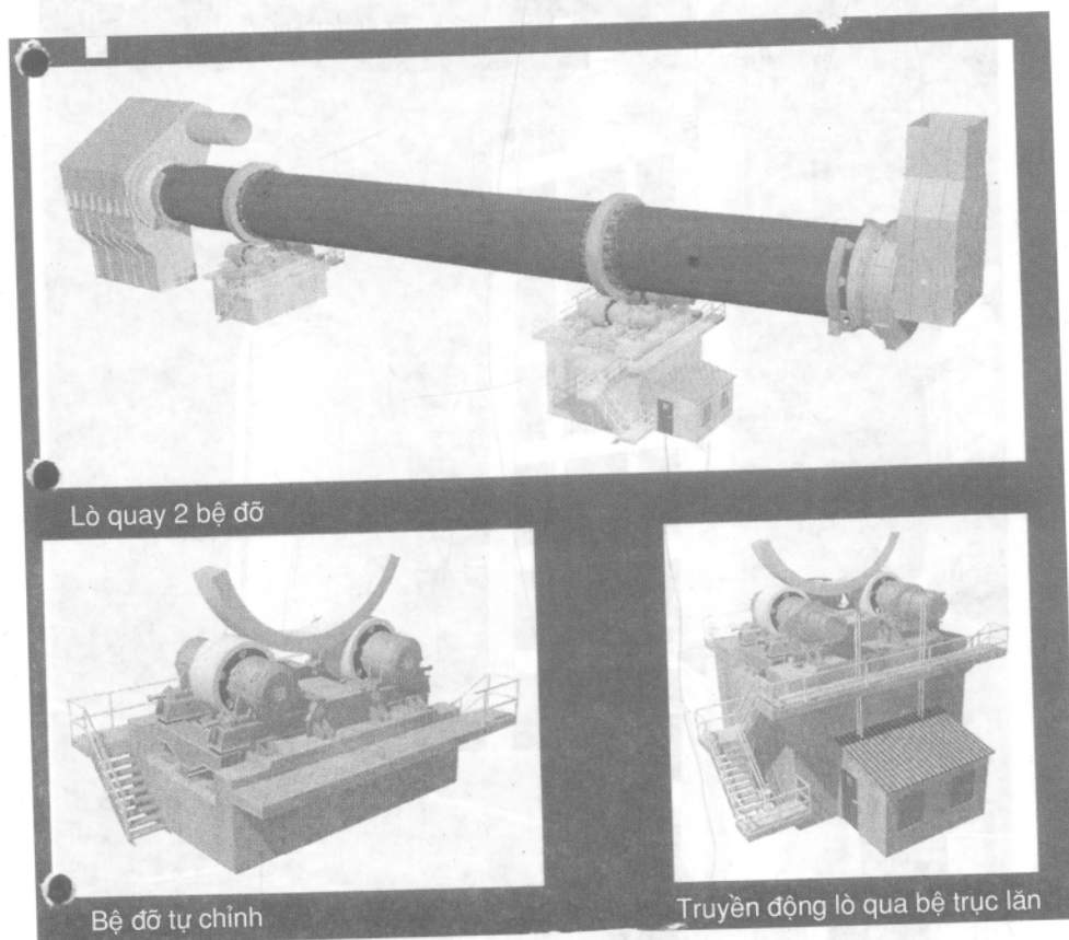
Hình 8. Lò quay khô 2 bộ và các bộ đỡ của Hãng F.L. Smidth Đan Mạch.
