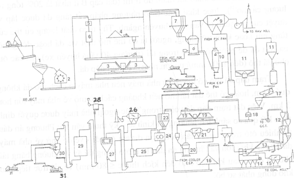
Hình 1. Sơ đồ tổng quát công nghệ dây chuyền sản xuất xi măng:
