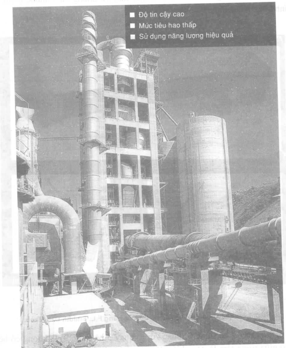
Hình 9. Lò quay khô 3 bệ.
