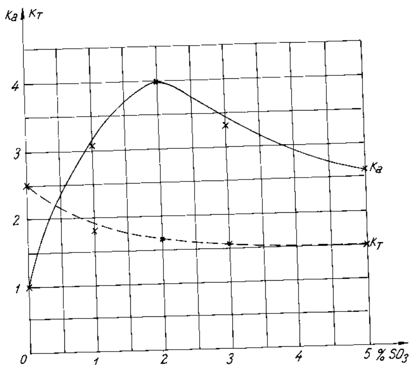
Hình 17. Đường cong biến thiên của K a và K T .
