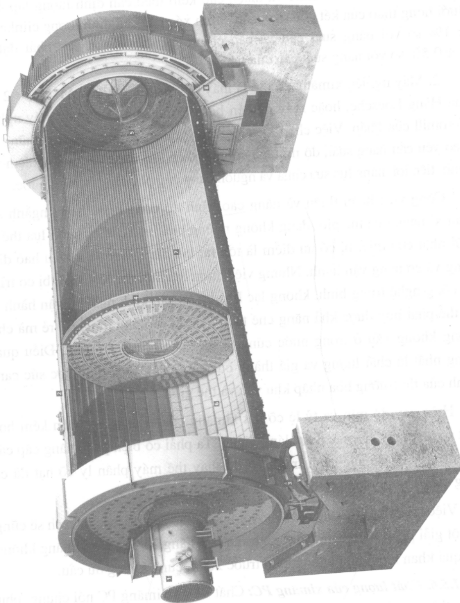
Hình 12. Máy nghiền xi măng.
