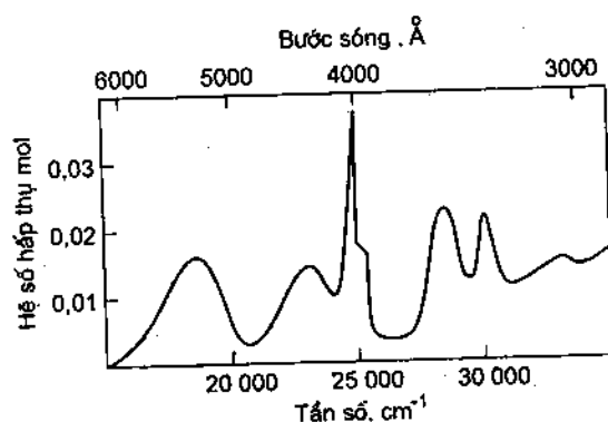
Hình 35. Phổ hấp thụ electron của ion [\text{Mn(H}_2\text{O)}_6]^{2+} ở trong vùng trông thấy
