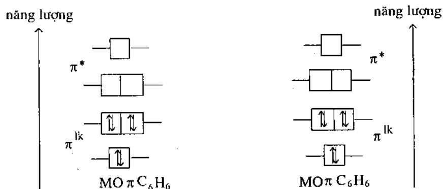
Hình 27. Biểu đồ năng lượng các MO \pi trong hai phân tử C_6H_6 riêng rẽ.
