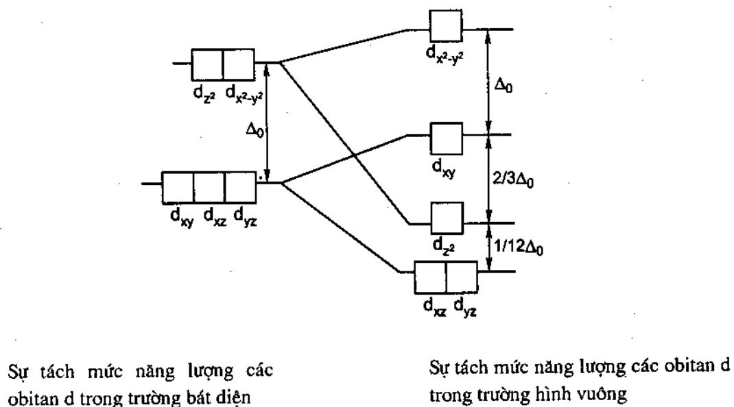
Hình 5. Sự tách mức năng lượng của obitan d trong phức chất
