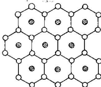
Hình 35 - Kiến trúc lớp của AlB_2
