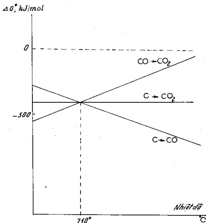
Hình 54 - Biến thiên năng lượng Gíp tạo thành các oxit của cacbon theo nhiệt độ (tính theo 1 mol \text{O}_2 ).
