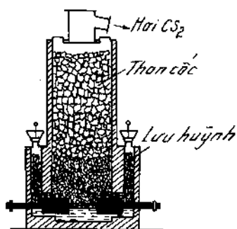
Hình 56 - Sơ đồ lò điện điều chế \text{CS}_2
