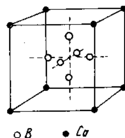
Hình 36 - Kiến trúc tinh thể của CaB_6
