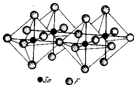
Hình 65 - Kiến trúc tinh thể của SnF_4
