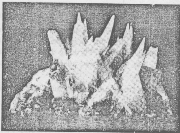
Hình 27 - Tinh thể aragonit.
