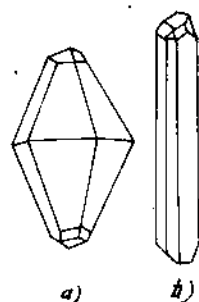
Hình 81 - Tinh thể lưu huỳnh a) Tà phương b) Đơn tà
