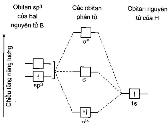
Hình 32 – Giản đồ năng lượng các obitan phân tử của liên kết ba tâm trong điboran
