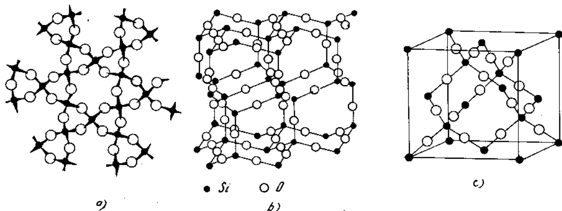
Hình 57 - Kiến trúc tinh thể của thạch anh \beta (a), tridimit \beta (b) và cristobalit (c)
