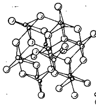
Hình 43 - Kiến trúc tinh thể của Al_2O_3 - \alpha
