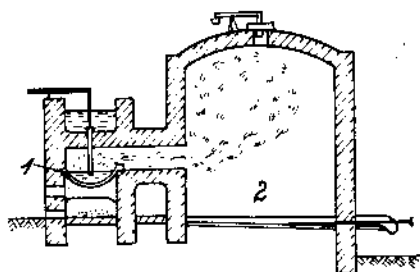
Hình 86 - Lò chưng cất lưu huỳnh 1. Lò 2. Buồng ngưng tụ
