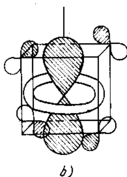
Hình 88 - Các obitan 2p của O và các obitan 3d_{x^2-y^2} (hình a), 3d_{z^2} (hình b) của S ở trong ion \text{SO}_4^{2-} .
