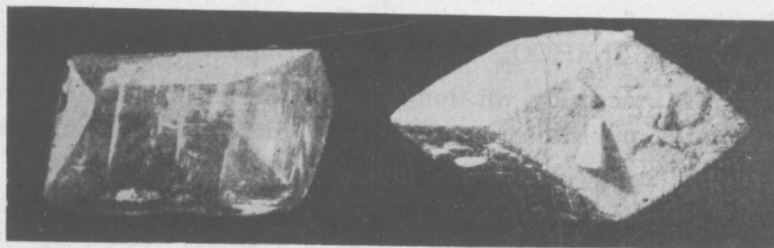
Hình 26 - Tinh thể canxit.
