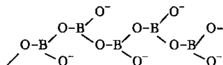
Ion (\text{BO}_2)_n^{a-}
