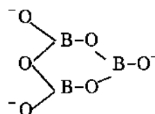
Ion (\text{BO}_2)_3^{3-}
