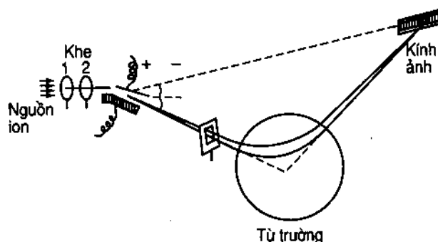
Hình 2 - Sơ đồ của máy quang phổ khối
