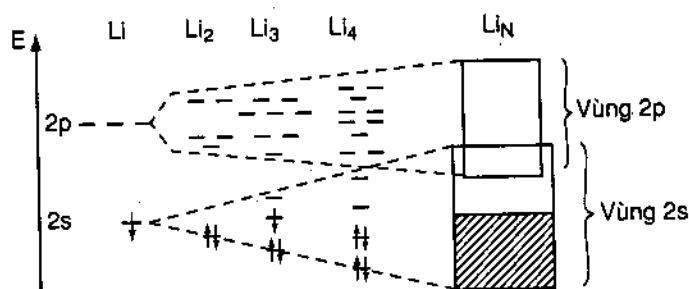
Hình 70-Sự tạo thành các vùng năng lượng 2s và 2p
