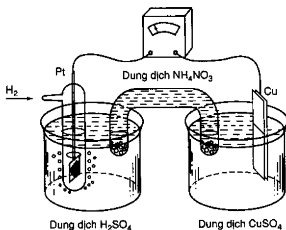
Hình 100 - Pin với điện cực hidro
