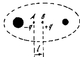
Hình 37-Lưỡng cực điện
