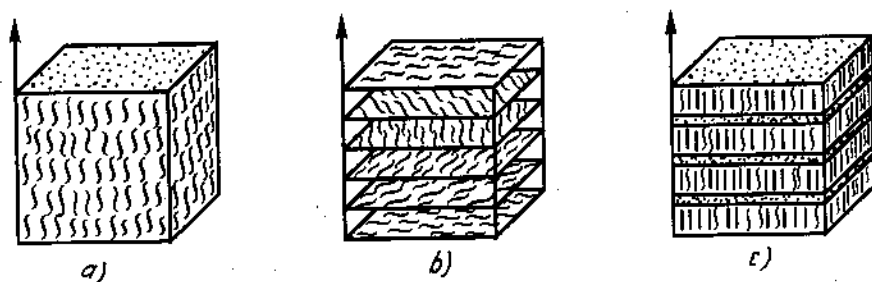
Hình 75- Cấu tạo của tinh thể lỏng a) loại nematic. b) loại colesteric. c) loại smetic
