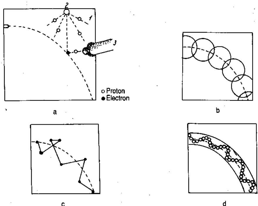
Hình 7 - Thí nghiệm tưởng tượng về nguyên lý bất định
