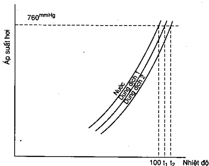
Hình 89- Sự tăng nhiệt độ sôi của dung dịch nước
