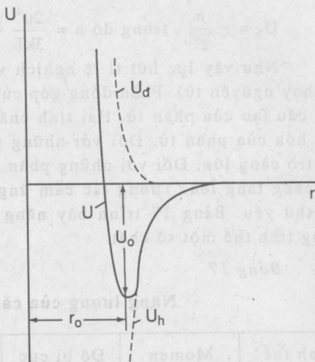
Hình 40- Đường cong thế năng của tương tác giữa các phân tử
