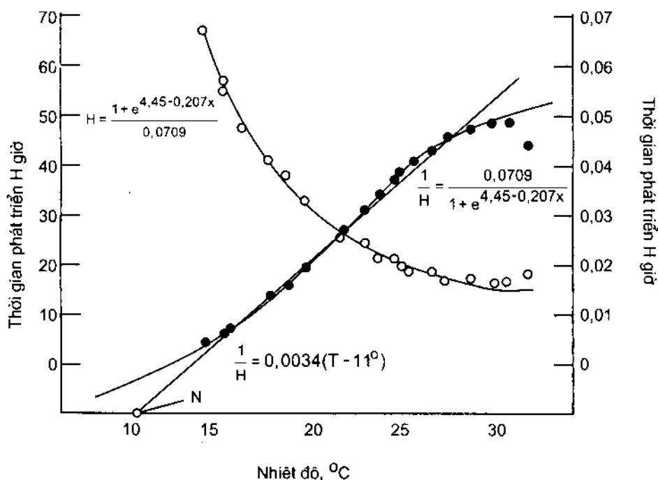
HÌNH 4.3. Ảnh hưởng của nhiệt độ đến sự phát triển của trứng ruồi quả Drosophyla melanogaster (theo Davidson. 1944), N- nhiệt độ ngưỡng phát triển
