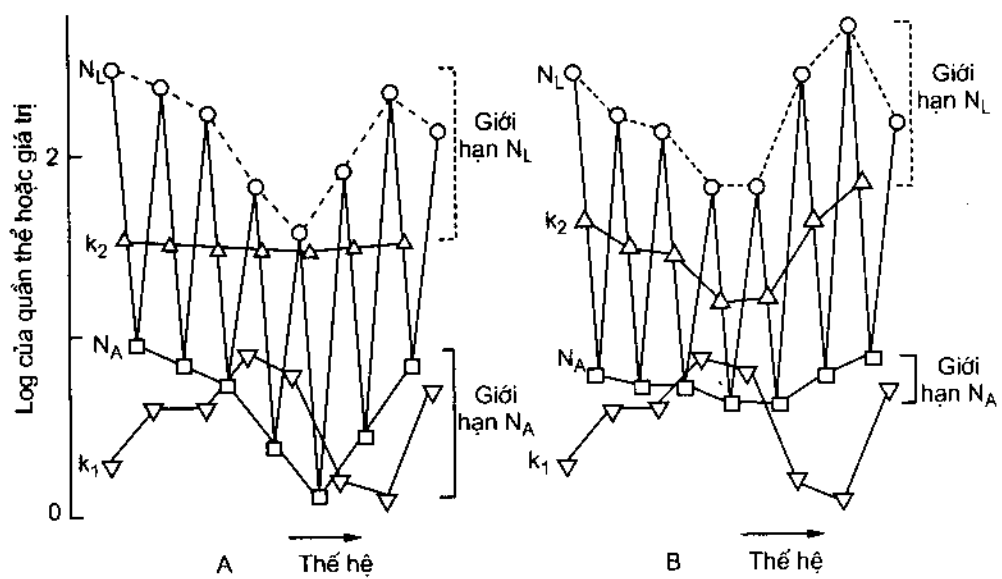
HÌNH 4.6. Trong mô hình A và B, quần thể của các cá thể trưởng thành được quyết định bởi tốc độ sinh sản bậc 10
