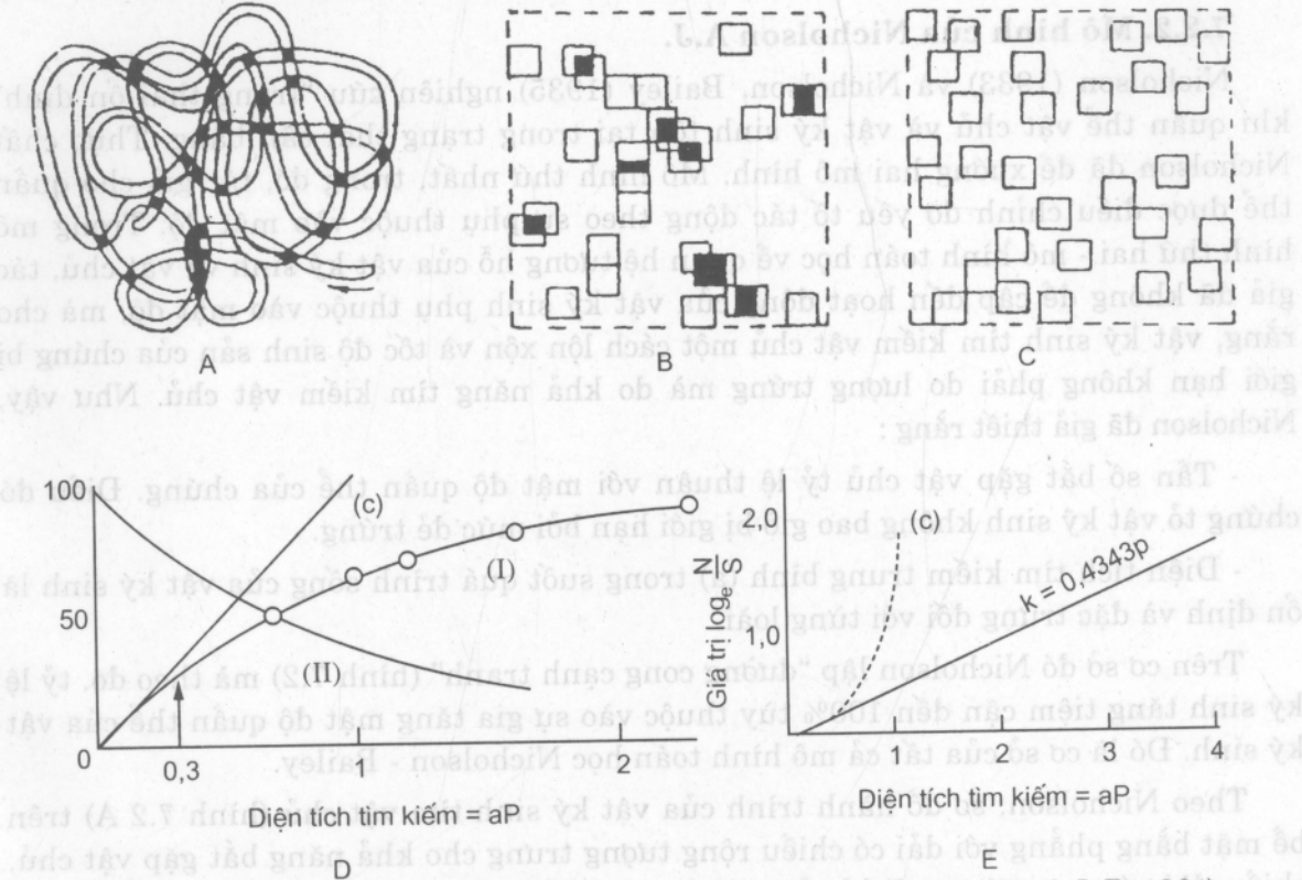
HÌNH 7.2. Sơ đồ hành trình của vật ký sinh tìm kiếm vật chủ (theo Clark L.R. 1964) :
