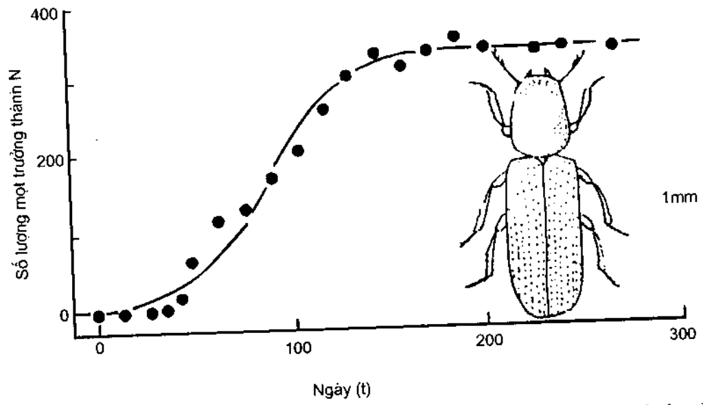
HÌNH 7.6. Số lượng một Rhyzopertha dominica nuôi bắt đầu với một đôi trong 10g hạt lúa mì (theo Crombie, 1954), và cứ sau mỗi tuần lại sàng để loại bỏ bột, rồi bổ sung cho đủ 10g.
