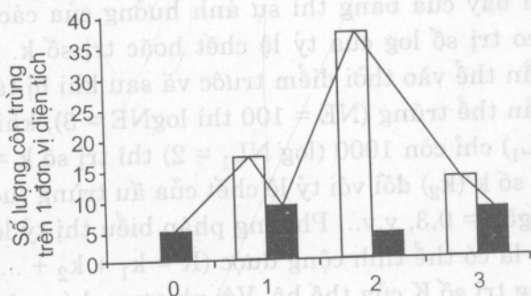
HÌNH 9.2. Tổ chức đồ và đường cong thế hệ của quần thể côn trùng giả thiết với mỗi năm phát triển được ba thế hệ
