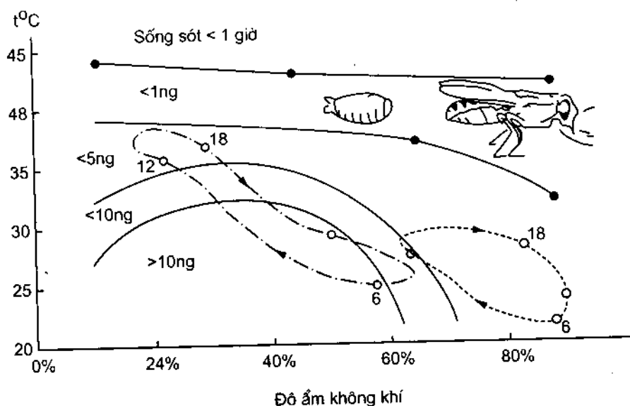
HÌNH 4.4. Ảnh hưởng của độ ẩm tương đối và nhiệt độ đến thời gian sống của ruồi Xexe ( Grossia tachynoides ) trưởng thành ở trong điều kiện thí nghiệm và điều kiện bình thường, phổ biến ở Tây Phi vào tháng IV và tháng VII (theo Buxton, Lewis, 1934)
