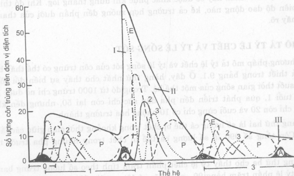
HÌNH 9.1. Biến động số lượng của quần thể côn trùng giả thiết với mỗi năm phát triển được ba thế hệ
