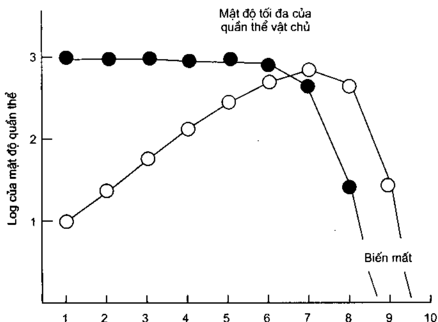
HÌNH 7.1. Mô hình quần thể theo Thompson đối với quần thể ổn định của vật chủ bị vật ký sinh tấn công
