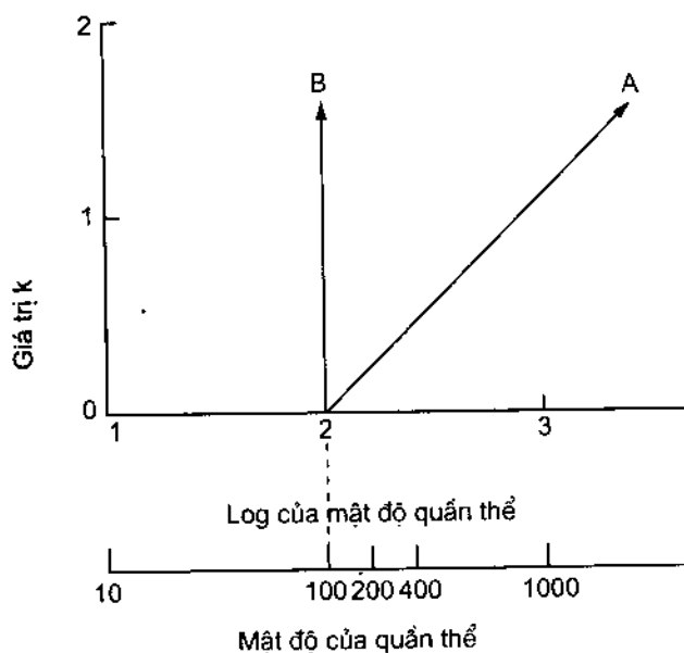
HÌNH 7.8. Tỷ lệ chết trong hai loại cạnh tranh A- Cạnh tranh đối kháng ; B- Cạnh tranh tàn bạo (Varley, 1974)
