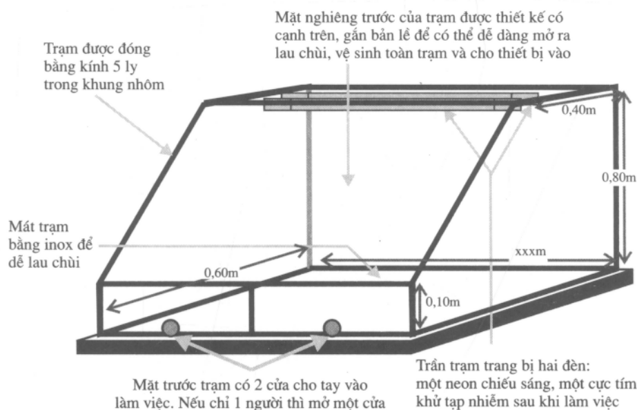
Hình 21.1: Mô hình một tủ cấy vi sinh khí tĩnh. Kích thước chiều cao 0,8m, chiều sâu 0,6m. Riêng kích thước chiều dài thì tùy thuộc vào bàn để tủ cấy, trung bình là 1,2m.
