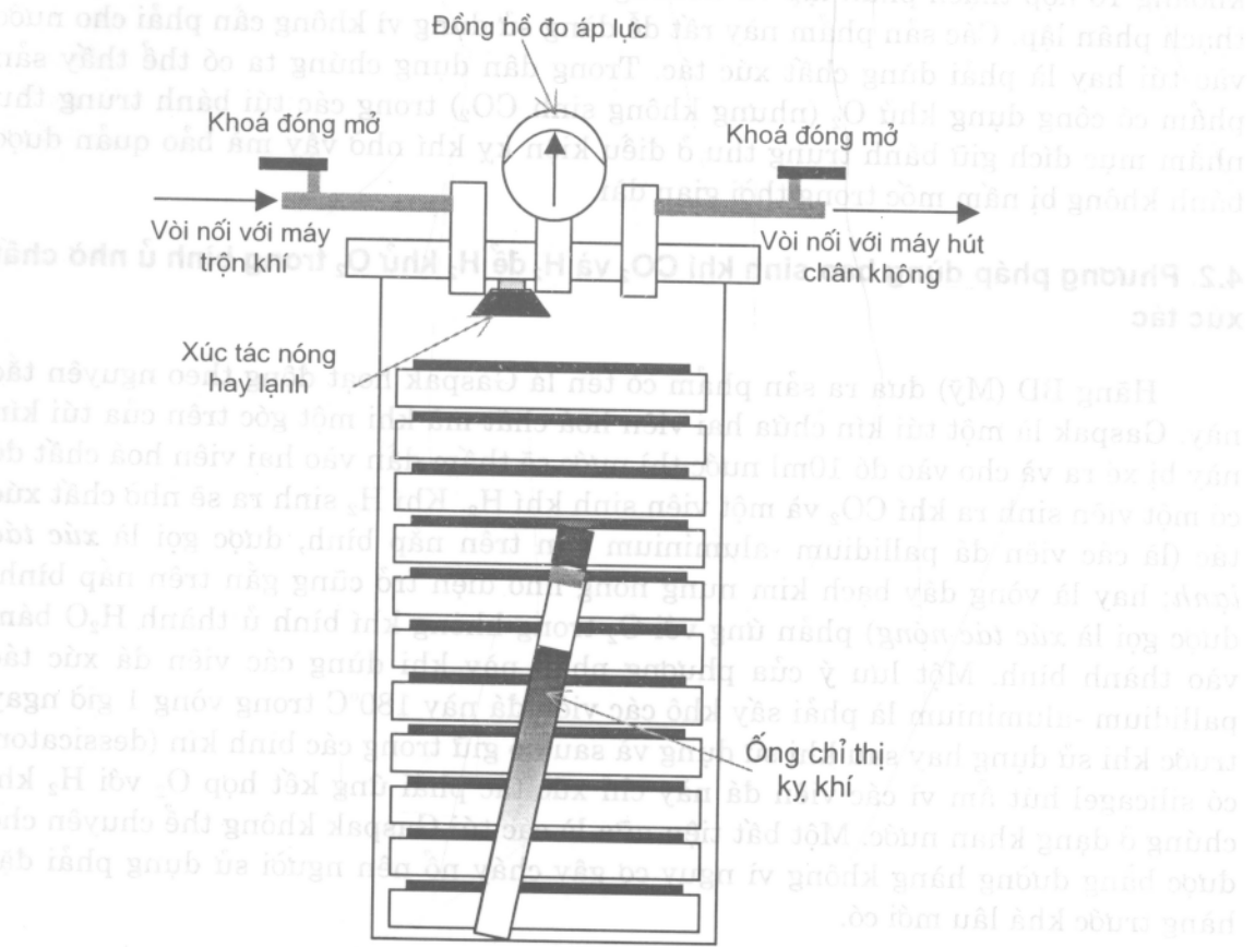
Hình 11.1: Cấu trúc một bình ủ kỵ khí dùng phương pháp thay khí
