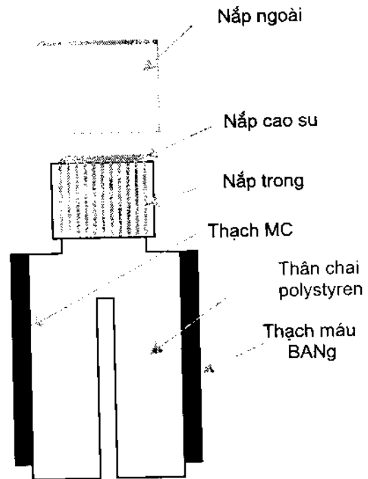
Hình 4.1: Cấu tạo chai cấy nước tiểu 2 mặt thạch BANG và MC
