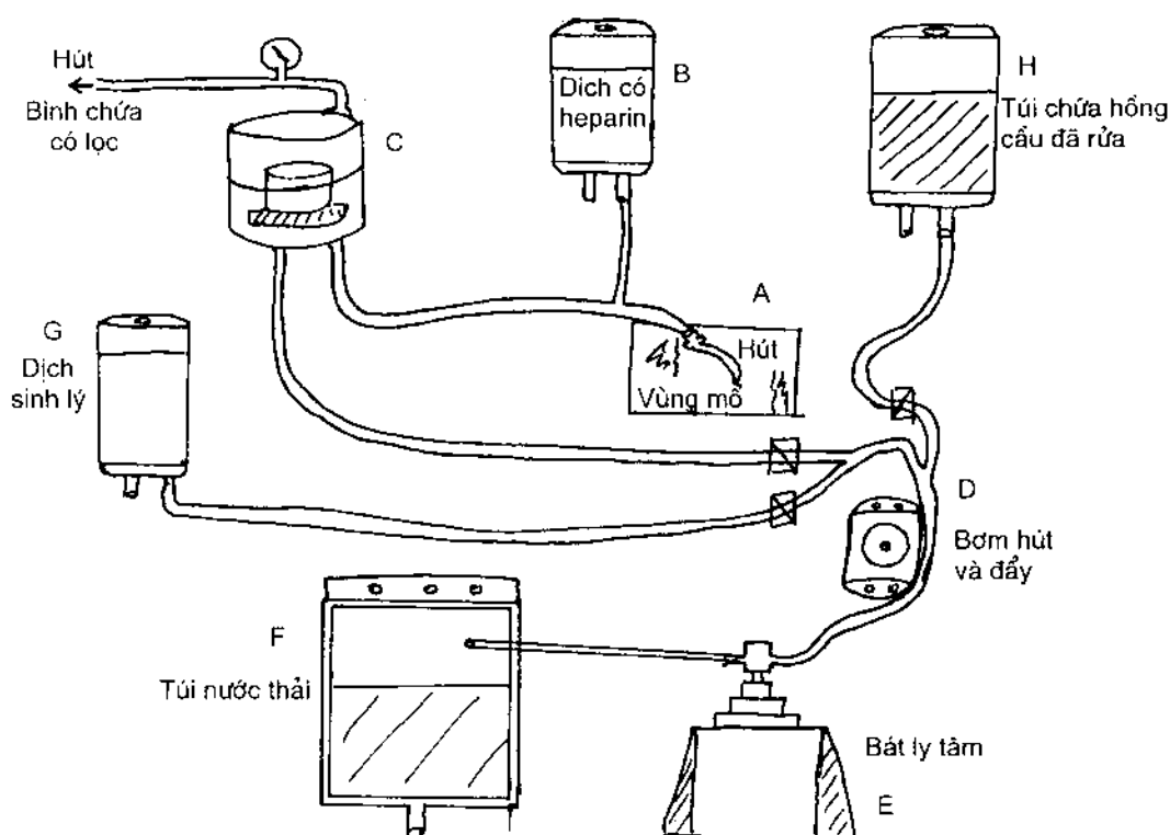
Hình 18.1. Sơ đồ máy "Cell Saver"
