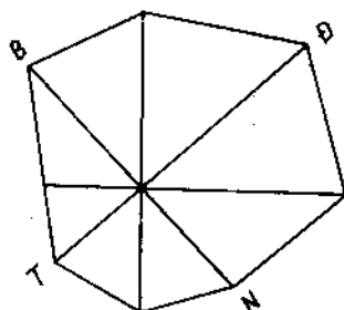
Hình 6-17 Hoa hồng gió.
