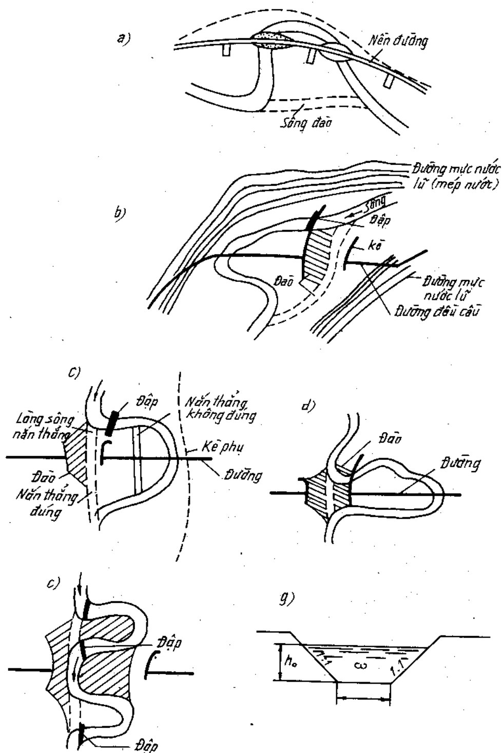
Hình 6-2. Một số ví dụ các trường hợp uốn khúc lòng sông. a, b - uốn khúc lòng sông để tránh phá hoại nền đường; c - ví dụ cách uốn khúc lòng sông cong đúng và không đúng kỹ thuật; d, e - một số ví dụ cách uốn khúc lòng sông ở đoạn sông cong; g - trắc ngang thoát nước đoạn sông đào nhân tạo.
