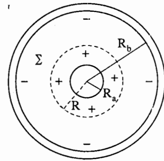
Hình 19-6. Mặt cắt của một tụ điện cầu.
