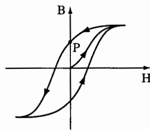
Hình 25-9: Vật liệu sắt từ bậc lộ tính từ trễ. Mỗi liên hệ giữa B và H phụ thuộc vào sự xử lí trước đó của mẫu.
