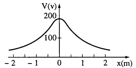
Hình 18-6. Ví dụ 18-4 : V(x) ở dọc theo trục của vòng tích điện trên hình 18-5; Q = 11,1\text{nC} , a = 0,50\text{m} .
