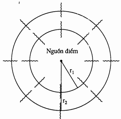
Hình 28-16. Nguồn điểm tạo ra một sóng cầu ổn định. Do bảo toàn năng lượng, mà năng lượng trong một giây, hay công suất, đi qua mặt cầu trong bằng năng lượng đi qua mặt cầu ngoài trong một giây.
