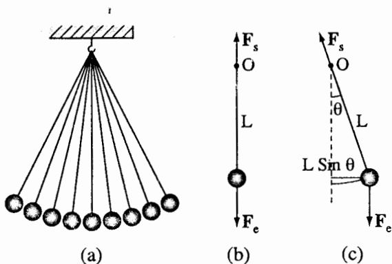
Hình 26-7. (a) Bức ảnh hoạt nghiệm cho thấy con lắc đơn đưa từ phía này sang phía kia như thế nào. (b) Tổng momen lực đối với trục O bằng không khi con lắc ở vị trí cân bằng. (c) Momen của trọng lượng đối với trục O có xu hướng kéo con lắc về vị trí cân bằng. Momen của lực do giá treo tác dụng đối với trục O bằng không.
