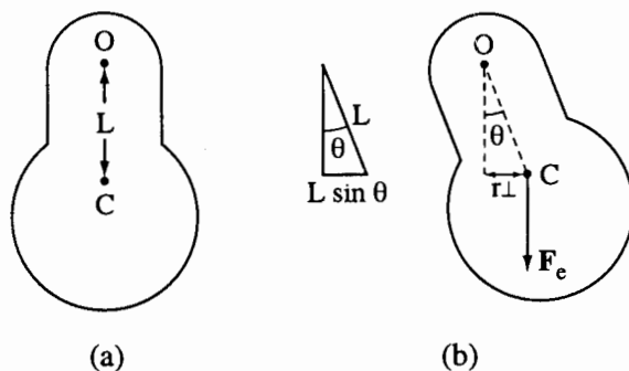
Hình 26-8. (a) Một vật rắn ở trạng thái cân bằng quay với khối tâm C nằm thẳng dưới trục quay O . (b) Thành phần của momen trọng lượng M_z = -r_{\perp} F_e = -(L \sin \theta)(mg) . Trục z đi qua O và có hướng đi ra phía ngoài mặt phẳng hình vẽ.
