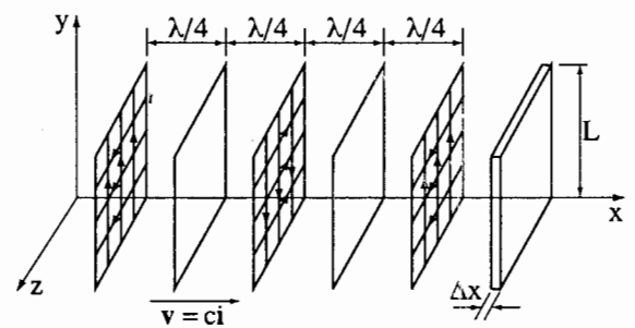
Hình 30-7. Sóng điện từ phẳng đi qua một yếu tố thể tích có dạng một tấm phẳng với diện tích A = L^2 và độ dày \Delta x . Vì tốc độ sóng là c , thời gian cần thiết để năng lượng \Delta W = w(A\Delta x) chứa trong bản phẳng đi qua mặt bên phải của tấm đó là
