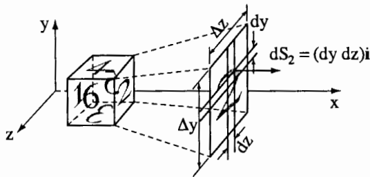
Hình 30-2. Định luật Gauss áp dụng cho một hình lập phương. Các mặt của hình lập phương được đánh số từ 1 đến 6. Phép chiếu phóng đại mặt 2 cho thấy rằng d\mathbf{S}_2 = (dydz)\mathbf{i} .
