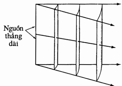
Hình 27-22. Câu hỏi 12. Phần các mặt được dùng để biểu diễn các mặt sóng trụ phát ra từ một nguồn thẳng. Các sóng này được gọi là các sóng trụ.
