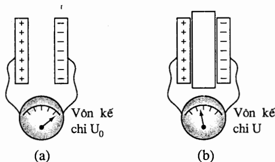
Hình 19-11. (a) Với chân không ở giữa các bản của một tụ điện tích điện, vôn kế chỉ U_0 . (b) Với một chất điện môi ở giữa các bản của một tụ điện tích điện, vôn kế chỉ U , và bao giờ ta cũng có U_0 > U .
