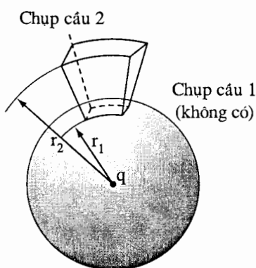
Hình 17-8. Thông lượng của điện trường do một điện tích điểm đặt ở tâm mặt Gauss gây ra, nó gần như là một mặt cầu ngoại trừ một mặt cầu lõm ra. Thông lượng đi qua chóp cầu 2 bằng thông lượng bị mất do không có chóp cầu 1, cho nên thông lượng đi qua cả mặt cũng chính là thông lượng đi qua mặt cầu
