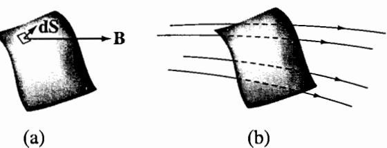
Hình 22-18. (a) Từ thông đối với một diện tích vô cùng bé dS được cho bởi d\phi_B = \mathbf{B} \cdot d\mathbf{S} . (b) Từ thông đối với một mặt tỉ lệ với số đường cảm ứng từ cắt xuyên qua mặt đó.
