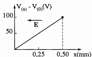
Hình 18-10. Ví dụ 18-6 : Trong khoảng không gian giữa các bản của một tụ điện, thì V(x) - V_0 biến đổi tuyến tính từ một bản này sang một bản kia và tăng theo chiều ngược với \mathbf{E} .
