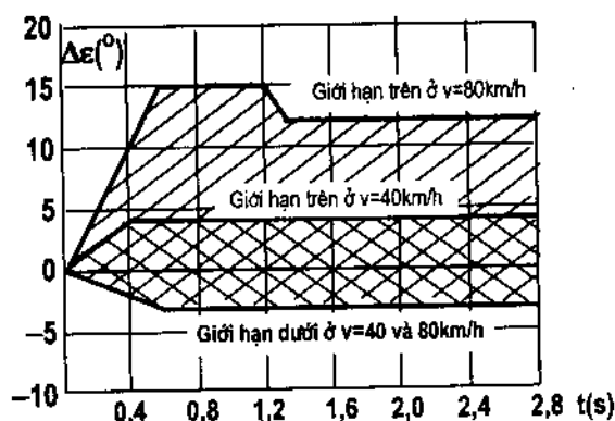
Hình 2-78: Vùng giới hạn của sự biến đổi góc quay thân xe ( \Delta\epsilon ) khi thả tay lái trên đường vòng theo thời gian
