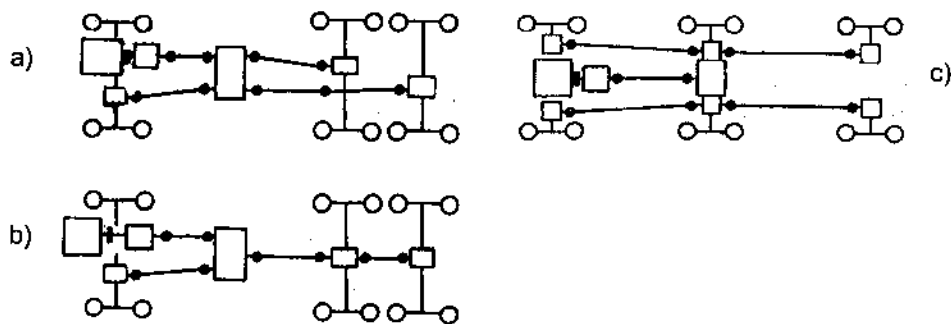
Hình 4-34: Các sơ đồ HTTL ô tô 3 cầu chủ động
