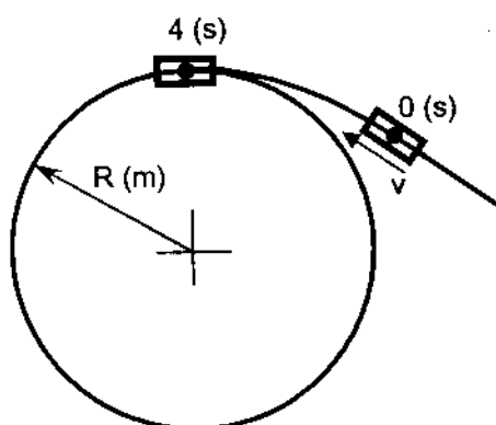
Hình 2-75: Quy đạo xác định tiêu chuẩn về lực điều khiển vành lái
