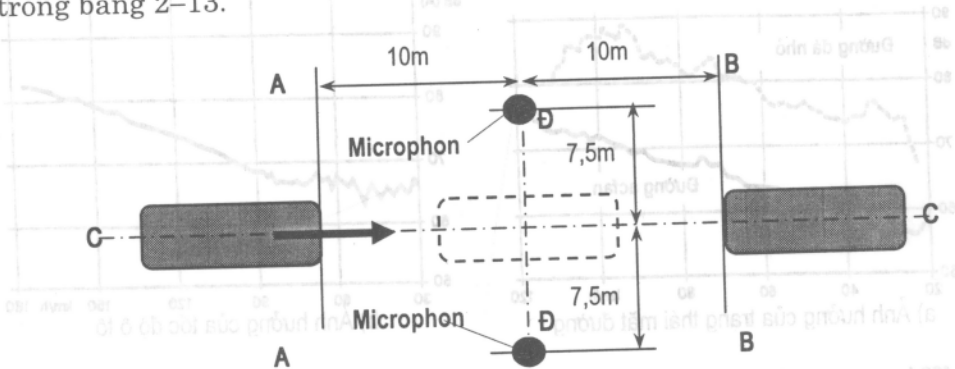
Hình 2.49. Đo độ ồn ngoài
