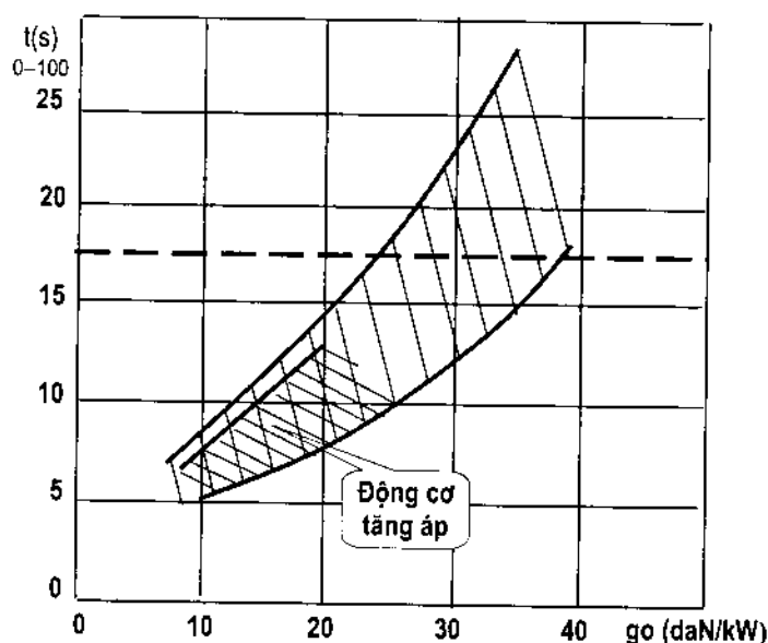
Hình 2-1: Quan hệ của thời gian tăng tốc với trọng lượng đơn vị g_0
