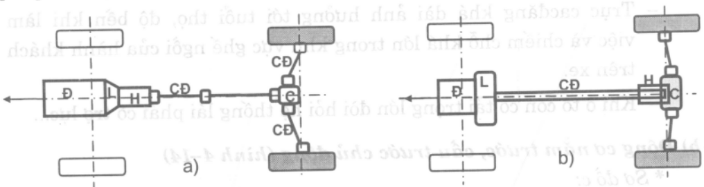
Hình 4-13: Các sơ đồ bố trí chung HTTL truyền thống ô tô con.
