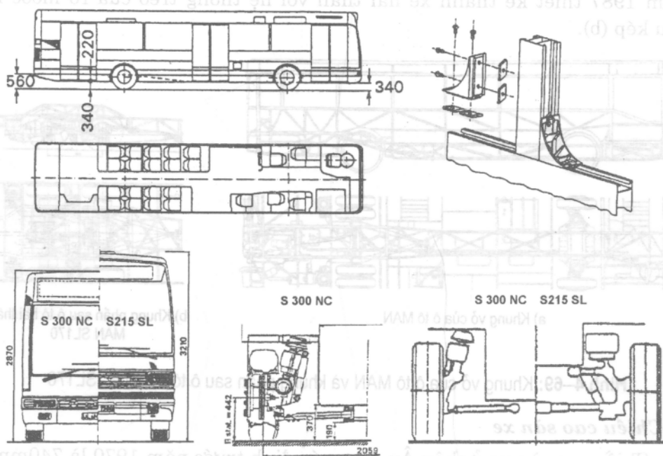
Hình 4-70: Cấu trúc Setra S 300 NC và các thông số so sánh với S 215 SL
