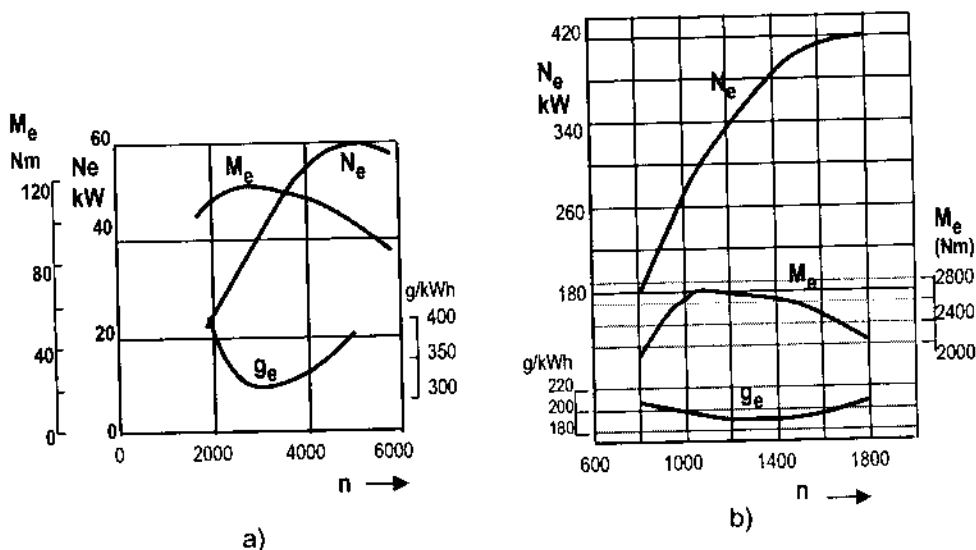
Hình 2-19: Các đường đặc tính tốc độ của động cơ xăng (a) và diesel (b)
