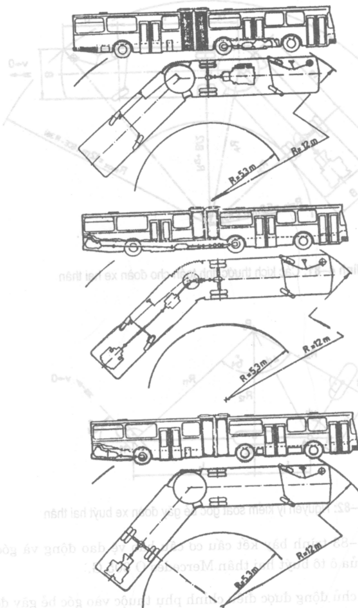
Hình 4-80: Tiêu chuẩn ECE về cơ động khi quay vòng của kết cấu ô tô hai thân
