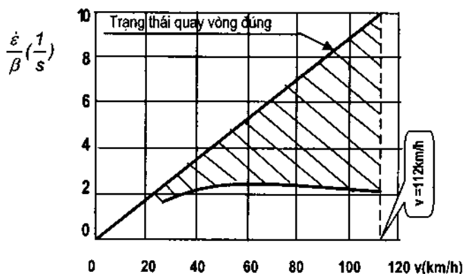
Hình 2-76: Quan hệ của hàm chuyển vị vận tốc góc quay thân xe \epsilon/\beta
