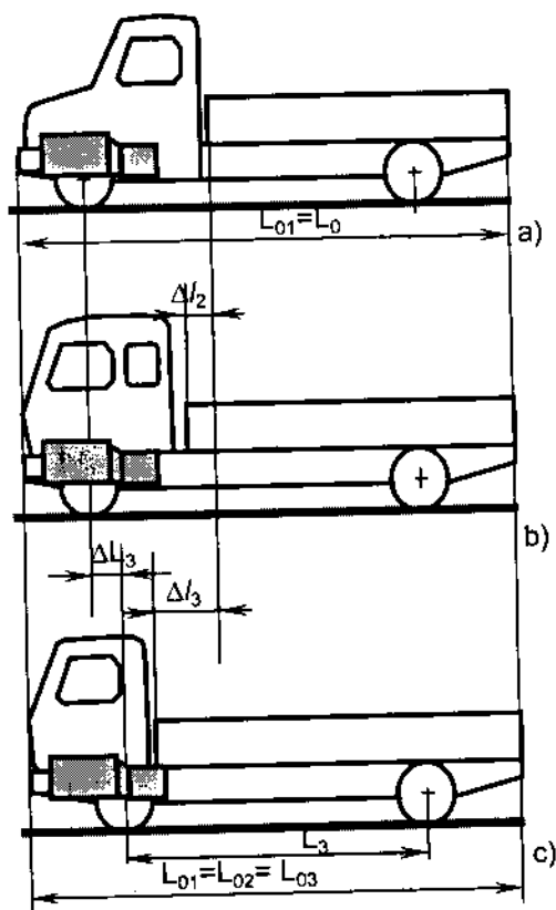
Hình 4-28: Khả năng tăng chiều dài sử dụng hữu ích với kết cấu đầu rụt của xe tải
