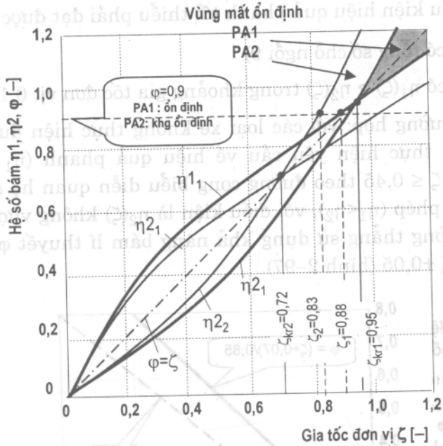
Hình 2-95: Vùng ổn định khi phanh với sự phân chia lực phanh khác nhau (x = 0,475; y = 0,211; i = F_{p2}/(F_{p1} + F_{p2})) i_1 = 0,274 (PA1); i_2 = 0,323 (PA2);
