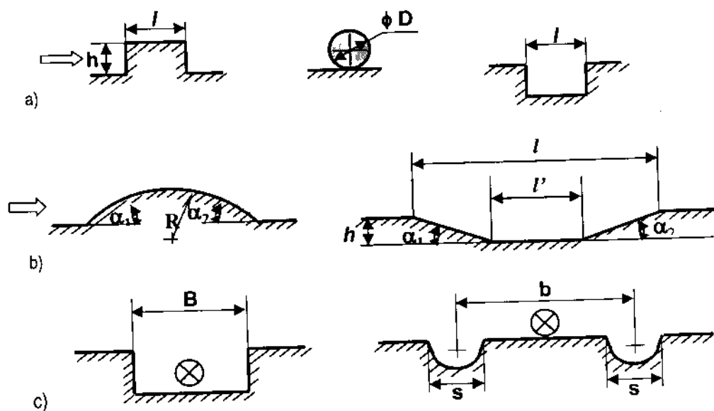
Hình 2-54: Các dạng điển hình của chướng ngại trên đường xấu
