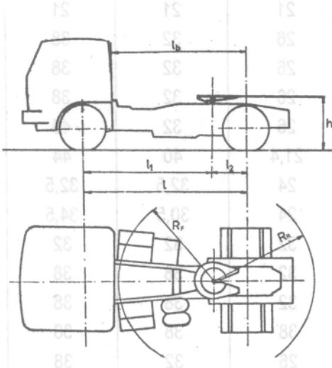
Hình 4-37: Các kích thước cơ bản của ô tô đầu kéo
