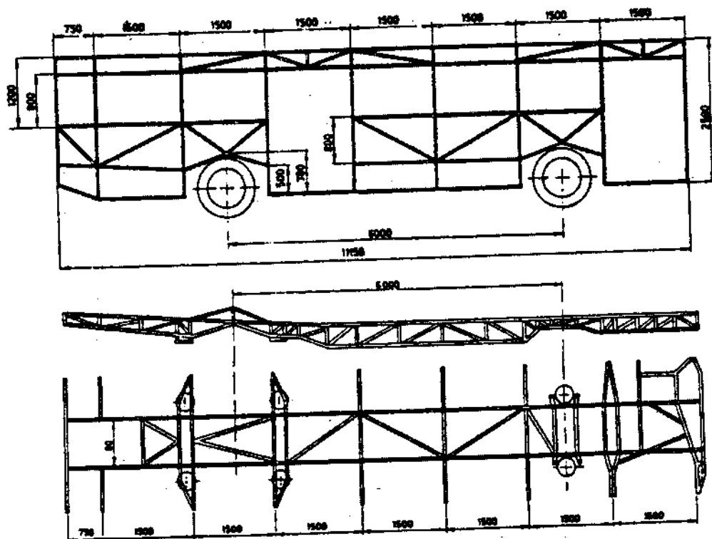
Hình 4-66: Cấu trúc khung dàn của ô tô buýt tiêu chuẩn
