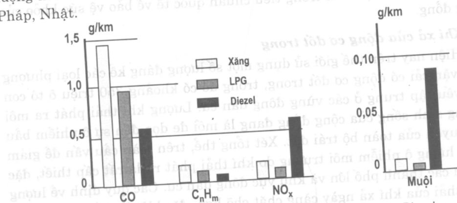
Hình 2-46: So sánh khí xả của các loại nhiên liệu Xăng, LPG, Diesel
