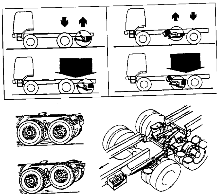
Hình 4-40: Cấu trúc đoàn xe kéo bán rơmooc có thể có khả năng nâng 1 trục
