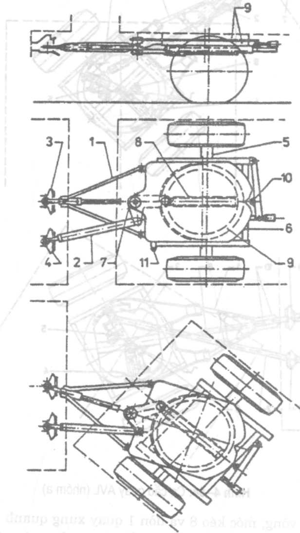
Hình 4-55: Cơ cấu quay KAV (nhóm a)
