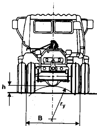
Hình 2-52: Bán kính thông qua ngang r_y và khoảng sáng gầm xe h
