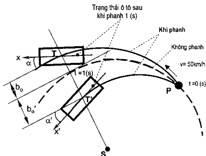
Hình 2-84: Sự quay thân xe khi phanh trên đường vòng
