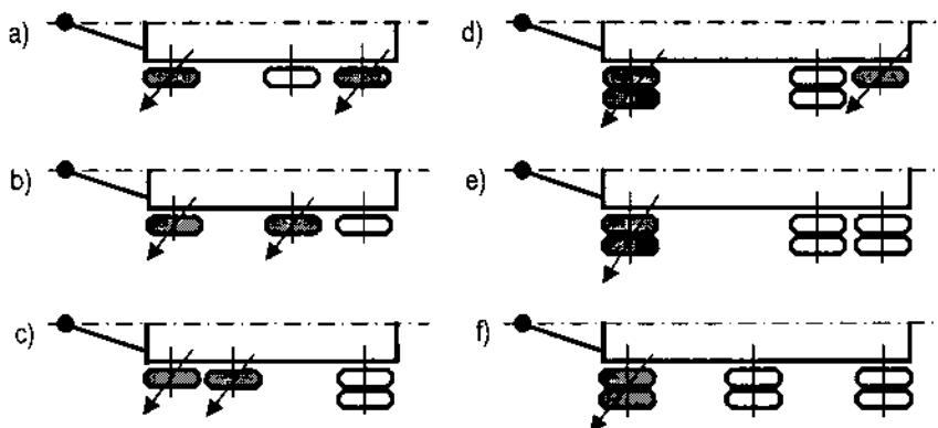
Hình 4-47: Các phương pháp bố trí trục đoàn xe rơmooc nhiều trục
