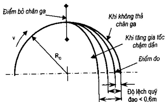
Hình 2-79: Đo độ lệch quỹ đạo khi bỏ chân ga
