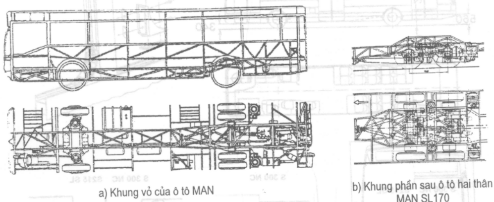
Hình 4-69: Khung vỏ của ô tô MAN và khung phần sau ô tô hai thân SL170
