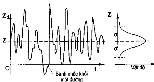
Hình 2-70: Quá trình biến đổi Z_d theo t , và mật độ xác suất
