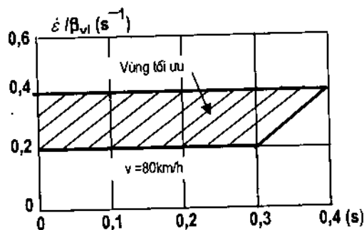
Hình 2-81: Vùng giới hạn cho phép của \varepsilon/\beta_v ( s^{-1} ) và thời gian chậm hiệu quả khi quay vành lái chu kỳ khi có gió bên
