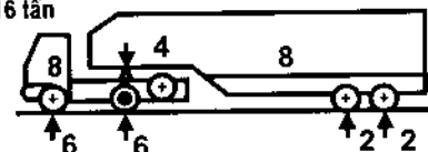
Hình 4-39: Trọng lượng giới hạn của đoàn xe bán rơmooc
