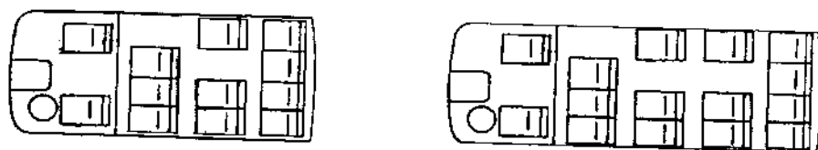
Hình 4-92: Bố trí không gian trong xe chở người
