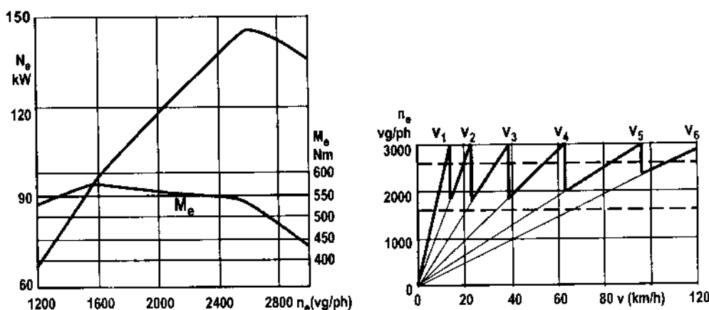
Hình 2-20: Đặc tính động cơ diesel và hộp số 6 số tiến của ô tô tải 11,5 tấn
