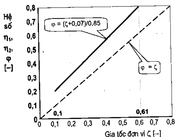
Hình 2-96: Tiêu chuẩn chung cho tất cả ô tô hai cầu
