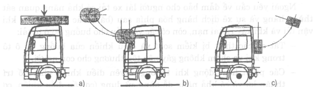
Hình 2-45: Thử nghiệm buồng lái theo tiêu chuẩn của Mỹ FMVSS
