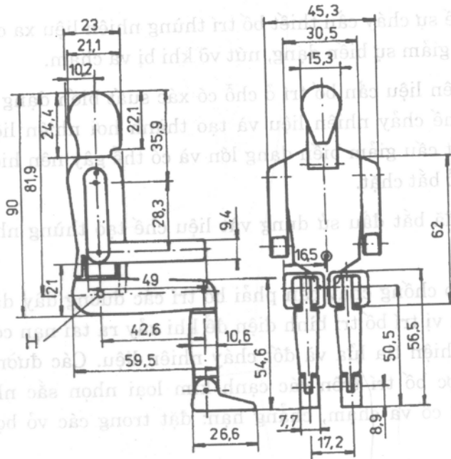
Hình 2-40: Hình mẫu không gian theo tiêu chuẩn ECE R29
