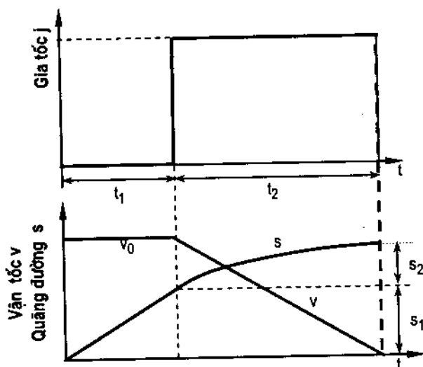
Hình 2-90: Phương pháp tính toán theo ECE
