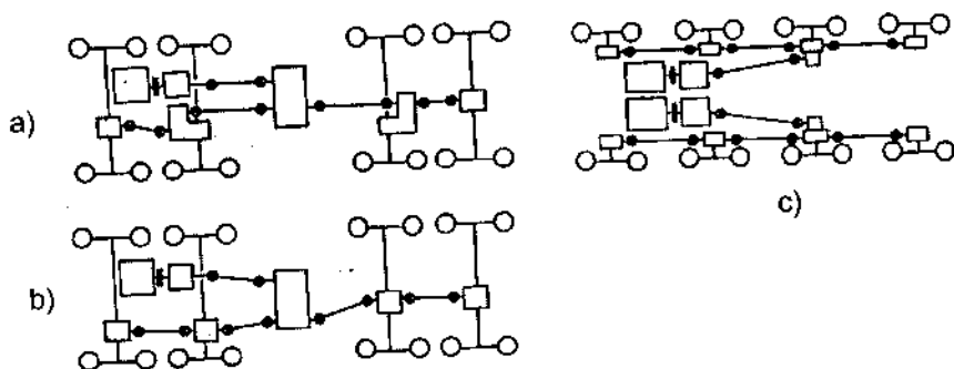
Hình 4-35: Các sơ đồ HTTL ô tô 4 cầu chủ động
