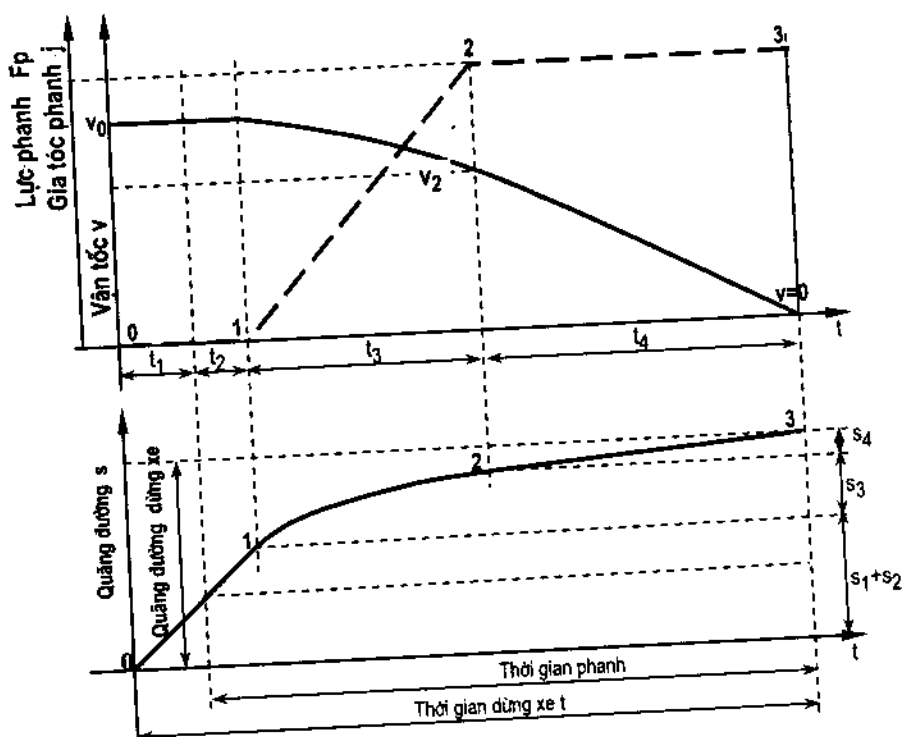
Hình 2-89: Quá trình phanh và phương pháp tính toán
