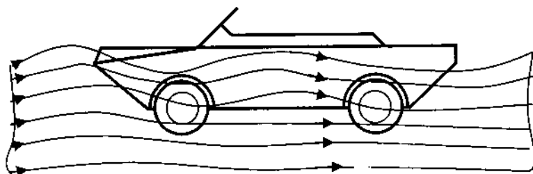
Hình 2-68: Dòng chảy xung quanh ô tô khi bơi
