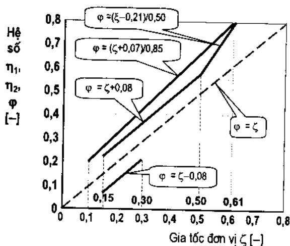
Hình 2-98: Tiêu chuẩn cho ô tô N1
