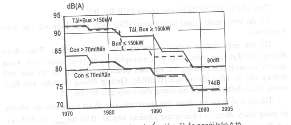
Hình 2-50: Xu hướng tiêu chuẩn giảm độ ồn ngoài trên ô tô
