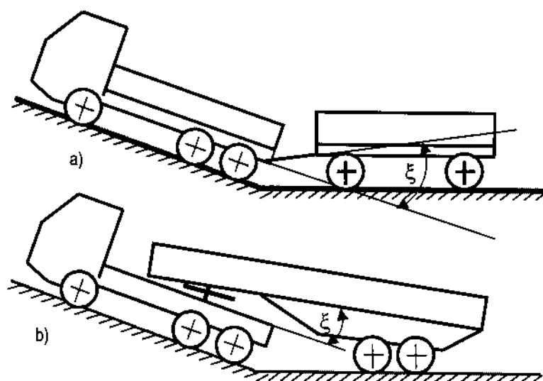
Hình 2-53: Góc bề gãy đoàn xe theo mặt phẳng dọc: a – đối với xe kéo rơmooc, b – đối với xe kéo bán rơmooc.
