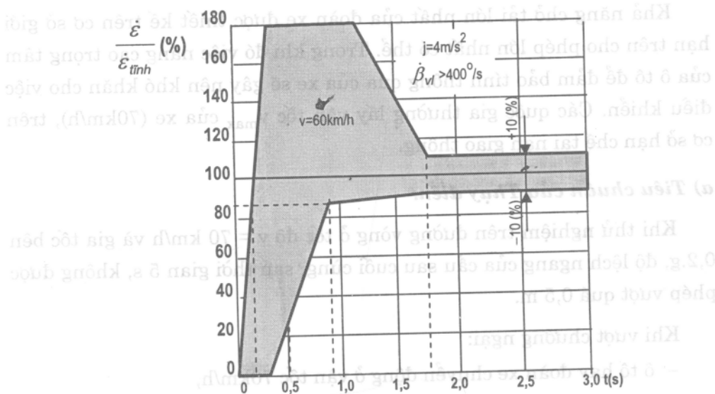
Hình 2–87: Vùng cho phép của hàm chuyển vị (%) khi đánh lái đột ngột cho ô tô tải và buýt
