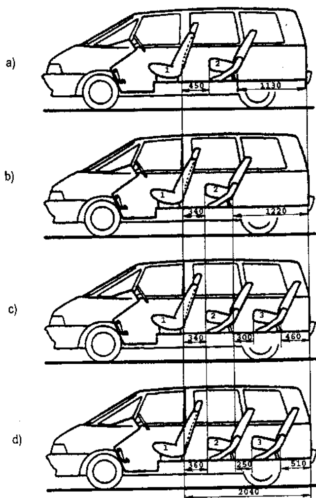
Hình 4-20: Các phương án bố trí Combi lớn
