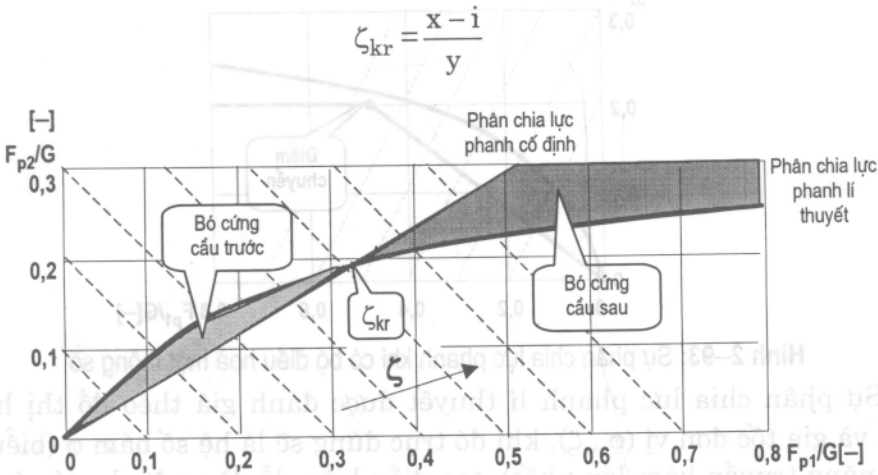
Hình 2-92: Quan hệ của lực phanh trên các cầu
