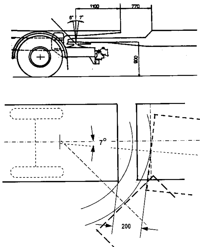
Hình 4-56: Cơ cấu quay AVL (nhóm b)
