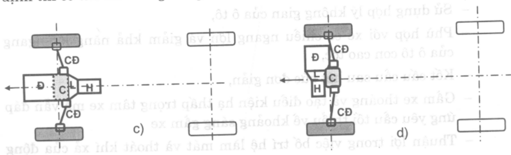
Hình 4-14: Các sơ đồ bố trí chung động cơ nằm trước.
