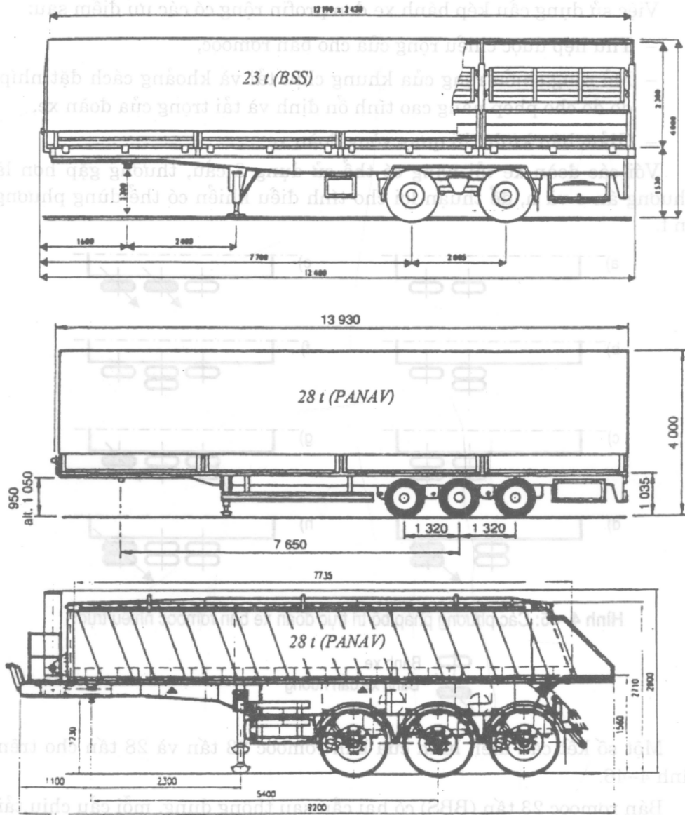
Hình 4-46: Bán rơmooc 2 trục sau – 23 Tấn, 3 trục sau – 28 Tấn
