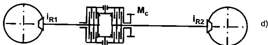
Hình 2-62: Sơ đồ gài truyền lực thường xuyên cho ô tô 4x4
