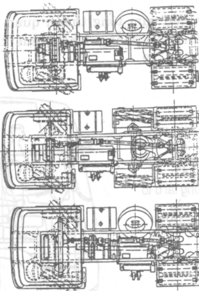
Hình 4-41: Cấu trúc ô tô đầu kéo của hãng MAN-UXT
