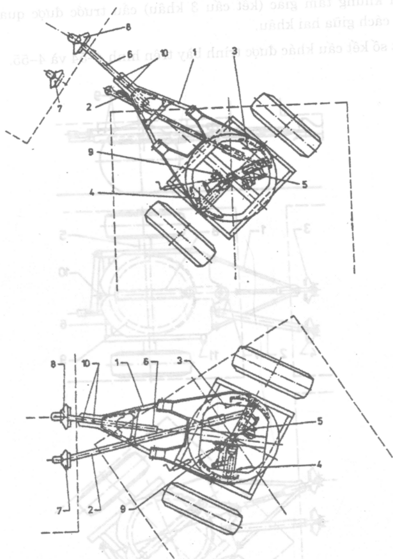
Hình 4-54: Cơ cấu quay AVL (nhóm a)
