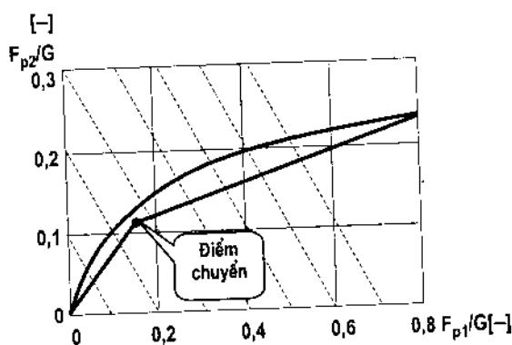
Hình 2-94: Sự phân chia lực phanh khi có bộ điều hoà hai thông số
