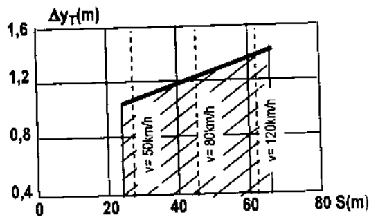
Hình 2-80: Vùng giới hạn cho phép của độ lệch bên trọng tâm ô tô \Delta y_T (m) sau 2s khi có gió bên
