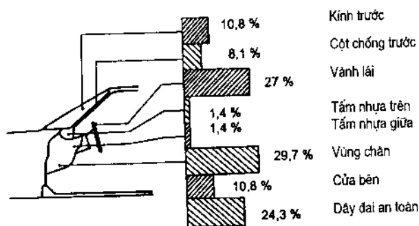
Hình 2-41: Xác suất gây thương tích khi va chạm trước
