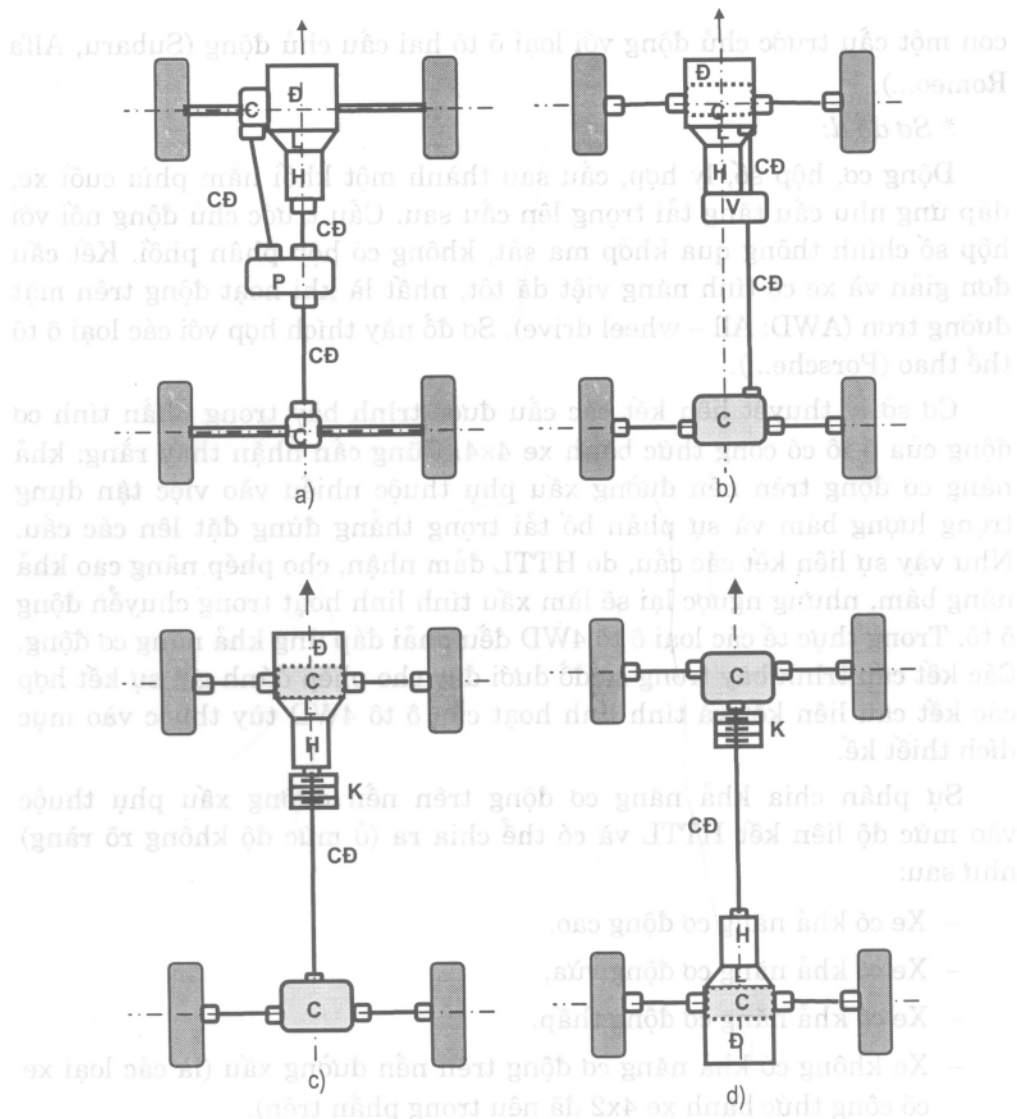
Hình 4-16: Các sơ đồ bố trí chung hai cầu chủ động.
