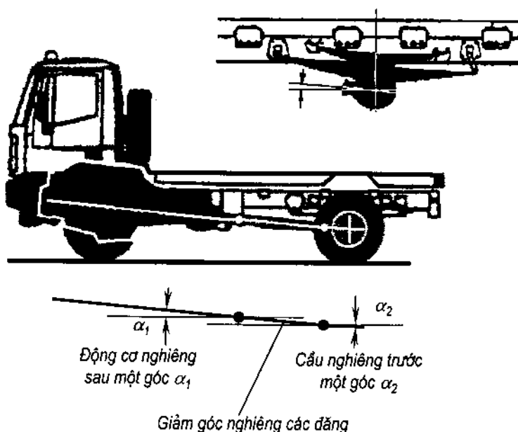
Hình 4-36: Bố trí giảm góc nghiêng các đặng
