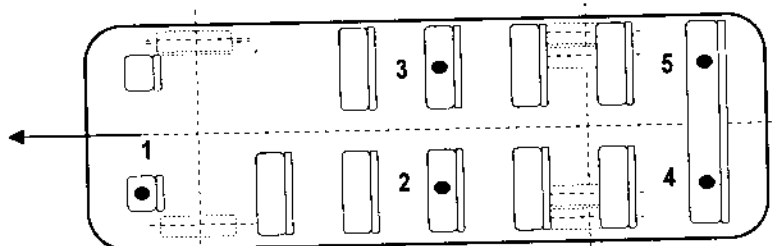
Hình 2-33. Đo độ ồn trong cửa ô tô buýt
