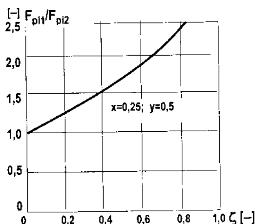
Hình 2-91: Sự phân chia lực phanh lý thuyết theo gia tốc đơn vị
