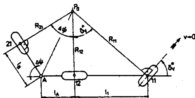
Hình 4-82: Nguyên lý kiểm soát góc bề gãy đoàn xe buýt hai thân
