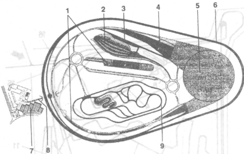
Hình 1-5: Sơ đồ Polygon của hãng BOSCH - Đức
