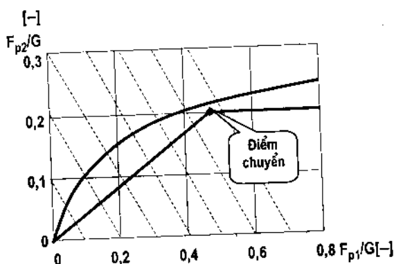
Hình 2-93: Sự phân chia lực phanh khi có bộ điều hoà một thông số
