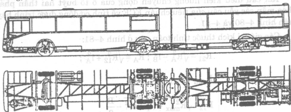
Hình 4-79: Cấu trúc của hãng MAN NG 272 hai thân
