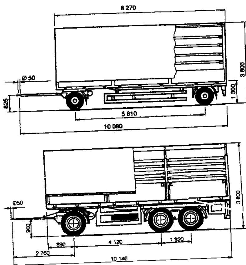
Hình 4-48: Rơmoóc 18 tấn
