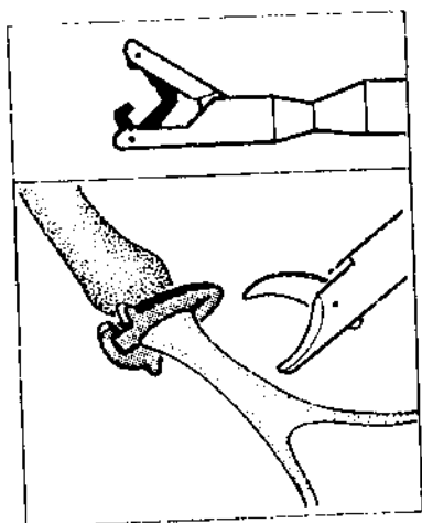
Hình 20: Kỹ thuật cầm máu bằng clip
