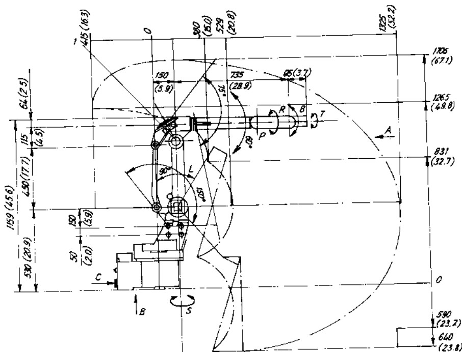
Hình 2.14. Vùng làm việc của robot Motoman
