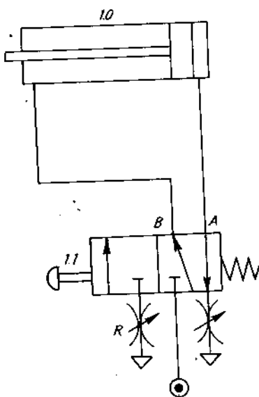
Hình 11.15. Tiết lưu khí xả
