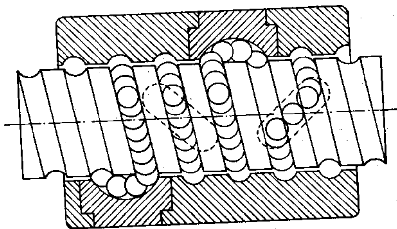
Hình 10.12. Sơ đồ kết cấu bộ truyền vít đai ốc bi
