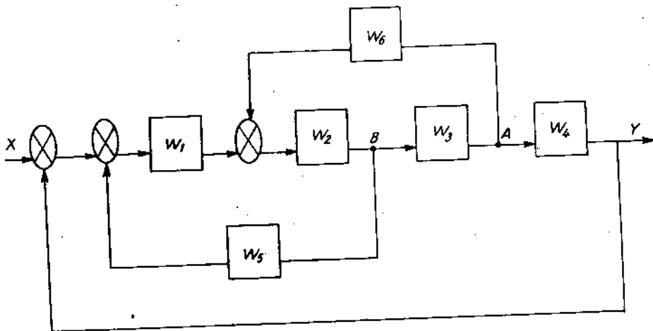
Hình 9.13. Ví dụ sơ đồ cấu trúc
