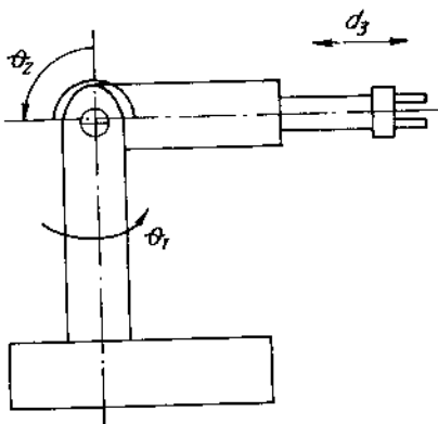
Hình 4.8. Robot RRT
