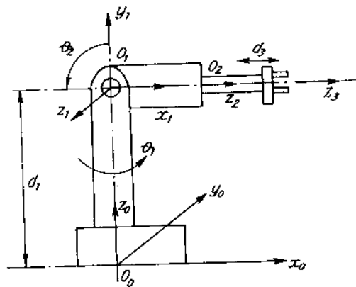
Hình 4.9. Đặt các hệ toạ độ theo phương án 1
