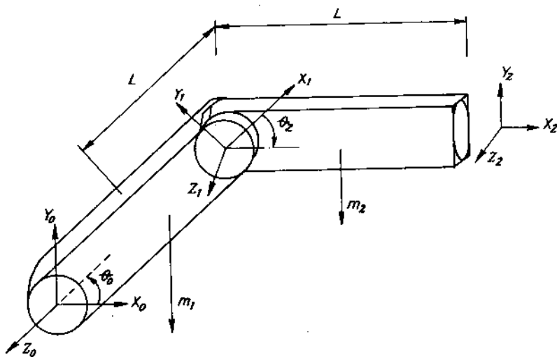
Hình 8.1. Cơ cấu tay máy 2 khâu
