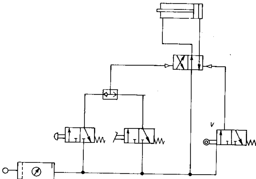
Hình 11.5. Sơ đồ mạch khí nén
