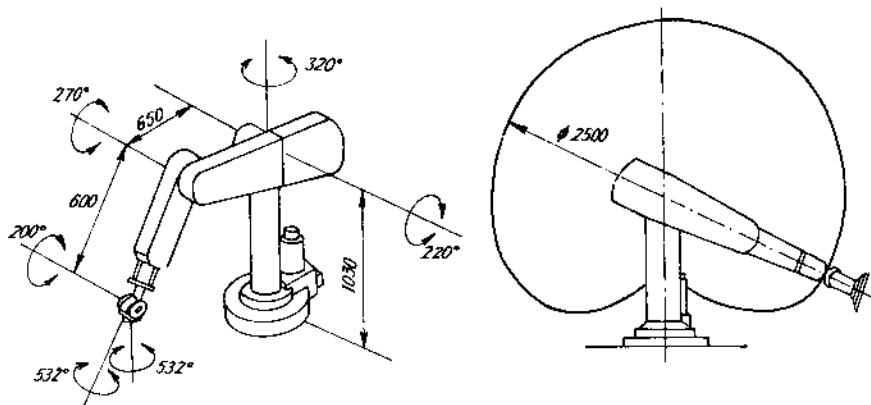
Hình 2.12 . Robot Puma 760 với hệ tọa độ phỏng sinh.
