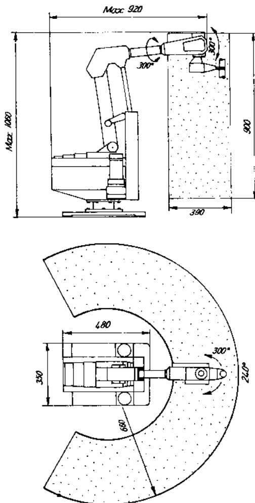
Hình 2.16. Robot RP
