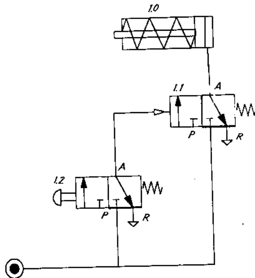
Hình 11.21. Điều khiển gián tiếp các xilanh tác động đơn
