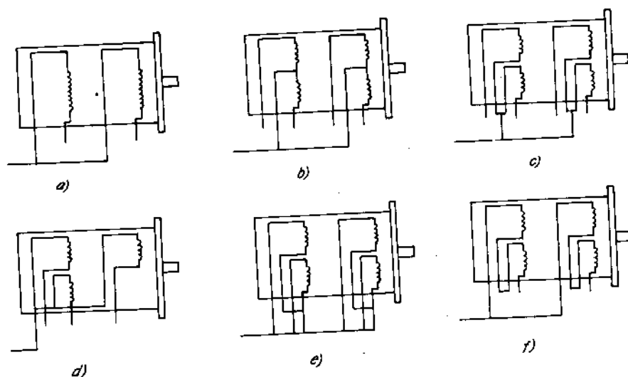
Hình 10.15. Pha của động cơ và các cách nối dây.
