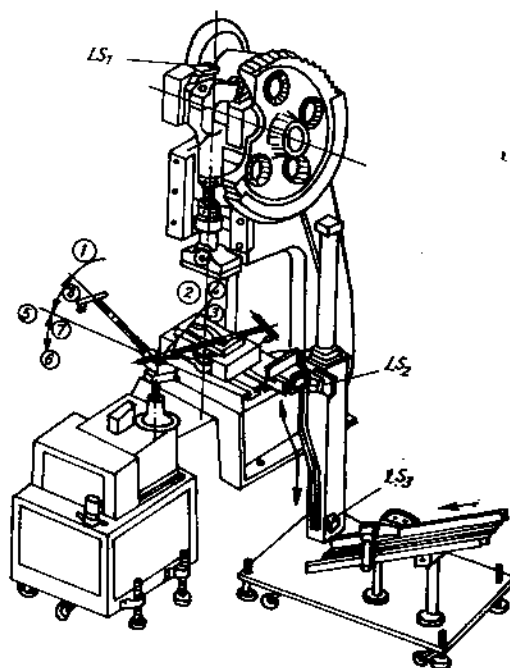
Hình 1.5. Sơ đồ làm việc của robot RBM - 5 phục vụ máy đúc áp lực cỡ nhỏ.
