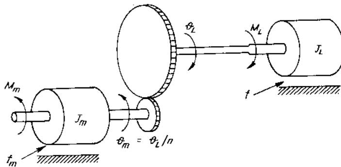
Hình 9.20. Sơ đồ động cơ điện cùng phụ tải
