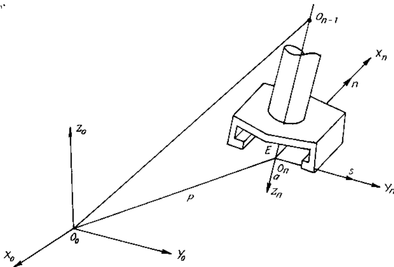
Hình 4.1. Hệ toạ độ gắn liền với bàn kẹp
