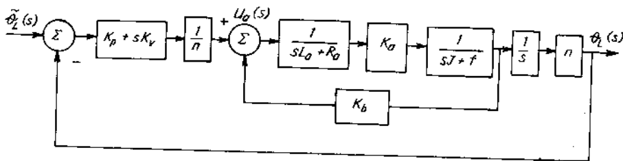
Hình 9.22. Sơ đồ điều khiển chuyển dịch 1 khớp động có liên hệ phản hồi.
