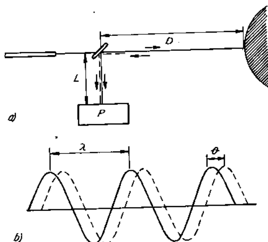
Hình 12.21. Đo khoảng cách theo thời gian truyền tín hiệu.
