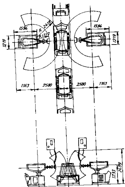
Hình 1.7. Sơ đồ làm việc của robot trên dây chuyền hàn vỏ ô tô Toyota.
