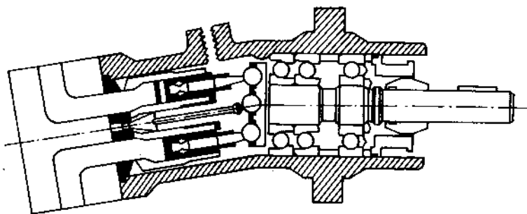
Hình 10.33. Mô tơ thuỷ lực có bloc xilanh nghiêng một góc với trục quay.
