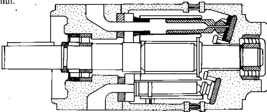
Hình 11.32. Mô tơ thuỷ lực chiều trục (hãng Rexroth-Sigma).
