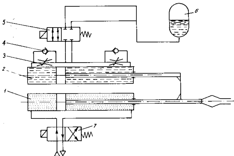
Hình 11.41. Sơ đồ hệ truyền dẫn thuỷ lực - khí nén
