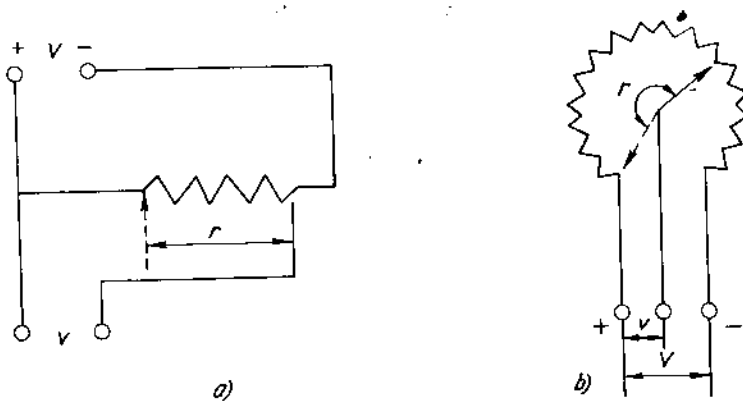
Hình 12.1. Sơ đồ mạch chiết áp
