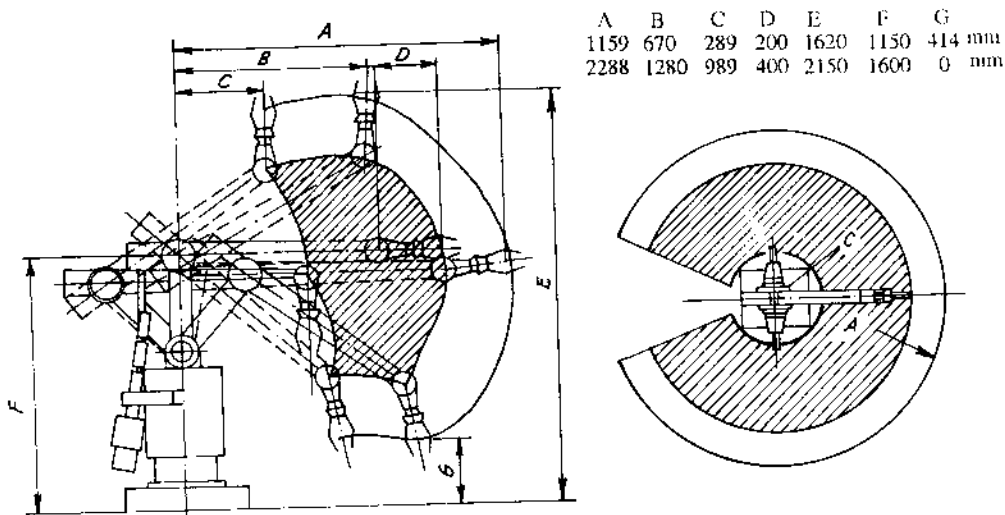
Hình 2.13. Vùng làm việc của Robot IRb-6 và IRb-60
