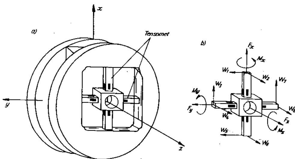
Hình 12.9. Cảm biến lực chữ thập
