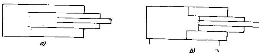
Hình 11.3. Các xilanh lồng.
