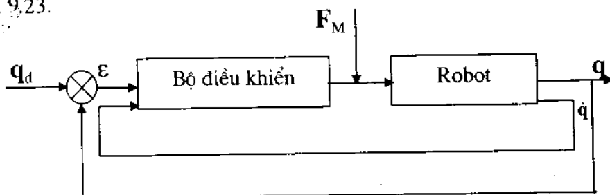
Hình 9.23. Sơ đồ hệ thống điều khiển
