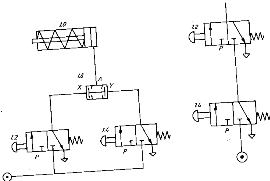
Hình 11.19. Điều khiển van song áp.
