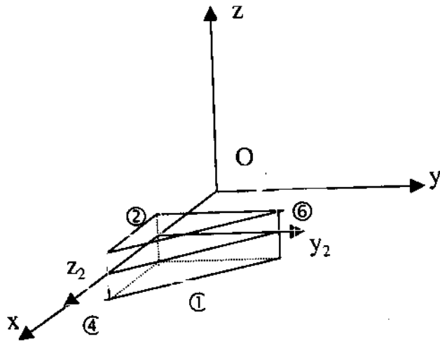
Hình 7.5. Vật thể sau các phép biến đổi H_2 = T_p(4,0,0) \cdot R(y,90^\circ)
