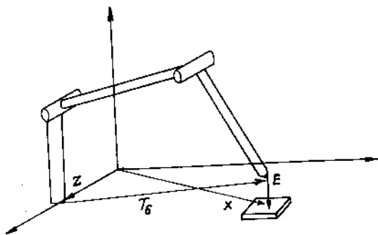
Hình 4.11. Robot và vật thể đối tác
