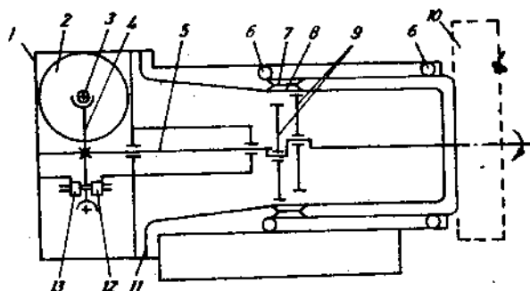
Hình 10.6. Sơ đồ khớp quay robot dùng bánh răng sóng làm việc ở môi trường độc biệt
