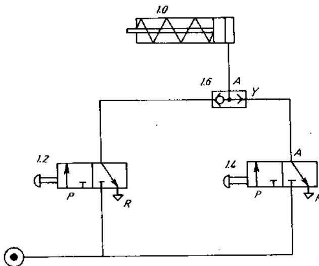
Hình 11.11. Điều khiển dùng van con thoi.
