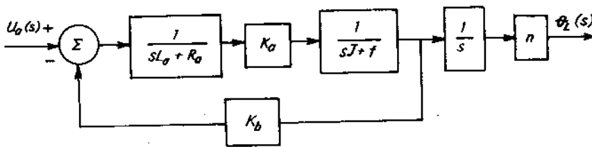
Hình 9.21. Hàm truyền chuyển động một bậc tự do
