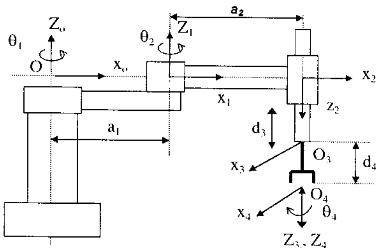
Hình 4.7. Robot SCARA và các hệ toạ độ
