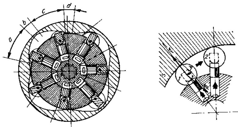
Hình 11.34. Mô tơ thủy lực hướng kính (hãng Samm)
