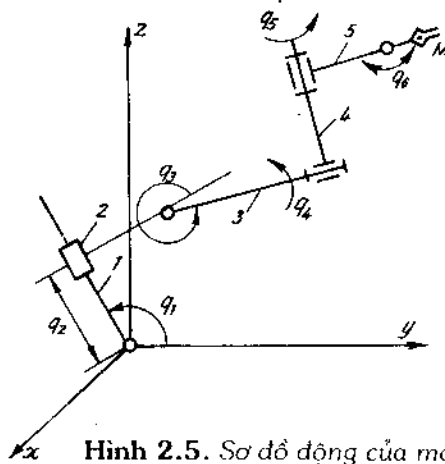
Hình 2.5. Sơ đồ động của một tay máy tọa độ suy rộng.
