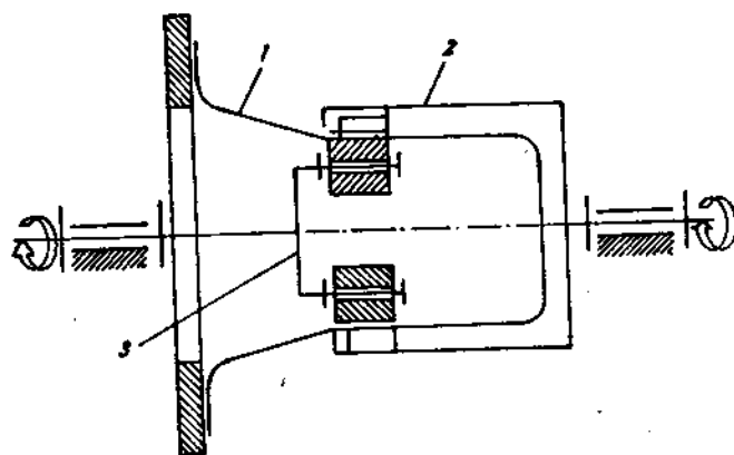
Hình 10.3. Bộ truyền bánh răng sóng xuyên qua vách ngăn
