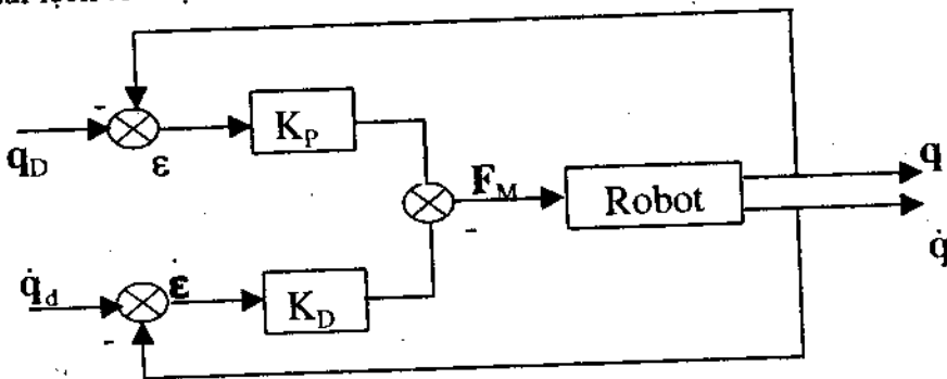
Hình 9.25. Sơ đồ cấu trúc hệ thống với bộ điều khiển PD
