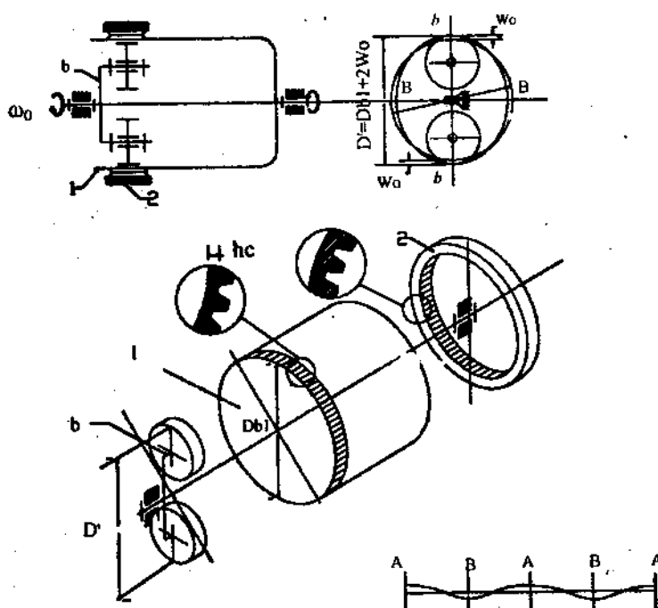
Hình 10.1. Bộ truyền bánh răng sóng.
