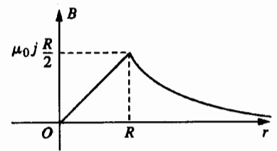
Hình 20. Sự biến thiên của B(r) .
