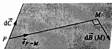
Hình 4. d\vec{B} vuông góc với mặt phẳng xác định bởi điểm P và các vector d\vec{C} và \vec{PM} .
