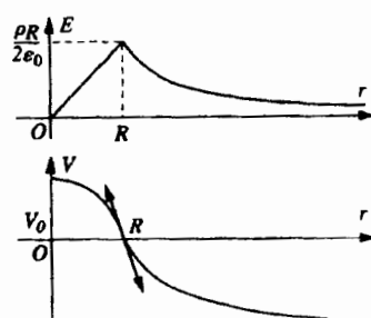
Hình 13. Trường và thế của một trụ vô hạn.
