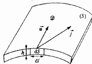
Hình 7a. Vỏ được định hướng với h nhỏ.
