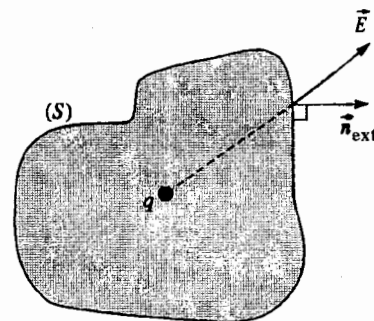
Hình 3. Mặt kín S chứa điện tích q .
