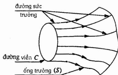
Hình 13. Ống trường.
