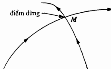
Hình 14. Điểm trường bằng không.
