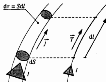
Hình 3. Mạch hình sợi chỉ.
