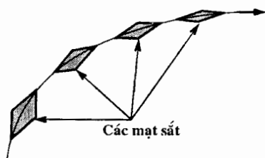
Hình 9. Các phần tử mạt sắt giống như các nam châm con định hướng song song với từ trường
