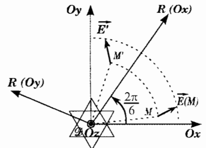
Hình 18. Phân bố bất biến với phép quay.
