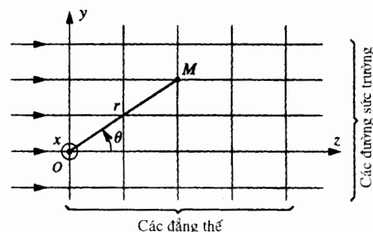
Hình 6. \vec{E} = E_0 \vec{u}_z
