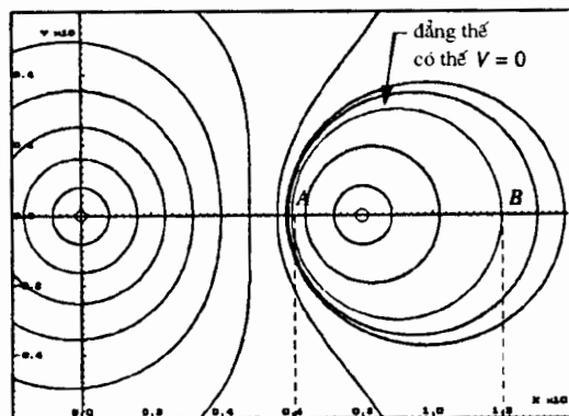
Hình 11. Đẳng thế có thế V = 0 là một vòng tròn có đường kính AB, với A(+6) và B(+12) .
