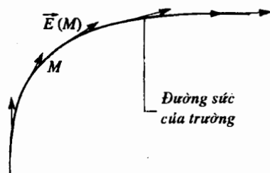
Hình 6. Đường sức của trường.
