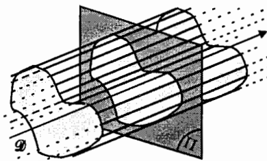
Hình 9. Phân bố bất biến đối với phép tịnh tiến dọc theo một trục.
