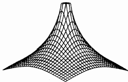
Hình 4. Thế của một sợi dây thẳng vô hạn
