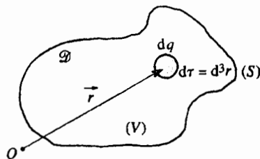
Hình 5. Phân bố khối của các điện tích.
