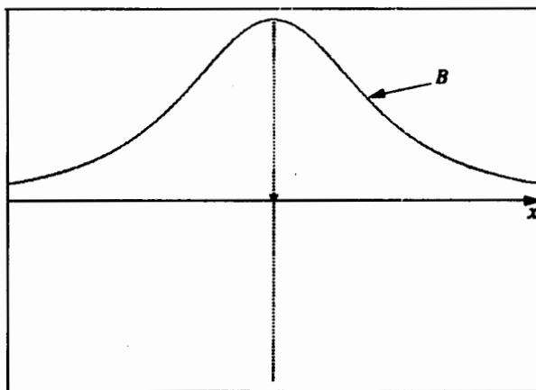
Hình 30. Trường ở trên trục của một vòng dây.
