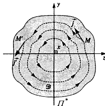
Hình 14. Phản đối xứng phẳng : \vec{j}' là vector đối của vector đối xứng của \vec{j} . \Pi^* là một mặt phẳng phản đối xứng.
