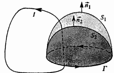
Hình 7. Dòng qua hai mặt tựa trên \Gamma .
