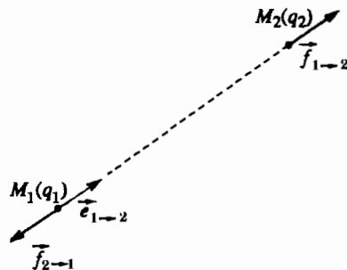
Hình 1. Lực tương tác giữa hai điện tích đứng yên ( q_1 q_2 > 0 ).
