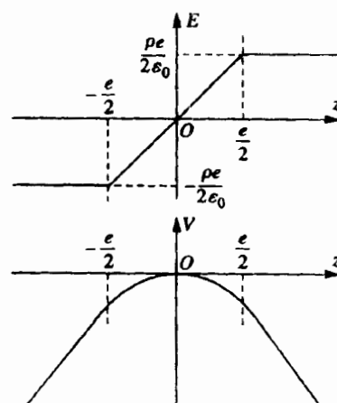
Hình 11. Trường E và thế V tạo ra bởi lớp phẳng vô hạn dày e và có mật độ điện khối đều \rho .
