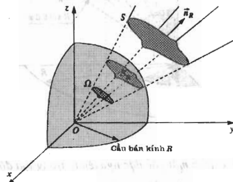
Hình 3. \Omega = \frac{S_R}{R^2} .
