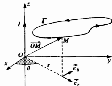
Hình 3. Đường cong kín \Gamma không quanh lấy sợi dây.
