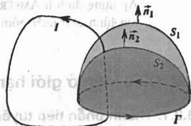
Hình 7. Dòng qua hai mặt tựa trên \Gamma .
