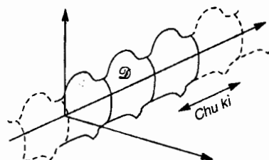
Hình 10. Phân bố bất biến do phép tịnh tiến.
