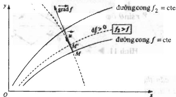
Hình 4. \text{grad} f được định hướng theo chiều của hàm f tăng.
