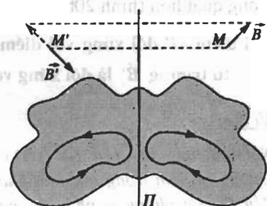
Hình 16b. Các trường của hai điểm đối xứng.
