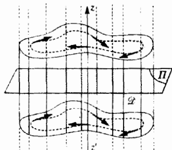
Hình 15. Sự bất biến bởi phép tịnh tiến đối với các dòng phẳng
