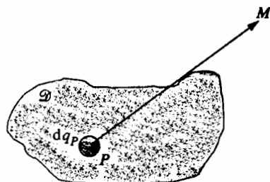
Hình 4. Phân bố điện tích \mathcal{D} .
