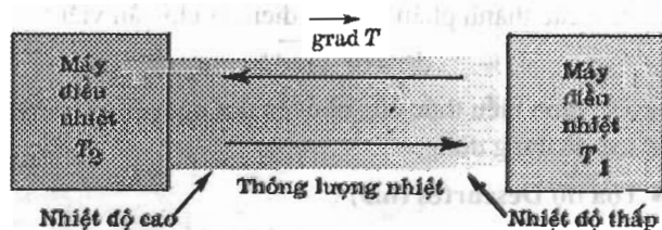
Hình 6. T_2 > T_1
