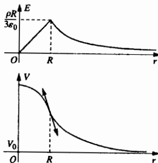
Hình 18. Trường và thế của một khối cầu tích điện.
