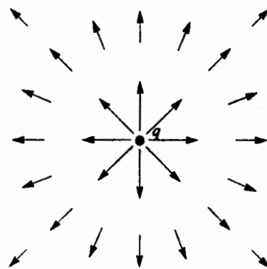
Hình 2. Trường của một điện tích điểm ( q > 0 ).
