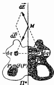
H.14a. Phân đối xứng phẳng.
