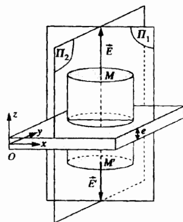
Hình 10. Sử dụng các tính đối xứng và sự lựa chọn “mặt Gauss”.
