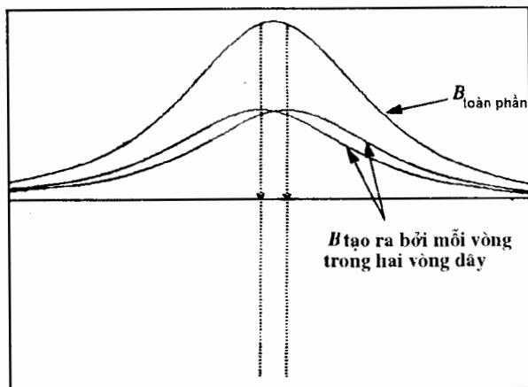
Hình 31b. Hình dáng của B(x) trong trường hợp của hai vòng dây có dòng giống nhau chạy qua.
