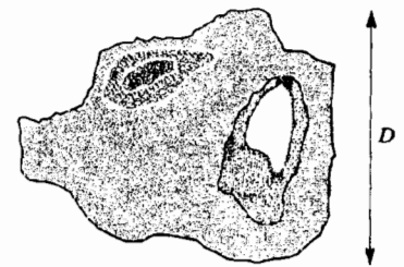
Hình 3. Quan sát ở thang vĩ mô.
