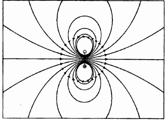
Hình 7b. Các đường sức trường từ tĩnh.
