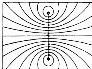
Hình 12. Các đường sức trường của vector cảm ứng từ tạo ra bởi một vòng dây.
