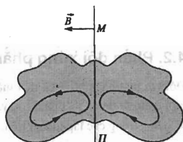
Hình 16a. Từ trường trên một mặt phẳng đối xứng.
