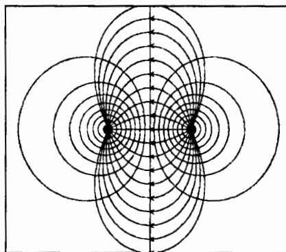
Hình 14. Vết của các mặt đẳng thế và các đường sức trường (trường) trực giao.
