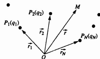
Hình 3. Phân bố các điện tích điểm.
