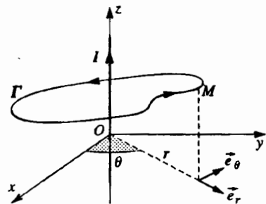
Hình 2. Đường cong kín \Gamma quanh lấy một sợi dây theo chiều thuận.
