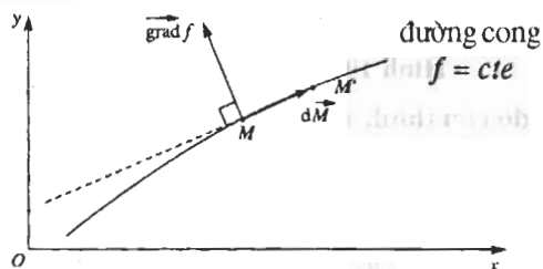
Hình 3. \text{grad} f vuông góc với mặt f = \text{cte} .
