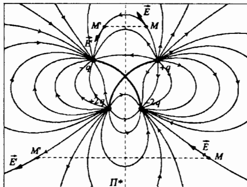
Hình 15b. Trường tĩnh điện \vec{E}' là vector đối của đối xứng của \vec{E} .
