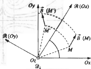
Hình 23. Bất biến bởi phép quay với n = 6 .
