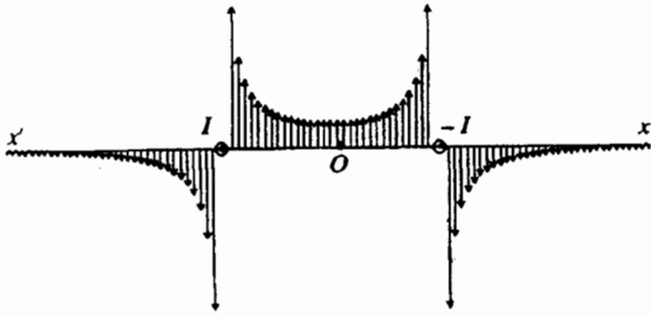
S. 3. Sự phát triển theo đồ thị của \vec{B} trên trục (x'Ox).
