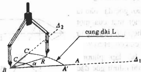
Hình 1. \alpha = \frac{L}{R} .
