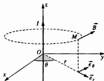
Hình 1. Dây thẳng vô hạn.
