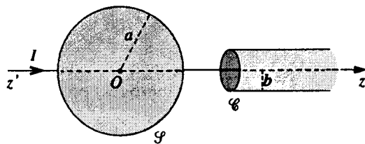
Hình 12. Vật dẫn.
