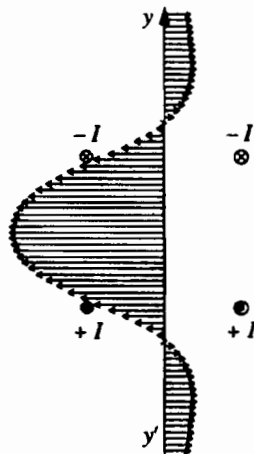
S. 7. Sự phát triển của \vec{B} trên trục (y'Oy) .
