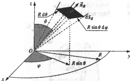
Hình 4. Tính một góc đặc nguyên tố trong tọa độ cầu.
