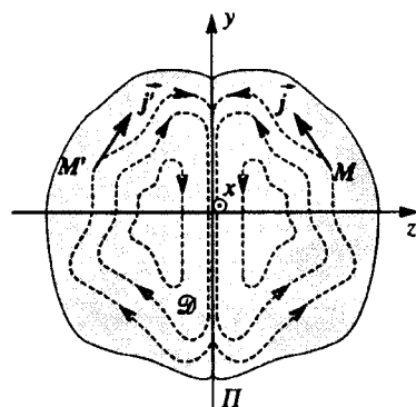
Hình 13. Đối xứng phẳng.
