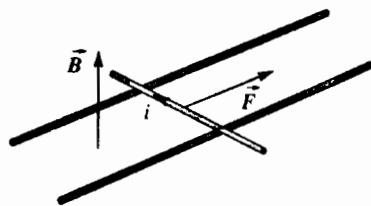
Hình 1. Lực LAPLACE.
