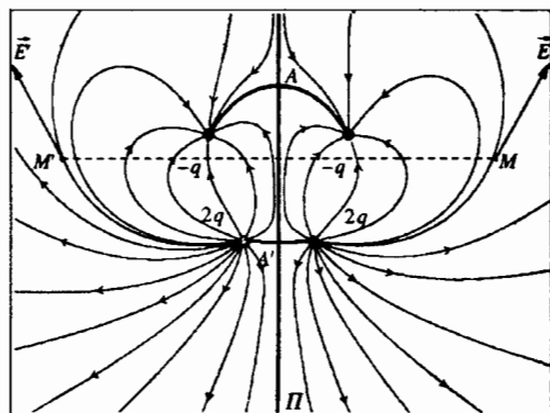
Hình 15a. Sự đối xứng của các trường \vec{E} và \vec{E}' .
