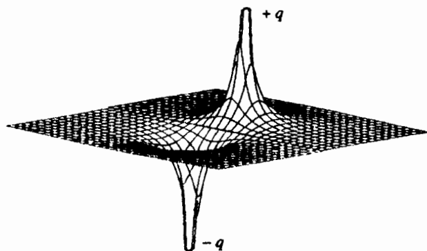
Hình 11. Sự thể hiện của thế tạo ra bởi hai điện tích -q và +q (nét đậm V > 0 , nét nhạt V < 0 ).
