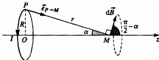
Hình 7. Phần tử từ trường.
