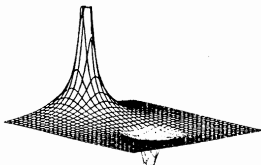
Hình 12. Sơ đồ này cho thấy rõ đẳng thế tròn V = 0 (màu đậm V > 0 và màu nhạt V < 0 ).
