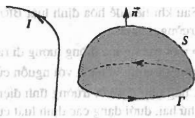
Hình 5. Dòng I không đi qua mặt S tựa trên đường cong kín \Gamma .
