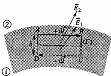
Hình 2. Thành phần tiếp tuyến của \vec{E} là liên tục khi đi qua một mặt mang điện.
