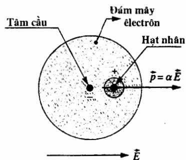
Hình 4. Sự phân cực của một nguyên tử đặt trong trường \vec{E} : \vec{p} = \alpha \vec{E} , với \alpha > 0 .
