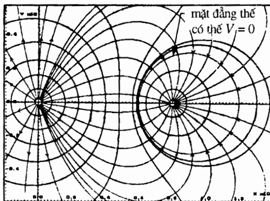
Hình 13. Hình dáng của các đường sức trường.
