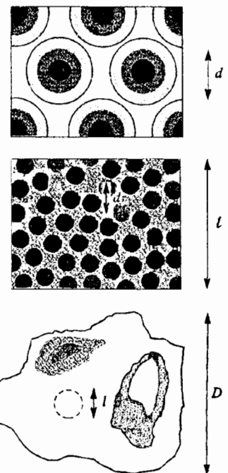
Hình 4. Các thang vi mô d , san bằng l và vĩ mô D .
