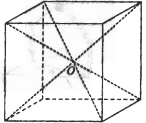
Hình 5. Sáu mặt của lập phương được nhìn từ điểm O dưới cùng một góc đặc.
