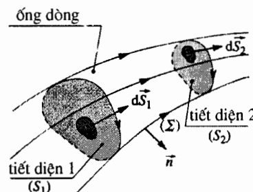
Hình 6. Ống dòng.
