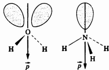
Hình 3. Mômen lưỡng cực của các phân tử H_2O và NH_3 .
