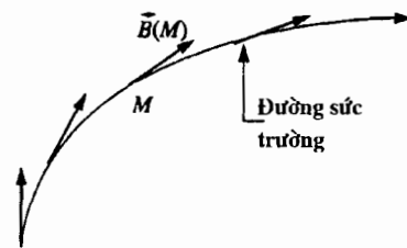
Hình 8. Ví dụ về đường sức trường.
