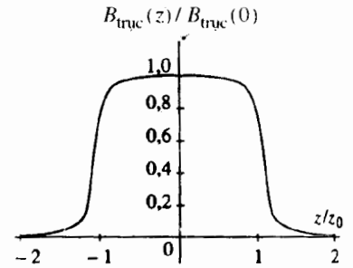
Hình 36. Ống dây với các đầu có hoành độ -z_0 và z_0 .
