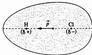
Hình 2. Phân tử lưỡng nguyên tử.
