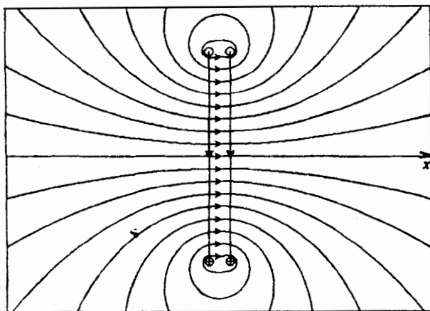
Hình 31a. Các đường sức từ trường của một tập hợp hai vòng dây có dòng điện giống nhau chạy qua.
