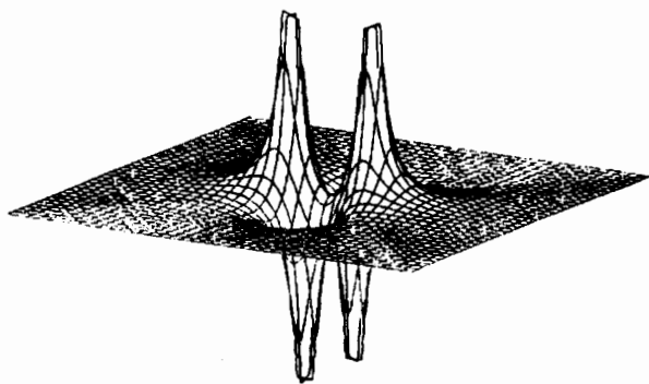
Các đường sức trường và đẳng thế tạo ra bởi bốn điện tích.
