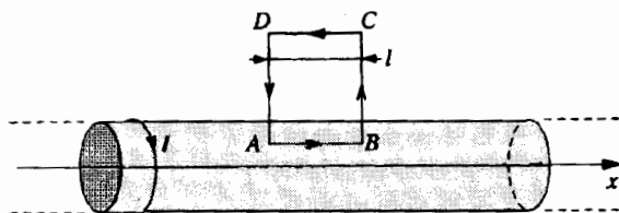
ống dây vô hạn
