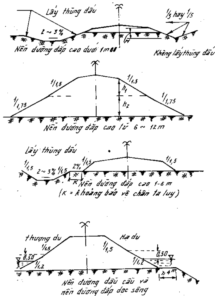
Hình 8 - 2. Các trắc ngang định hình nền đường đắp.
