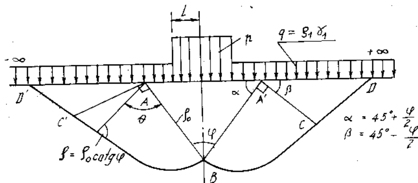
Hình 8 – 30. Sơ đồ tính tải trọng giới hạn theo Prăngđơ.
