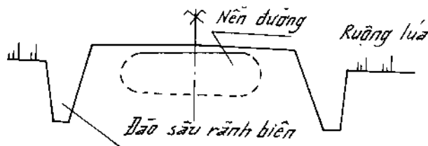
Hình 9 – 14. Đào sâu rãnh biên để cắt đứt và hạ cao độ mức nước ngầm (nền đường qua vùng ruộng lúa không cho phép đắp cao).
