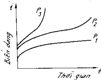
Hình 11 - 2. Hiện tượng lưu biến I = f(t) khi trị số tải trọng tác dụng thay đổi P_1 < P_2 < P_3 .
