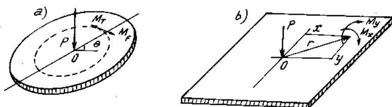
Hình 12 - 5. Sơ đồ tính toán mômen uốn do tải trọng tập trung tác dụng cách tiết diện tính toán một khoảng cách r gây ra. a - trong toạ độ một cực ; b - trong toạ độ x, y.
