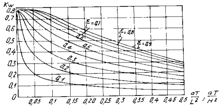
Hình 9 - 8. Đồ thị xác định trị số K_w .
