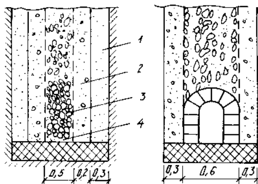
Hình 13 – 35. Rãnh thoát nước ngầm có các lớp vật liệu thay đổi theo chiều đứng. 1 – cát ; 2 – sỏi ; 3 – đá dăm nhỏ ; 4 – đá
