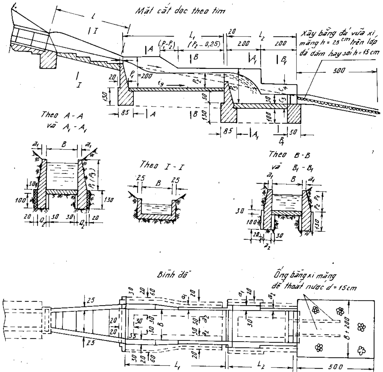
Hình 13-28. Cấu tạo bậc nước bằng bê tông sâu 1 – 2m.
