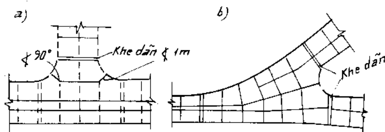
Hình 12-3. Bố trí chia tấm tại các chỗ giao nhau.
