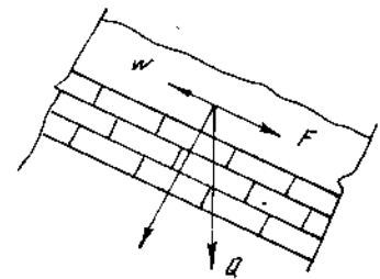
Hình 8 - 13. Sơ đồ tính ổn định sườn dốc trường hợp mặt trượt phẳng.
