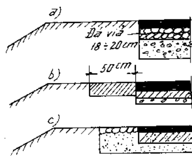
Hình 10 – 7. Cấu tạo gia cố lề đường dọc mép áo đường a – gia cố bằng đá vữa; b – bề dày đất gia cố; c – bề dày đá lát, cuội sỏi.
