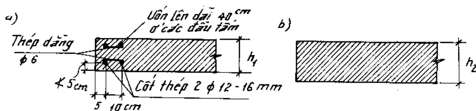
Hình 12 – 2. Cấu tạo mặt cắt ngang tấm bê tông xi măng mặt đường. a – có dùng cốt thép tăng cường mép tấm (bề dày tấm mỏng hơn) ; b – không dùng cốt thép (bề dày tấm dày hơn).
