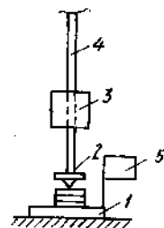
Hình 11 – 18. Sơ đồ thiết bị chùy xung lực. 1 – tấm ép có đường kính D = 34\text{cm} ; 2 – lò xo ; 3 – quả tạ ; 4 – thanh dẫn hướng ; 5 – máy ghi chấn động cầm tay.
