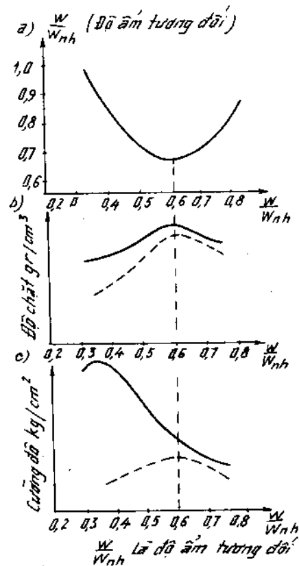
Hình 9 - 13. Kết quả thực nghiệm về tính ổn định nước của đất sau khi đầm nén — đường liên là mẫu đất chưa ngâm nước — đường đứt là sau khi ngâm nước.
