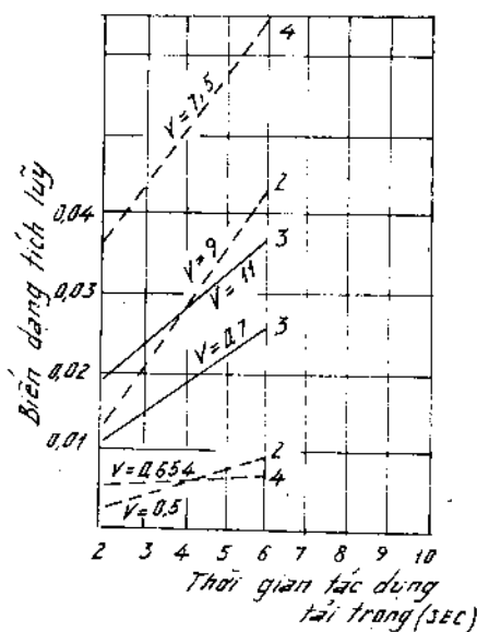
Hình 11 – 6. Ảnh hưởng của thời gian tác dụng tải trọng đến trị số tích lũy biến dạng. v – tốc độ gia tải ; 1, 2, 3, 4 là số hiệu mẫu thí nghiệm.
