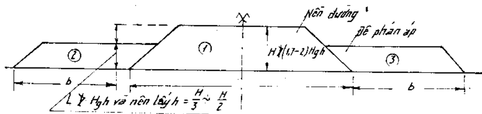
Hình 8 – 28. Đắp thêm bề phản áp hai bên để tăng sự ổn định của nền đắp.
