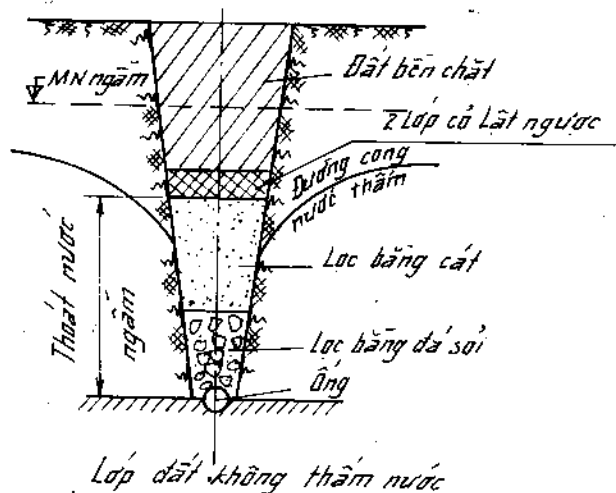
Hình 13-32. Rãnh thoát nước ngấm kiểu kín.
