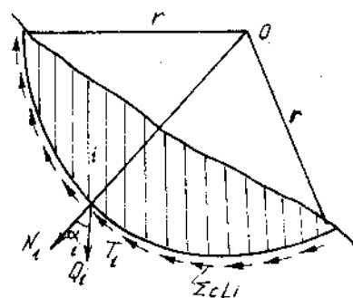
Hình 8 – 15. Sơ đồ tính ổn định sườn dốc trường hợp trượt quay (O là tâm trượt).
