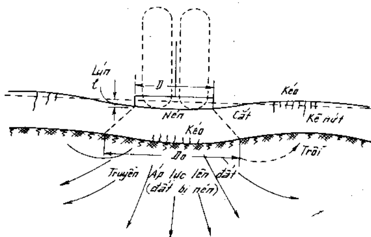
Hình 11 - 7. Các hiện tượng phá hoại áo đường mềm ở trạng thái giới hạn dưới tác dụng của tải trọng xe chạy.
