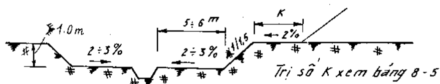
Hình 8 – 3. Mặt cắt ngang thùng đấu.
