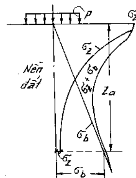
Hình 9 – 10. Sơ đồ xác định phạm vi khu vực tác dụng ( z_a ) ;
