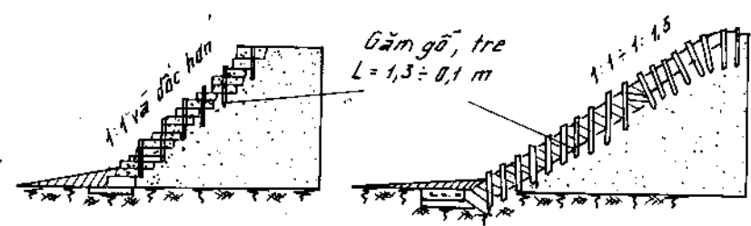
Hình 13 - 3. Lát cô chất thành tường.
