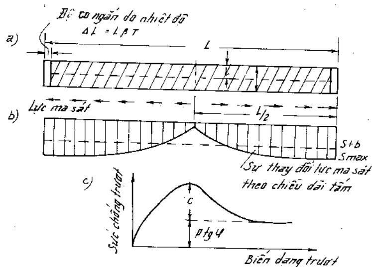
Hình 12 – 9. Sơ đồ tính toán xác định chiều dài tấm (khoảng cách giữa hai khe co).
