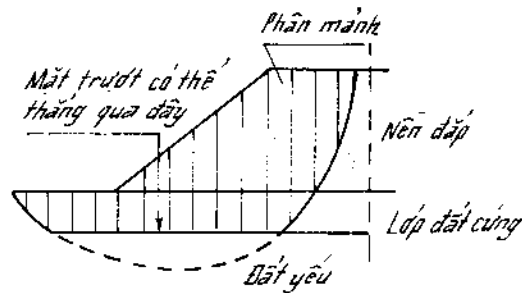
Hình 8 – 23. Ứng dụng phương pháp phân mảnh cổ điển trường hợp đất không đồng nhất và có tầng yếu ở dưới.
