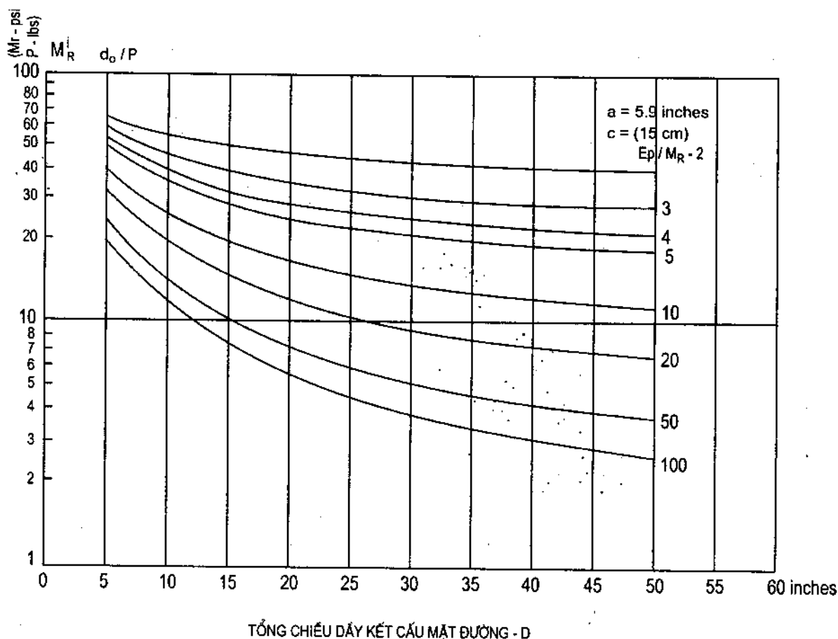
Hình 11 – 24. Toán đồ để xác định tỉ số \frac{E_p}{M_R^i} khi biết M_R^i , d_o , P với a_c = 15\text{ cm} (5,9 inches)
