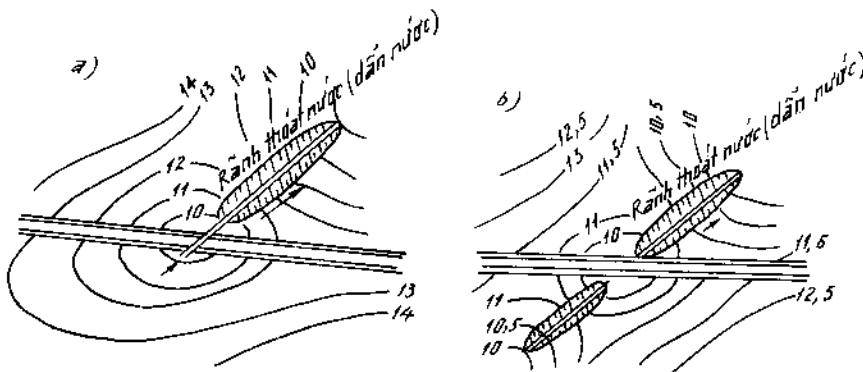
Hình 13 – 14. Sơ đồ thiết kế rãnh tập trung nước để dẫn nước từ nơi trũng của nền đường.
