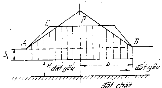
Hình 8 - 31. Sơ đồ tính toán tải trọng giới hạn Iugenxon.
