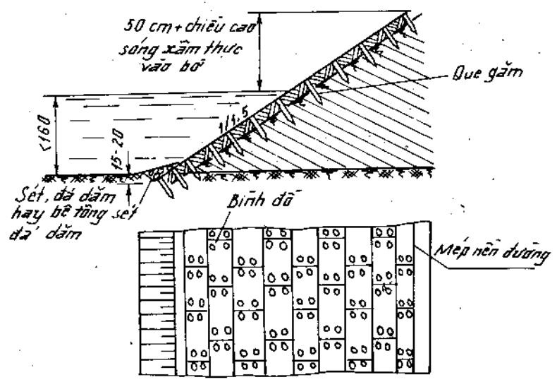
Hình 13 - 1. Lát cô nằm trên taluy.
