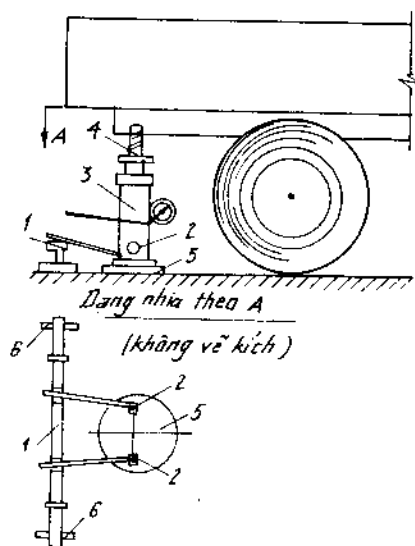
Hình 11 – 17. Thí nghiệm ép ở hiện trường.
