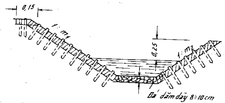
Hình 13 - 4. Gia cố đáy rãnh bằng đá dăm, tường bằng lát cô.
