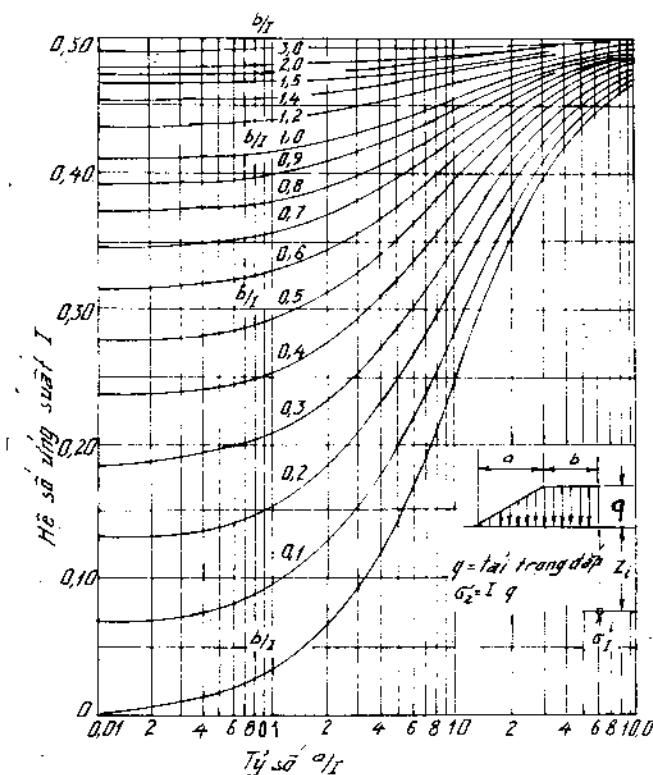
Hình 8 – 34. Toán đồ Osterberg để tính ứng suất (áp lực)
