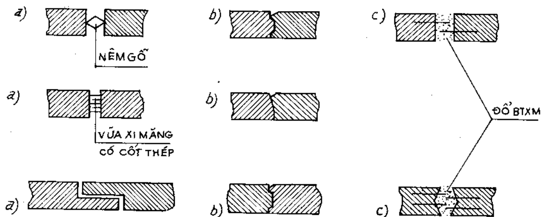
Hình 12 - 12. Các hình thức liên kết giữa các tấm
