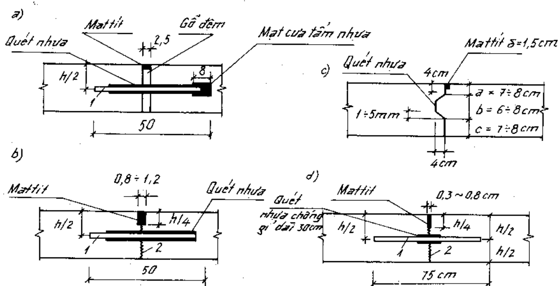
Hình 10 - 9. Cấu tạo khe áo đường bê tông xi măng.
