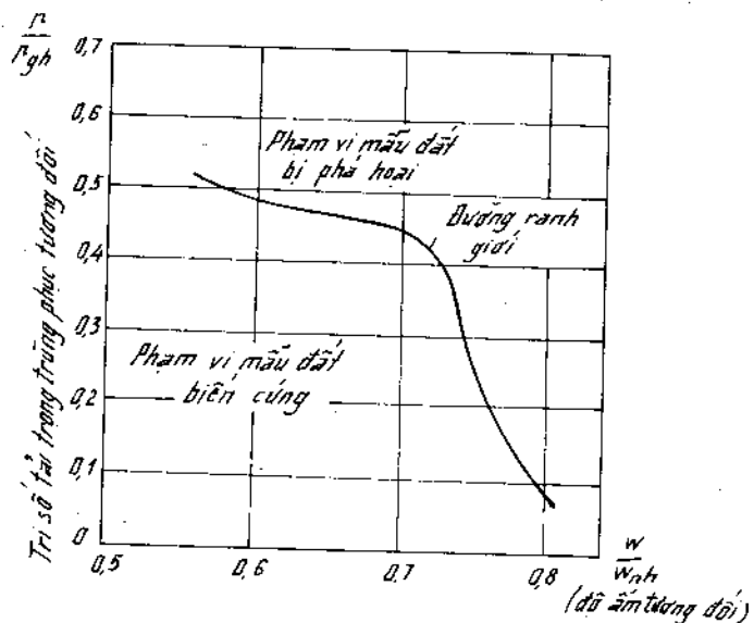
Hình 9 - 1. Quan hệ giữa trạng thái cuối cùng của đất với tác dụng của tải trọng trùng phục (đất á sét bụi):
