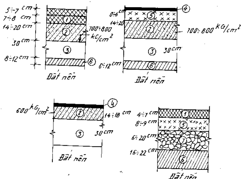
Hình 10 - 10. Các kết cấu áo đường mềm cấu tạo kín (lề đường đủ rộng để nước ngập không thấm vào vùng dưới đáy áo đường) : 1 - bê tông nhựa ; 2 - đất hoặc đá gia cố chất liên kết vô cơ ; 3 - đất nền chặt với hệ số đầm nén K = 1.02 \div 1.04 ; 4 - lớp tráng nhựa ; 5 - lớp thấm nhập nhựa ; 6 - đất gia cố chất liên kết vô cơ hoặc hữu cơ ; 7 - cấp phối đá đầm.
