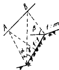
Hình 8 - 20. Xác định đường quỹ tích tâm trượt nguy hiểm trường hợp nền đào vùng núi có taluy 1 : 1 và độ dốc mặt đất trên đỉnh taluy không nằm ngang (kèm bảng 8 - 10).
