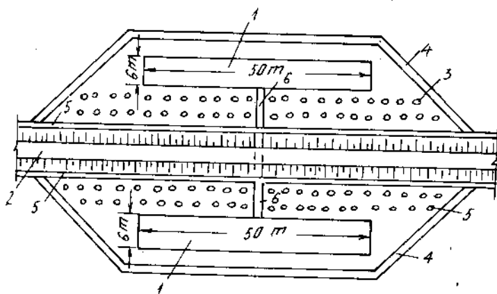
Hình 13 - 18. Sơ đồ cấu tạo bể bốc hơi.
