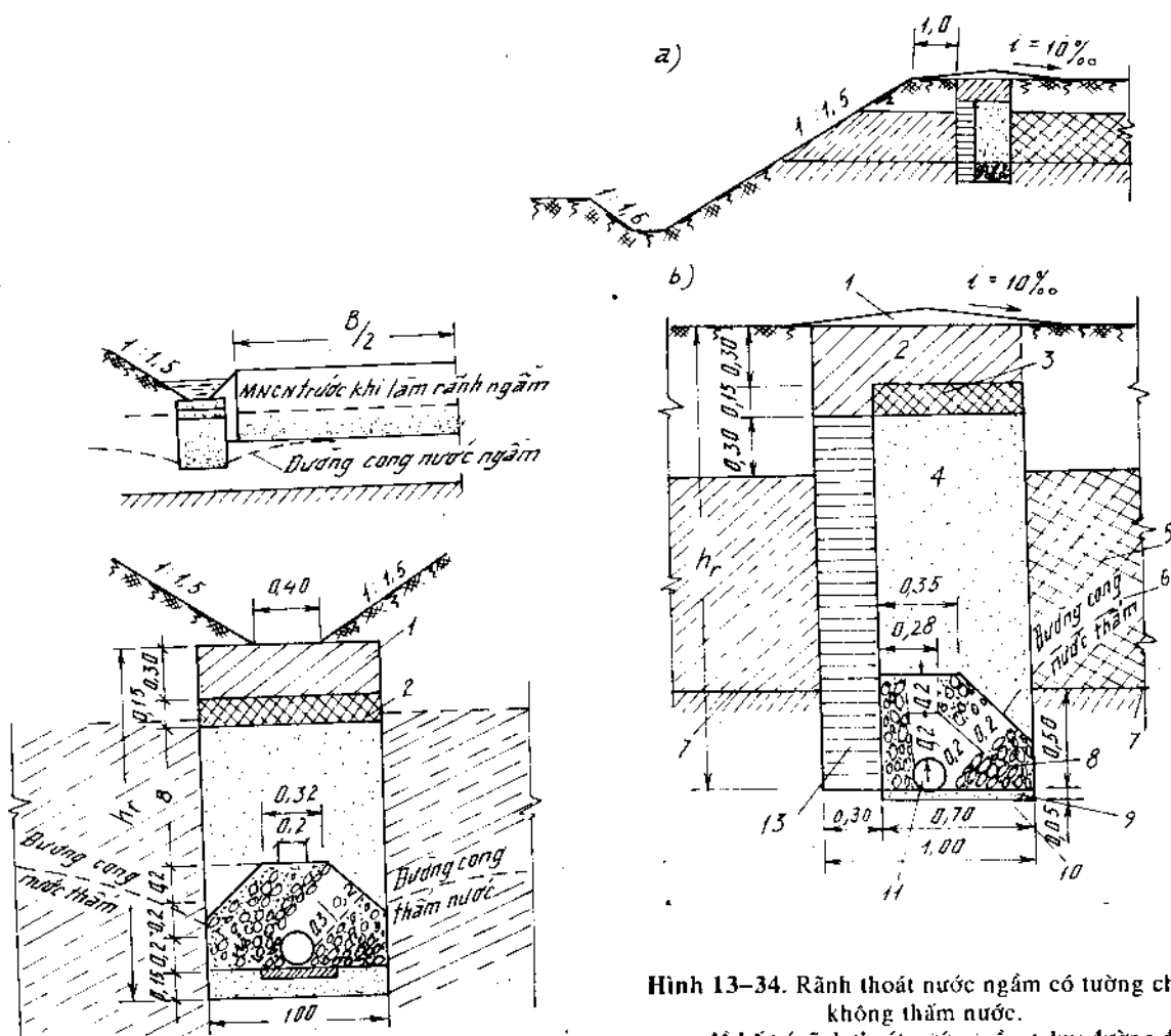
Hình 13-33. Sơ đồ rãnh thoát nước ngầm dưới rãnh dọc.
