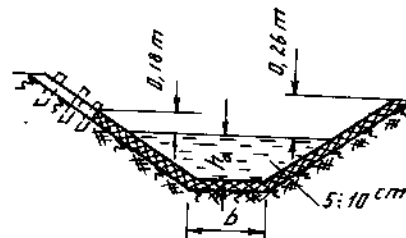
Hình 13 - 6. Gia cố rãnh bằng đất trộn nhựa.
