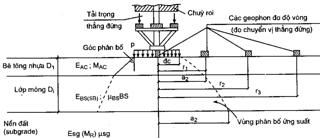
Hình 11 – 23. Đo độ võng và chịu võng bằng các loại thiết bị NDT động (thiết bị FWD) (NDT – No – destructive test) và sơ đồ vùng phân bố ứng suất. (thường r_1 = 0,2 - 0,3 m ; r_2 = 0,5 - 0,7 m ; r_3 = 0,9 - 1,2 m)
