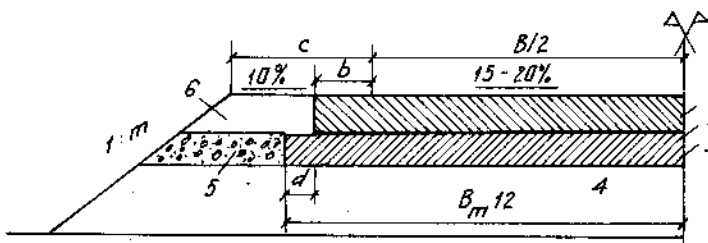
Hình 12 - 1. Cấu tạo kết cấu của áo đường bê tông xi măng đổ tại chỗ.
