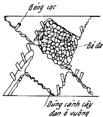
Hình 8-12. Gia cố taluy bằng biện pháp bỏ đá, cuội (dùng cành cây đóng cọc đan thành các ô vuông rồi bỏ đá).
