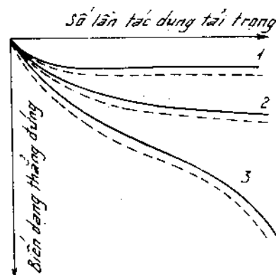
Hình 11 - 4. Quy luật biến dạng của vật liệu hoặc đất nền khi chịu tải trọng trùng phục.
