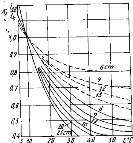
Hình 11 – 20. Đồ thị xác định hệ số quy đổi K_t .
