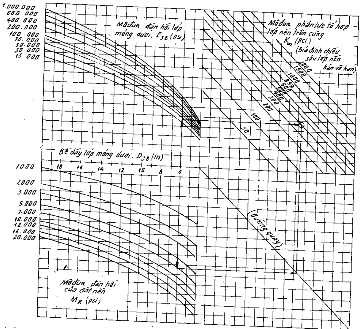
Hình 12 - 15. Đồ thị để tính môđun phản lực nền tổ hợp của móng và nền đất k_{\infty} với giả định bề sâu lớp nền trên cùng bán vô hạn (một chiều, sâu lớn hơn 10f, dưới bề mặt lớp nền trên cùng được coi là chiều sâu bán vô hạn).
