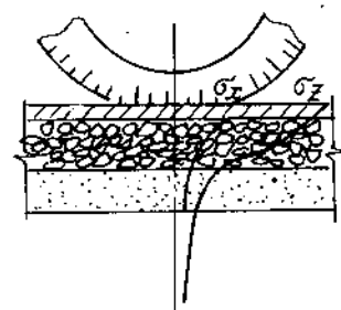
Hình 10 - 1. Sơ đồ phân bố ứng suất trong kết cấu áo đường theo chiều sâu.
