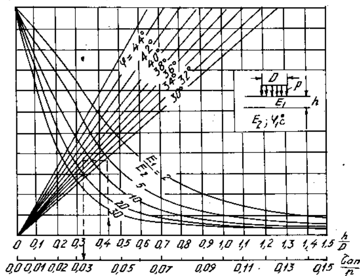
Hình 11 - 12b. Như hình 11 - 12a nhưng tính toán với giả thiết 2 lớp trên và dưới chuyển vị tự do (nghĩa là không có dính kết giữa 2 lớp)
