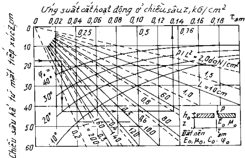
a - Toán đồ xác định ứng suất cắt hoạt động khi các khe không có thiết bị truyền lực (liên kết ngầm)
