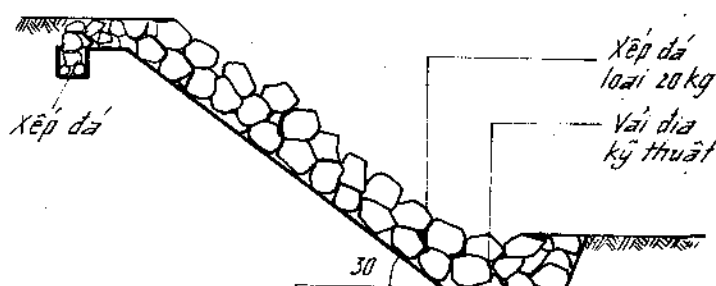
Hình 8-11b. Dùng vải địa kỹ thuật thay cho tầng đệm làm chức năng tầng lọc ngược khi gia cố taluy
