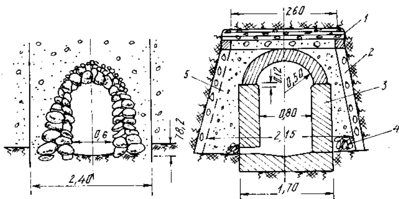
Hình 13-36. Hầm thoát nước bằng đá. 1 – gỗ ; 2 – bê tông ; 3 – xây đá bằng vữa ; 4 – sỏi hay đá dăm ; 5 – cát lớn.
