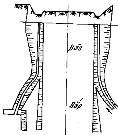
Hình 13 – 9. Thoát nước rãnh dọc từ nền đào ra nền đắp.
