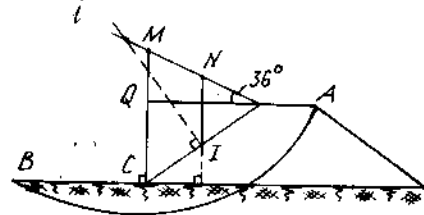
Hình 8 – 29a. Cách mò tìm tâm trượt nguy hiểm nếu nghiệm toán ổn định nền đắp trên đất yếu theo phương pháp mặt trượt tròn.
