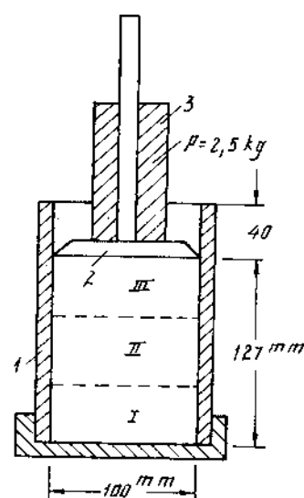
Hình 9 – 11. Cối đầm nén đất tiêu chuẩn (Việt Nam).
