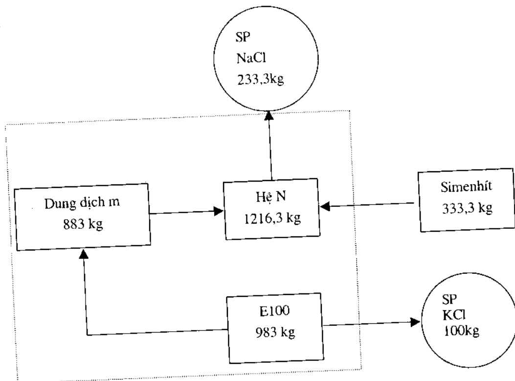
Hình 32: Sơ đồ tuần hoàn sản xuất \text{NaCl} và \text{KCl} từ Simenhít.
