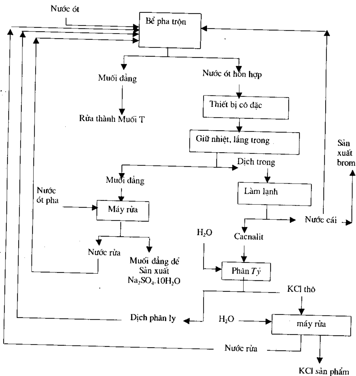
Hình 74: Sản xuất KCl từ nước ớt của muối biển.
