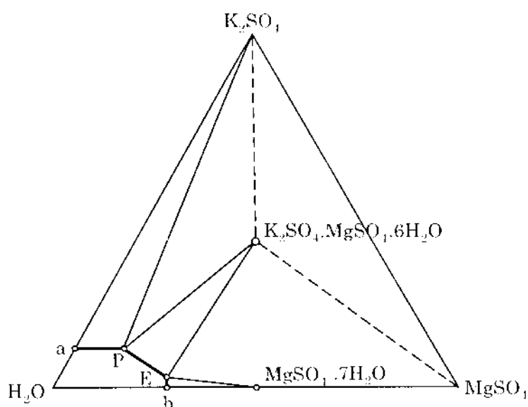
Hình 27: Hệ \text{K}_2\text{SO}_4 - \text{MgSO}_4 - \text{H}_2\text{O} , 25%, % KL.
