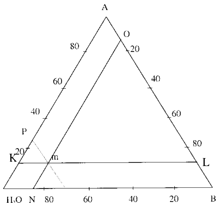
Hình 13: Hệ A - B - H 2 O, %KL.
