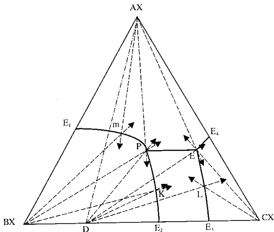
Hình 51: Ứng dụng vectơ kết tinh.
