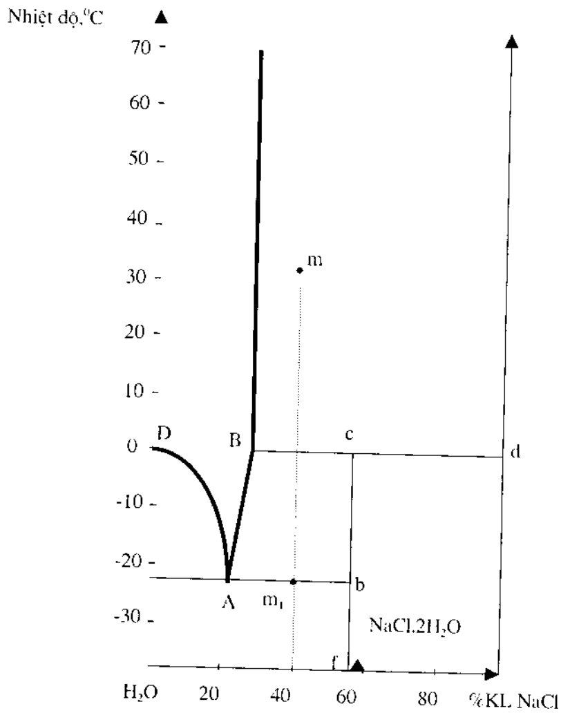
Hình 11: Hệ NaCl - H 2 O.
