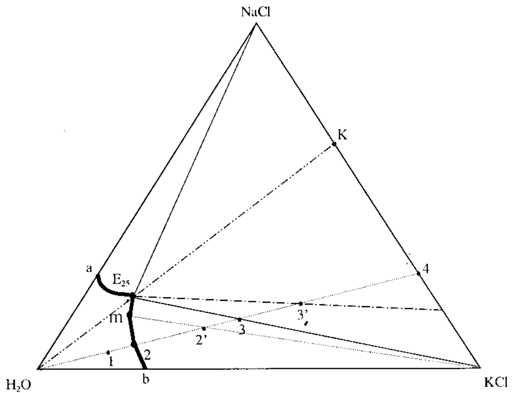
Hình 18: Hệ NaCl, KCl, H 2 O, 25 0 C, %KL.
