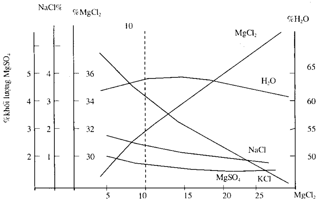
Hình 76: Thành phần bão hòa chung ở 100°C.
