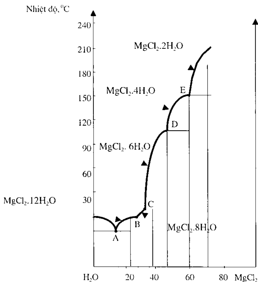
Hình 10: Hệ \text{MgCl}_2 - \text{H}_2\text{O} .
