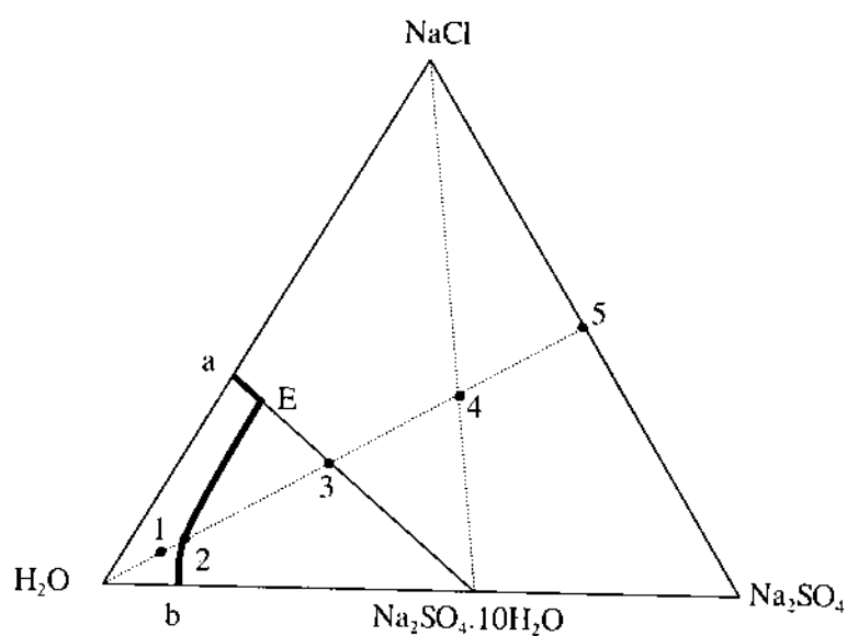
Hình 20: Hệ NaCl - \text{Na}_2\text{SO}_4 - \text{H}_2\text{O} , °C %KL.
