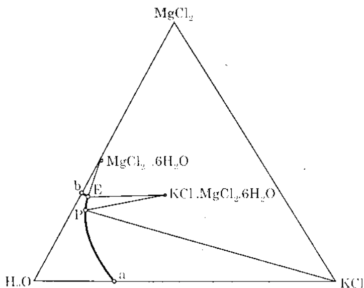
Hình 28: Hệ KCl - \text{MgCl}_2 - \text{H}_2\text{O} , 25°C , %KL
