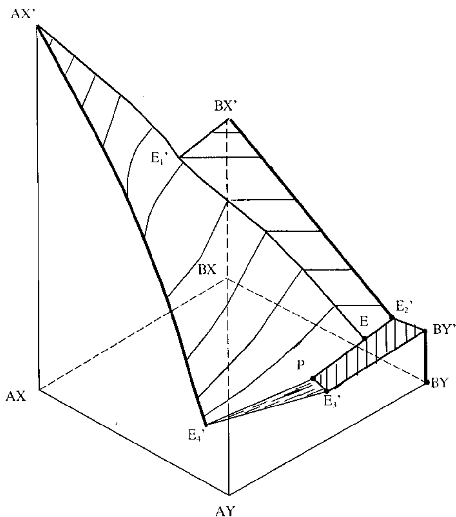
Hình 55: Hệ A^+, B'//X, Y - H_2O, t^\circ C Đồ thị không gian H_2O .
