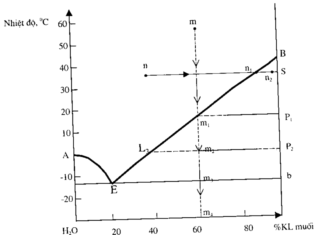
Hình 3: Hệ muối - nước.
