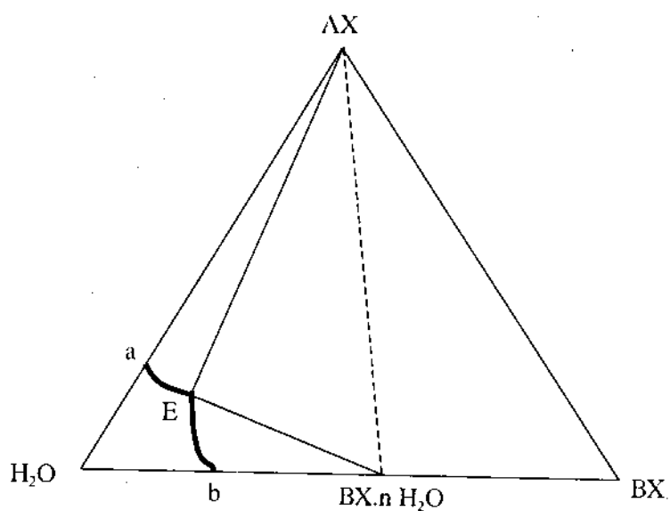
Hình 19: Đồ thị hệ bậc 3 tạo hợp chất hydrat.
