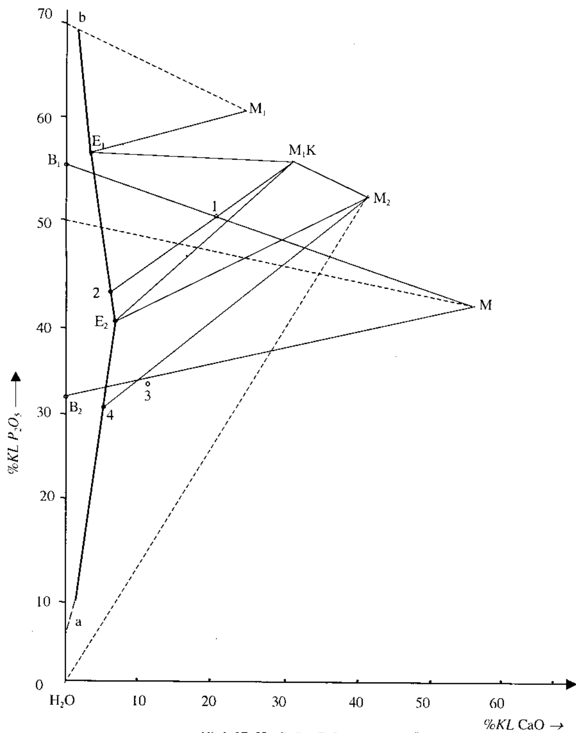
Hình 37: Hệ \text{CaO} - \text{P}_2\text{O}_5 - \text{H}_2\text{O} , 100^\circ\text{C} , % KL.
