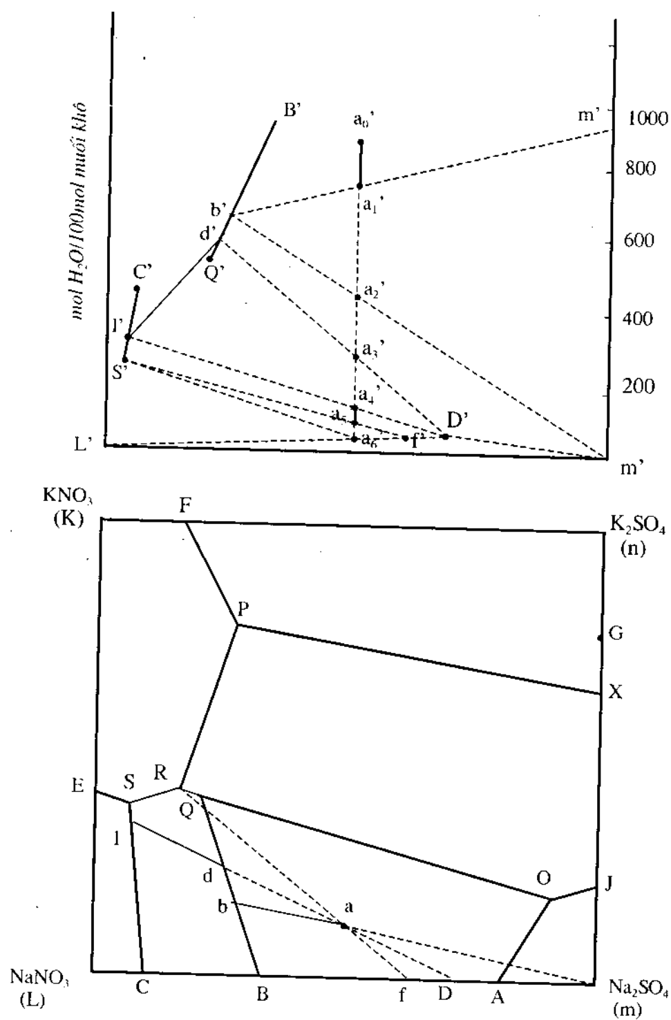
Hình 59: Hệ \text{K}^+ , \text{Na}^+/\text{NO}_3^- , \text{SO}_4^{2-} , \text{H}_2\text{O} , 30^\circ\text{C} . Bốc hơi đẳng nhiệt dung dịch a.
