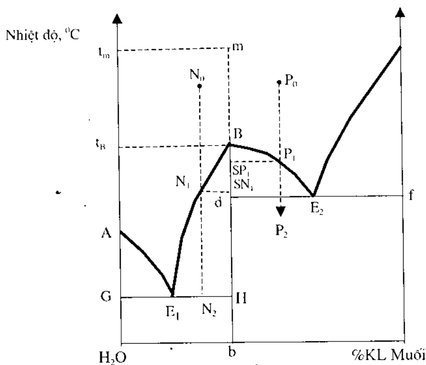
Hình 8: Hệ muối - nước tạo hợp chất hydrat ổn định.
