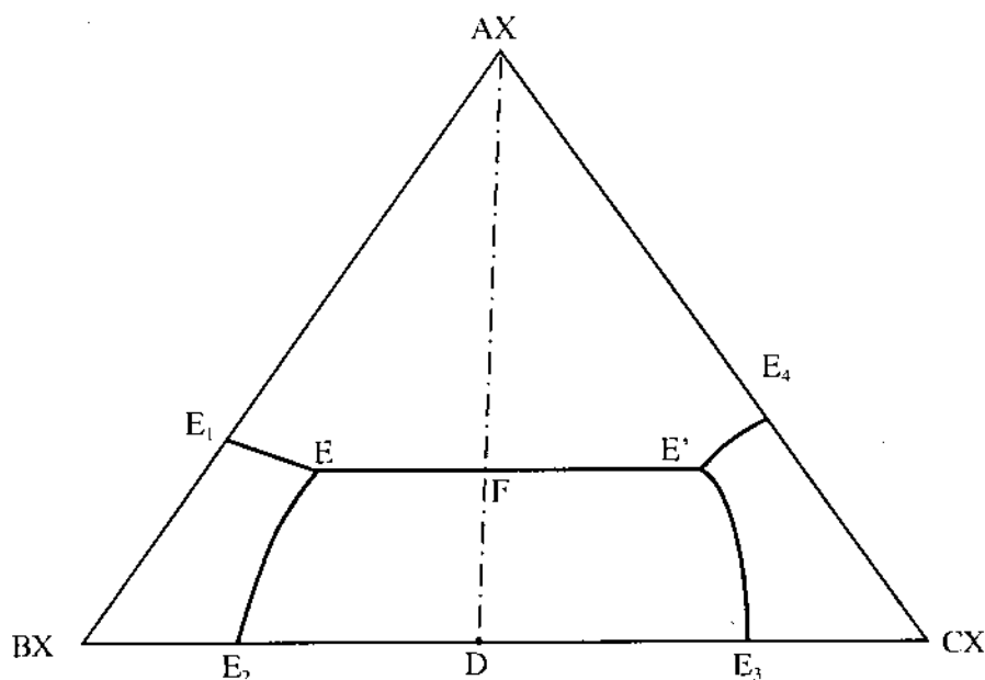
Hình 49: Đồ thị bậc bốn đơn giản tạo muối kép tương hợp.
