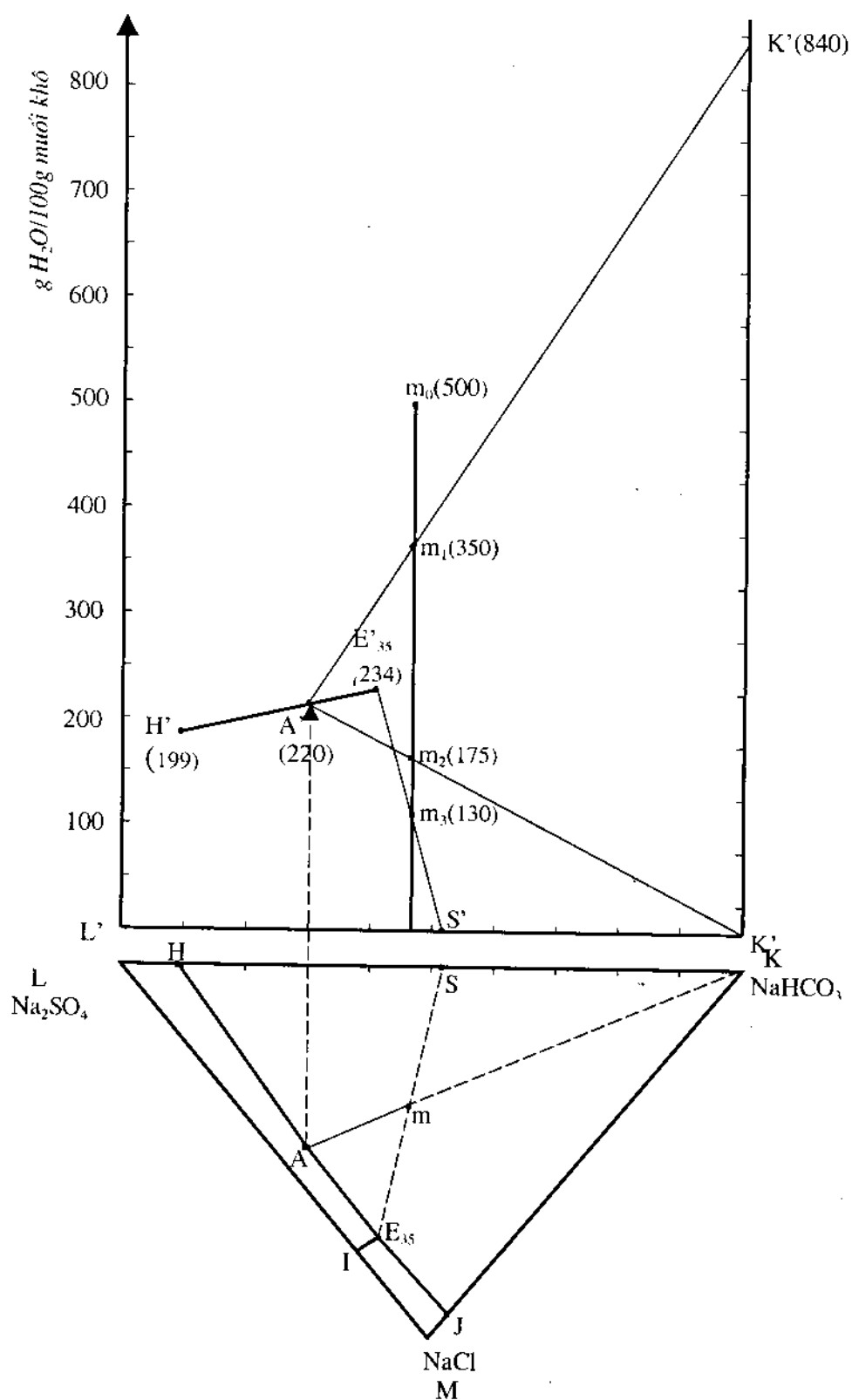
Hình 53: NaCl - Na_2SO_4 - NaHCO_3 - H_2O , 35^\circ C , %KL.
