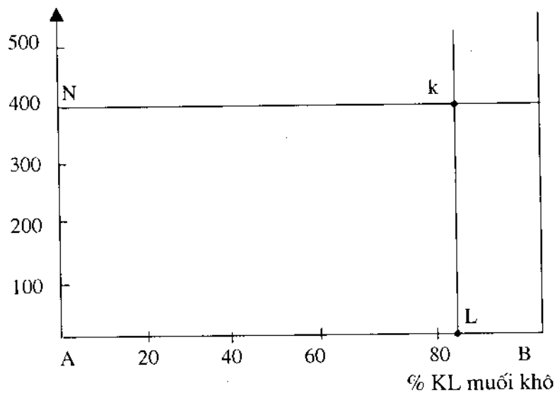
Hình 16: Hệ A - B - H 2 O.
