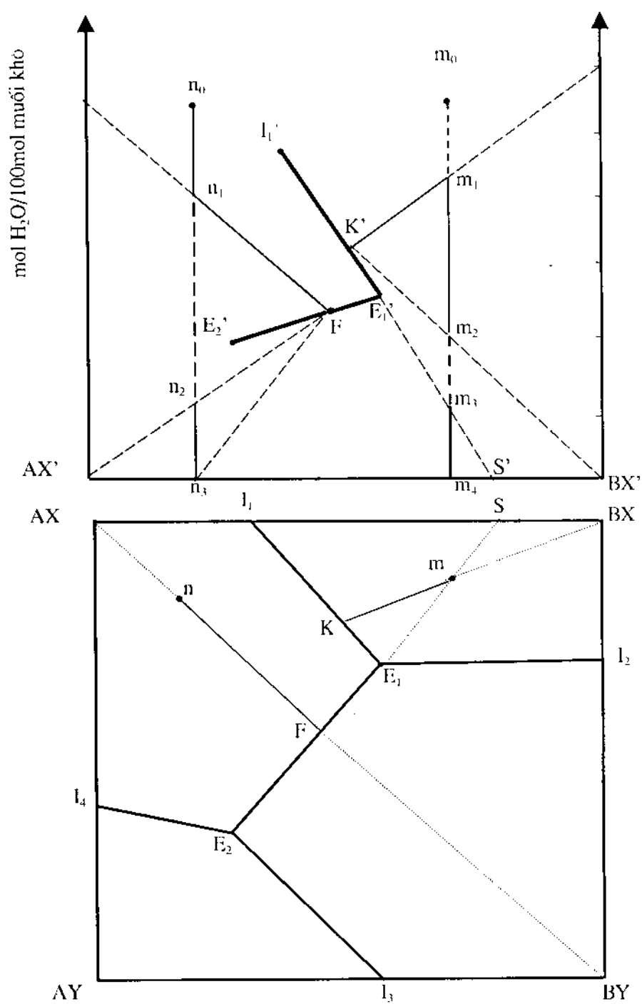
Hình 57: A.B// X.Y- \text{H}_2\text{O} , t^\circ\text{C} Đồ thị khan và đồ thị nước.
