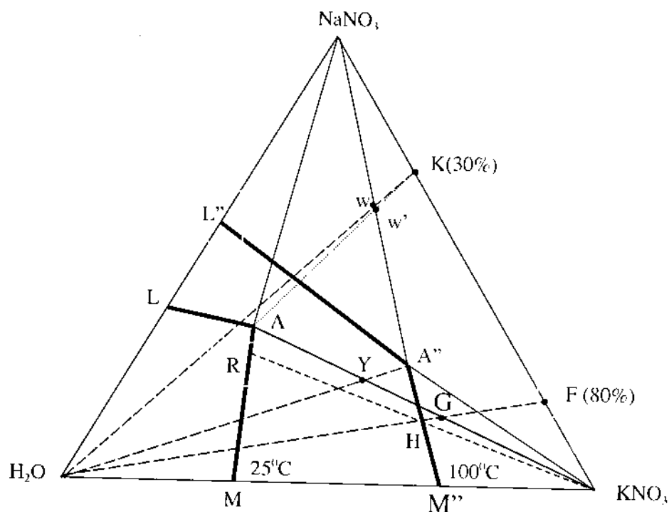
Hình 33: Hệ \text{NaNO}_3 - \text{KNO}_3 , \text{H}_2\text{O} , 25^\circ\text{C} và 100^\circ\text{C} , %KL.
