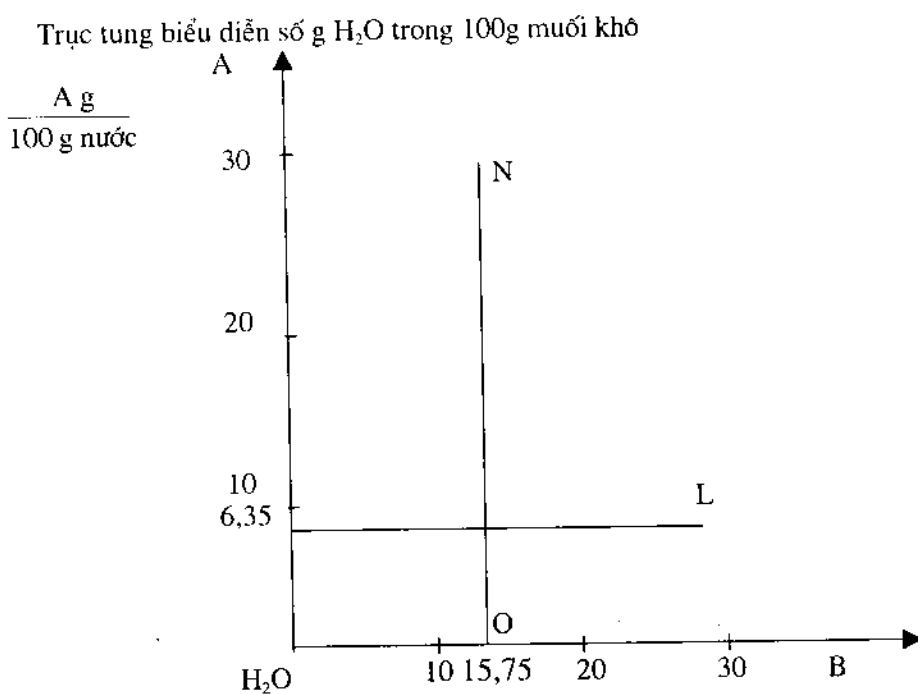
Hình 15: Hệ A - B - H 2 O
