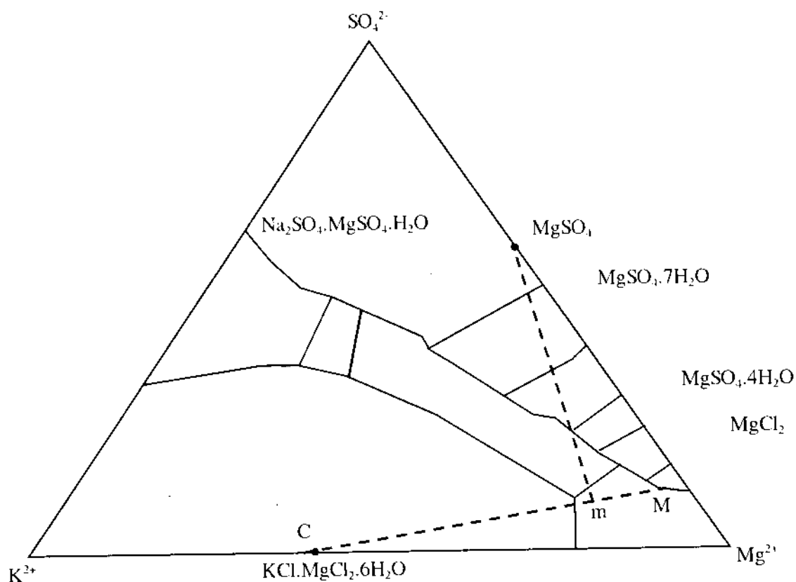
Hình 77: Hệ K_2^{2+} , Mg^{2+} , SO_4^{2-} .
