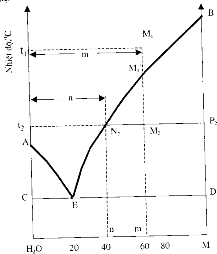
Hình 5: Hệ muối - nước.
