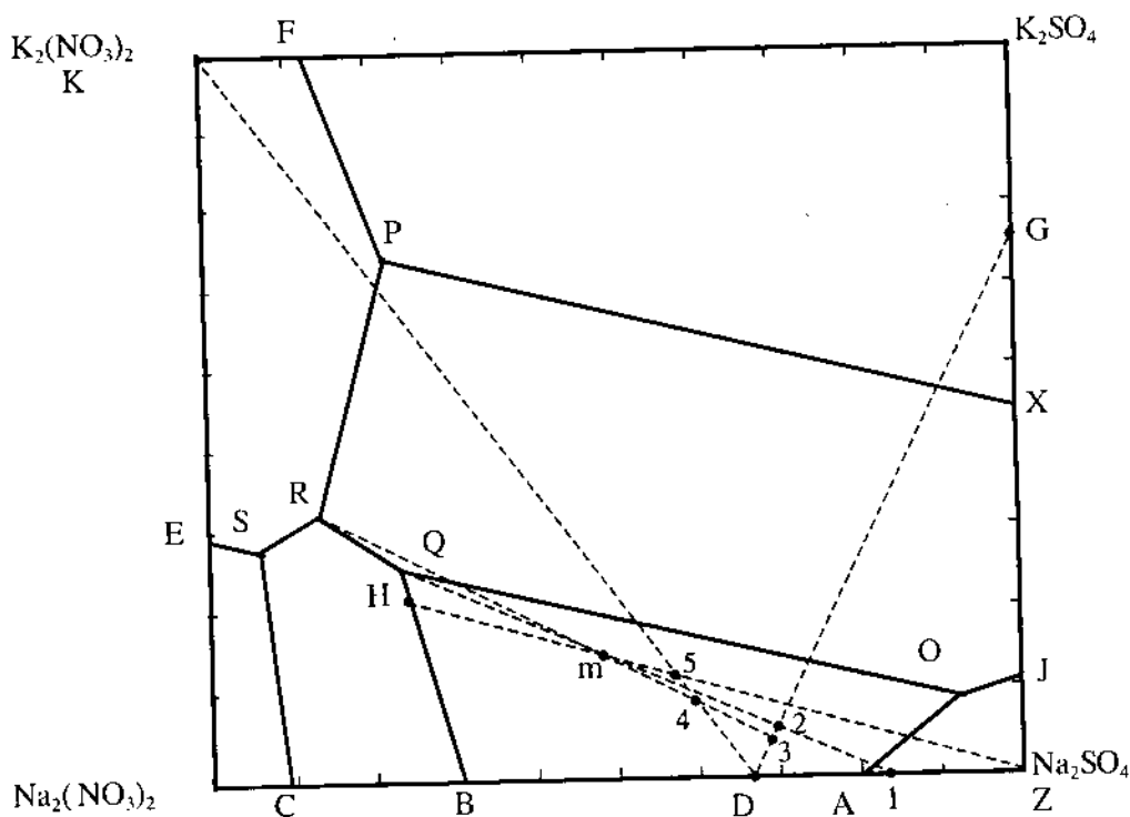
Hình 60: Hệ \text{K}^+ \cdot \text{Na}^+ // \text{NO}_3^-, \text{SO}_4^{2-}, \text{H}_2\text{O}, 30^\circ\text{C} .
