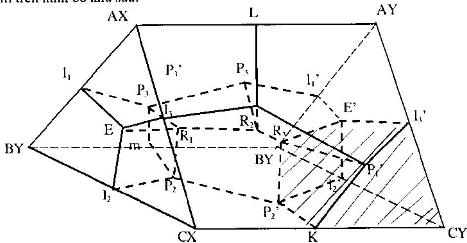
Hình 66: Đồ thị không gian đẳng nhiệt hệ bậc 5 muối - nước tương tác đơn giản nhất.
