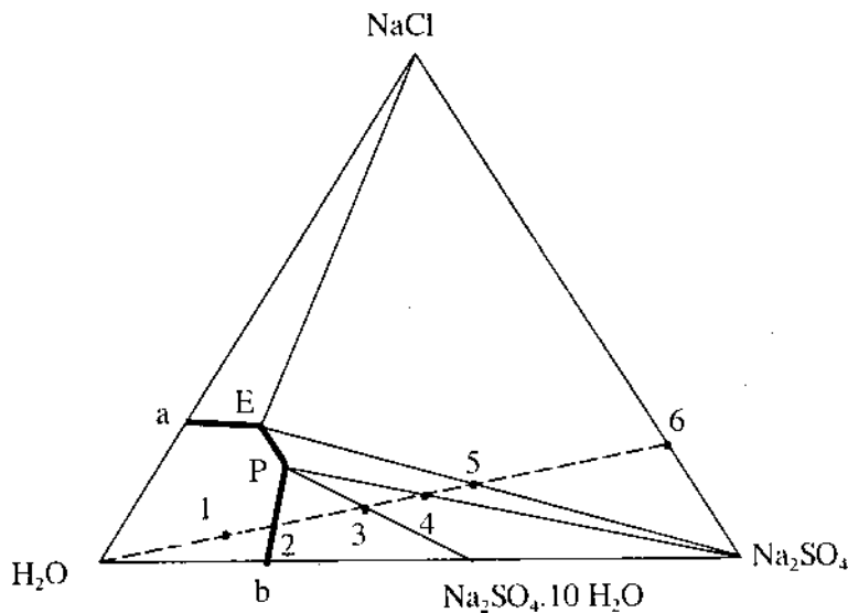
Hình 22: Hệ NaCl - Na 2 SO 4 - H 2 O, 25°C, %KL.
