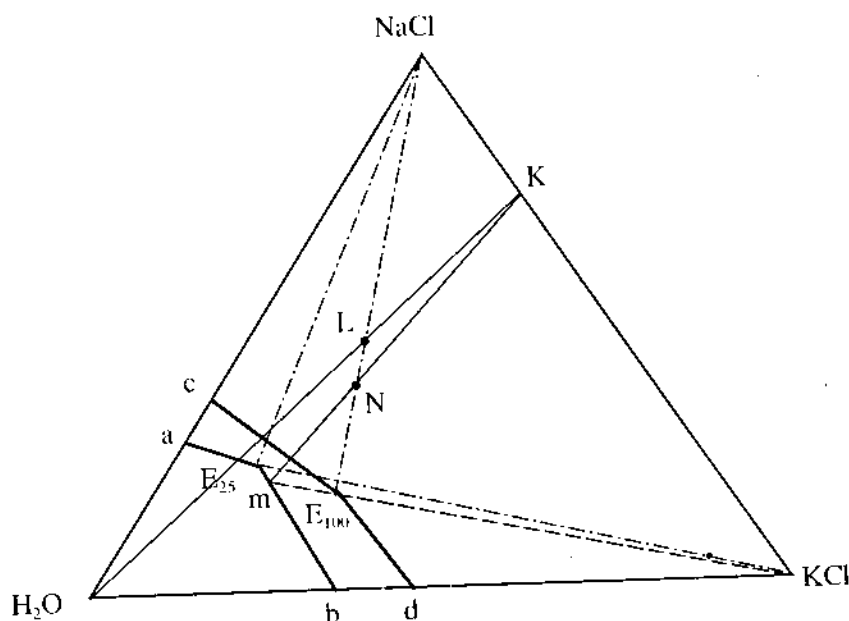
Hình 31: NaCl - KCl - H 2 O, 25 0 C và 100 0 C, %KL.
