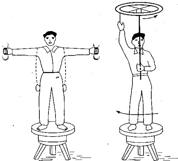
Hình 3-9. Thí nghiệm ghế Giucôpxki
