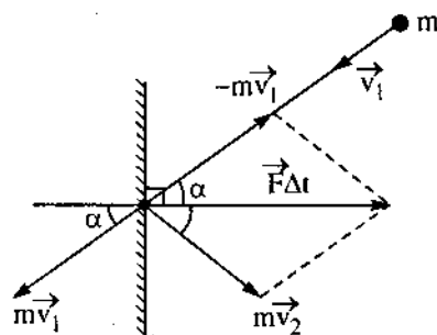
Hình 2-3. Bài toán va chạm vào tường
