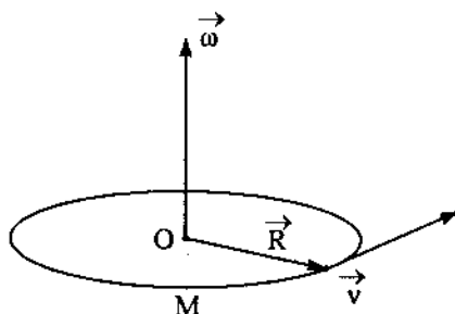
Hình 1-7. Vector vận tốc góc
