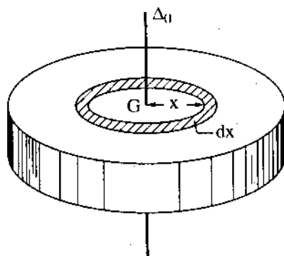
Hình 3-7. Tính mômen quán tính của đĩa
