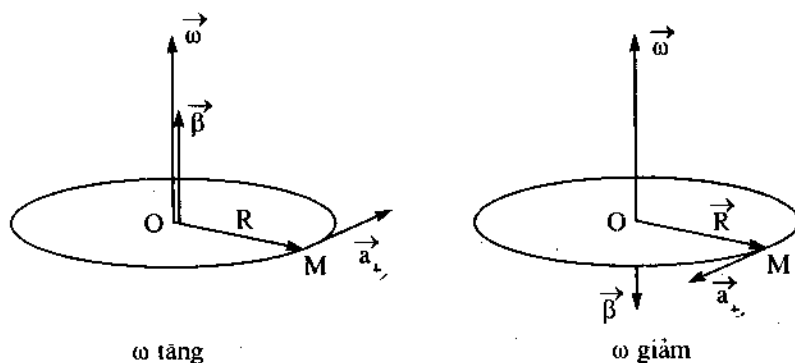
Hình 1-8. Vectơ gia tốc góc
