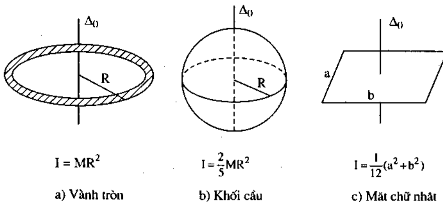
Hình 3-8. Momen quán tính của một số vật rắn
