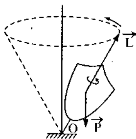
Hình 3-12. Chuyển động tuế sai
