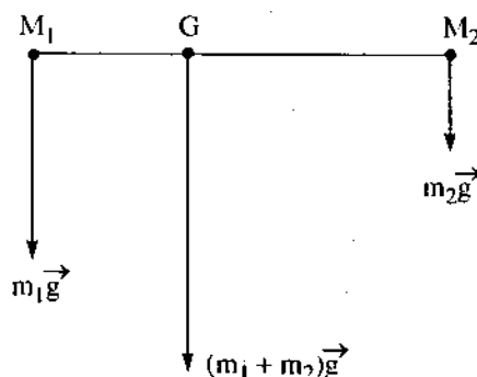
Hình 3-1. Khối tâm
