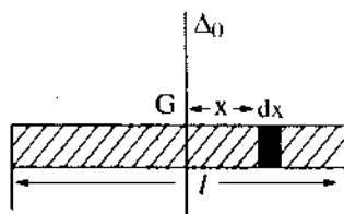
Hình 3-6. Tính mômen quán tính của thanh
