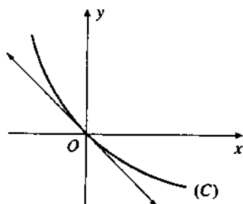
Dáng điệu của (C) trong lân cận của (0, 0)
