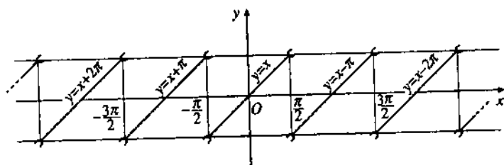
Biểu diễn đồ thị của \text{Arctan} \circ \tan
