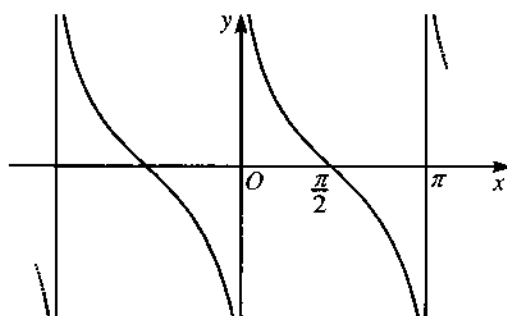
Biểu diễn đồ thị của hàm cotan
