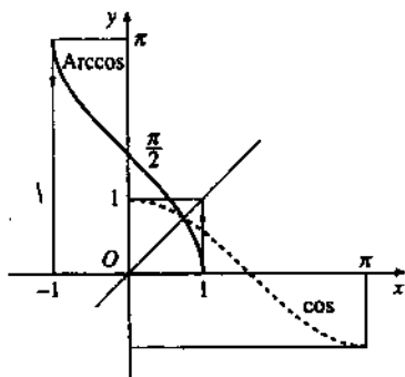
Biểu diễn đồ thị của hàm \text{Arccos}
