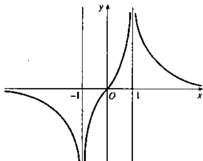
Biểu diễn đồ thị của f
