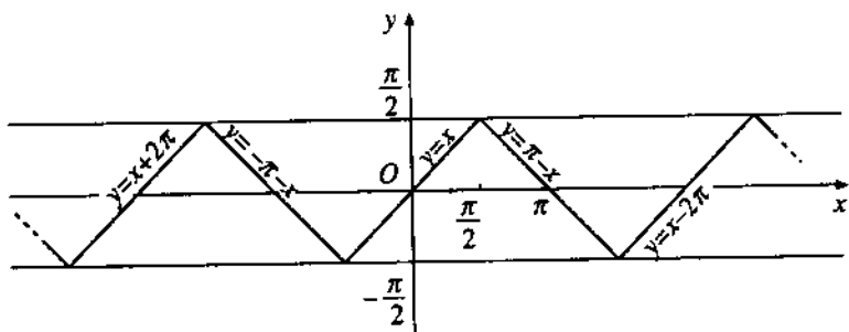
Biểu diễn đồ thị của \text{Arcsin} \circ \sin
