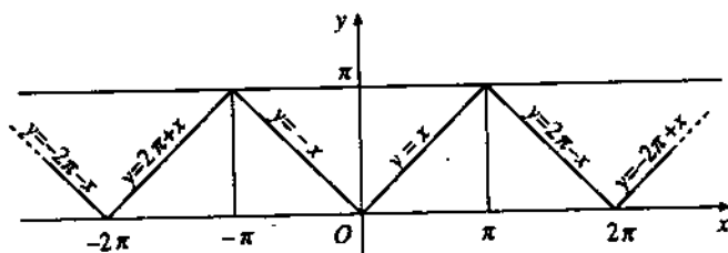
Biểu diễn đồ thị của \text{Arccos} \circ \cos
