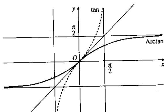
Biểu diễn đồ thị của hàm Arctan
