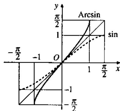
Biểu diễn đồ thị của hàm \text{Arcsin}
