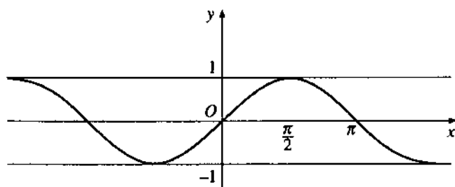
Biểu diễn đồ thị của hàm sin
