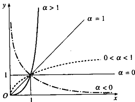
Biểu diễn đồ thị hàm số x \mapsto x^\alpha
