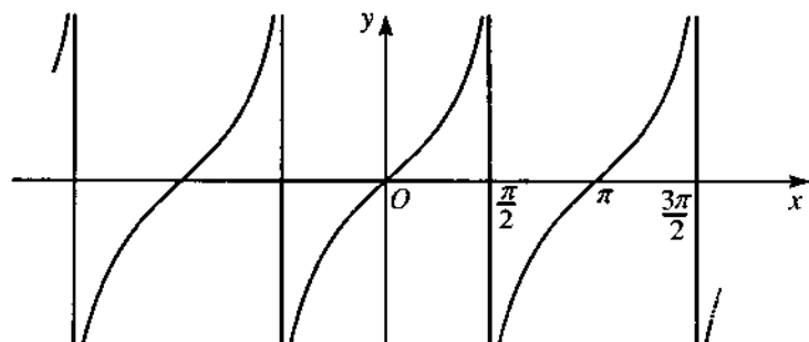
Biểu diễn đồ thị của hàm tan
