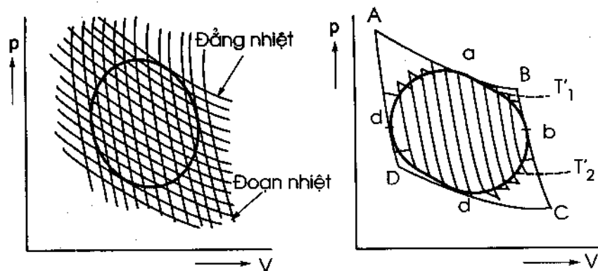
Hình IV - 3. Sự chia một chu trình bất kì abceda thành một số lớn chu trình Cacno nhỏ
