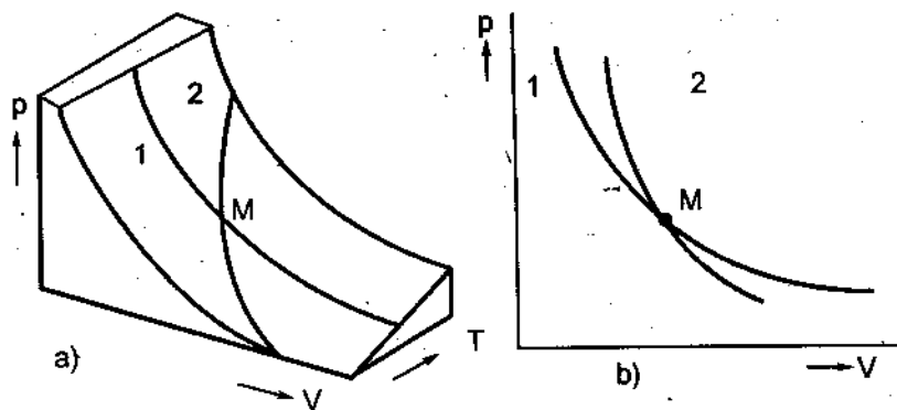
Hình 1-3. So sánh đường đẳng nhiệt (1) và đoạn nhiệt (2) của khí lí tưởng :
