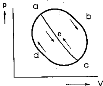
Hình IV - 2. Sự chia một chu trình bất kì thành hai chu trình con.
