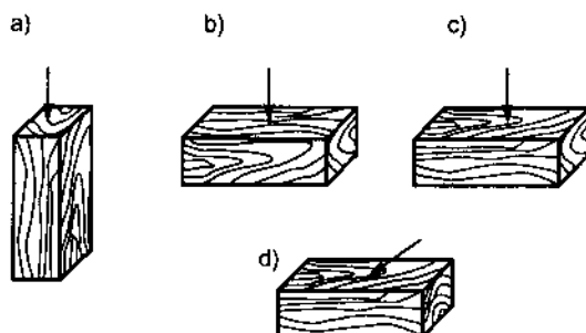
Hình 10.6. Các dạng chịu nén của gỗ
