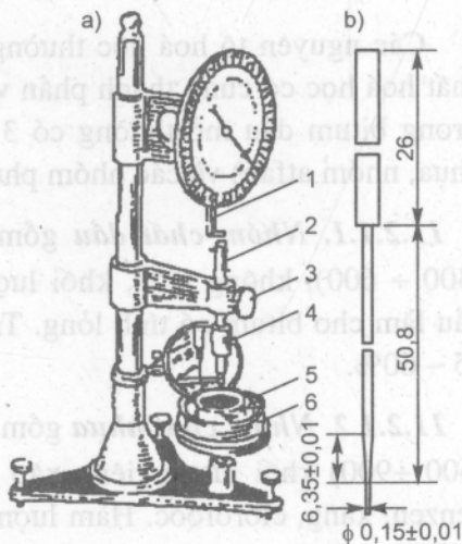
Hình 11.1. Dụng cụ đo độ quánh
