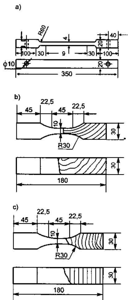
Hình 10.7. Mẫu thí nghiệm kéo
