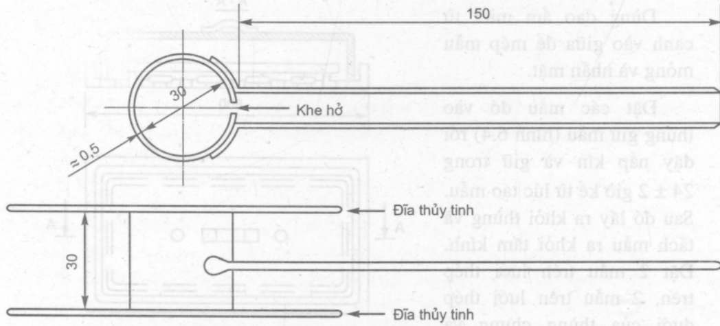
Hình 6.8. Khuôn Losatolie
