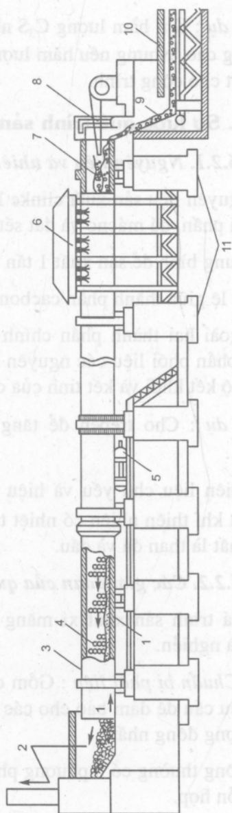
Hình 6.2. Sơ đồ lò quay
