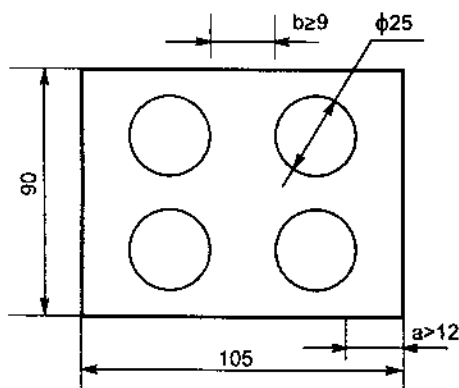
Gạch rỗng 4 lỗ tròn 220 x 105 x 90 mm
