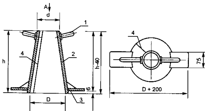
Hình 7.4. Khuôn nón cụt
