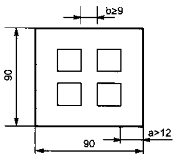
Gạch rỗng 4 lỗ vuông 190 x 90 x 90 mm
