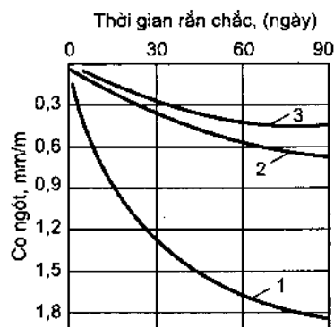
Hình 7.10. Độ co ngót
