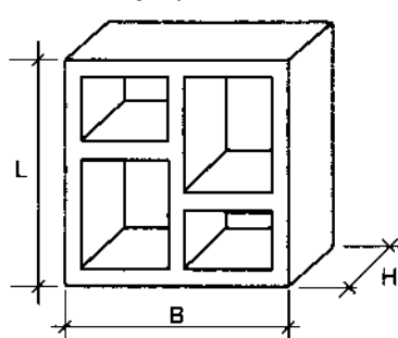
Gạch tứ kết ký hiệu 08
