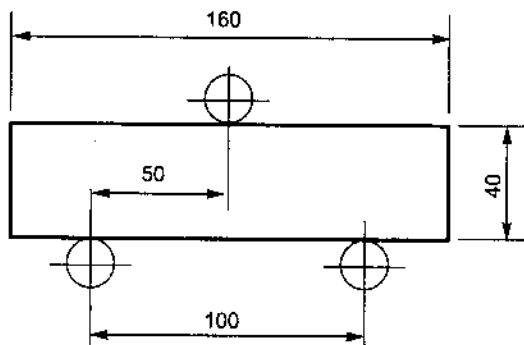
Hình 6.9. Sơ đồ uốn mẫu
