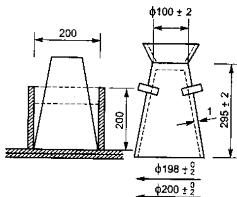
Hình 7.6. Dụng cụ xác định độ cứng của hỗn hợp bê tông
