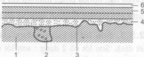
Hình 12.1. Sơ đồ sơn
