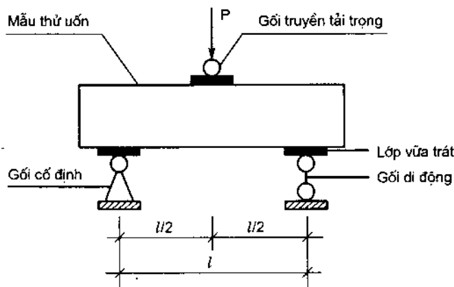
Hình 3.3. Sơ đồ uốn mẫu gạch
