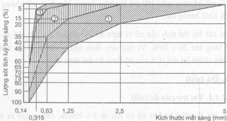
Hình 7.2. Biểu đồ xác định nhóm cát
