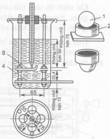
Hình 11.3. Dụng cụ vòng và hòn bi
