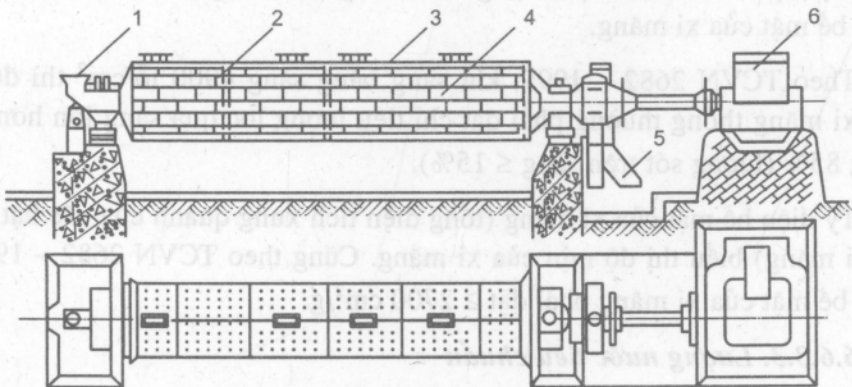
Hình 6.3. Máy nghiền clinke nhiều buồng
