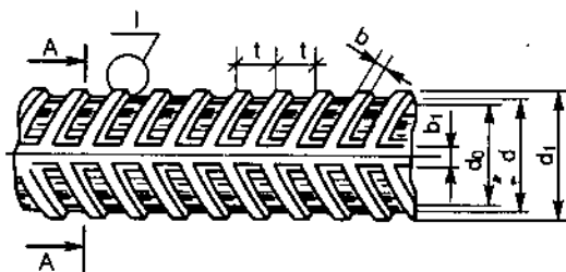
Hình 5.2. Thép cốt nhóm CIII
