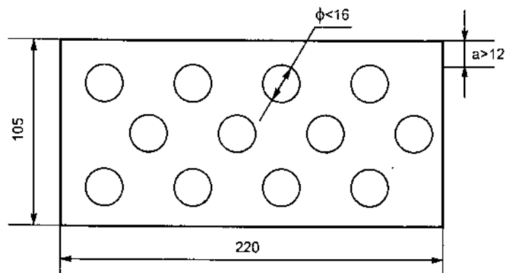
Gạch rỗng 12 lỗ tròn 220 x 105 x 60 mm
