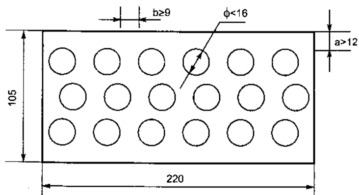
Gạch rỗng 18 lỗ tròn 220 x 105 x 60 mm
