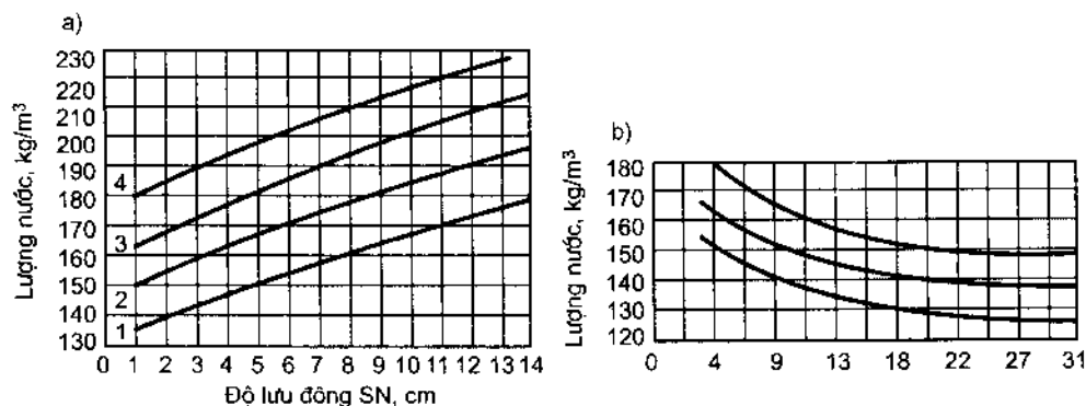
Hình 7.7. Lượng nước dùng cho 1m 3 hỗn hợp bê tông dùng xi măng pooc lăng, cát trung bình N_{yc} = 7\% và sỏi với D_{max} .
