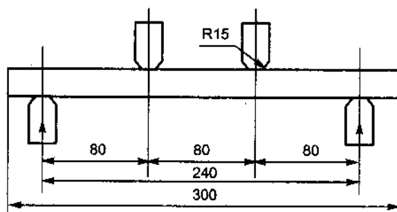
Hình 10.8. Sơ đồ mẫu thí nghiệm uốn
