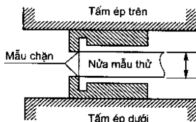
Hình 6.10. Sơ đồ nén mẫu
