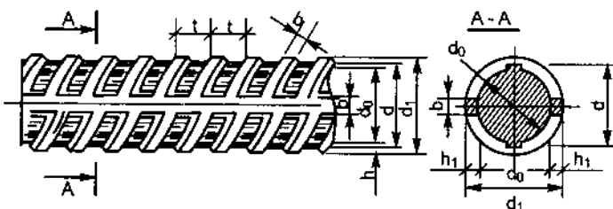
Hình 5.1. Thép cốt nhóm CII
