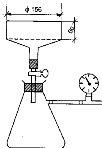
Hình 8.3. Dụng cụ thử khả năng giữ nước
