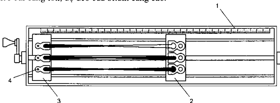
Hình 11.2. Dụng cụ đo độ kéo dài
