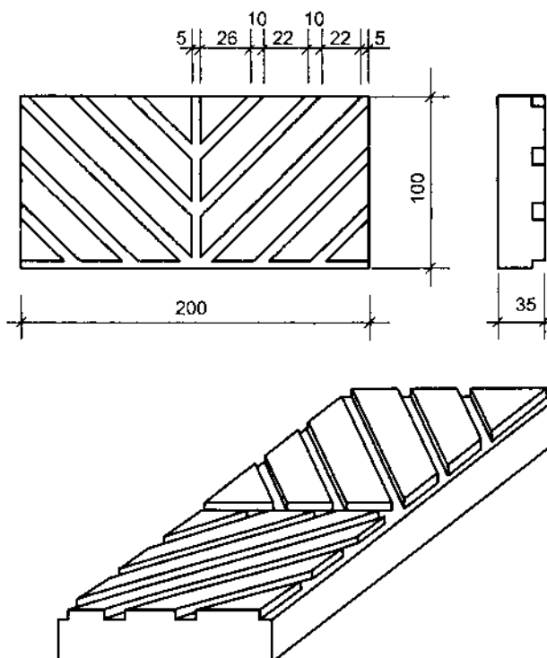
Hình 3.4. Gạch lá dừa
