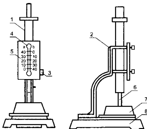
Hình 6.1. Dụng cụ vi ka
