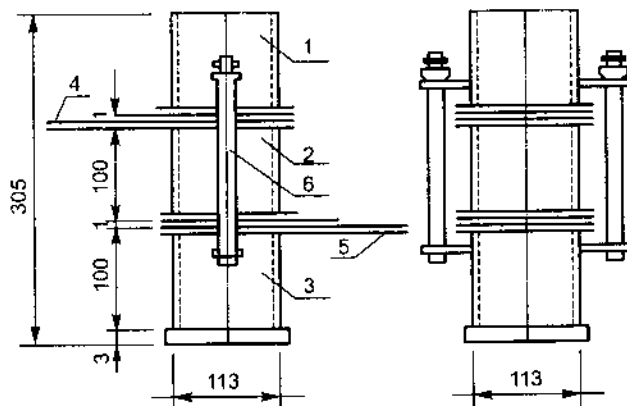
Hình 8.2. Dụng cụ thử độ phân tầng
