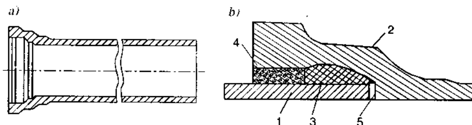
Hình 4-13. Các loại ống gang 1. Đầu tròn ; 2. Đầu loe ; 3. Sợi gai tẩm bitum ; 4. Vữa xi măng amiăng ; 5. Khe hở
