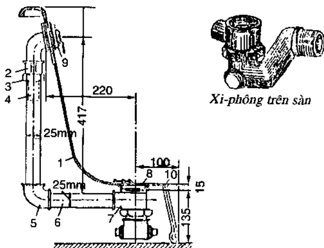
Hình 6.15. Xi-phông thu nước bồn ở chậu tắm
