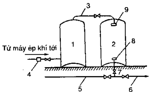
Hình 4.24. Trám khí ép
