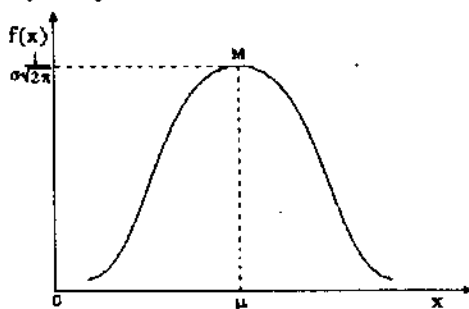
Hình 5.2 Đồ thị của phân phối chuẩn:
