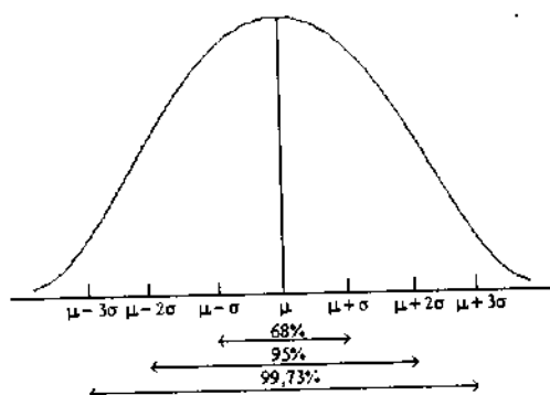
Hình 4.2 Phân phối các lượng biến trong phân phối chuẩn
