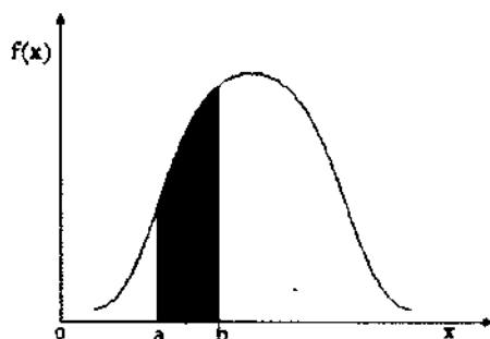
Hình 5.1 xác suất để X nhận giá trị trong đoạn [a, b]
