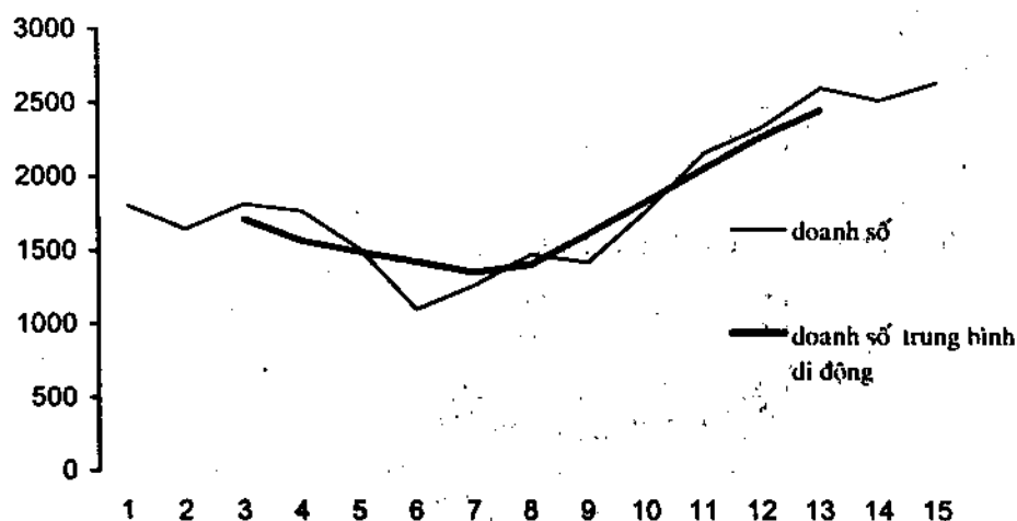
Hình 12.1: đồ thị biến động của doanh số thực tế và doanh số trung bình di động.
