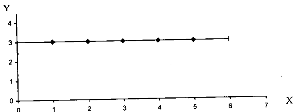
Hình 11.4: Y không đổi với mọi giá trị của X
