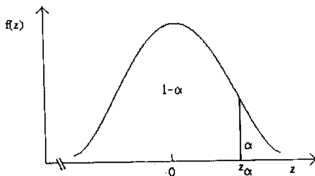
Hình 6.3 Ước lượng bên phải
