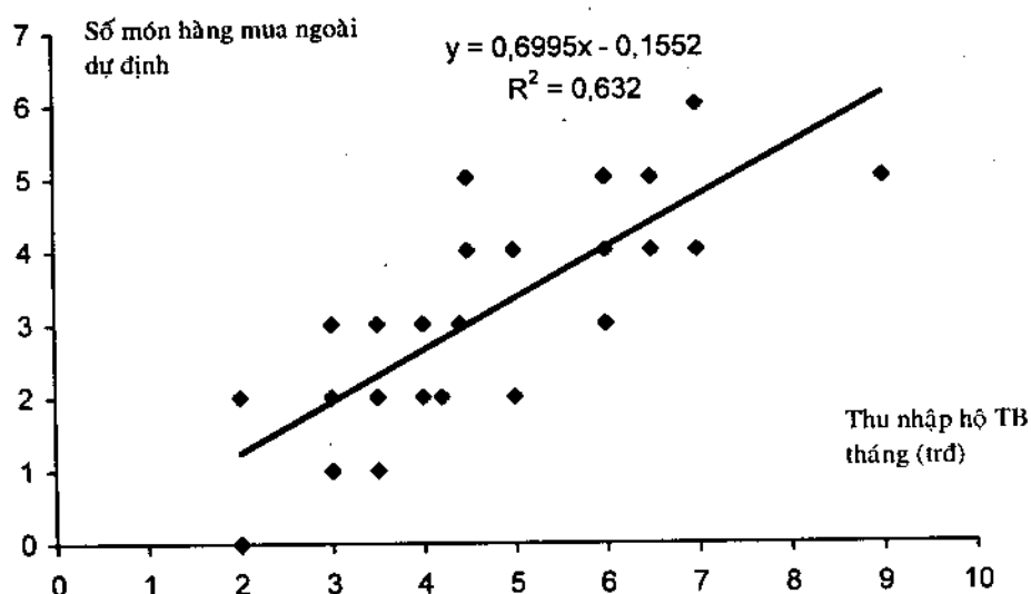
Hình 11.2: Đồ thị hồi qui tuyến tính
