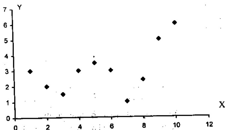
Hình 11.5: X và Y không có liên hệ tuyến tính
