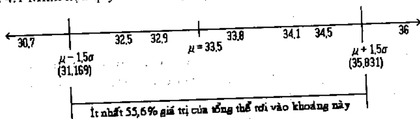
Hình 4.1 Minh họa quy tắc Tchebychev
