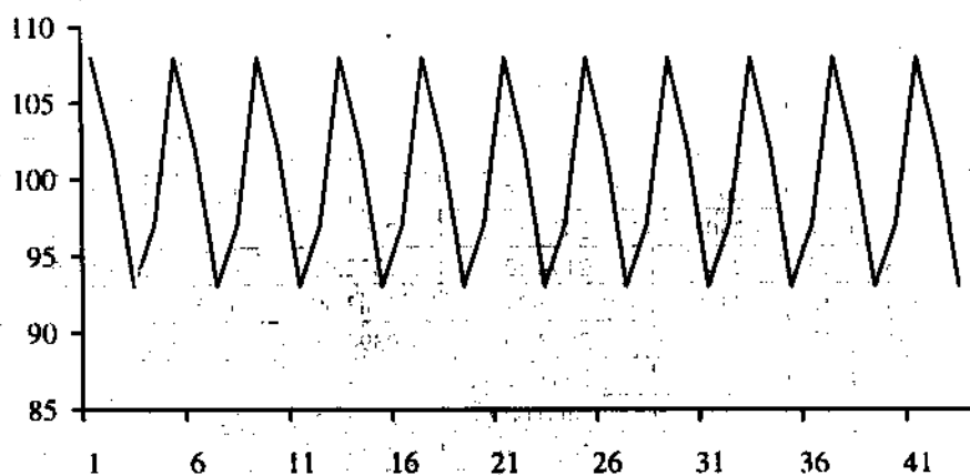
Hình 12.6: chỉ số thời vụ
