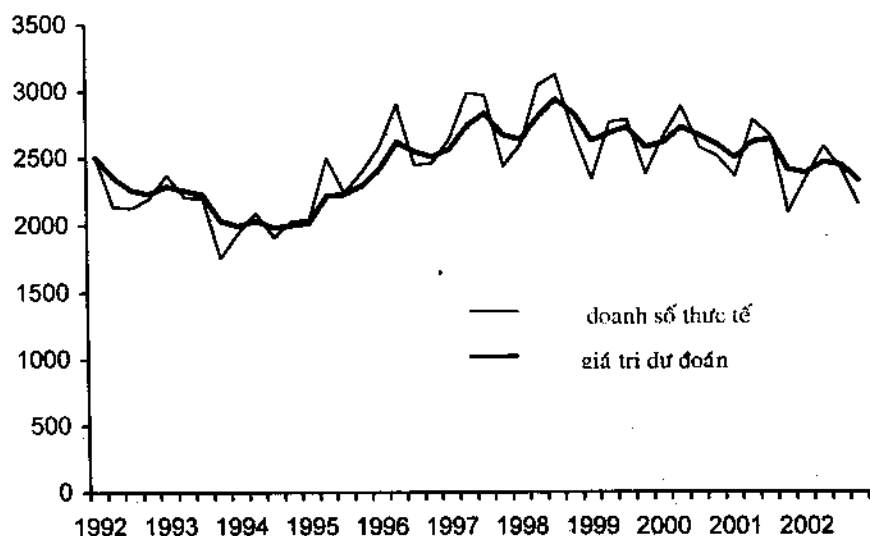
Hình 12.10: Sản lượng bán thực tế và giá trị dự đoán với w tối ưu = 0,3417
