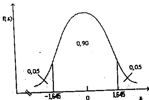
Hình 6.2 P(-1,645 < Z < 1,645) = 0,9 với Z là biến ngẫu nhiên có phân phối chuẩn.
