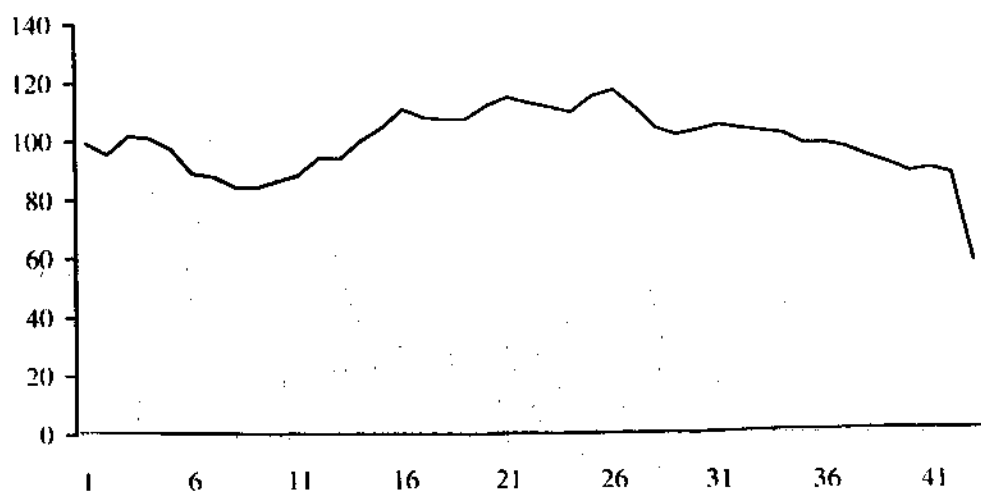
Hình 12.7: Chỉ số chu kỳ.
