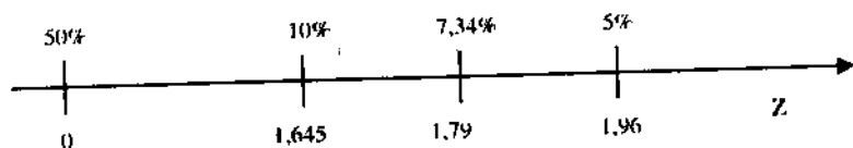
Hình 8.1 Miền chấp nhận, miền bác bỏ theo p -value
