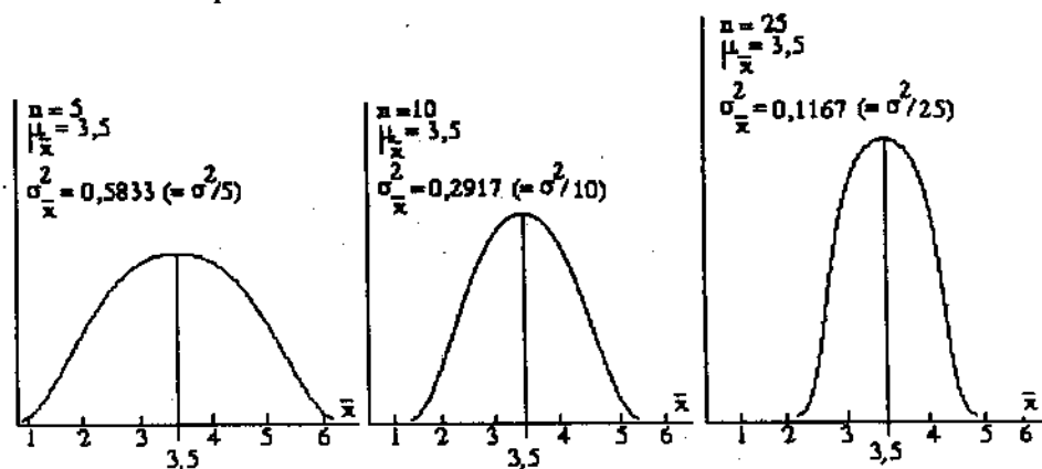
Hình 5.5 Phân phối mẫu của \bar{X} khi n = 5, 10 và 25 .
