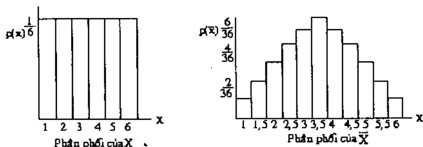
Hình 5.4 Phân phối của X và \bar{X}
