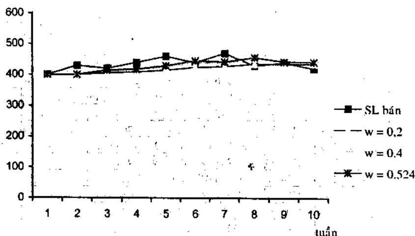
Hình 12.9: số lượng sản phẩm bán thực tế và giá trị dự đoán với w = 0,2 , w = 0,4 và w = 0,524
