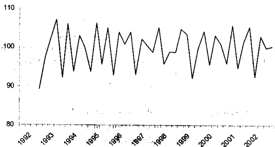
Hình 12.8: Chỉ số biến động ngẫu nhiên
