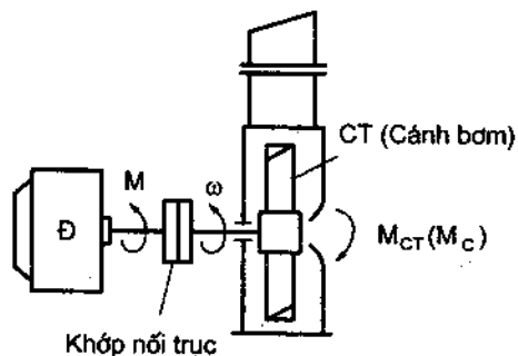
Hình 1 -1. Truyền động của máy bơm nước
