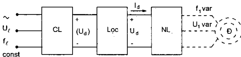
Hình 3 - 20. Sơ đồ khối của bộ biến tần có khâu trung gian một chiều
