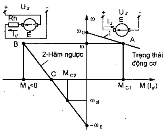
Hình 2 - 10. Hãm ngược khi đảo cực tính điện áp nguồn U_r
