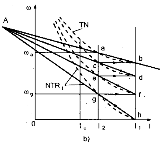
Hình 3 - 7. Sơ đồ nguyên lý (a) và các đặc tính khởi động (b) của động cơ một chiều kích từ nối tiếp
