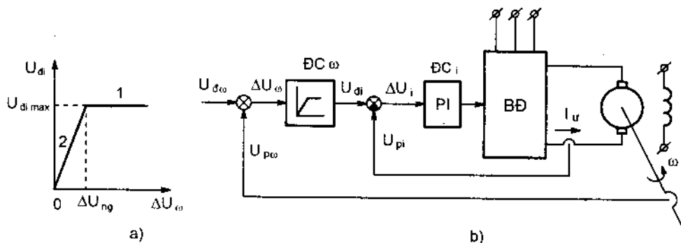
Hình 3 - 33. Nguyên tắc hạn chế dòng điện và momen nhờ khâu hạn chế ở đầu vào
