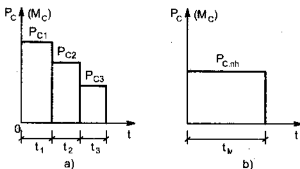
Hình 6 - 6. Quy đổi đồ thị phụ tải biến đổi về dạng không đổi
