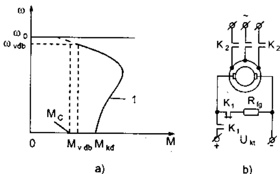
Hình 3 - 27. a) Đặc tính khởi động của động cơ đồng bộ; b) Sơ đồ nối dây để khởi động hai giai đoạn
