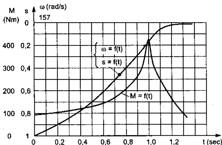
Hình 5 - 5. Đặc tính quá độ \omega = f(t) khi khởi động trực tiếp (không tải) động cơ 28kw 1460v/gi/ph
