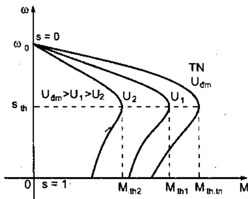
Hình 2 - 28. Họ đặc tính cơ nhân tạo khi thay đổi điện áp stato của động cơ không đồng bộ
