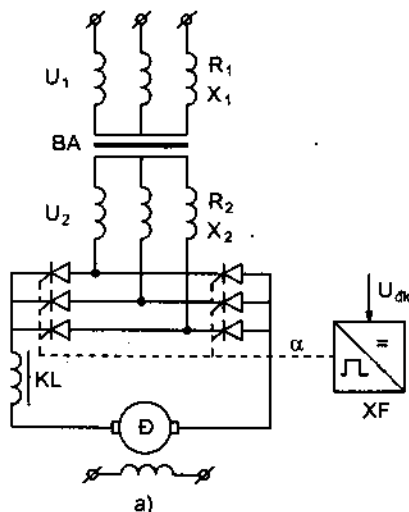
Hình 4 - 7. Sơ đồ nguyên lý và sơ đồ thay thế của hệ CL - Đ trong ví dụ 4-1
