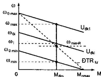
Hình 3-11. Các đặc tính cơ điều chỉnh khi điều khiển động cơ một chiều bằng điện áp phản ứng
