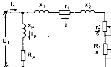
Hình 2 - 23. Sơ đồ thay thế một pha của động cơ không đồng bộ
