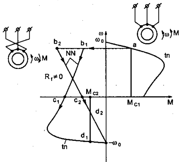
Hình 2 - 34. Hãm ngược bằng cách đảo thứ tự pha điện áp stato : dùng cho động cơ lồng sóc (đoạn b_1c_1 ) và động cơ roto dây quấn có R_1 \neq 0 (đoạn b_2c_2 )
