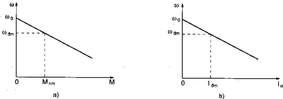
Hình 2 - 3. a) Đặc tính cơ tự nhiên của động cơ điện một chiều kích từ độc lập ; b) Đặc tính cơ điện tự nhiên của động cơ điện một chiều kích từ độc lập.
