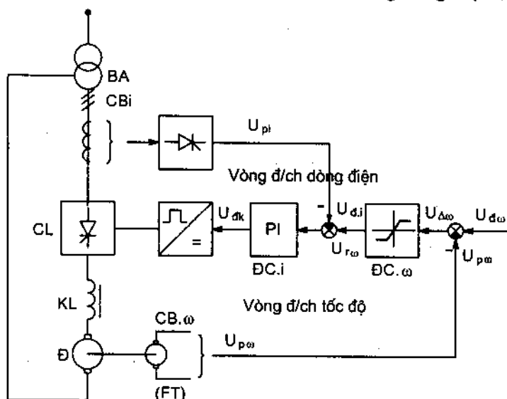
Hình 4 - 13b. Sơ đồ nguyên lý hệ CL - Đ tự động có điều chỉnh độc lập các toạ độ kiểu nối tiếp
