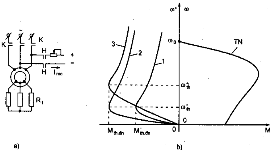
Hình 2 - 35. Hãm động năng động cơ không đồng bộ. a) Sơ đồ nguyên lý ; b) Đặc tính cơ - đường 1 và 2 : có cùng điện trở R_2 nhưng khác nhau về dòng I_1 ; đường 2 và 3 : có cùng giá trị I_1 nhưng khác nhau về điện trở R_2
