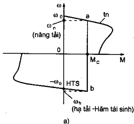
Hình 2 - 32. Các đặc tính cơ của động cơ không đồng bộ khi hãm tái sinh
