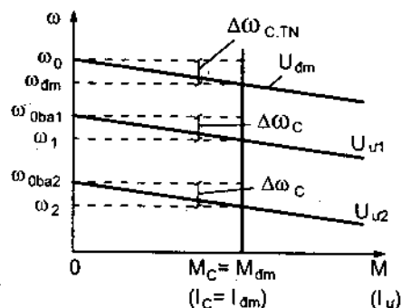
Hình 2-5. Họ đặc tính nhân tạo khi thay đổi điện áp phản ứng
