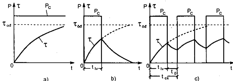
Hình 6 - 4. Đồ thị phụ tải và đường cong nhiệt sai ở các chế độ làm việc của động cơ a) Dài hạn ; b) Ngắn hạn ; c) Ngắn hạn lặp lại
