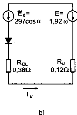
Hình 4 - 7. Sơ đồ nguyên lý và sơ đồ thay thế của hệ CL - Đ trong ví dụ 4-1
