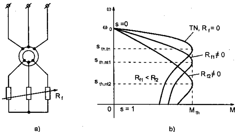
Hình 2 - 27. Sơ đồ nối dây (a) và họ đặc tính cơ nhân tạo khi thay đổi điện trở mạch roto(b) của động cơ không đồng bộ
