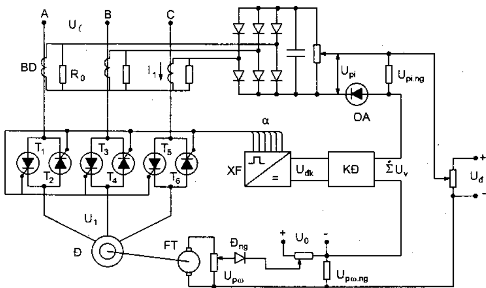
Hình 4 - 24. Sơ đồ nguyên lý của một hệ "Bộ điều chỉnh pha tiristo - Động cơ" tự động
