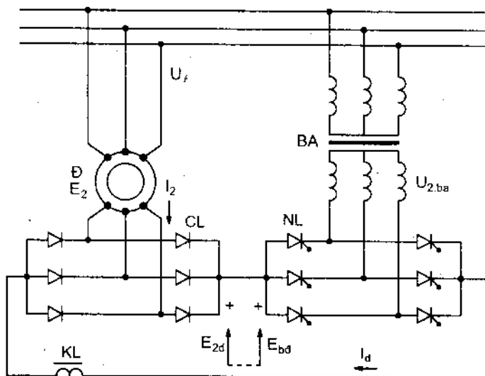
Hình 4 - 28. Sơ đồ tăng điện
