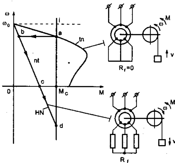
Hình 2 - 33. Hãm ngược nhờ tải trọng (hạ tải) thực hiện bằng cách nối điện trở phụ vào mạch roto (đoạn cd) dùng cho động cơ roto dây quấn
