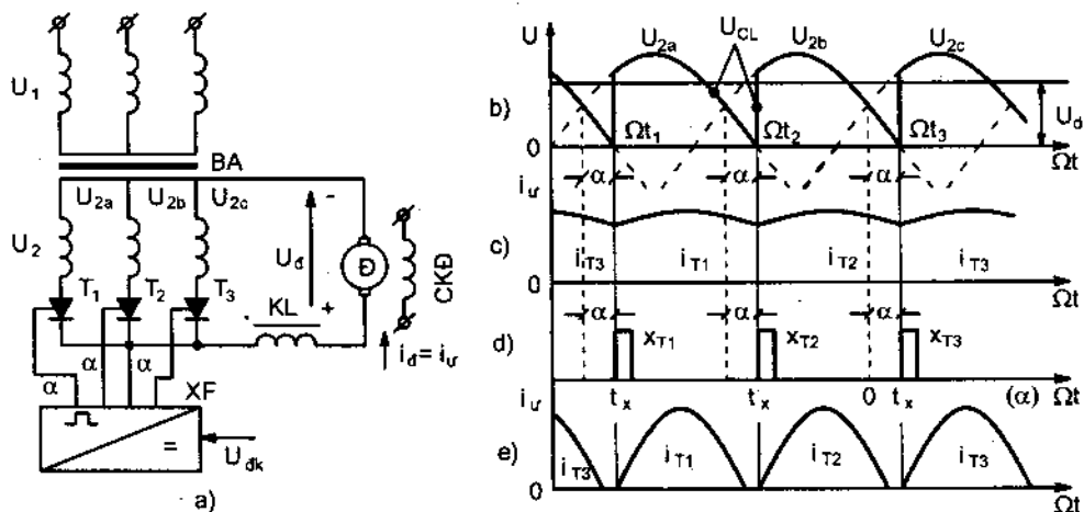
Hình 4-3. Sơ đồ nguyên lý (a) và các đồ thị điện áp, dòng điện (b,c,e) và xung mở van (d) của hệ CL-D không đảo chiều
