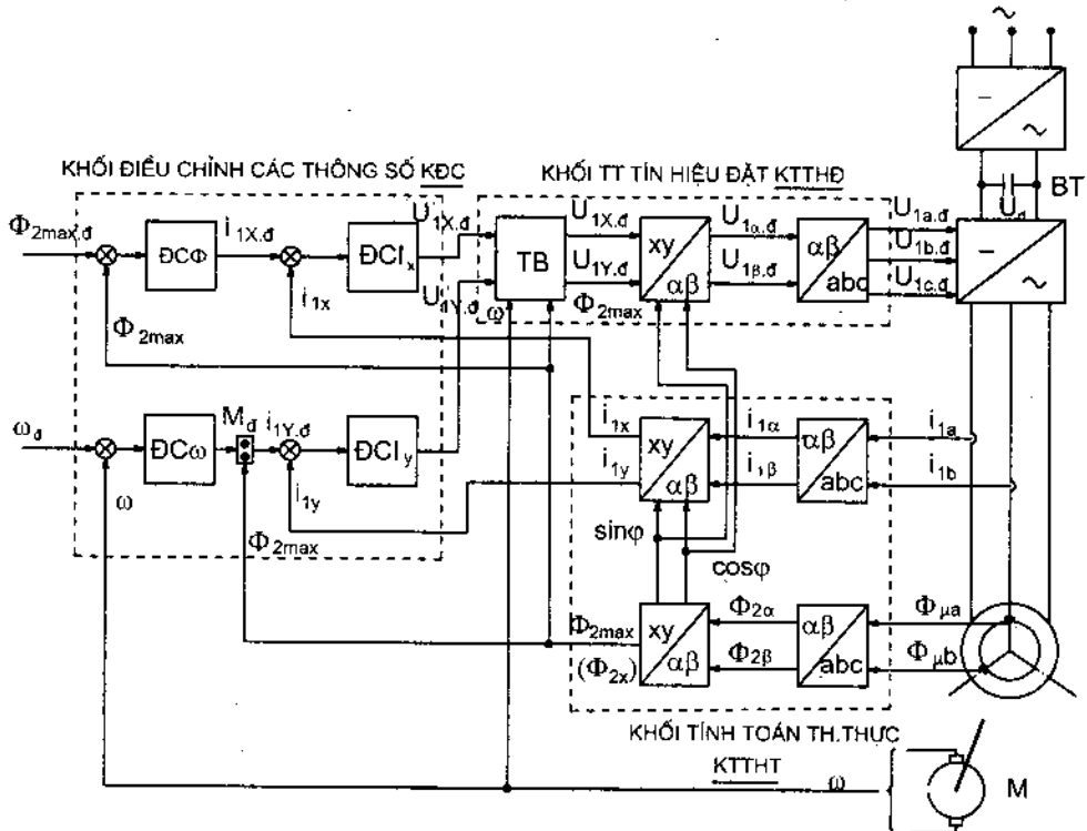
Hình 4 - 25. Sơ đồ khối (nguyên lý) của hệ BT-ĐKĐB có điều khiển vector duy trì từ thông \Phi_{2\max} và dùng cảm biến từ thông (Hệ thống Transvector)
