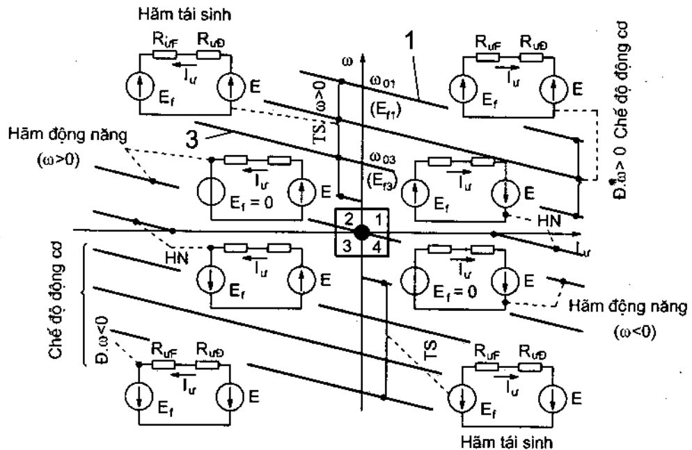
Hình 4 - 2. Đặc tính cơ và sơ đồ thay thế của hệ F - Đ đảo chiều (bốn góc phần tư)
