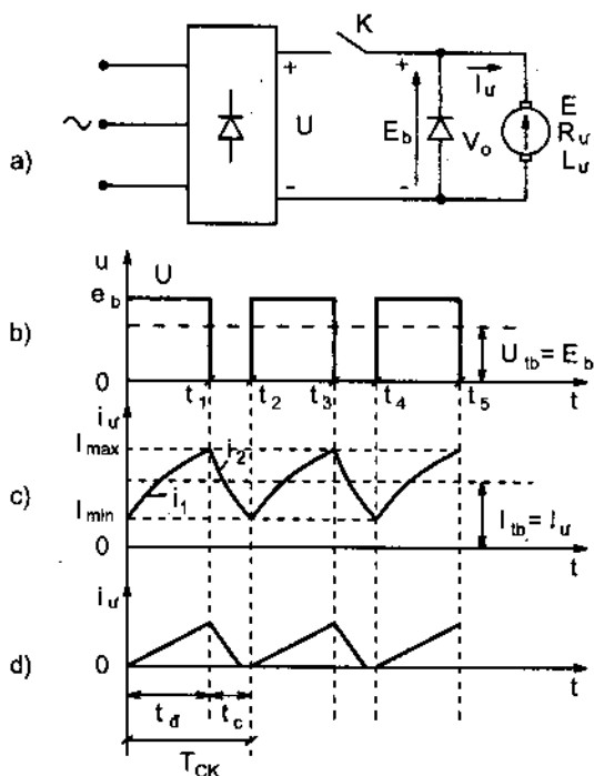
Hình 4 - 16. a) Sơ đồ nguyên lý hệ ĐAX - Đ;
