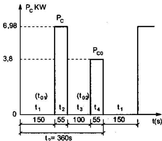
Hình 6 - 8. Đồ thị phụ tải tính của truyền động xe trục
