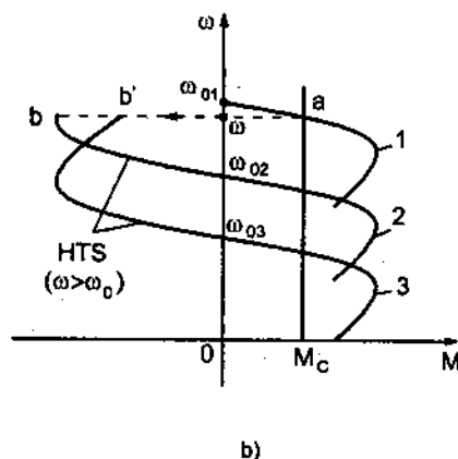
Hình 2 - 32. Các đặc tính cơ của động cơ không đồng bộ khi hãm tái sinh
