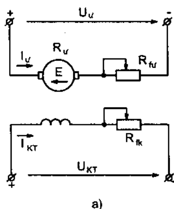
Hình 2 - 1. a) Sơ đồ nối dây của động cơ kích từ độc lập ; b) Sơ đồ nối dây của động cơ kích từ song song.
