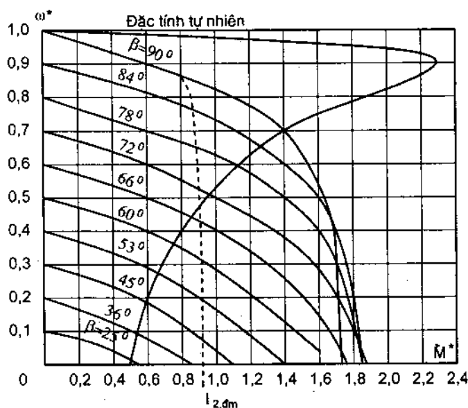
Hình 4 - 29. Họ đặc tính cơ của động cơ 100kW - 1450vòng/ph - 380V nối theo sơ đồ tăng điện
