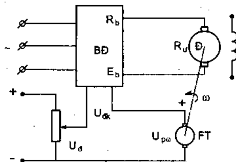
Hình 3 - 29. Sơ đồ nguyên lý hệ Bộ biến đổi - Động cơ điều khiển vòng kín có phản hồi âm tốc độ
