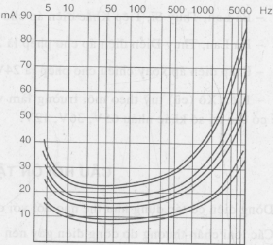
Hình 1-4. Quan hệ giữa dòng điện giạt và tần số
