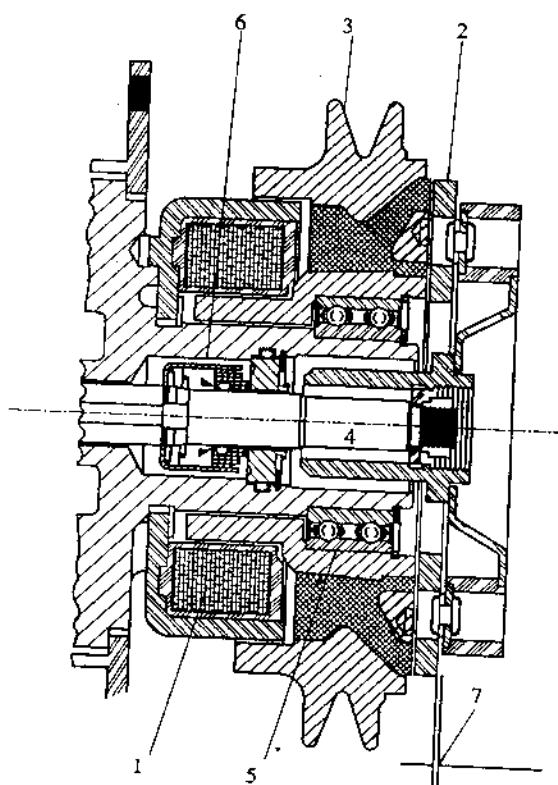
Hình 72. Kết cấu của khớp nối điện từ trang bị trong puly máy nén
