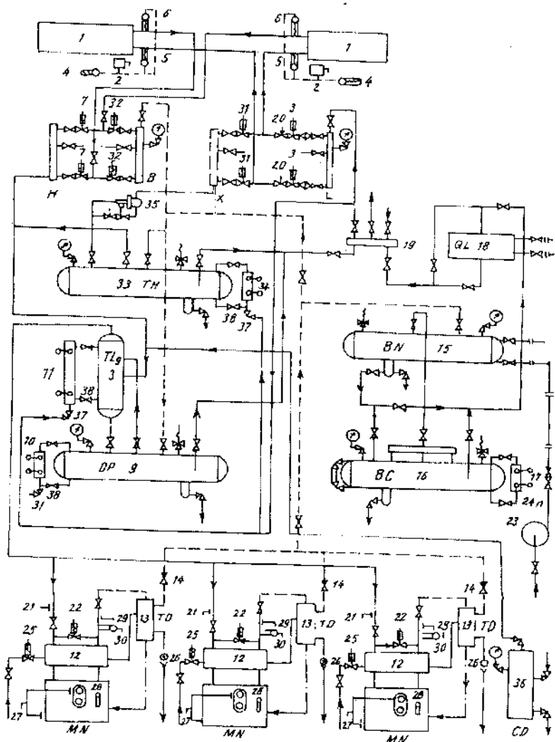
Hình 6-15. Sơ đồ hệ thống lạnh không bơm, bình tách lỏng dưới thấp 1- Dàn bay hơi; 2- Rơ le nhiệt độ; 3 - Van điện từ; 4,5,6 - Nhiệt kế điện trở 7 - Van điện từ; 8 - Bình tách dầu; 9- Bình chứa dự phòng; 10,11- Rơ le mức lỏng bán dẫn; 12- Máy nén; 13- Bình tách dầu; 14- Van 1 chiều; 15- Bình ngưng; 16- Bình chứa cao áp; 17- Mức lỏng kế; 18- Bình quá lạnh; 19- Ống góp; 20- Rơ le áp suất thấp....
