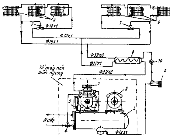
Hình 6.2. Sơ đồ hệ thống lạnh kiểu hở, bình ngưng làm mát bằng nước
