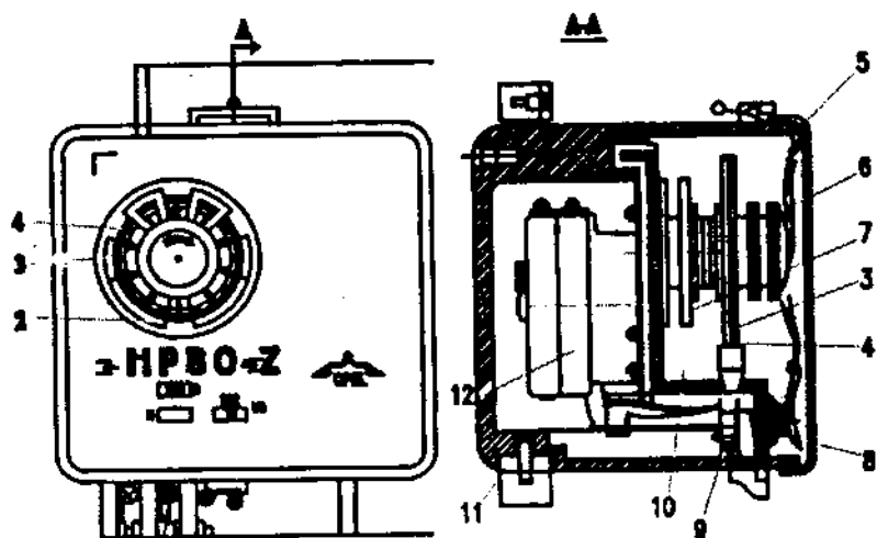
Hình 21. Cấu tạo của rơ le thời gian
