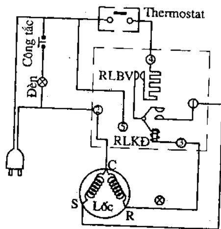
Hình 29. Sơ đồ điện đơn giản của tủ lạnh dùng role khởi động kiểu XP không lắp trực tiếp trên block
