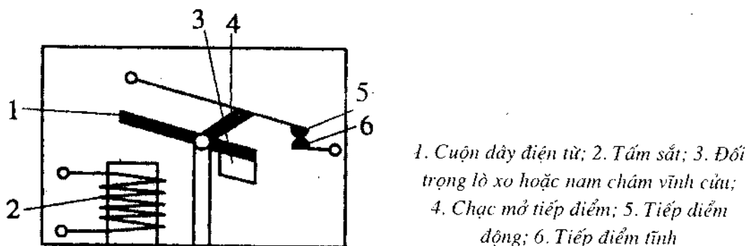
Hình 11. Nguyên tắc cấu tạo của role điện áp
