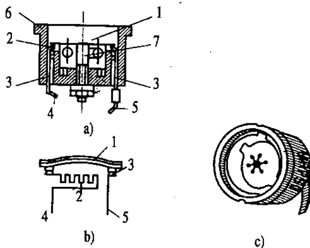
Hình 5: Role bảo vệ kiểu rời
