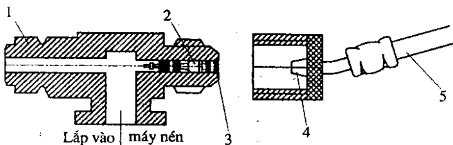
Hình 71. Van một chiều trong đầu nối
