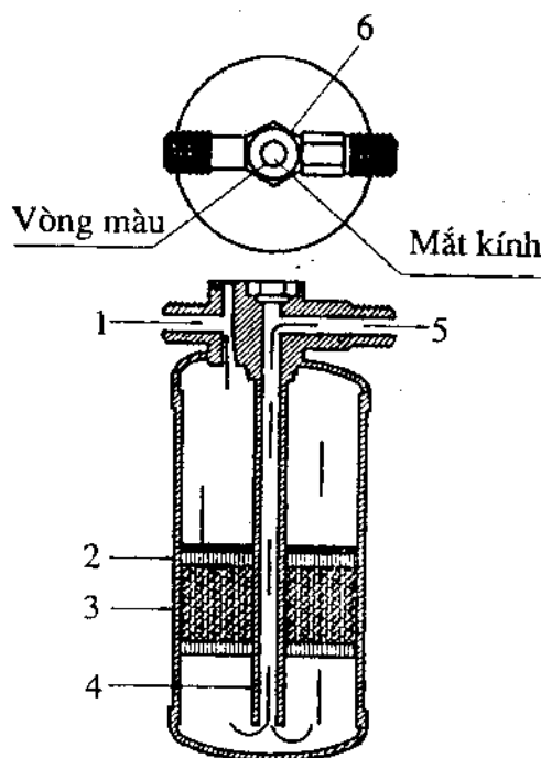
Hình 75. Kết cấu của bình lọc, hút ẩm 1. Tờ dàn ngưng đến; 2. Lưới lọc; 3. Hạt khô ẩm; 4. Ống tiếp nhận; 5. Đến van giãn nở; 6. Mắt ga
