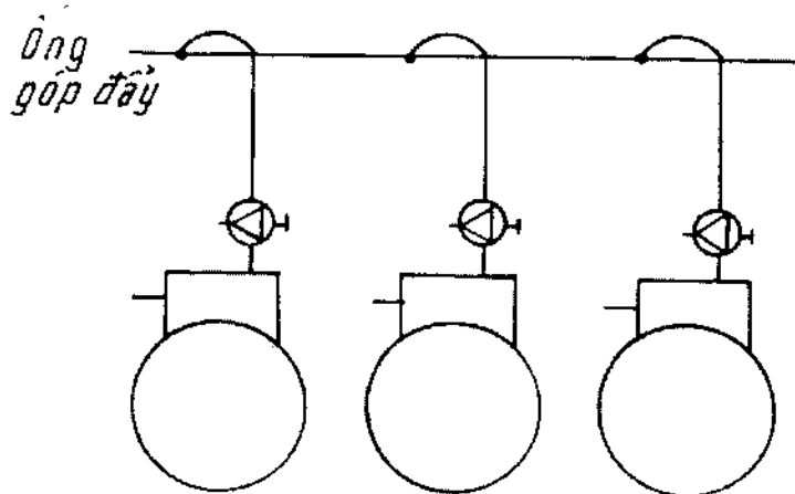
Hình 8-5. Ống góp đặt cao
