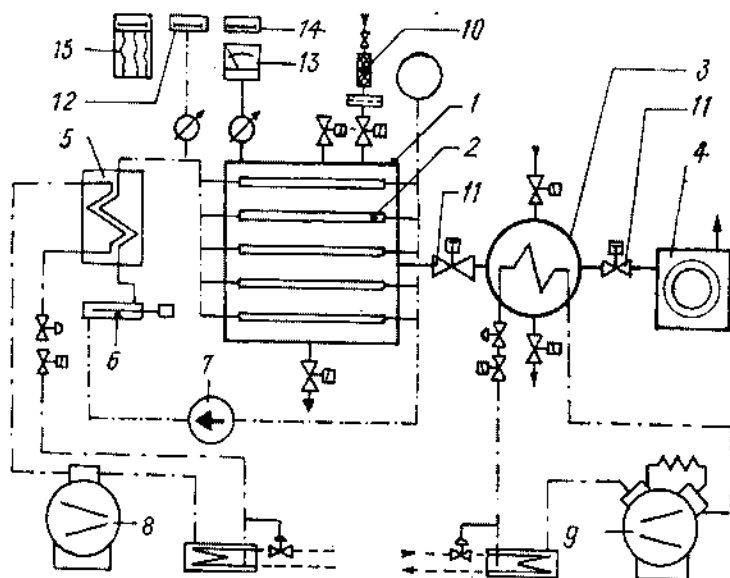
Hình 7.15. Sơ đồ một thiết bị sấy thăng hoa (hãng Leybold Heraeus)
