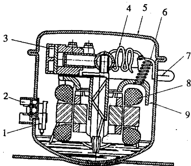
Hình 24b. Máy nén PW của Hãng DANFFOSS (Đan Mạch)
