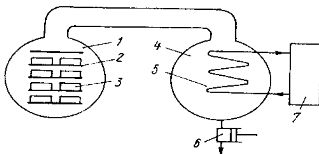
Hình 7.14. Nguyên lý cấu tạo của thiết bị sấy thăng hoa
