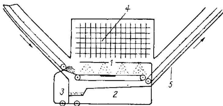
Hình 7.10. Thiết bị kết đông dùng R12 lỏng
