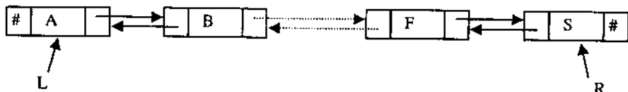
Hình 3.12. Hình ảnh của danh sách nối kép trong bộ nhớ.
