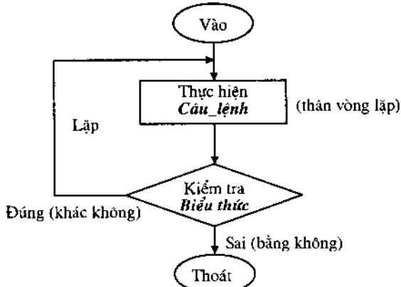
Hình 2.5. Sơ đồ hoạt động của toán tử do ... while.
