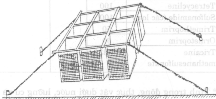
3. Bố cục tổ hợp lồng nuôi trong vịnh
