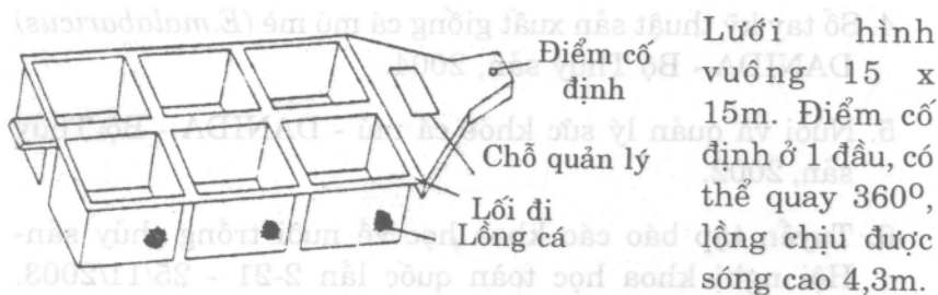
10. Tổ hợp kiểu lồng lưới hình vuông
