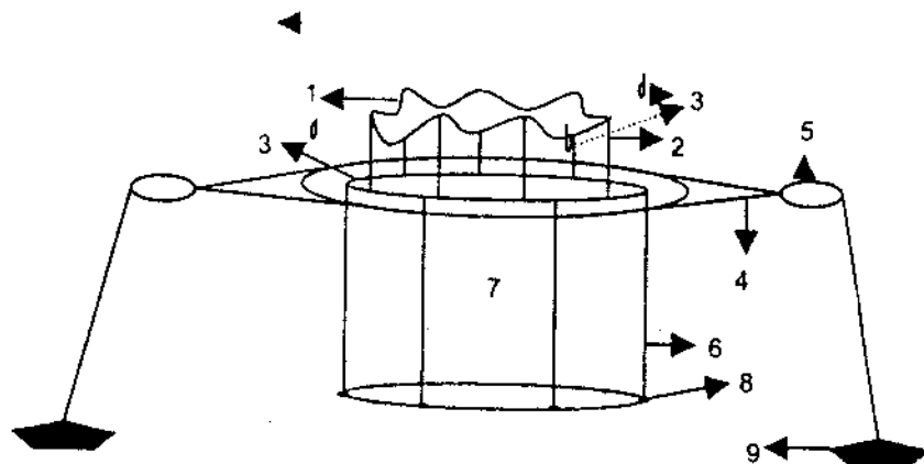
Hình 13. Lồng nuôi cá hình tròn (kiểu NaUy)
