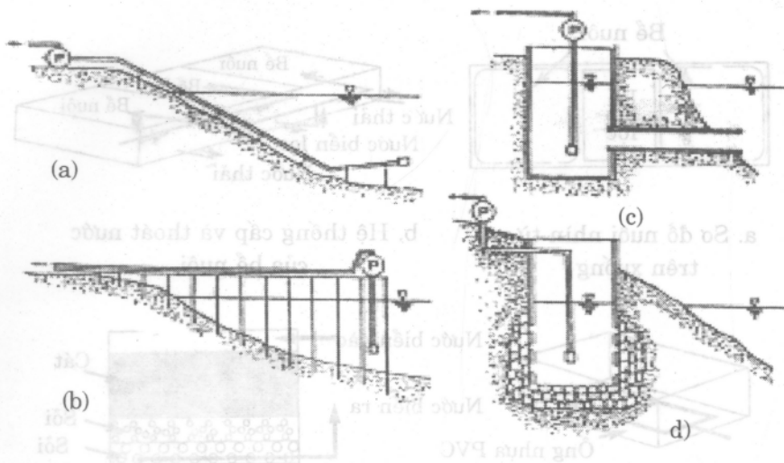
Hình 5. Hệ thống lấy nước biển (a) và (b) bơm trực tiếp (c) Bơm từ nước biển trong hố (d) Bơm nước biển từ 1 cái giếng
