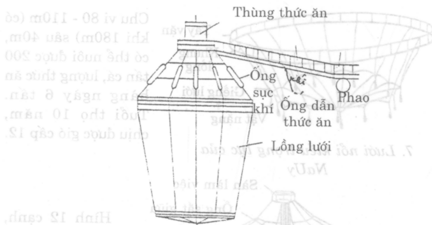
5. Lồng nuôi cá kiểu nổi
