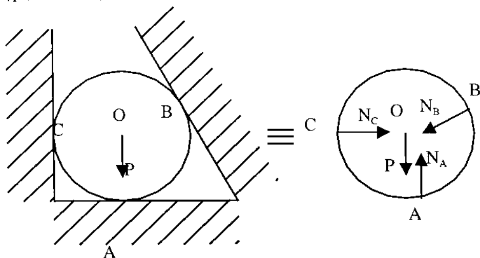
Hình 1.10. Phản lực tác dụng lên vật
