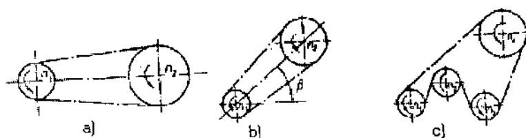
Hình 1.6. Các kiểu bộ truyền xích
