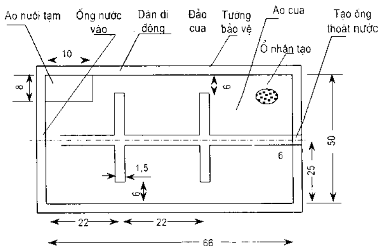
Hình 15. Sơ đồ thiết kế ao nuôi cua (mặt bằng)
