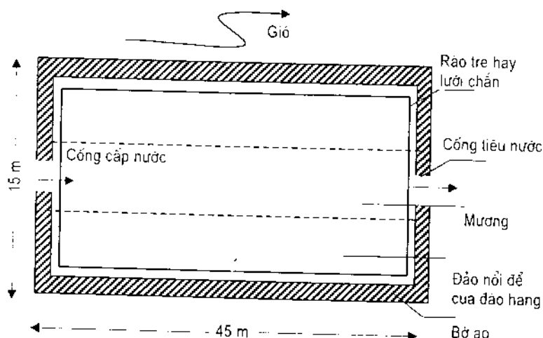
Hình 20. Sơ đồ ao nuôi cua thịt nhìn từ trên xuống
